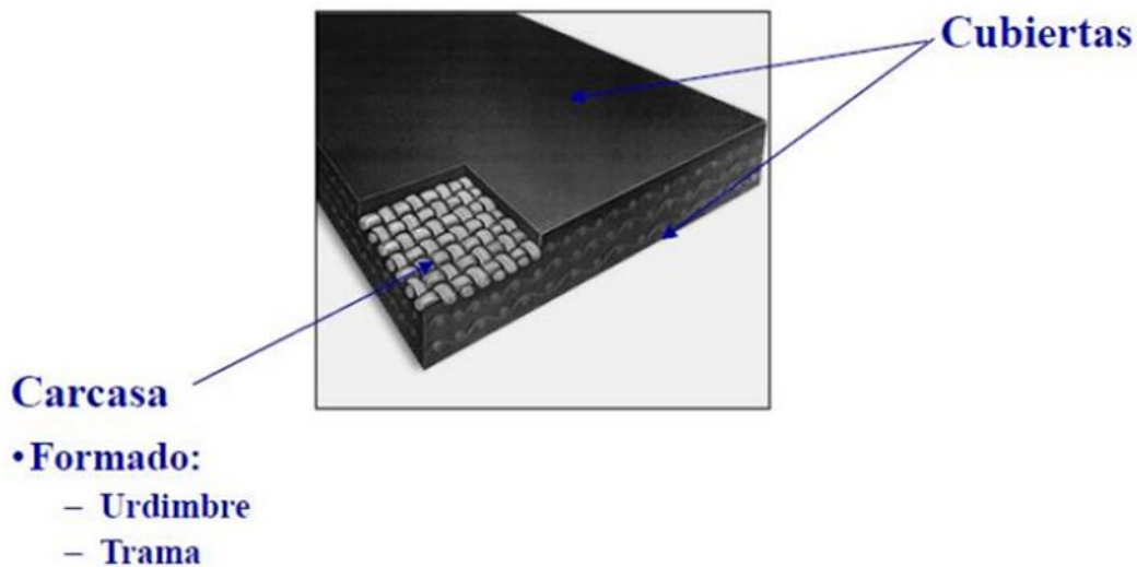
Imagen 2- 33 Componentes de una Banda.
