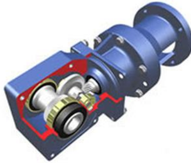
Imagen 2- 15 Conjunto Motorreductor HYPONIC.
