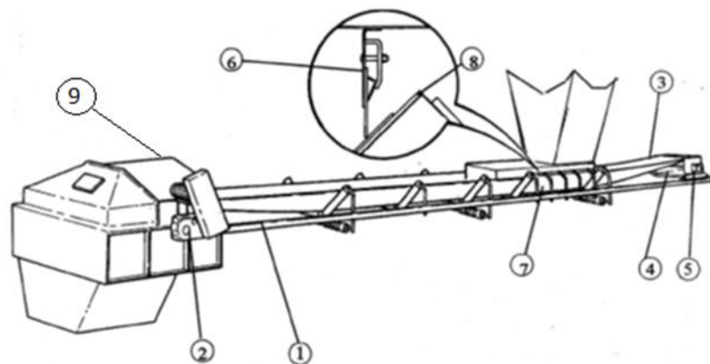
Imagen 2- 7 Esquema Cinta Transportadora.
