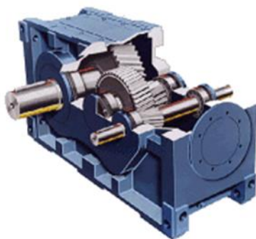
Imagen 2- 21 Reductor DRIVE ONE.
