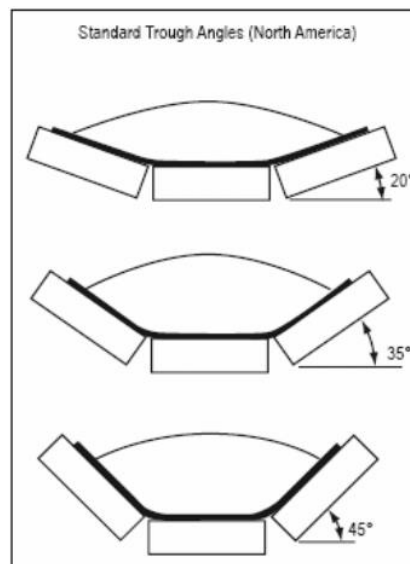
Imagen 2- 28 Inclinación De Instalación Polines De Carga.
