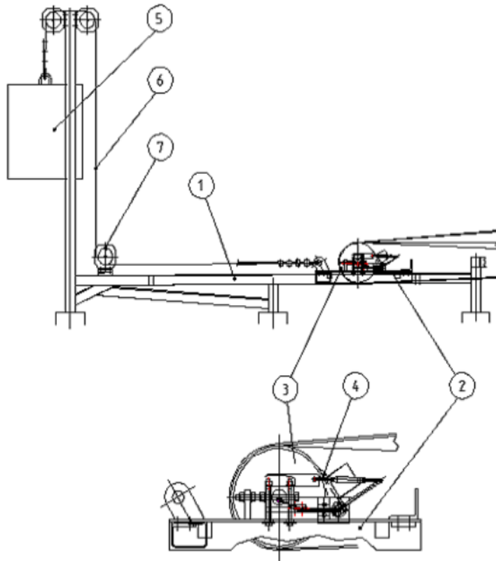
Imagen 2- 34 Esquema Mecanismo Tensado.
