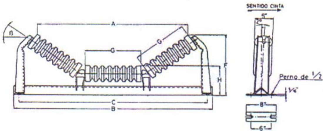
Imagen 2- 31 Polines de Impacto.
