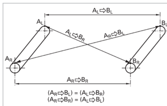
Imagen 3- 1 Método de Comprobación para Instalación.
