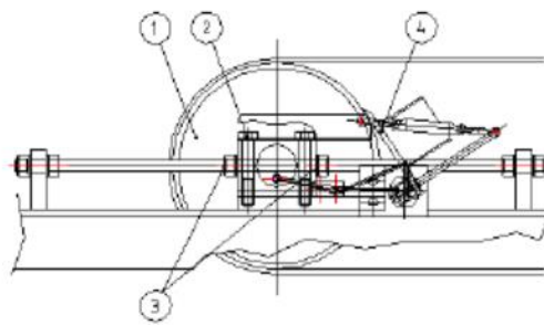
Imagen 2- 34 Esquema Mecanismo Tensado Horizontal
