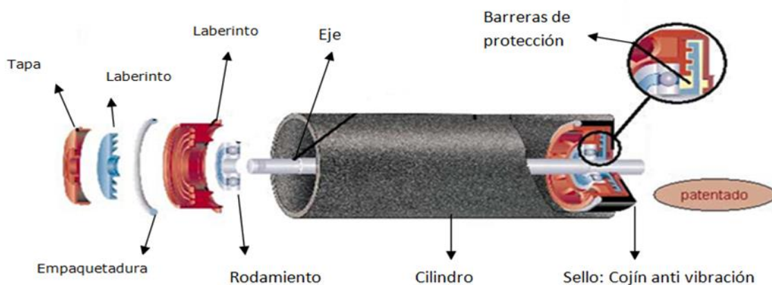
Imagen 2- 29 Vista en Corte de Polín de Carga.
