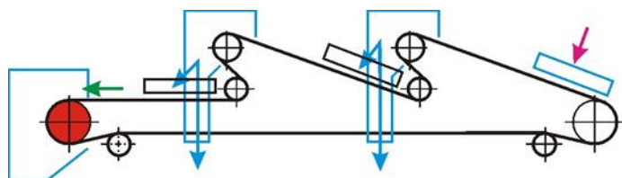
Imagen 2- 4 Esquema De Cinta Con Tripper Fijo.
