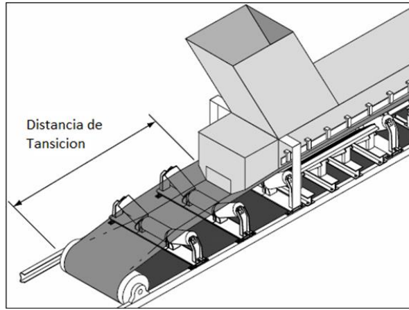
Imagen 2- 36 Zona de Transición.
