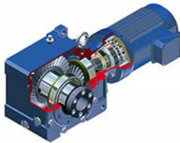
Imagen 2- 14 Reductor De Ciclo Cónico.
