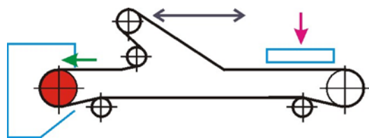
Imagen 2- 3 Esquema de Cinta con Tripper Móvil.
