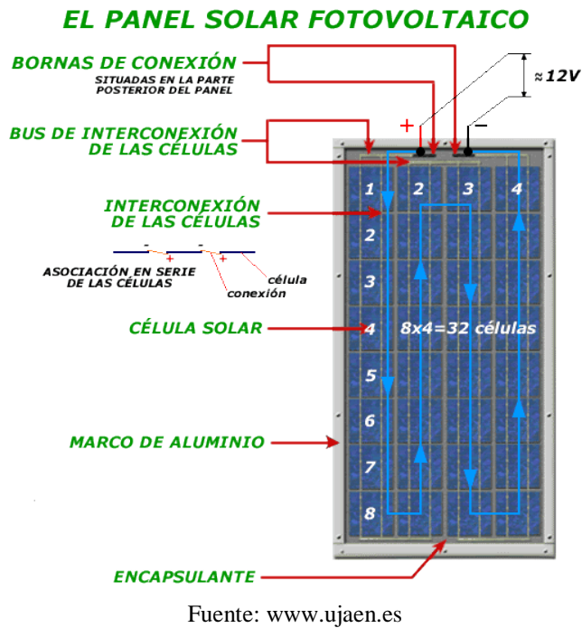
Figura 1-8. Vista frontal de los elementos de los paneles solares.
