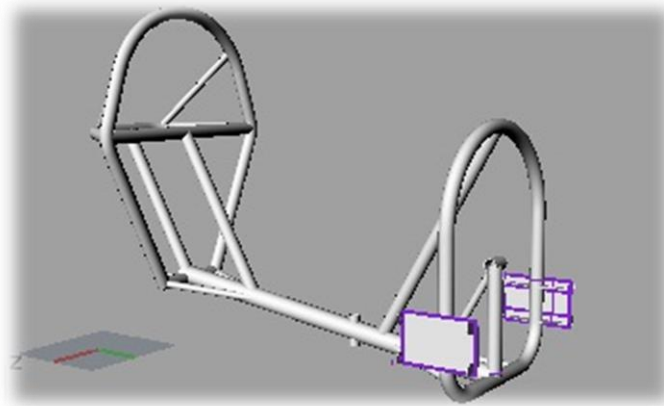
Ilustración 7: Chasis de perfil tubular de acero 1020
