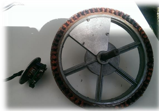
Ilustración 14: Controlador y estator, partes de esenciales del motor
