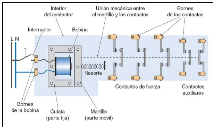
Ilustración 19: Diagrama de funcionamiento de un contactor
