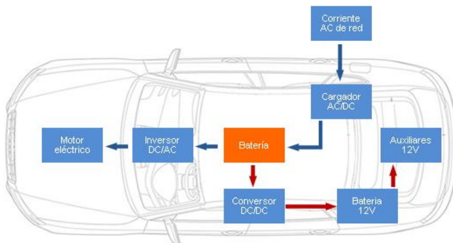
Ilustración 4: Esquema de componentes principales de un vehículo eléctrico
