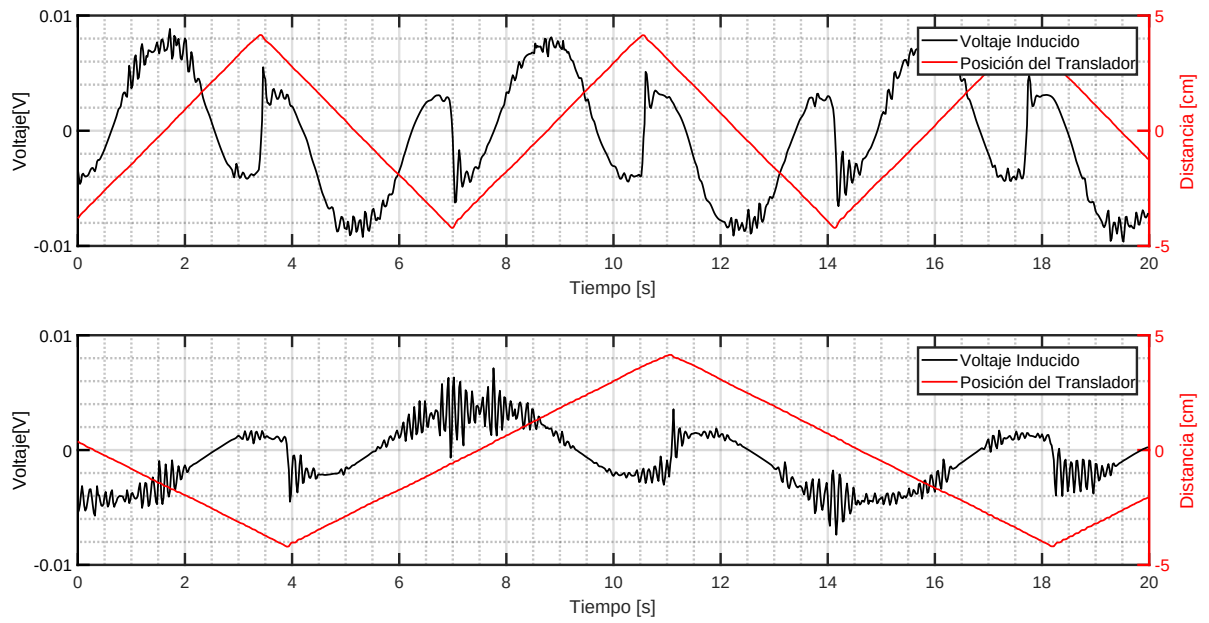
Figura B.2: 1x2 : Voltaje Inducido y Posición con T_s=7.28[s] y T_s=14.28[s]
