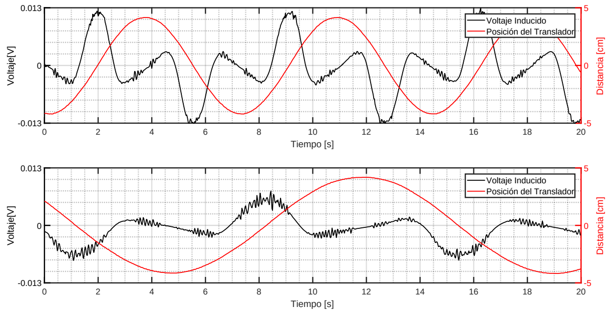
Figura 5.17: 1x2 : Voltaje Inducido y Posición con Período 14.28[s] y 7.14[s]
