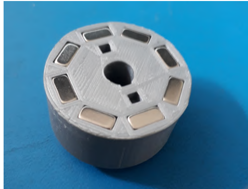
Figura 4.4: Traslador B Impreso y con Imanes Incrustados
