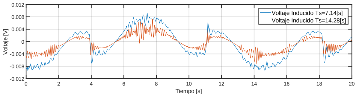
Figura B.8: 1x2 : Voltajes Inducidos por Referencias Triangulares y de Diferentes Períodos
