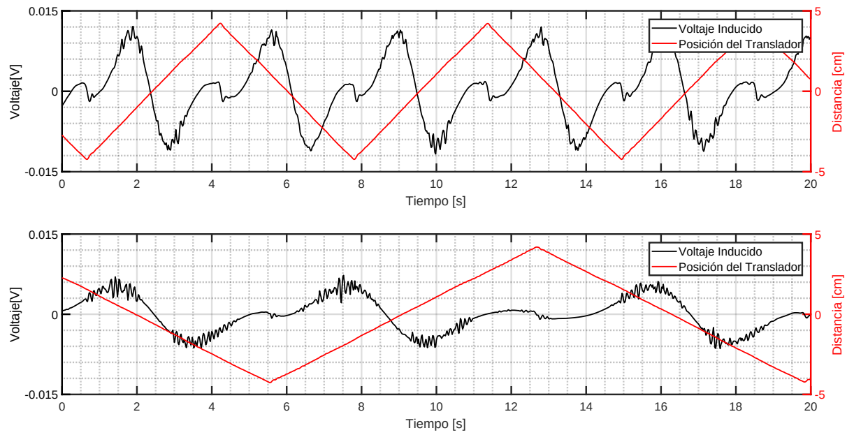
Figura B.4: 2x1 NS : Voltaje Inducido y Posición con T_s=7.28[s] y T_s=14.28[s]
