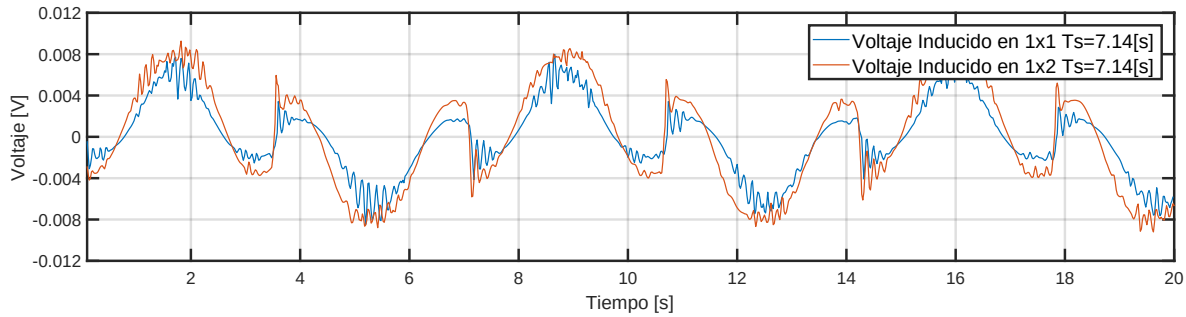
Figura 6.8: Comparación del Voltaje Inducido con Referencia Triangular de las Configuraciones 1x2 y 1x1
