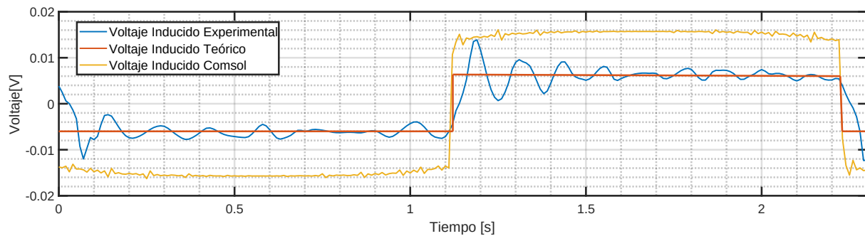
Figura 6.13: Comparación del Voltaje Inducido
