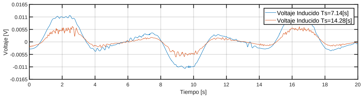
Figura 6.3: 2x1 NN : Voltajes Inducidos por Referencias Sinusoidales y de Diferentes Períodos
