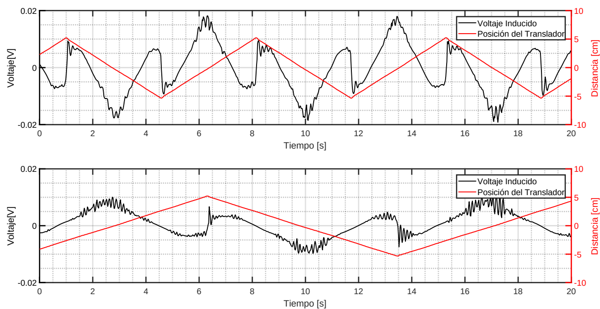
Figura B.6: 2x2 NN : Voltaje Inducido y Posición con T_s=7.28[s] y T_s=14.28[s]
