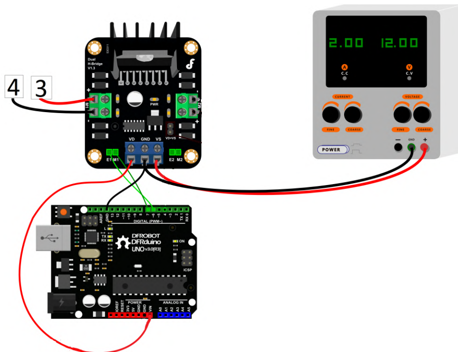
Figura 5.5: Conexiones entre el Driver y el Motor Actuonix
