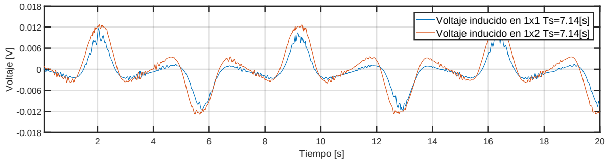
Figura 6.7: Comparación del Voltaje Inducido con Referencia Sinusoidal de las Configuraciones 1x2 y 1x1
