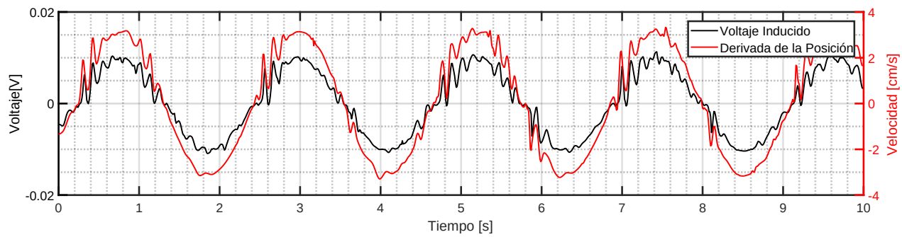
Figura 6.11: Comparación del Voltaje Inducido con la Velocidad del Traslador con Desplazamiento Sinusoidal
