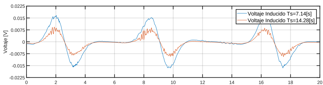
Figura 6.5: 2x1 NS : Voltajes Inducidos por Referencias Sinusoidales y de Diferentes Períodos
