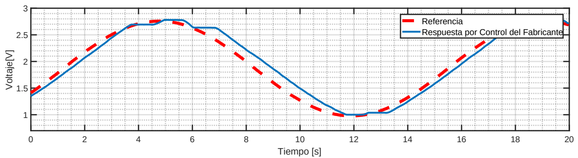
Figura 5.12: Seguimiento de la Referencia del Controlador del Fabricante
