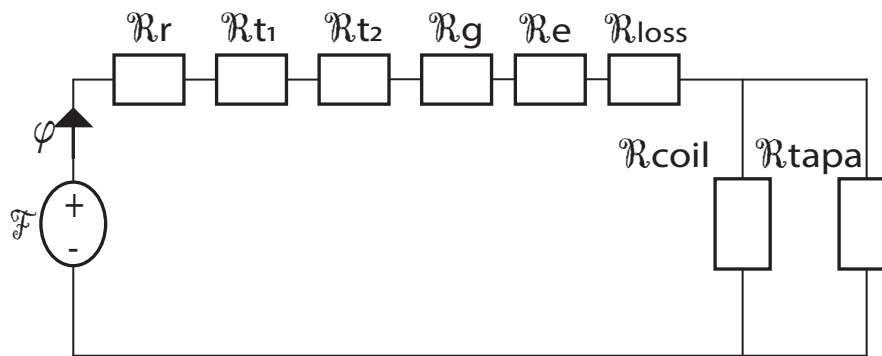
Figura 3.3: Circuito Magnético
