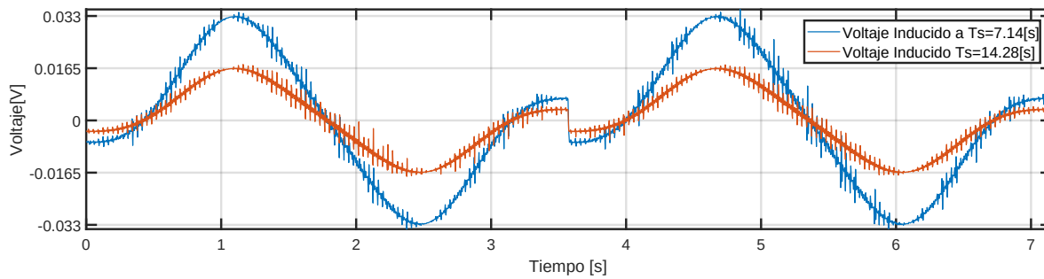
Figura 3.27: 2x2 NS : Comparación de Voltajes Inducidos por Referencias de Posición Triangulares
