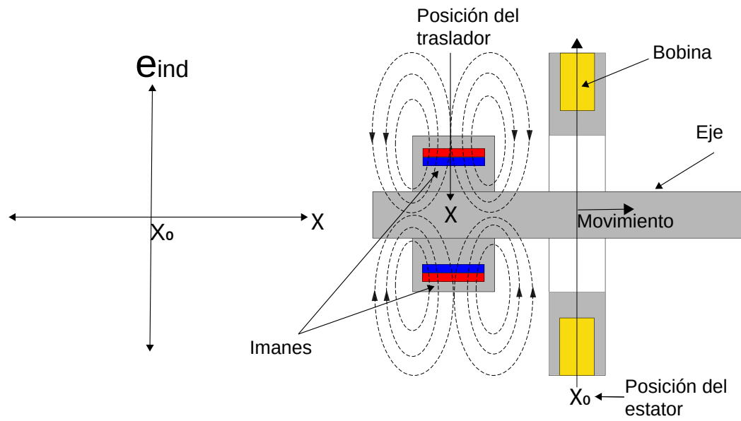
Figura 3.7: Configuración 1x1 del Generador Lineal
