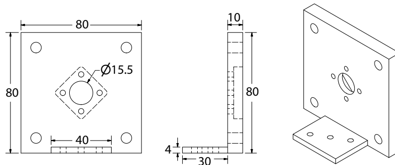
Figura 4.8: Esquema de la Tapa Sostenedora del Riel Metálico
