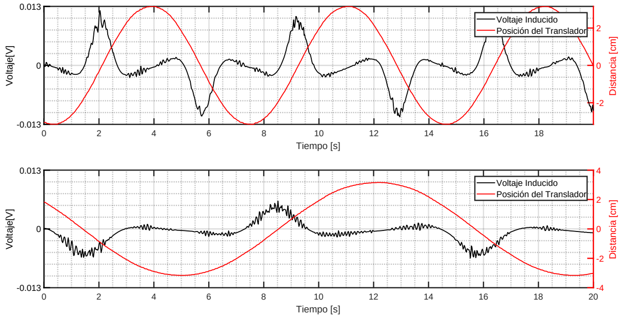
Figura 5.16: 1x1 : Voltaje Inducido y Posición con Período 14.28[s] y 7.14[s]
