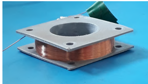
Figura 4.7: Estator Bobinado
