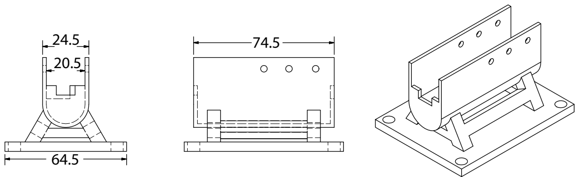
Figura 4.10: Esquema del Soporte del Motor Actuonix
