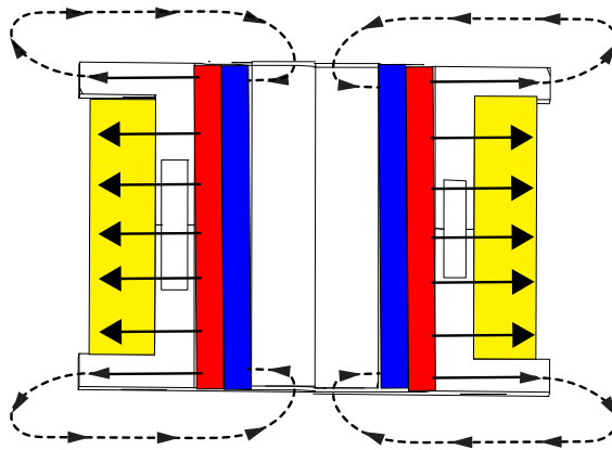
Figura 3.2: Vista Lateral: Líneas de Campo Magnético en el Traslador
