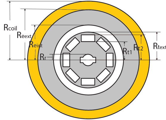
Figura 3.4: Radios de las Reluctancias
