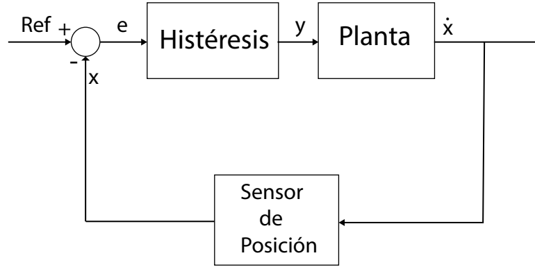
Figura 5.9: Diagrama de Control de Histéresis
