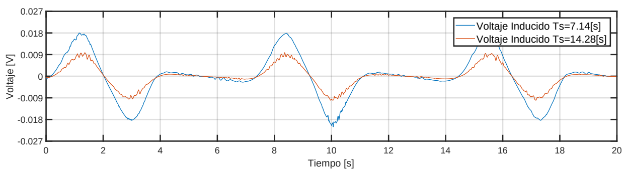
Figura 6.6: 2x2 NS : Voltajes Inducidos por Referencias Sinusoidales y de Diferentes Períodos
