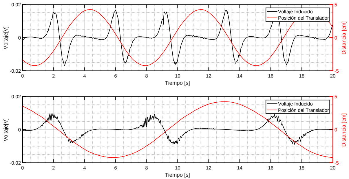
Figura 5.20: 2x1 NS : Voltaje Inducido y Posición con Período 14.28[s] y 7.14[s]
