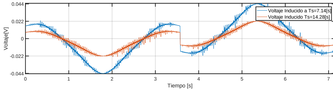
Figura 3.25: 2x2 NN : Comparación de los Voltajes Inducidos por Referencias de Posición Triangulares
