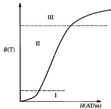
Figura 2.1: Curva B-H
