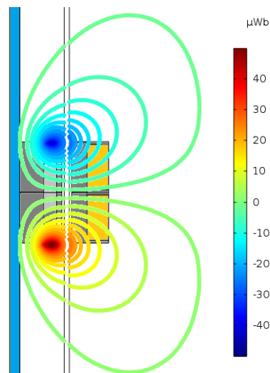
Figura 3.18: Líneas del Flujo Magnético en Configuración 2x2 NN
