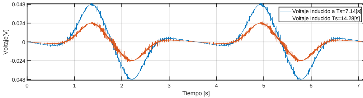
Figura 3.26: 2x2 NS : Comparación de los Voltaje Inducido por Referencias de Posición Sinusoidales
