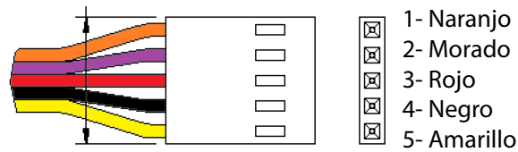
Figura 5.2: Señales del Motor Actuonix
