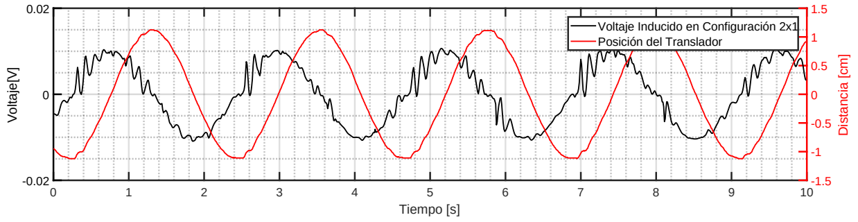
Figura 6.9: Voltaje Inducido por una Referencia Sinusoidal de Frecuencia 450[mHz]
