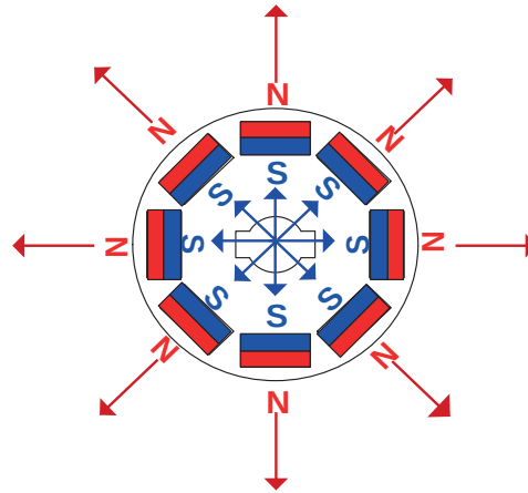
Figura 3.5: Módulo de Traslador Vista Superior
