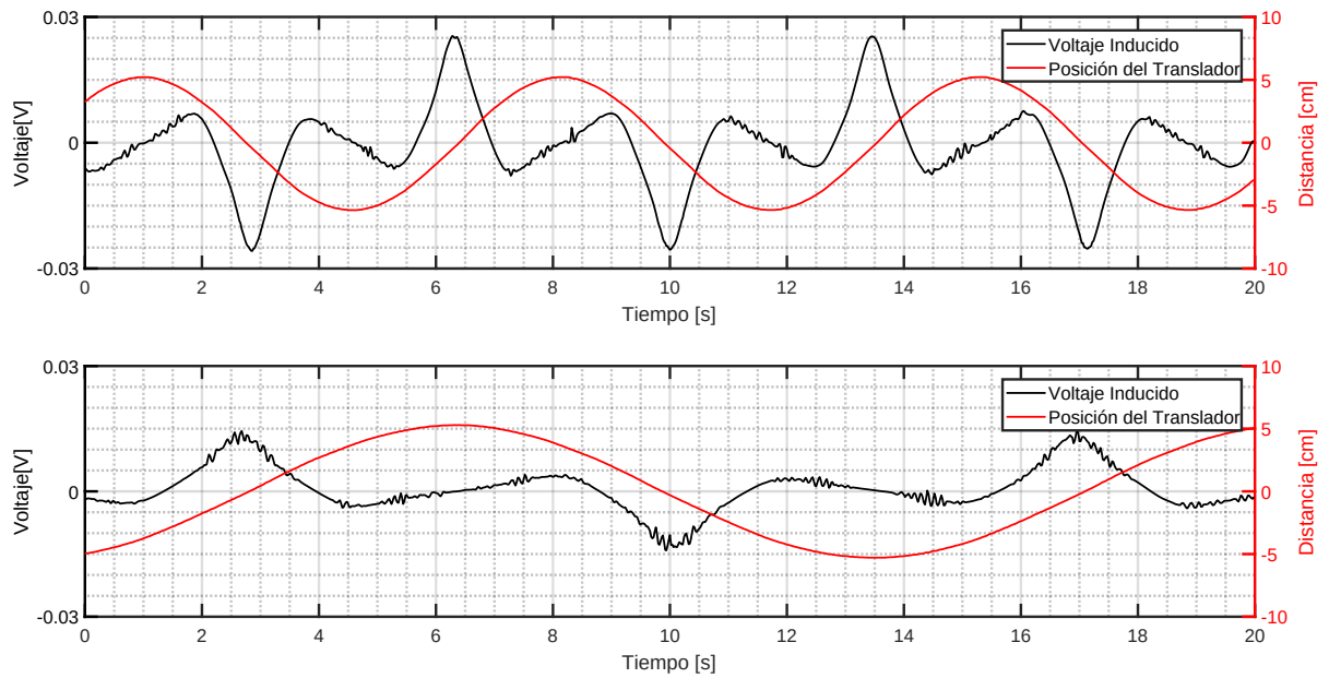
Figura 5.19: 2x2 NN : Voltaje Inducido y Posición con Período 14.28[s] y 7.14[s]
