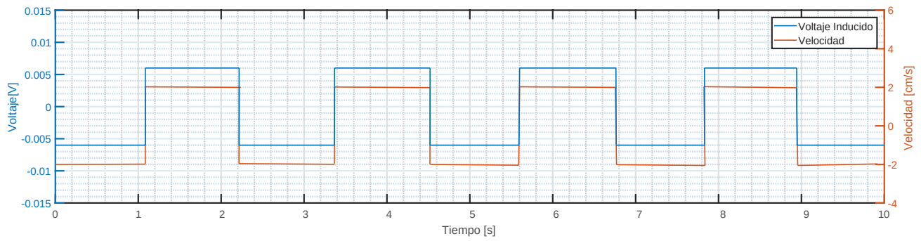
Figura 3.16: Voltaje Inducido Teórico
