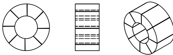
Figura C.1: Anillo de Imanes
