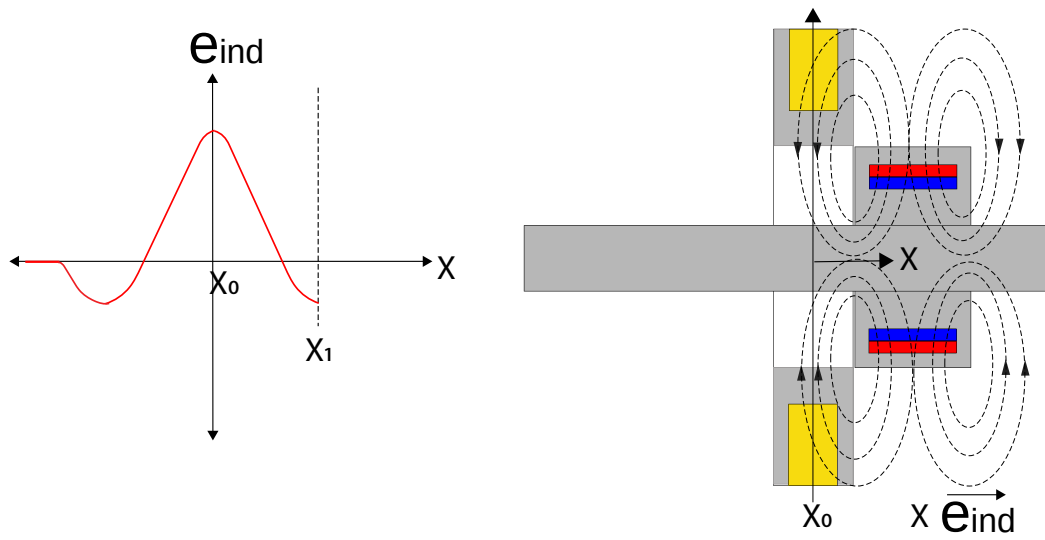
Figura 3.11: Voltaje Inducido en la Configuración 1x1 en la Posición x_1
