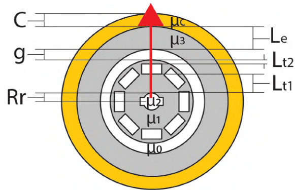
Figura 3.1: Vista Superior: Largos de las Reactancias
