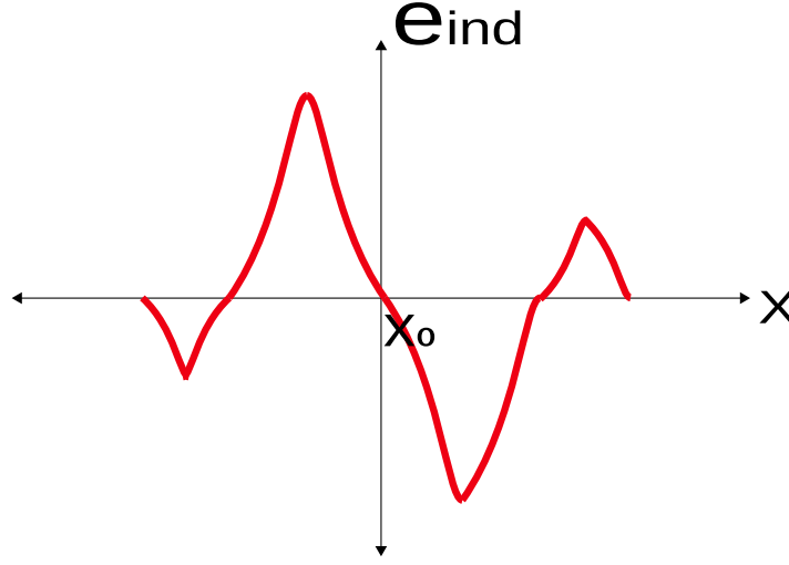
Figura 3.14: Voltaje Inducido en la Configuración 2x2 NS
