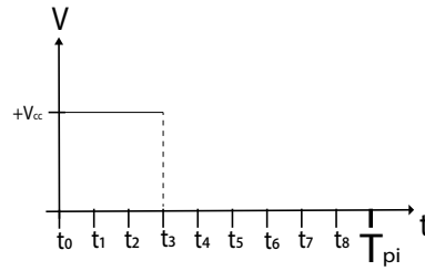
Figura 5.10: Ejemplo del PWM de una actuación de y[k]=0.3
