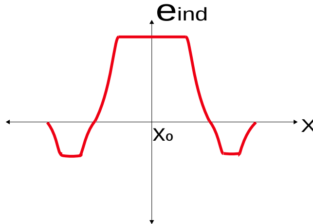
Figura 3.13: Voltaje inducido en la Configuración 2x1 NN
