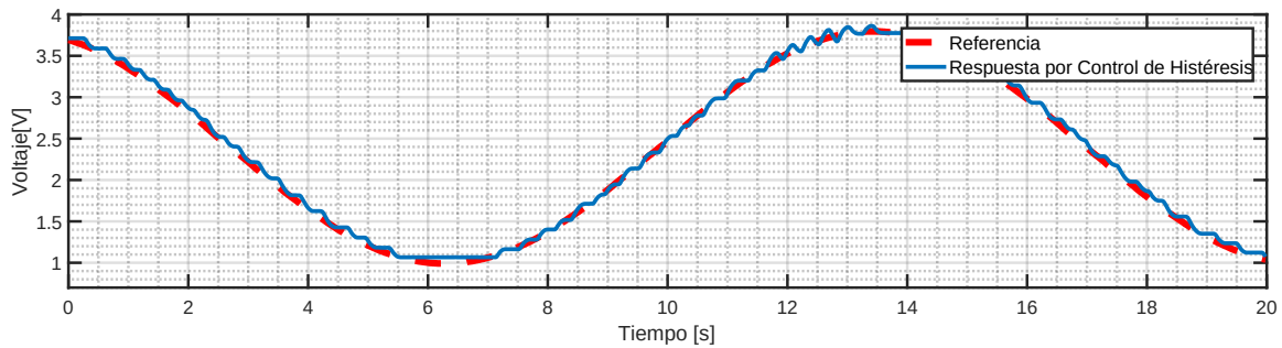
Figura 5.13: Seguimiento de la Referencia del Controlador por Histéresis
