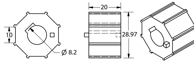
Figura 4.1: Esquema del Traslador A
