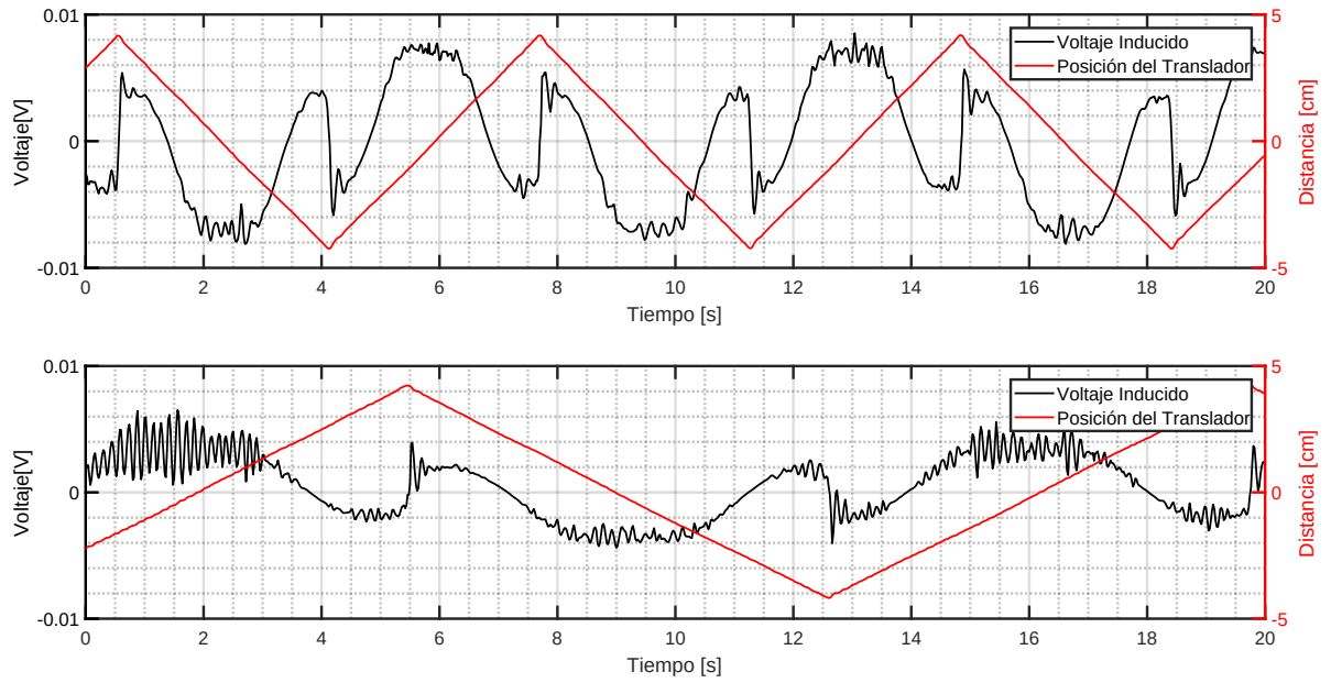
Figura B.3: 2x1 NN : Voltaje Inducido y Posición con T_s=7.28[s] y T_s=14.28[s]
