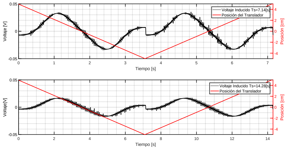
Figura 3.23: 2x2 NS : Voltaje Inducido por Referencias de Posición Triangulares
