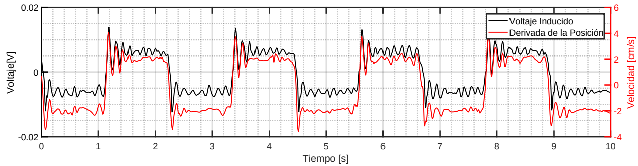
Figura 6.12: Comparación del Voltaje Inducido con la Velocidad del Traslador con Desplazamiento Triangular
