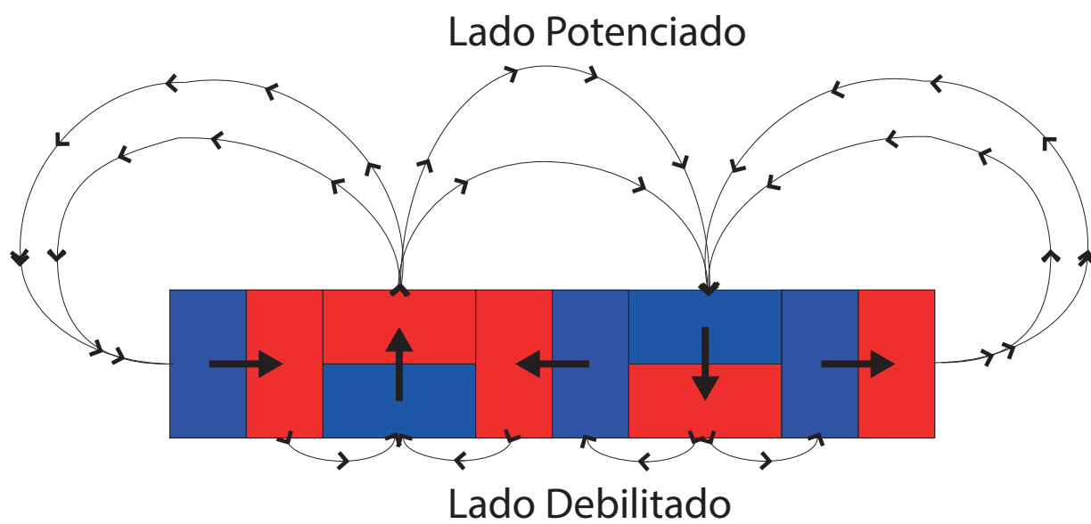
Figura C.4: Configuración Halbach
