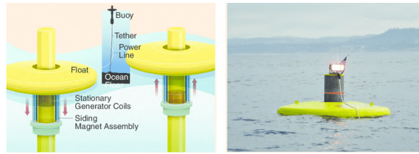
Figura 1.4: Generador lineal de la Universidad de Oregon
