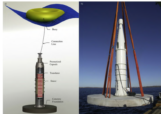
Figura 1.3: Generador lineal de la Universidad Upsala
