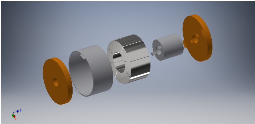
Figura C.2: Piezas del Traslador
