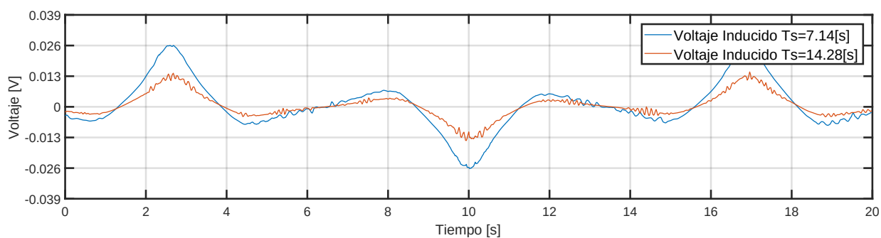
Figura 6.4: 2x2 NN : Voltajes Inducidos por Referencias Sinusoidales y de Diferentes Períodos
