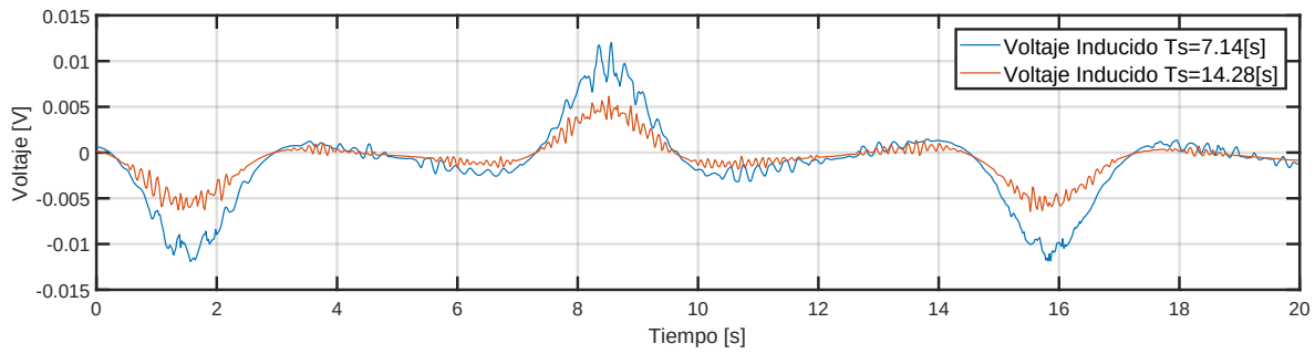
Figura 6.1: 1x1 : Voltajes Inducidos por Referencias Sinusoidales y de Diferentes Períodos
