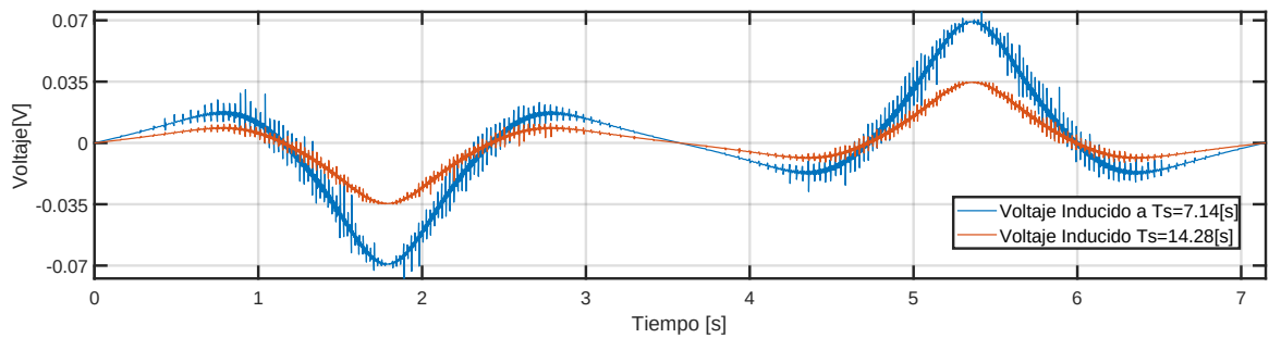
Figura 3.24: 2x2 NN : Comparación de los Voltajes Inducidos por Referencias de Posición Sinusoidales
