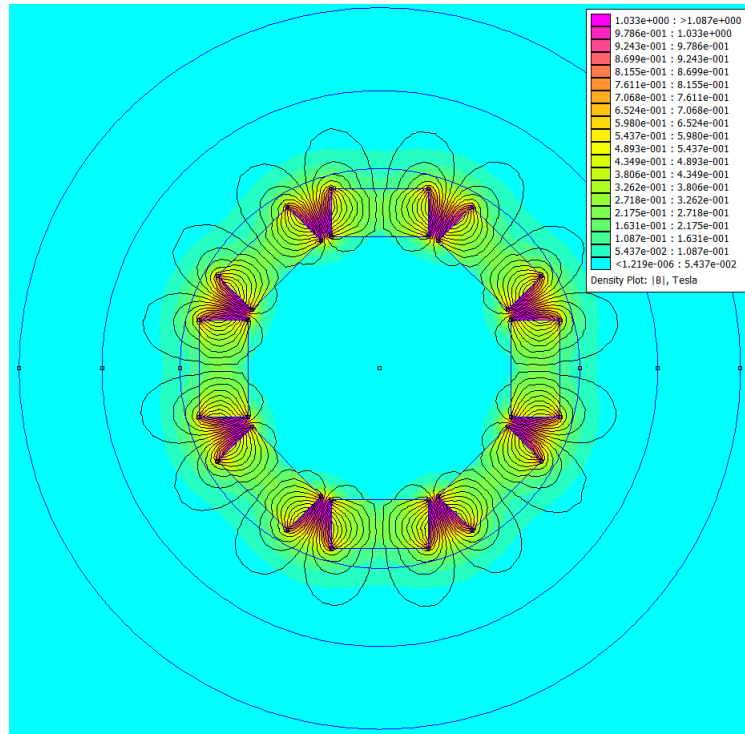
Figura 3.15: Vista Superior del Generador Lineal en FEMM
