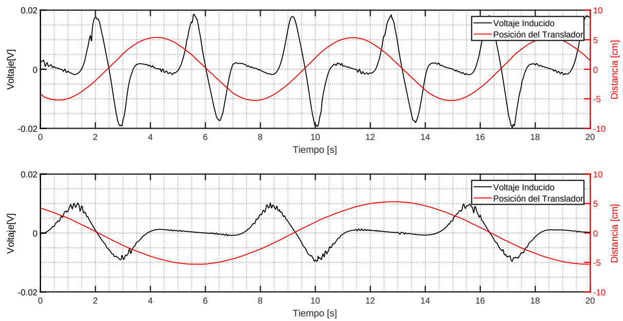
Figura 5.21: 2x2 NS: Voltaje Inducido y Posición con Período 14.28[s] y 7.14[s]
