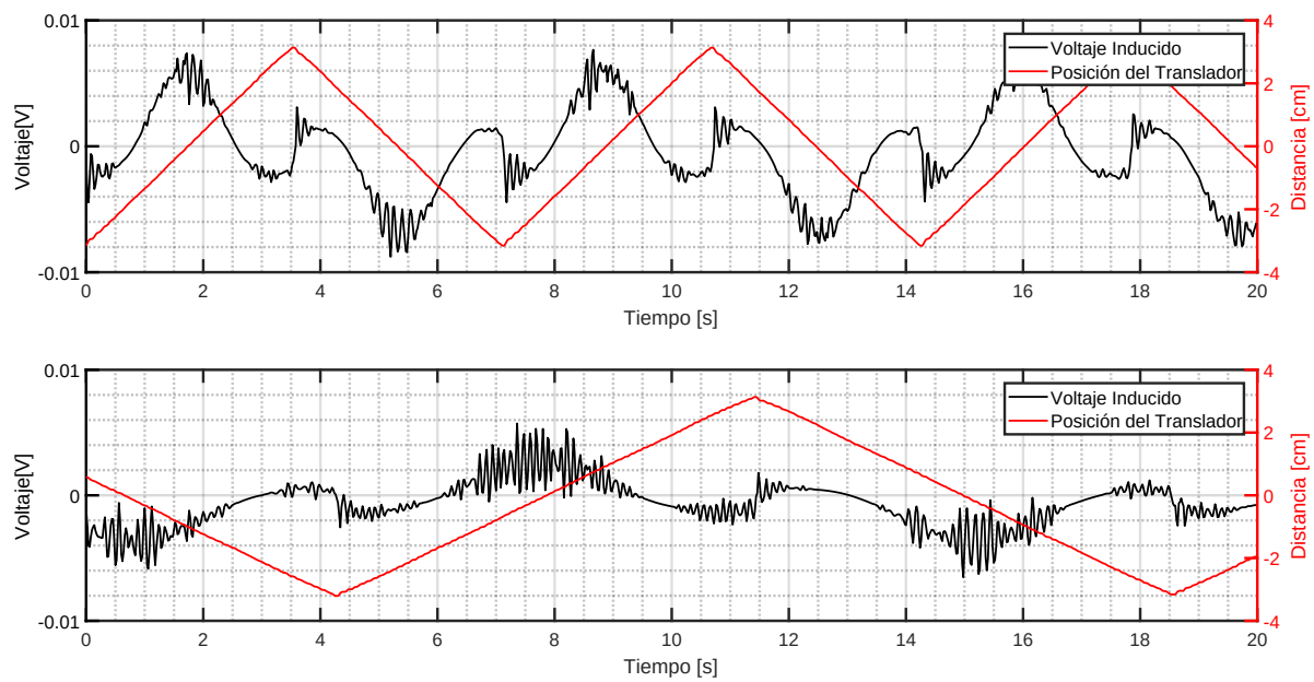
Figura B.1: 1x1: Voltaje Inducido y Posición con T_s=7.28 [s] y T_s=14.28 [s]
