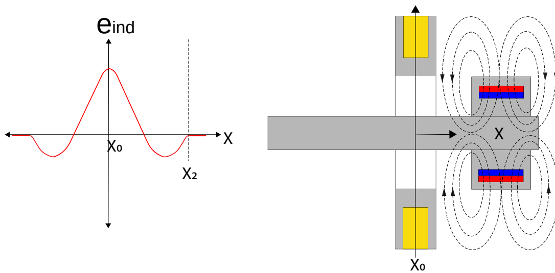
Figura 3.12: Voltaje Inducido en la Configuración 1x1 en la Posición x_2
