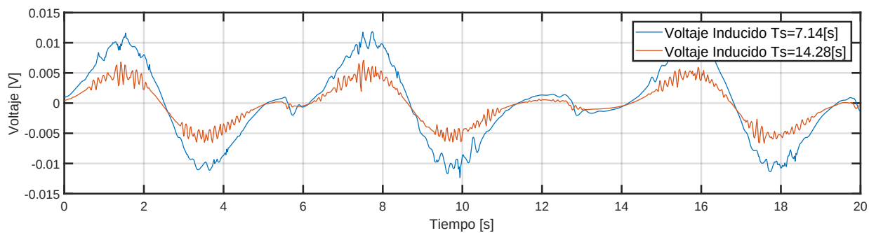
Figura B.11: 2x1 NS : Voltajes Inducidos por Referencias Triangulares y de Diferentes Períodos
