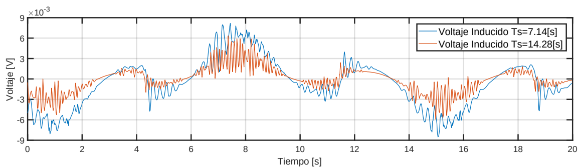
Figura B.7: 1x1 : Voltajes Inducidos por Referencias Triangulares y de Diferentes Períodos
