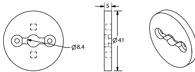
Figura 4.5: Esquema de las Tapas del Estator
