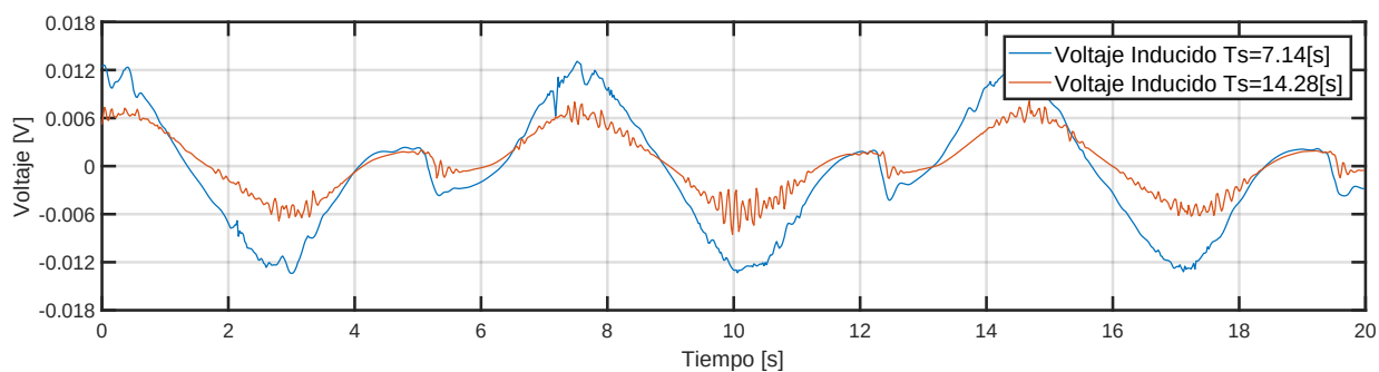
Figura B.12: 2x2 NS : Voltajes Inducidos por Referencias Triangulares y de Diferentes Períodos
