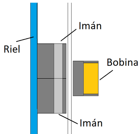
Figura 3.29: Representación en 2D del Generador Lineal 2x1 en Comsol
