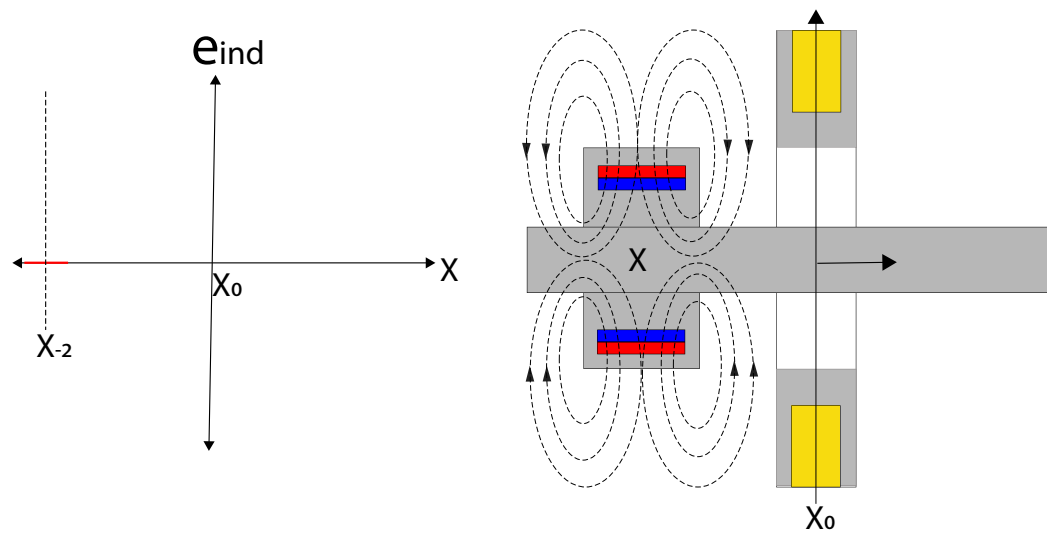
Figura 3.8: Voltaje Inducido en la Configuración 1x1 en la Posición x_{-2}
