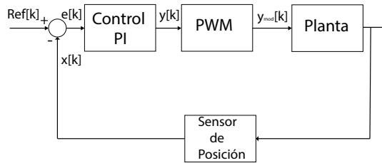
Figura 5.11: Diagrama de Control
