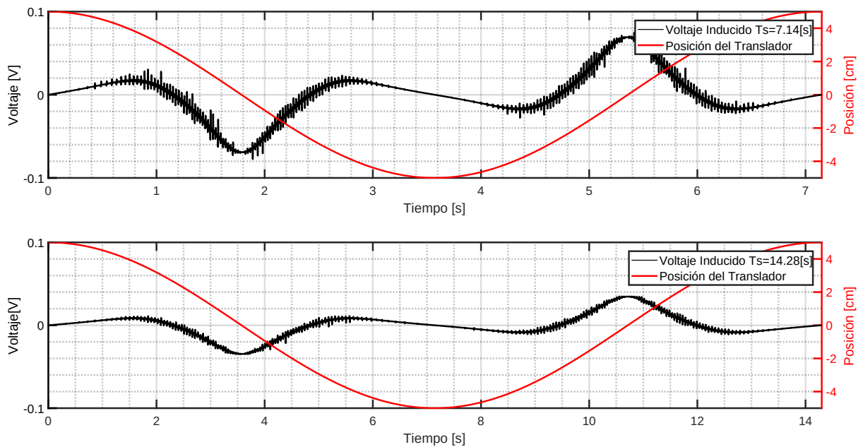
Figura 3.20: 2x2 NN : Voltaje Inducido por Referencias de Posición Sinusoidales
