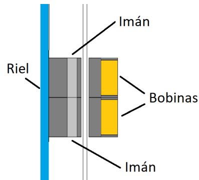
Figura 3.17: Representación en 2D del Generador Lineal 2x2 en Comsol
