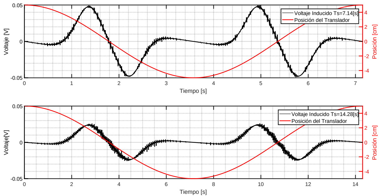
Figura 3.22: 2x2 NS : Voltaje Inducido por Referencias de Posición Sinusoidales
