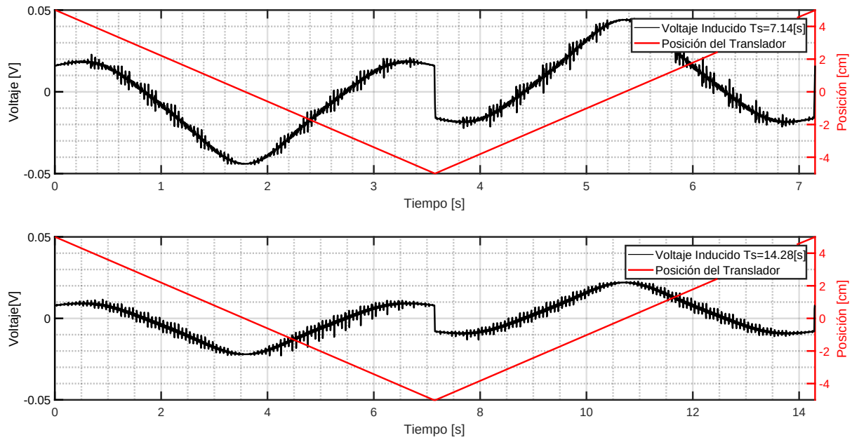
Figura 3.21: 2x2 NN : Voltaje Inducido por Referencias de Posición Triangulares
