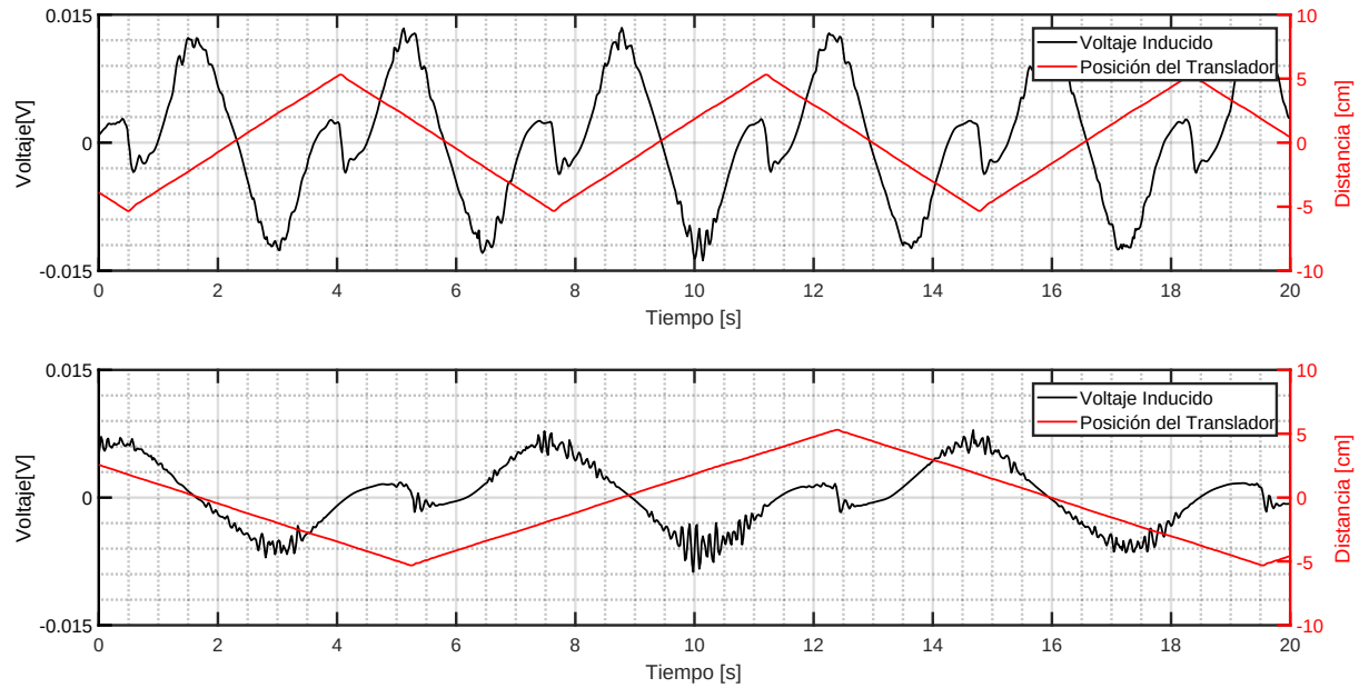
Figura B.5: 2x2 NS : Voltaje Inducido y Posición con T_s=7.28[s] y T_s=14.28[s]
