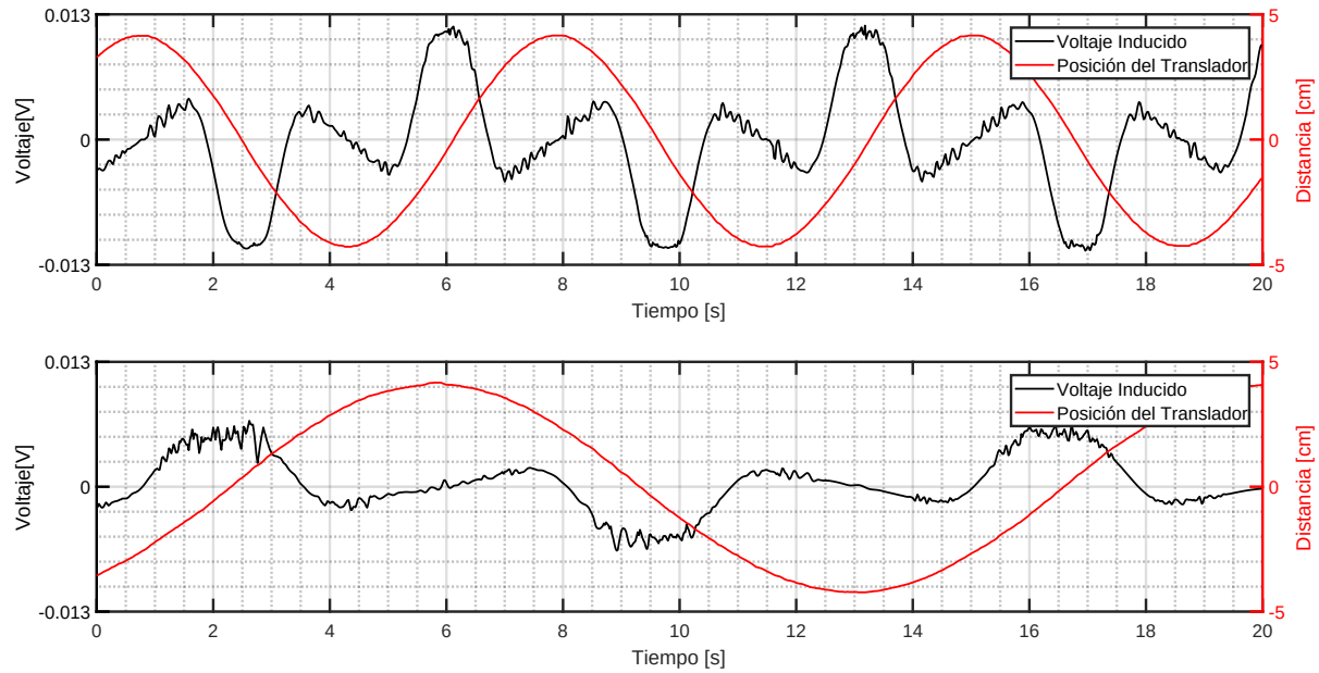
Figura 5.18: 2x1 NN : Voltaje Inducido y Posición con Período 14.28[s] y 7.14[s]
