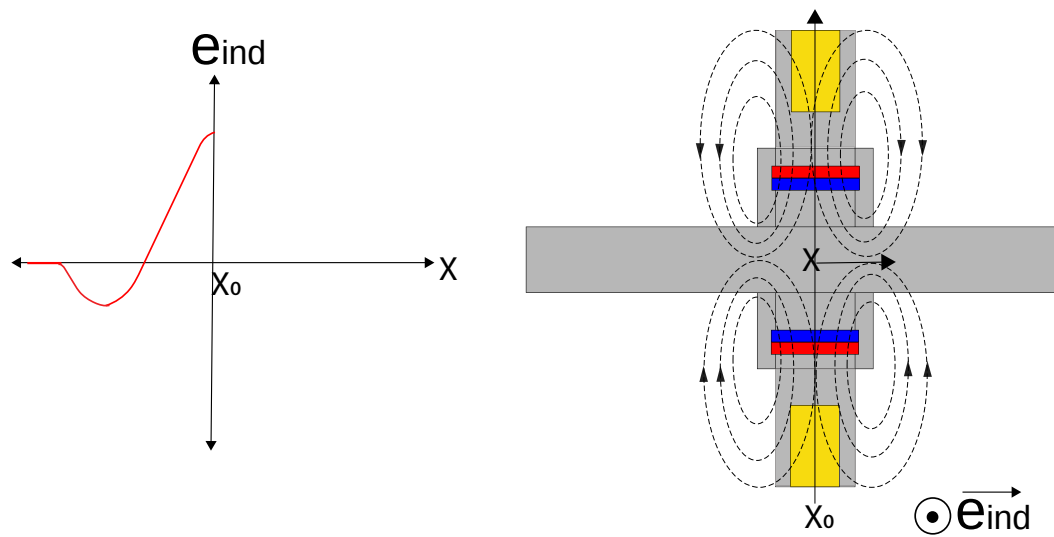
Figura 3.10: Voltaje Inducido en la Configuración 1x1 en la Posición x_0
