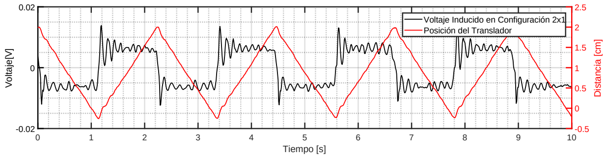
Figura 6.10: Voltaje Inducido por una Referencia Triangular de Frecuencia 450[mHz]
