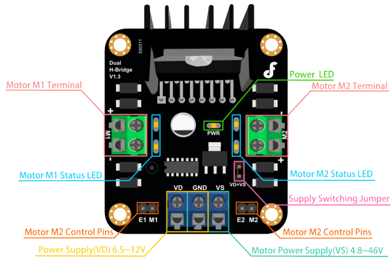
Figura 5.4: Conexiones del Driver
