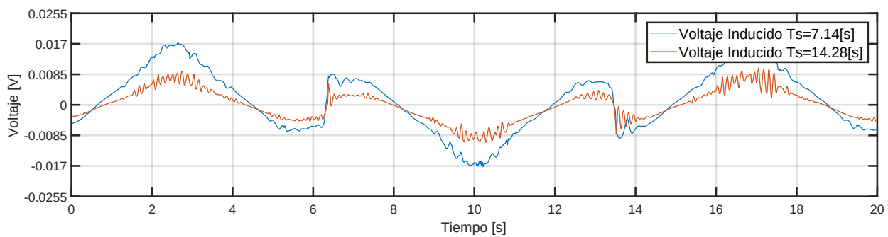
Figura B.10: 2x2 NN : Voltajes Inducidos por Referencias Triangulares y de Diferentes Períodos
