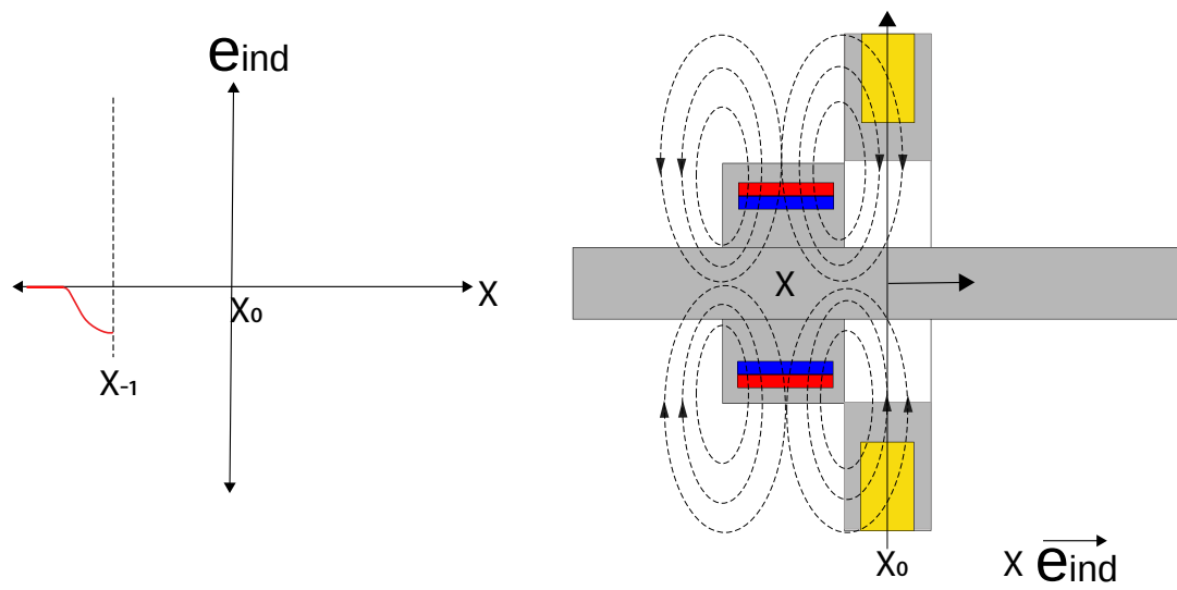
Figura 3.9: Voltaje Inducido en la Configuración 1x1 en la Posición x_{-1}
