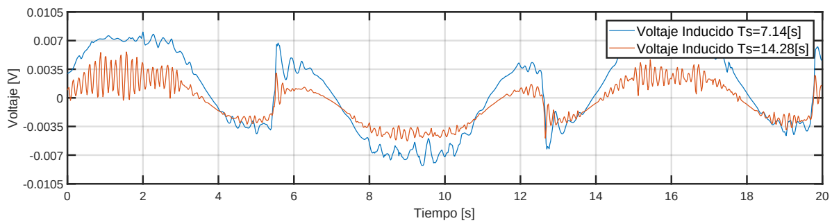
Figura B.9: 2x1 NN : Voltajes Inducidos por Referencias Triangulares y de Diferentes Períodos
