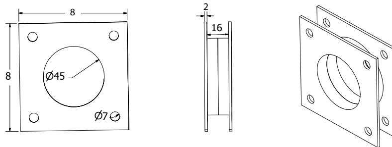
Figura 4.6: Esquema del Estator
