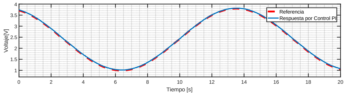
Figura 5.14: Seguimiento de la Referencia del Controlador PI en Tiempo Discreto
