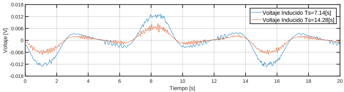
Figura 6.2: 1x2 : Voltajes Inducidos por Referencias Sinusoidales y de Diferentes Períodos
