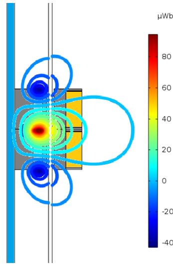
Figura 3.19: Líneas del Flujo Magnético en Configuración 2x2 NS
