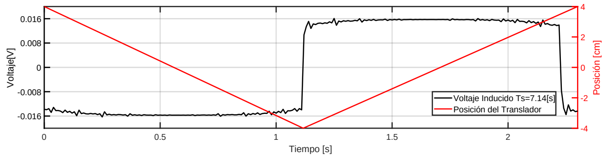
Figura 3.28: 2x1 NN : Voltaje Inducido por Referencia de Posición Triangular
