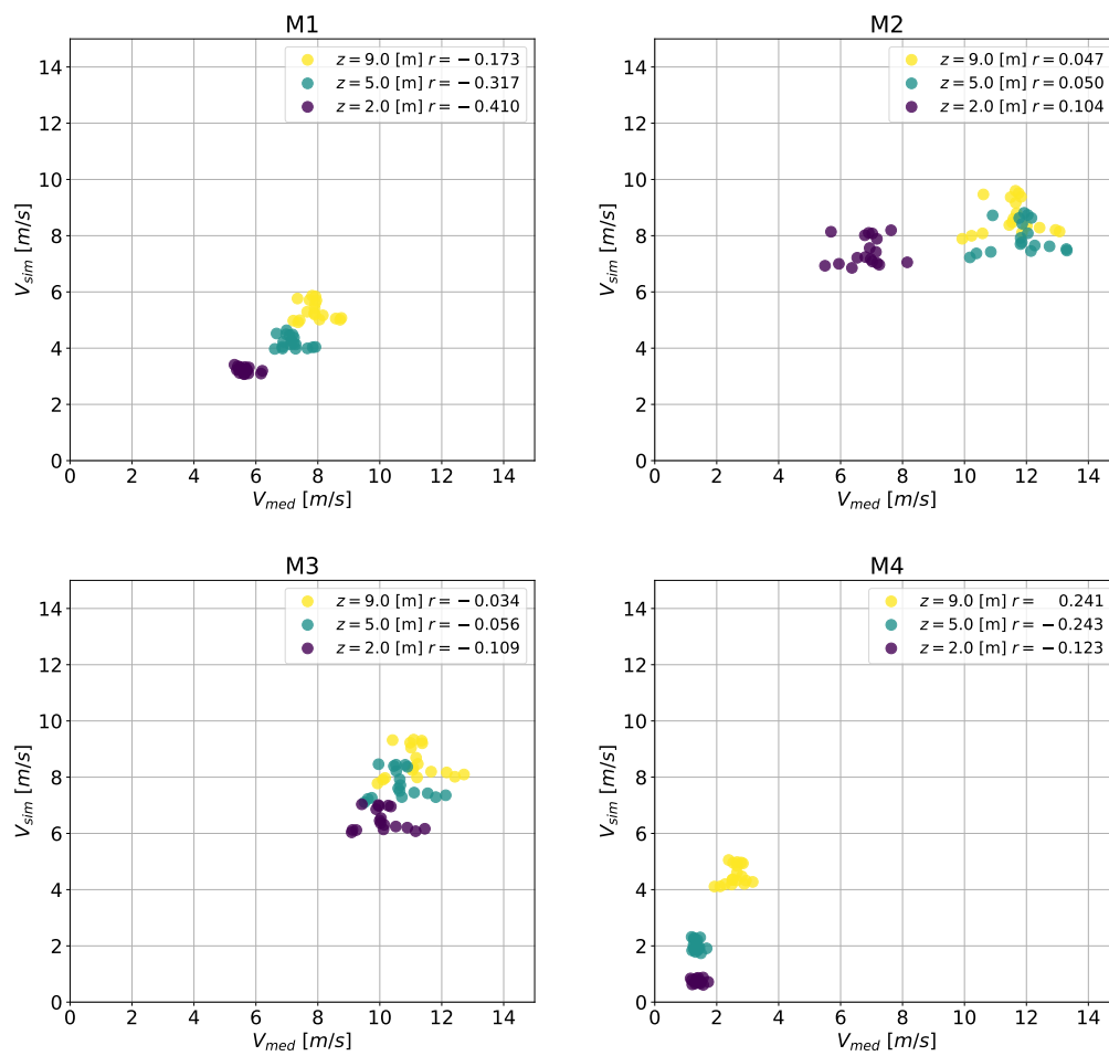
Figura 6.30: Gráfico de dispersión para las velocidades a distintas alturas en los mástiles M1-M4 en Bolund.
