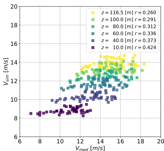
Figura 6.12: Gráfico de dispersión para las velocidades a distintas alturas en el mástil meteorológico de Høvsøre (con DA). Cada color corresponde a los valores cada 10 minutos desde las 12:00 horas.
