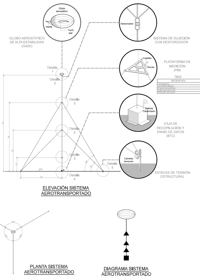
Figura 1.3: Esquema de la sonda FONDEF ID16110105.
