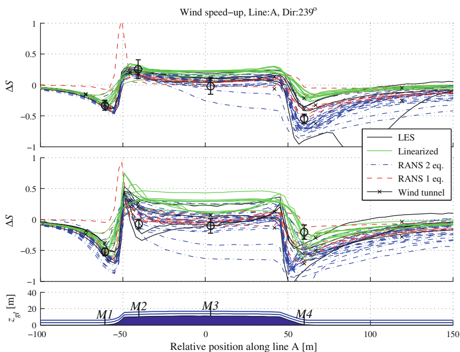
Figura A.2: Speedup medido y simulado a través de la sección transversal a 240^\circ . Arriba: valores para z = 5 [m]. Abajo: valores para z = 2 [m].
