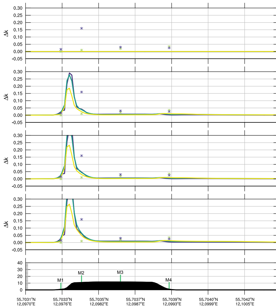
Figura 6.37: Incremento adimensional de energía cinética turbulenta (sgs) en los primeros 3 niveles del modelo (1,1 [m] azul; 3,4 [m] verde; 5,6 [m] amarillo) para la sección de corte a 240° en Bolund (con DA). Se muestran los resultados para las 12:00 (arriba), 13:00, 14:00 y 15:00 horas (abajo).
