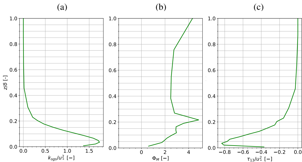
Figura 6.10: Variables adimensionalizadas (con u_* = 0,527 [m/s]) de segundo orden para el caso de Høvsøre con DA promediados entre las 12:00 y las 15:00 (atmósfera neutra, terreno plano homogéneo). (a) Energía cinética turbulenta de submalla, (b) Gradiente de velocidad, (c) Esfuerzo turbulento.
