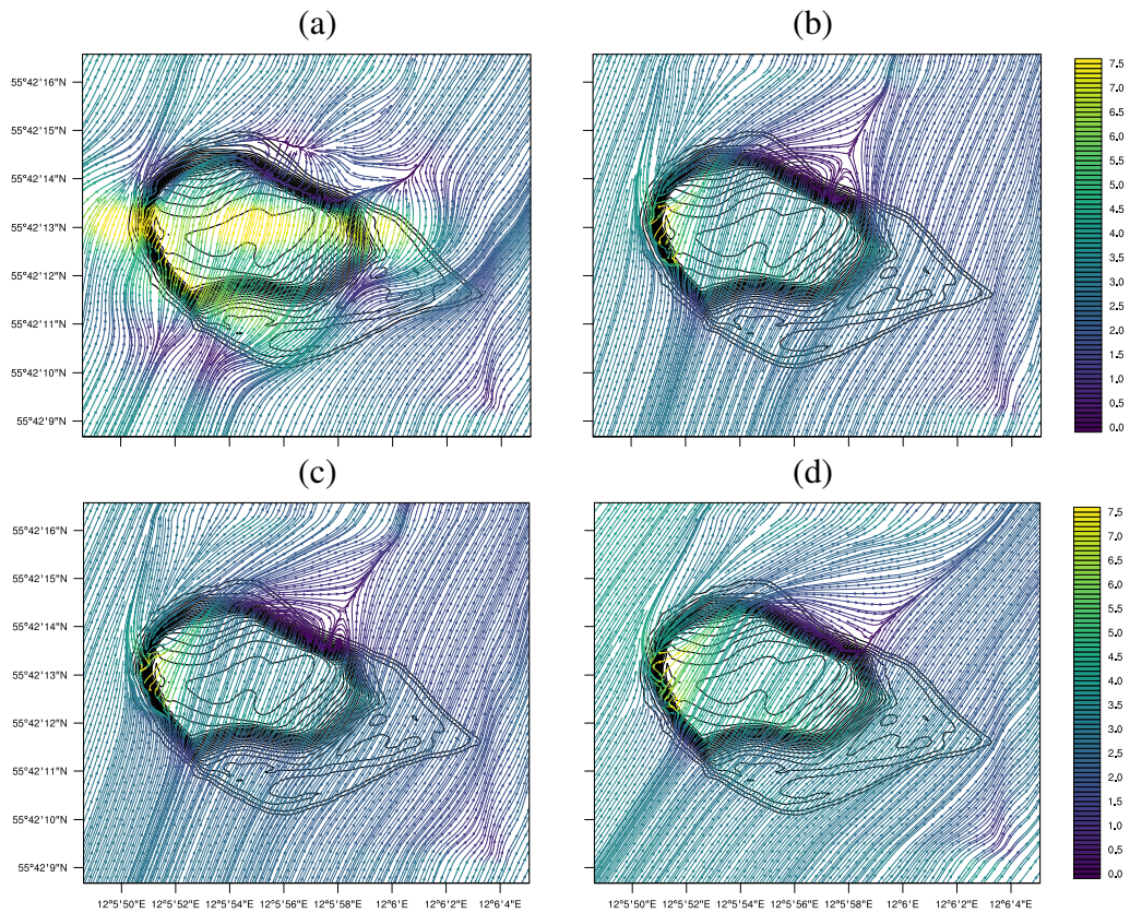
Figura 6.33: Líneas de flujo para la solución numérica en Bolund (con DA) en el primer nivel ( z_1 = 1,12 [m]) en las horas (a) 12:00, (b) 13:00, (c) 14:00 y (d) 15:00.
