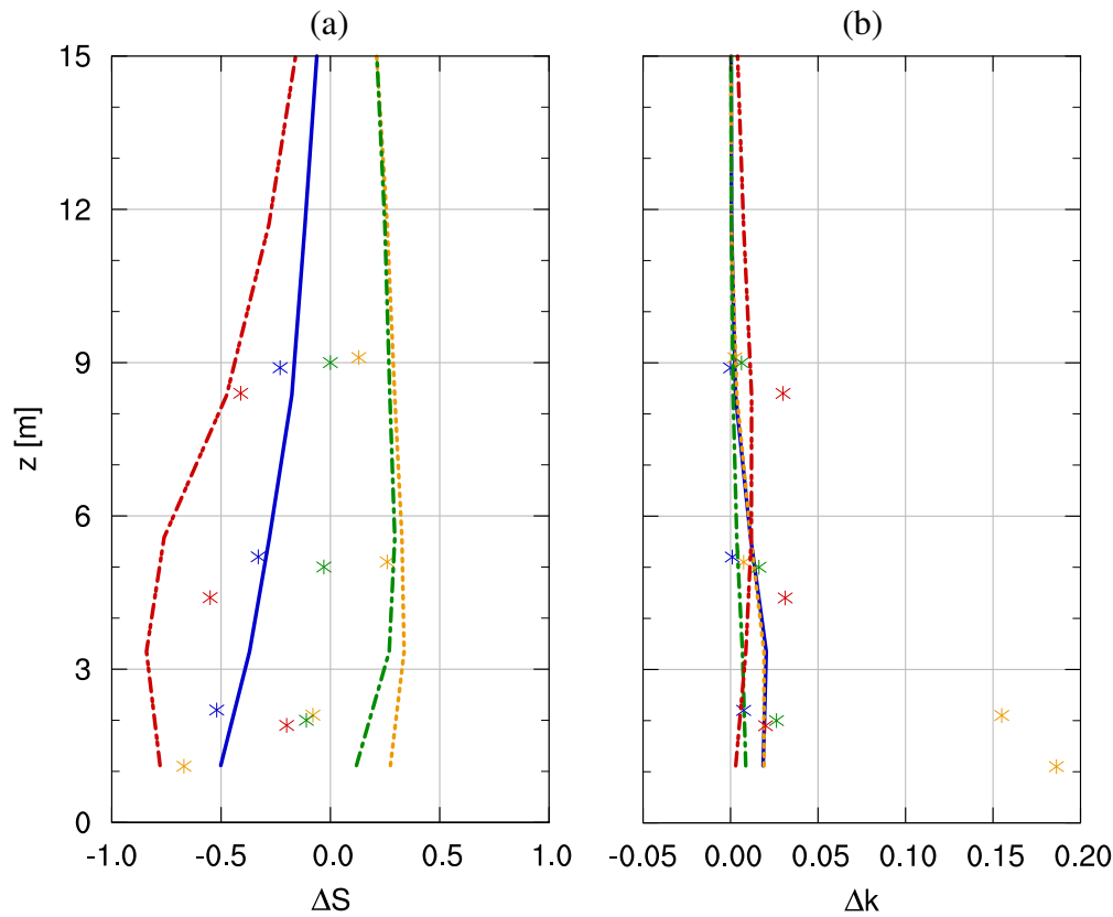
Figura 6.19: Perfil vertical promedio de 12:00 a 15:00 de (a) speedup y (b) variación adimensional de energía cinética turbulenta para las estaciones M1 (azul), M2 (naranja), M3 (verde) y M4 (rojo).
