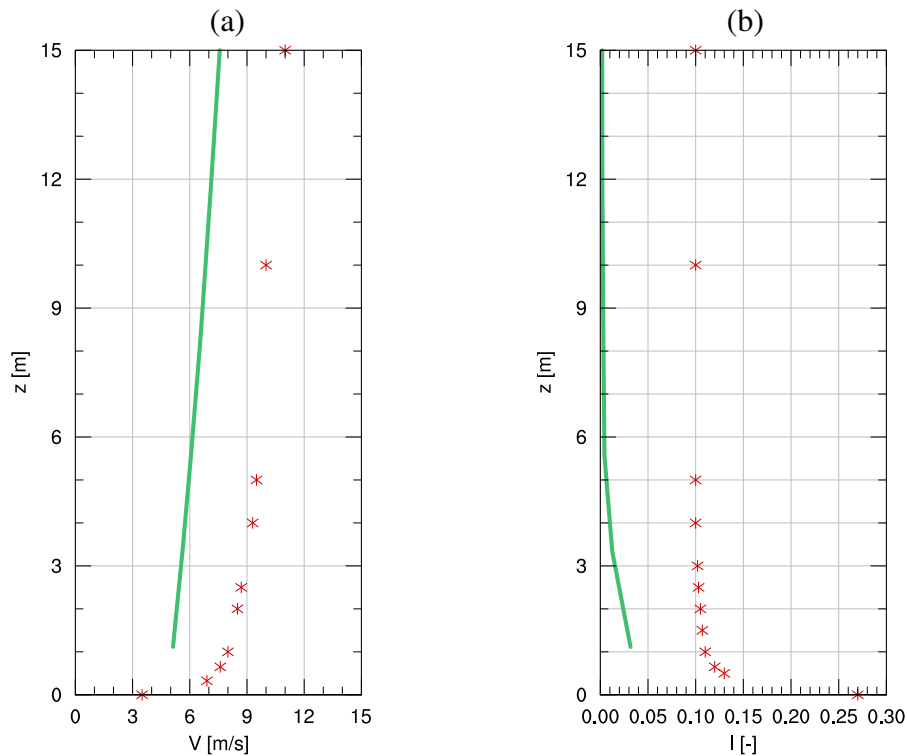
Figura 6.16: Perfiles promedio referenciales en el flujo no perturbado (caso Bolund) para: (a) Rapidez del viento (en asteriscos se presenta la condición de contorno presentada por Bechmann et al. (2011) ) (b) Intensidad de energía cinética turbulenta de submallá (sgs).
