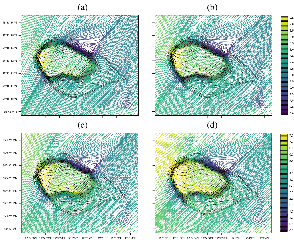
Figura 6.14: Líneas de flujo para la solución numérica en Bolund en el primer nivel numérico ( z_1 = 1,12 [m]) en las horas (a) 12:00, (b) 13:00, (c) 14:00 y (d) 15:00.
