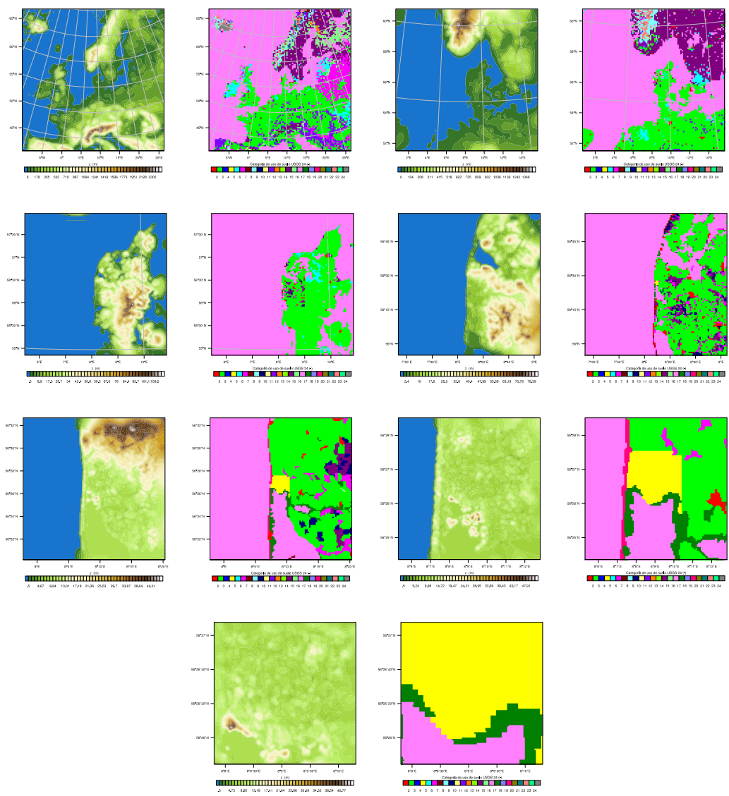
Figura B.1: Orografía (MSNM) y uso de suelo (categoría USGS24) de alta resolución para cada uno de las mallas anidadas (d01-d07) en Høvsøre.
