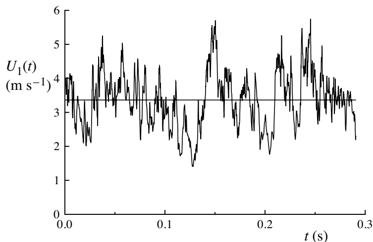
Figura 3.1: Serie de tiempo para una componente de la velocidad en un flujo turbulento. Fuente: Pope (2000).
