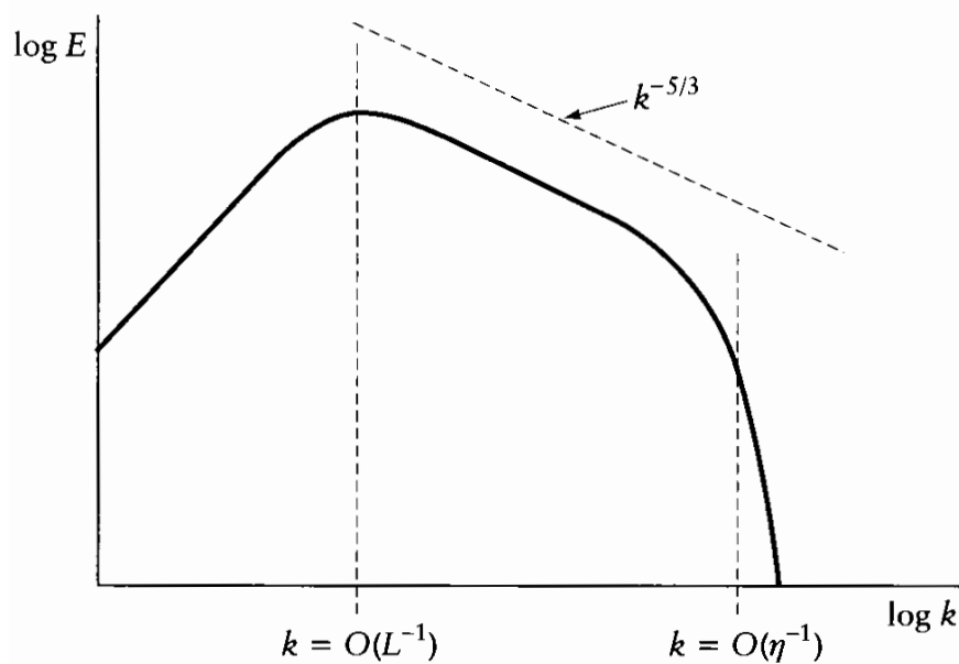
Figura 3.2: Gráfico típico log-log de distribución de energía cinética turbulenta con respecto al número de onda \kappa para un flujo con un número de Reynolds elevado. Fuente: Mathieu y Scott (2000).
