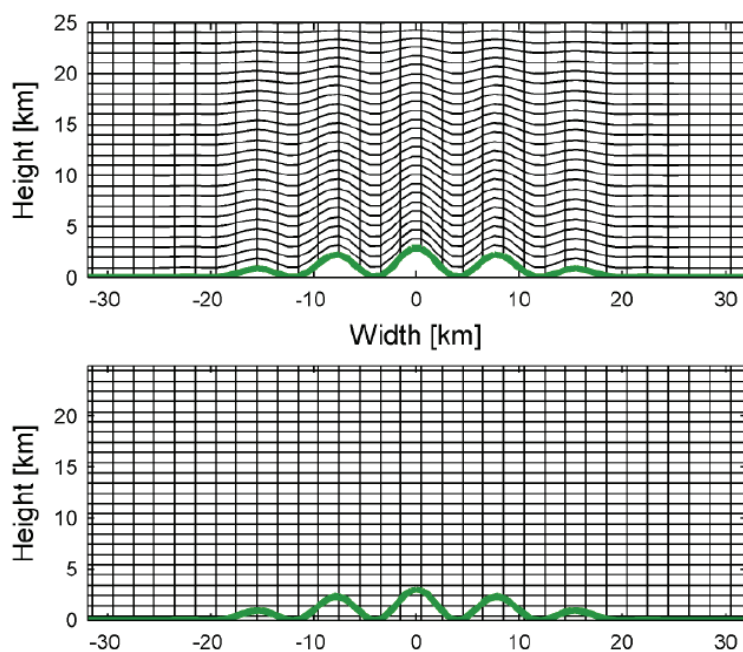
Figura 2.4: Comparación entre las coordenadas usuales sigma (arriba) y el método de frontera inmersa (abajo). Fuente: Arnold et al. (2012) .
