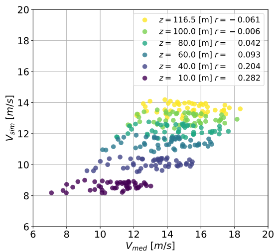
Figura 6.7: Gráfico de dispersión para las velocidades a distintas alturas en el mástil meteorológico de Høvsøre. Cada color corresponde a los valores cada 10 minutos desde las 12:00 horas.
