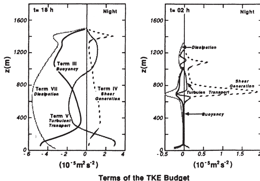
Figura 3.7: Términos normalizados en la ecuación de TKE para la noche (18:00 y 02:00). Fuente: Stull (1988).
