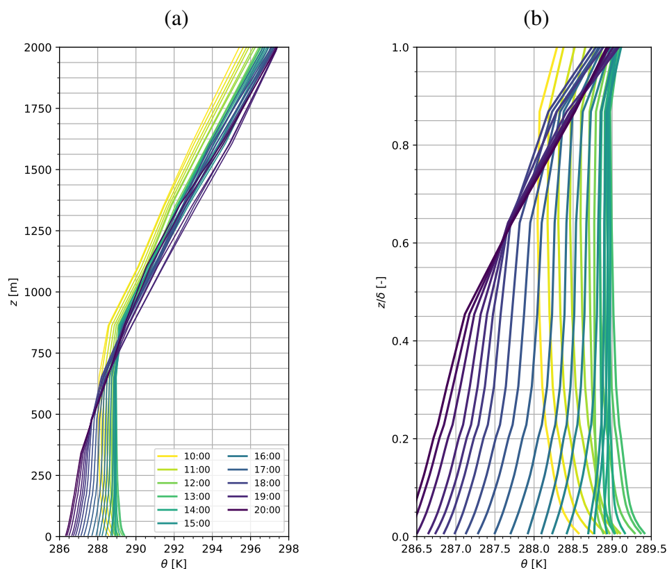
Figura 6.1: Ciclo diurno-nocturno del perfil de temperatura potencial virtual en el mástil meteorológico en Høvsøre. (a) Resultados cada 20 minutos del perfil de \theta_v . (b) Detalle del perfil de \theta_v dentro de la capa límite atmosférica ( \delta \approx 750 [m]).
