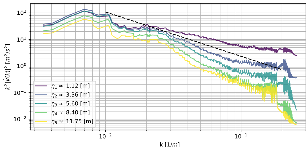
Figura 6.48: Espectros de energía cinética para la magnitud horizontal del viento a distintos niveles verticales en el dominio d08 caso Bolund con DA.
