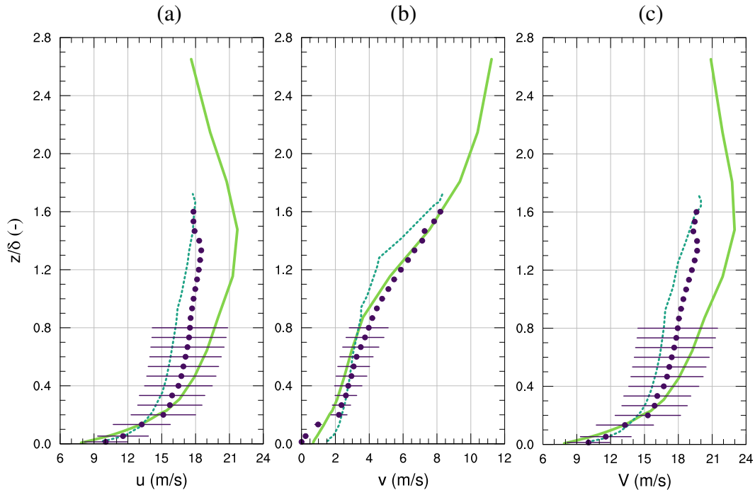
Figura 6.4: Comparación de la simulación con WRF (línea continua) con la simulación de Peña et al. (2013) (línea punteada) y valores medidos para (a) componente longitudinal u de la velocidad del viento, (b) componente transversal v y (c) magnitud de la velocidad del viento. Los datos corresponden a promedios temporales entre las 12:00 y 15:00, y han sido rotados de tal forma que su dirección sea 0^\circ a los 10m sobre el suelo, igualando lo representado por Peña et al. (2013).
