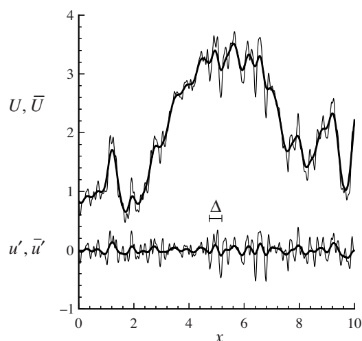
Figura 3.8: Curva superior: una muestra de un campo de velocidad u y su correspondiente campo filtrado \bar{u} (en negrita). Curva inferior: campo residual u' y campo residual filtrado \overline{u'} (en negrita). Fuente: Pope (2000).
