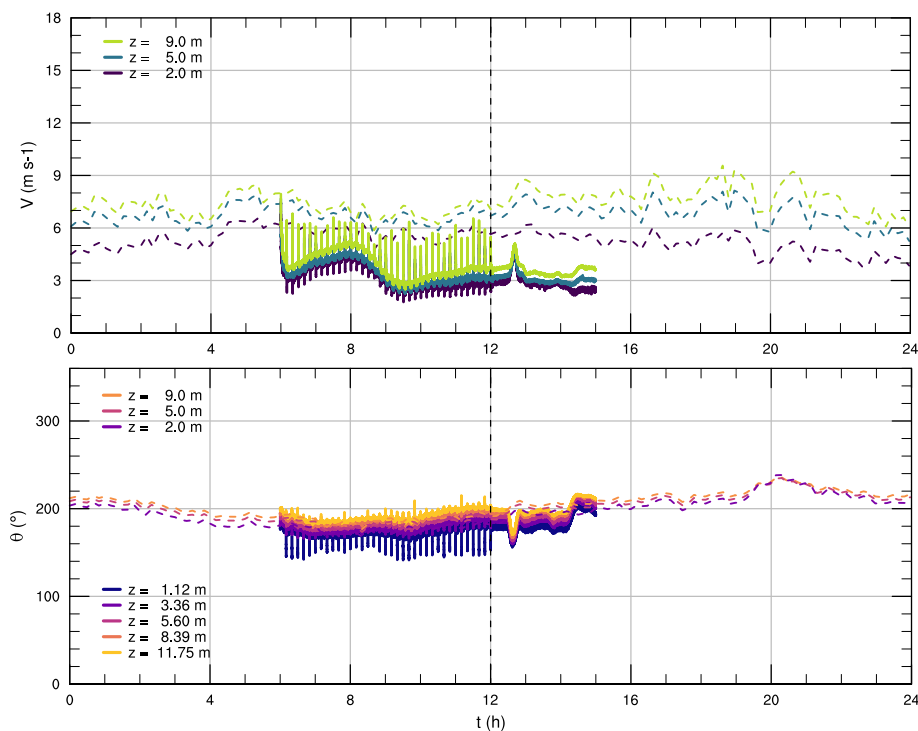
Figura 6.39: Series de tiempo para la rapidez V y dirección \theta del viento en M1 con DA.
