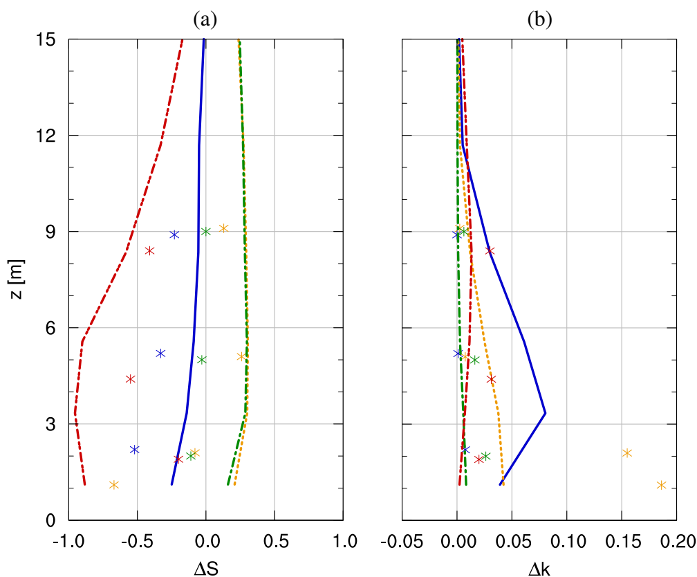
Figura 6.38: Perfil vertical de (a) speedup y (b) variación adimensional de energía cinética turbulenta para M1 (azul), M2 (naranja), M3 (verde) y M4 (rojo) para el caso con DA.
