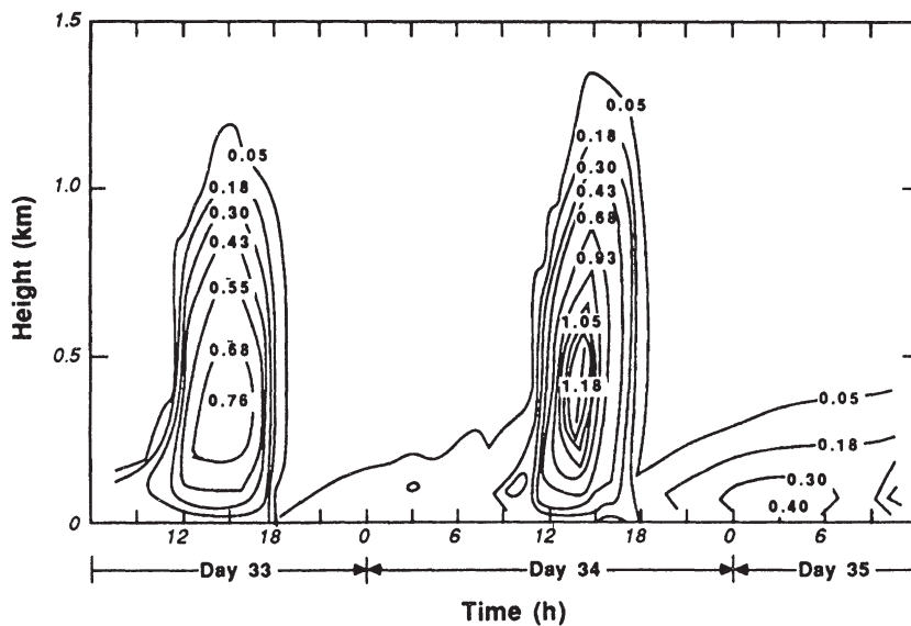
Figura 3.5: Variación espacial y temporal de TKE modelada. Fuente: Stull (1988).
