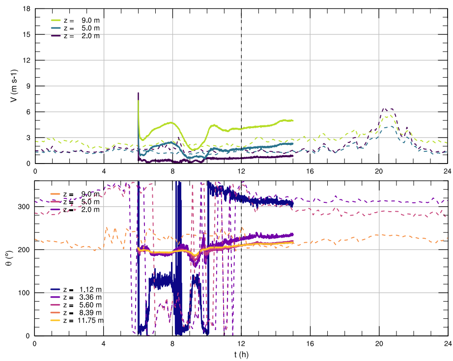
Figura 6.23: Series de tiempo para la rapidez V y dirección \theta del viento en M4.
