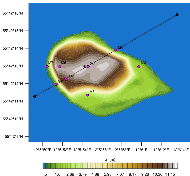
Figura 5.7: Ubicación espacial de los puntos de control en el dominio de Bolund. En cada punto de control se ubican anemómetros que miden a las alturas de 2m, 5m, y 9m sobre el suelo.
