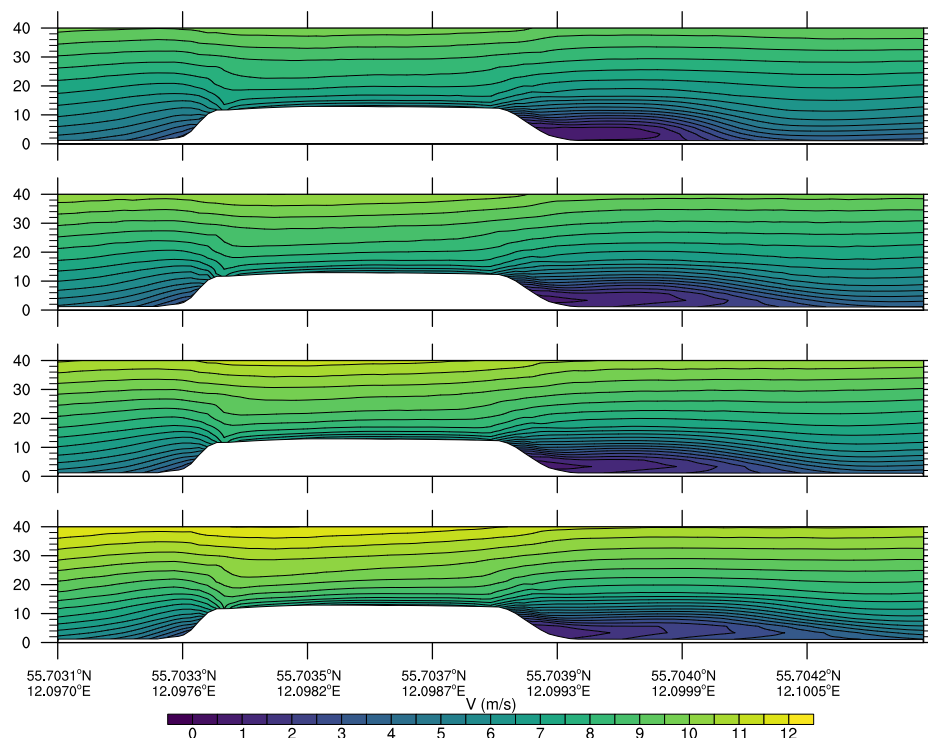
Figura 6.15: Contornos de rapidez del viento para la sección de corte vertical a 240^\circ en Bolund. Se muestran los resultados para las 12:00 (arriba), 13:00, 14:00 y 15:00 horas (abajo). Escala 1:1.
