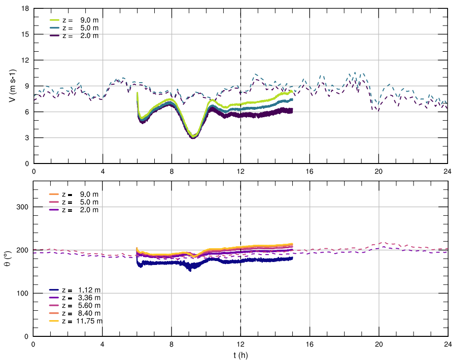
Figura 6.26: Series de tiempo para la rapidez V y dirección \theta del viento en M7.
