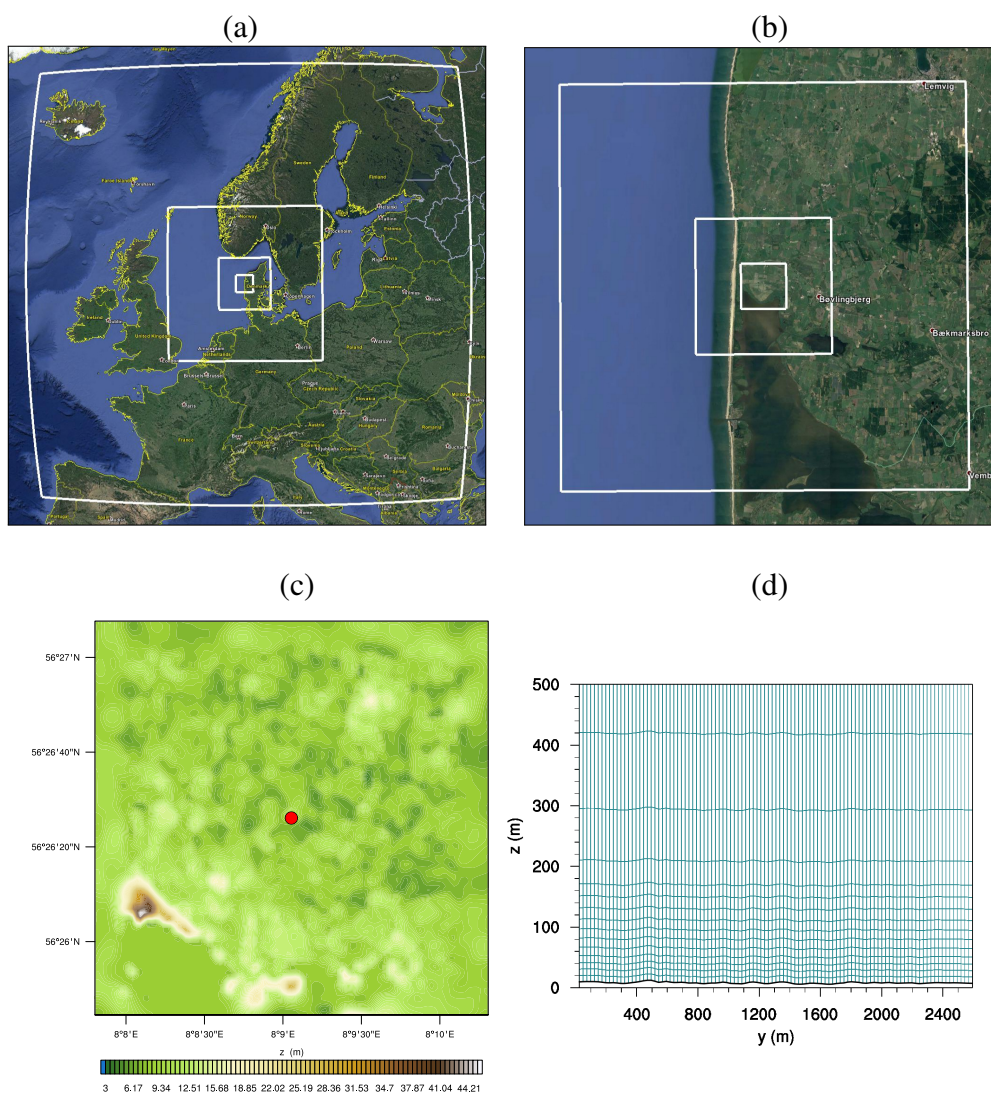
Figura 5.5: Información de los dominios de simulación para el caso Høvsøre. (a) Dominios d01-d04. (b) Dominios d05-d07. (c) Dominio d07 con el punto de control. (d) Distribución vertical de la malla adaptativa en escala 4:1.
