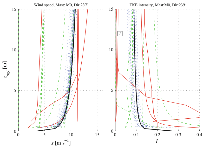
Figura A.1: Perfil del viento no perturbado en el punto referencial M0 (ver Figura 5.2). En línea negra está el perfil entregado por los desarrolladores (para utilizar como condición de borde) y el resto corresponde a distintos modelos. La línea sólida roja corresponde a simulaciones LES.
