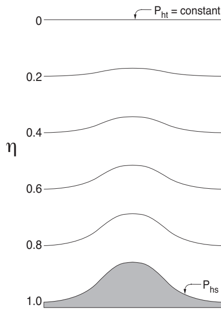
Figura 4.1: Estructura de la coordenada vertical. Fuente: Skamarock et al. (2008).
