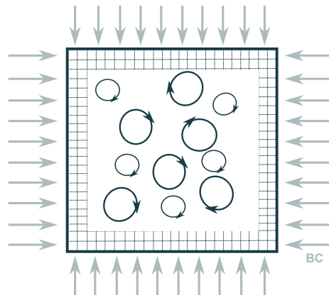
Figura 2.2: Idealización de los distintos tamaños de vórtices dentro de un dominio en la zona gris de la turbulencia. Fuente: Montornes et al. (2017) .
