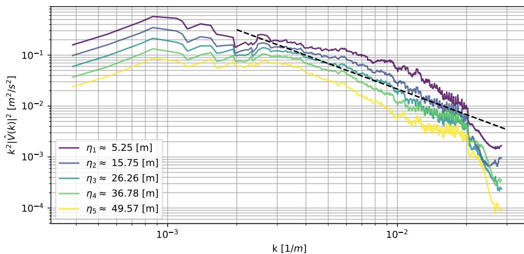
Figura 6.6: Espectros de energía cinética para la magnitud horizontal del viento a distintos niveles verticales en el dominio d07 caso Høvsøre.
