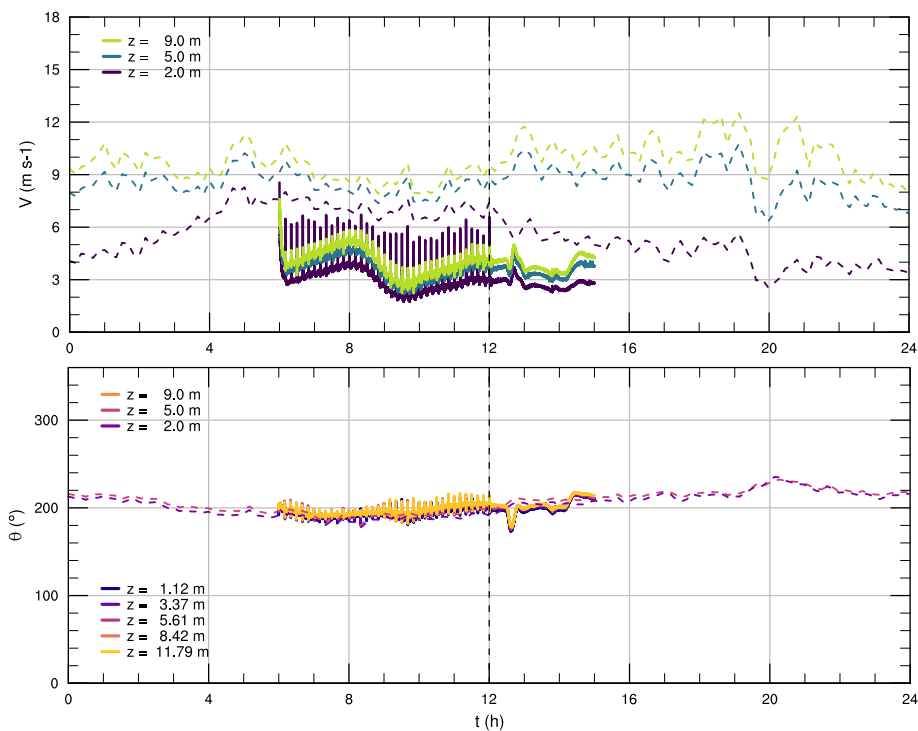
Figura 6.46: Series de tiempo para la rapidez V y dirección \theta del viento en M8 con DA.
