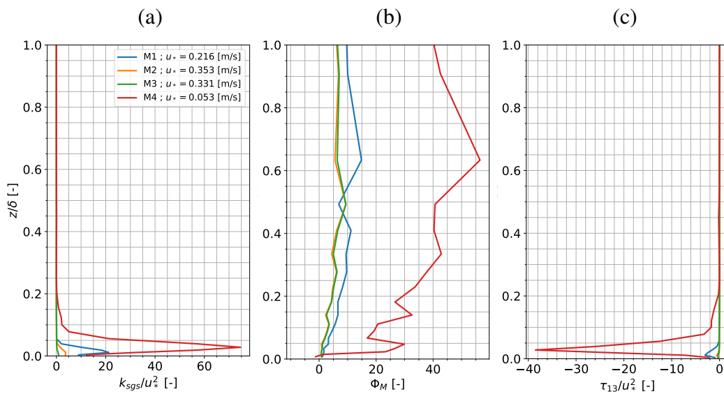
Figura 6.47: Variables adimensionalizadas de segundo orden para M1-M4 con DA, promediadas entre las 12:00 y las 15:00. (a) Energía cinética turbulenta de submalla, (b) Gradiente de velocidad, (c) Esfuerzo turbulento.
