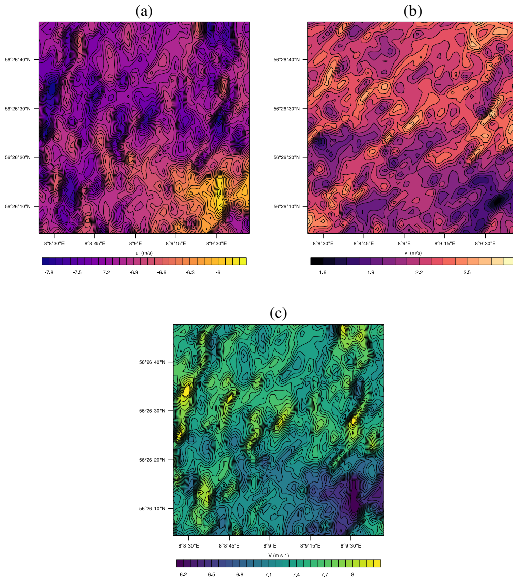
Figura 6.2: (a) Componente longitudinal u de la velocidad en el primer nivel de la coordenada vertical ( z_1 = 5,25 [m]) para las 15:00. (b) Idéntico al anterior pero para la componente transversal v . (c) Magnitud del campo de velocidad.
