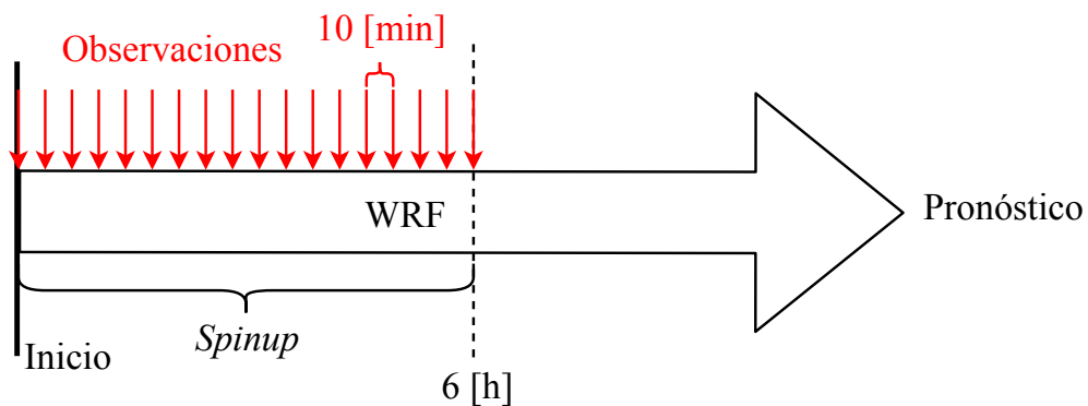
Figura 5.3: Esquema del proceso de asimilación de datos.
