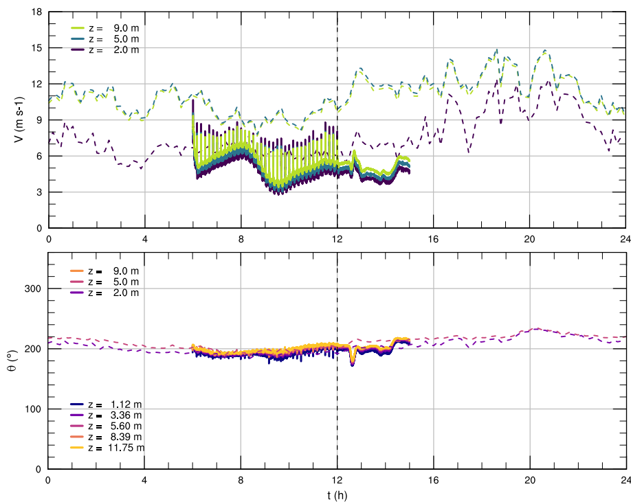
Figura 6.40: Series de tiempo para la rapidez V y dirección \theta del viento en M2 con DA.
