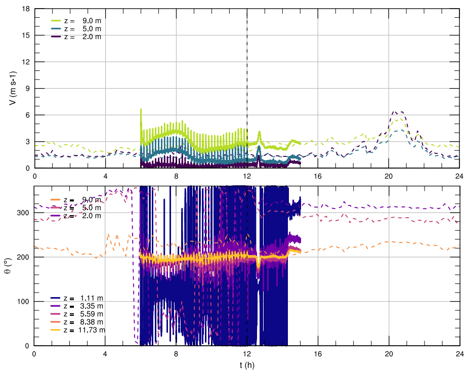
Figura 6.42: Series de tiempo para la rapidez V y dirección \theta del viento en M4 con DA.
