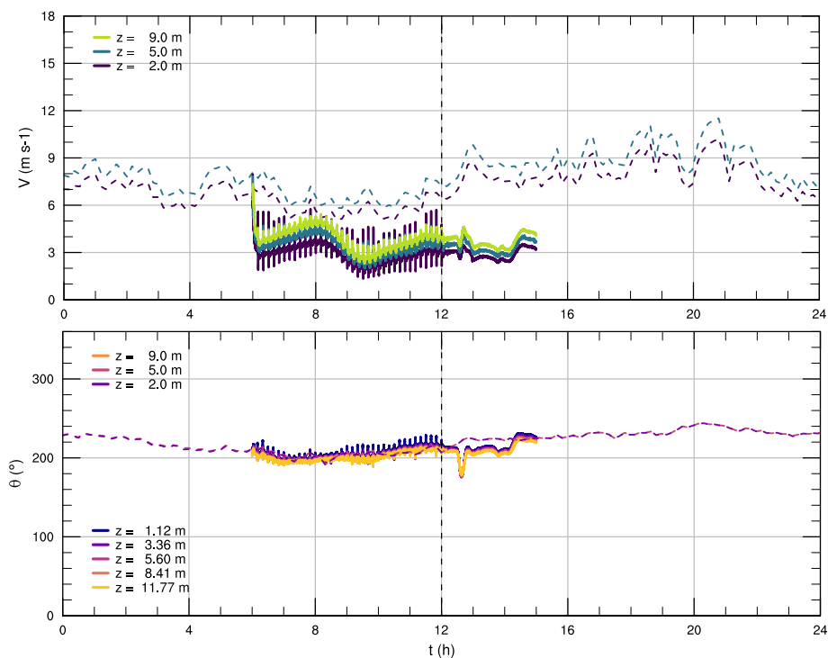
Figura 6.43: Series de tiempo para la rapidez V y dirección \theta del viento en M5 con DA.
