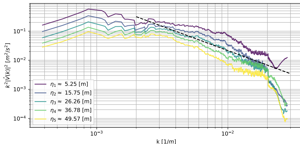
Figura 6.11: Espectros de energía cinética para la magnitud horizontal del viento a distintos niveles verticales en el dominio d07 caso Høvsøre con DA.
