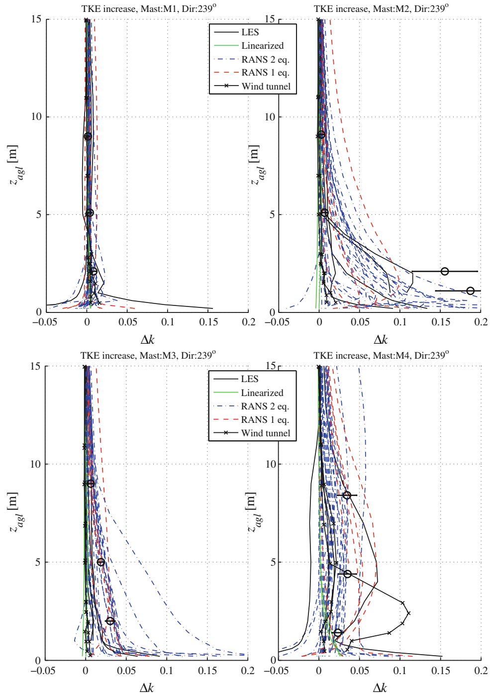
Figura A.5: Perfil de \Delta k medido y simulado en los distintos mástiles M1-M4.
