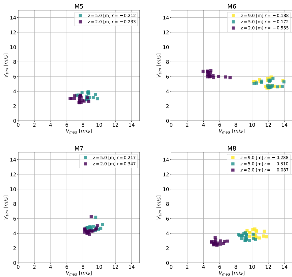
Figura 6.50: Gráfico de dispersión para las velocidades a distintas alturas en los mástiles M5-M8 en Bolund (con DA).
