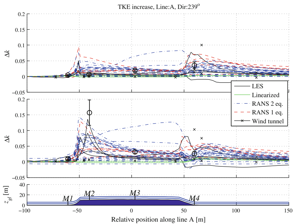
Figura A.4: \Delta k medido y simulado a través de la sección transversal a 240^\circ . Arriba: valores para z = 5 [m]. Abajo: valores para z = 2 [m].
