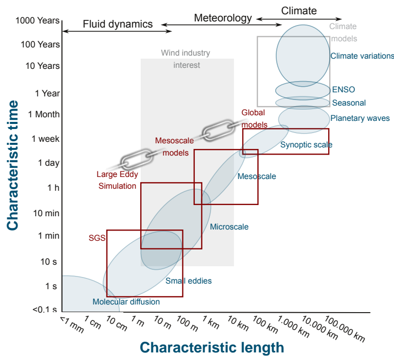
Figura 2.1: Separación de escalas para la dinámica atmosférica. Fuente: Montornes et al. (2017) .
