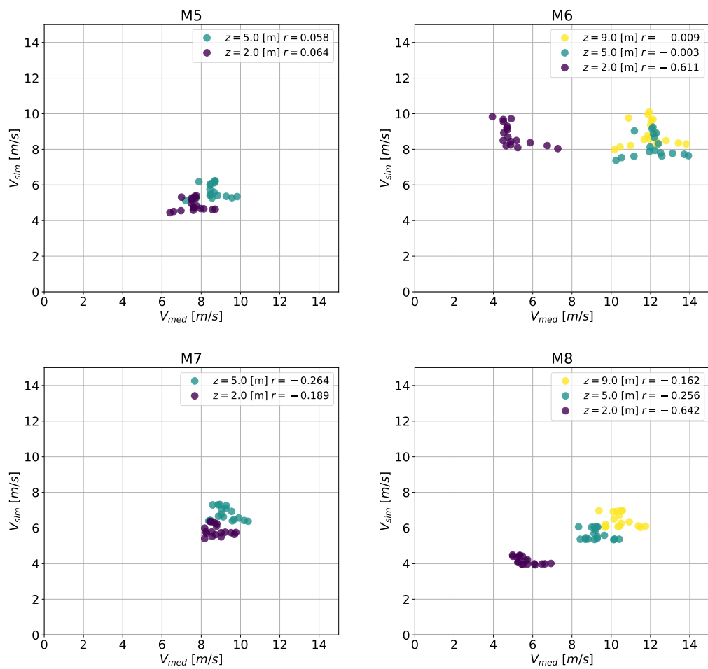
Figura 6.31: Gráfico de dispersión para las velocidades a distintas alturas en los mástiles M5-M8 en Bolund.
