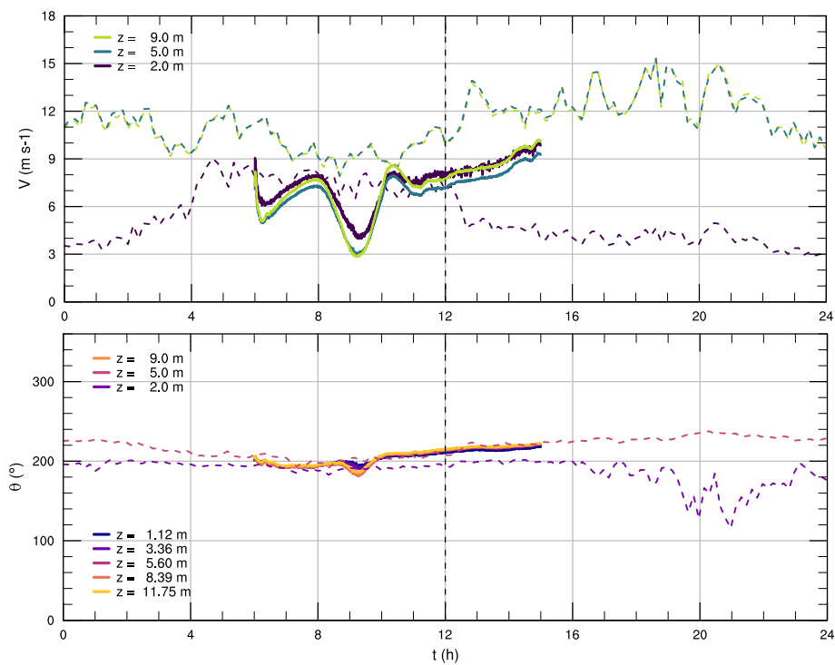
Figura 6.25: Series de tiempo para la rapidez V y dirección \theta del viento en M6.
