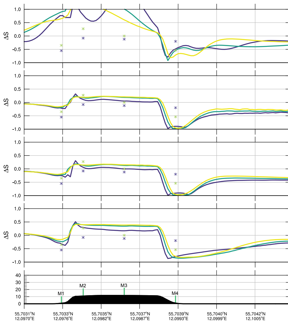
Figura 6.36: Speedup en los primeros 3 niveles del modelo (1,1 [m] azul; 3,4 [m] verde; 5,6 [m] amarillo) para la sección de corte a 240° en Bolund (con DA). Se muestran los resultados para las 12:00 (arriba), 13:00, 14:00 y 15:00 horas (abajo).
