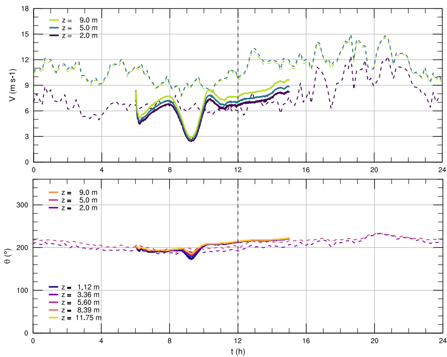
Figura 6.21: Series de tiempo para la rapidez V y dirección \theta del viento en M2.
