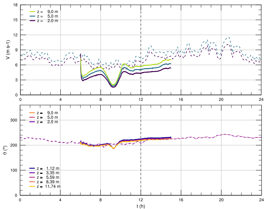
Figura 6.24: Series de tiempo para la rapidez V y dirección \theta del viento en M5.
