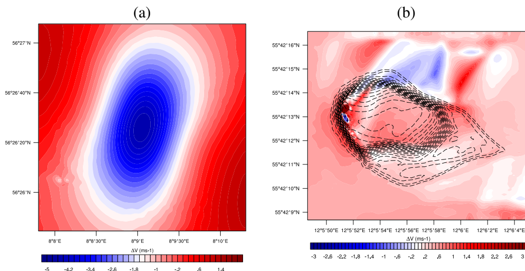
Figura 5.4: Diferencia de la magnitud del campo de velocidad en el primer nivel del modelo entre resultados sin y con asimilación de datos. (a) Caso I puntual. (b) Caso II con varios puntos.
