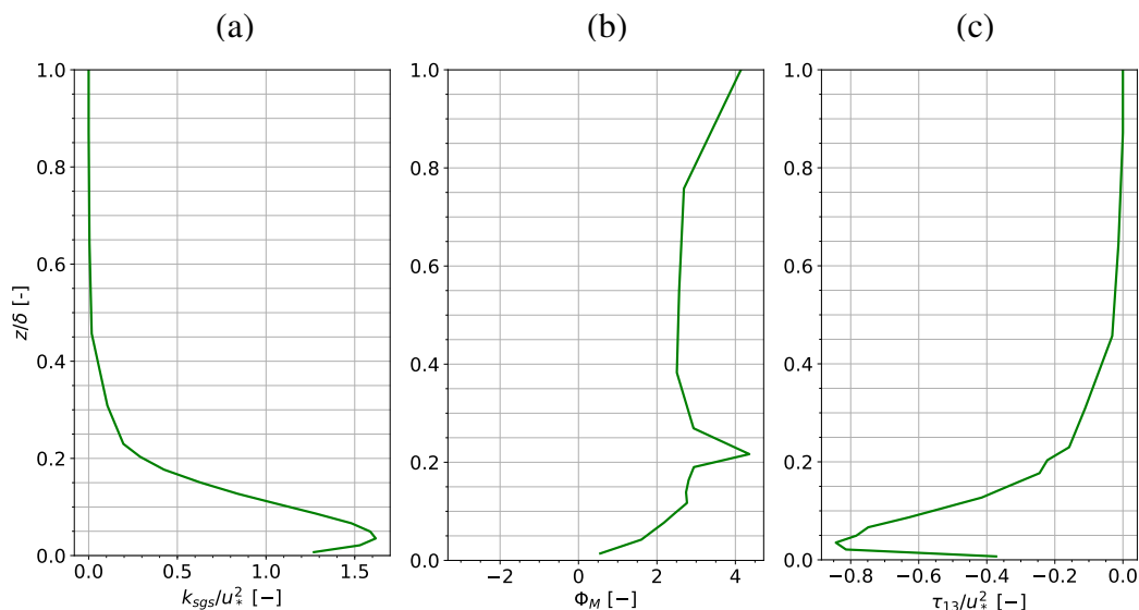
Figura 6.5: Variables adimensionalizadas (con u_* = 0,552 [m/s]) de segundo orden para el caso de Høvsøre promediados entre las 12:00 y las 15:00 (atmósfera neutra, terreno plano homogéneo). (a) Energía cinética turbulenta de submalla, (b) Gradiente de velocidad, (c) Esfuerzo turbulento.
