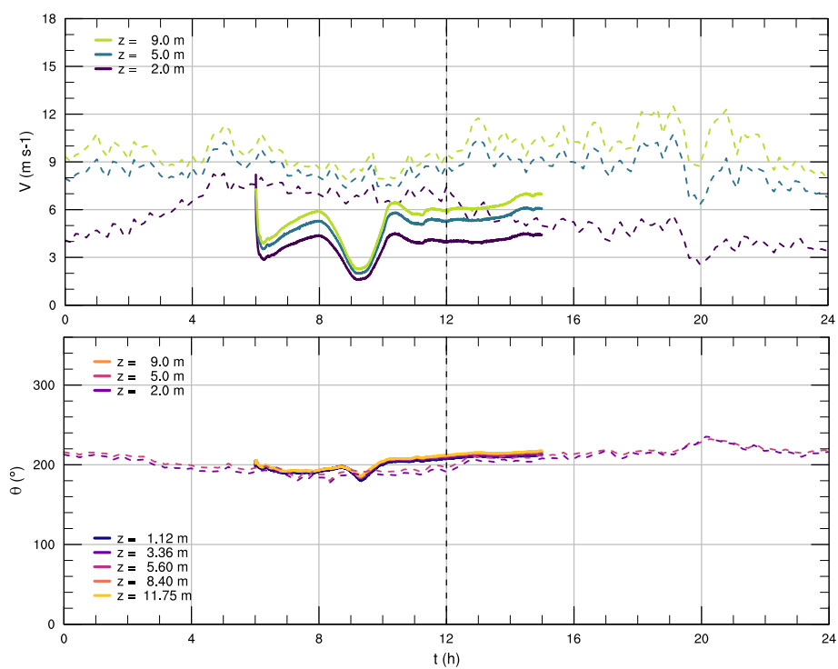
Figura 6.27: Series de tiempo para la rapidez V y dirección \theta del viento en M8.
