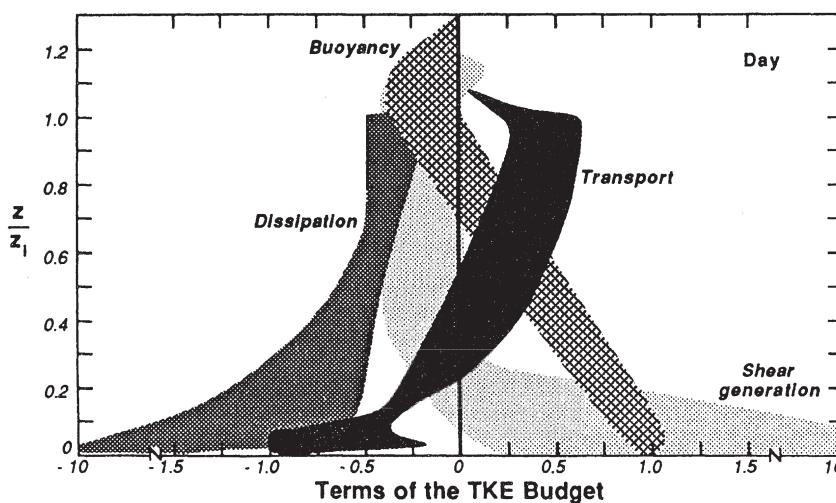
Figura 3.6: Términos normalizados en la ecuación de TKE para el día. Las áreas sombreadas corresponden a un rango de valores. Todos los términos son adimensionalizados por w_*^3/\delta . Fuente: Stull (1988).
