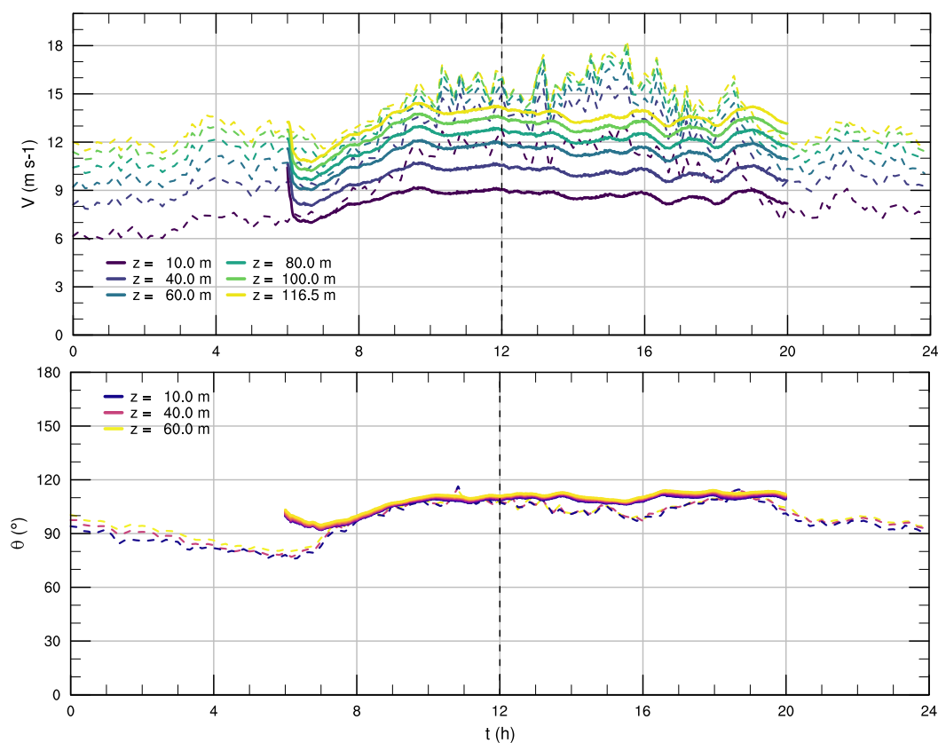
Figura 6.3: Serie de tiempo para la rapidez instantánea del viento V y su dirección en la ubicación del mástil meteorológico. La línea continua corresponde a lo datos simulados interpolados a las alturas de medición (solo para V ) y la línea punteada a los datos medidos en el mástil.
