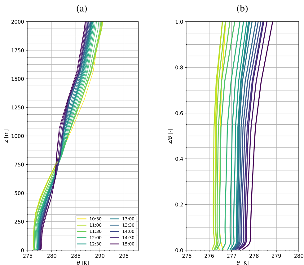
Figura 6.13: Ciclo horario del perfil de temperatura potencial virtual promedio de los 8 mástiles en Bolund. (a) Resultados cada 10 minutos del perfil de \theta_v . (b) Detalle del perfil de \theta_v dentro de la capa límite atmosférica con resultados cada 15 minutos ( \delta \approx 300 [m]).
