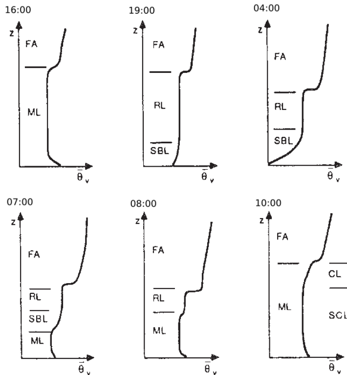
Figura 3.4: Evolución del perfil de \theta_v en el ciclo diurno. Fuente: Stull (1988).
