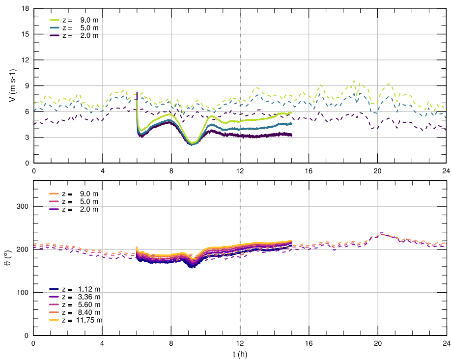
Figura 6.20: Series de tiempo para la rapidez V y dirección \theta del viento en M1.
