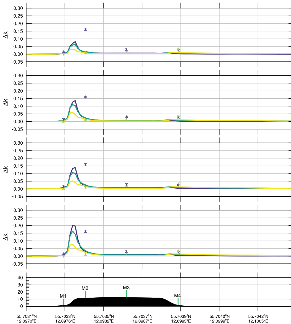
Figura 6.18: Incremento adimensional de energía cinética turbulenta (sgs) en los primeros 3 niveles del modelo (1,1 [m] azul; 3,4 [m] verde; 5,6 [m] amarillo) para la sección de corte a 240° en Bolund. Se muestran los resultados para las 12:00 (arriba), 13:00, 14:00 y 15:00 horas (abajo).
