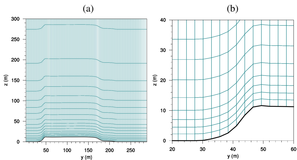
Figura 5.8: (a) Distribución de la malla vertical en la mitad del dominio en Bolund. (b) Detalle la pendiente abrupta (escala 1:1).
