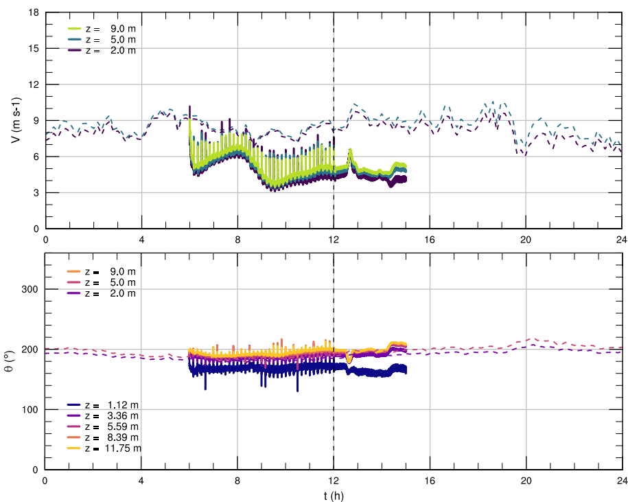
Figura 6.45: Series de tiempo para la rapidez V y dirección \theta del viento en M7 con DA.
