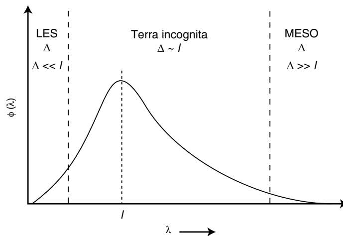
Figura 2.3: Espectro de energía cinética turbulenta multiescala. Fuente: Warner (2010)
