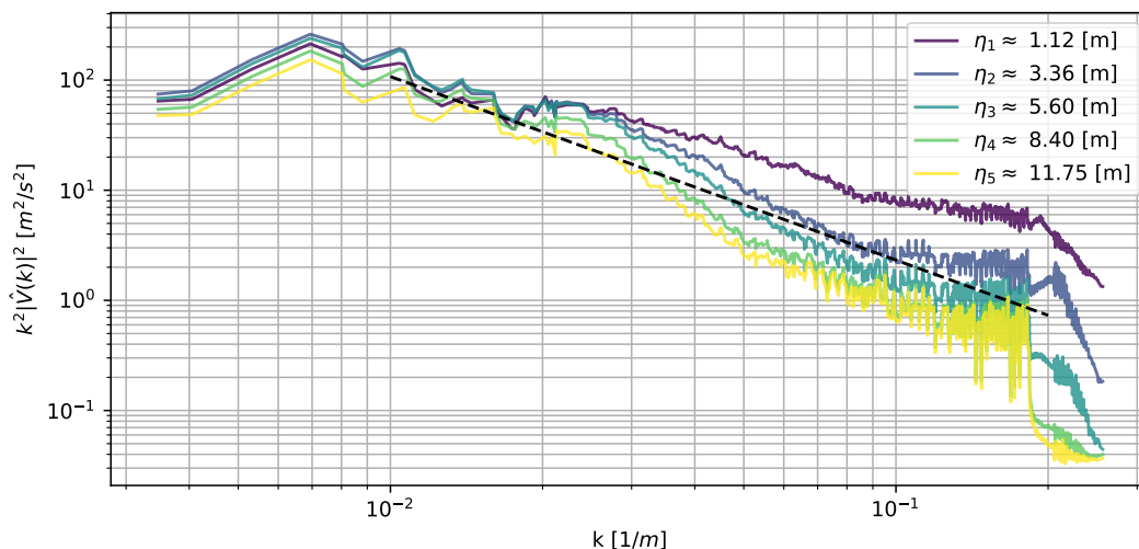
Figura 6.29: Espectros de energía cinética para la magnitud horizontal del viento a distintos niveles verticales en el dominio d08 caso Bolund.
