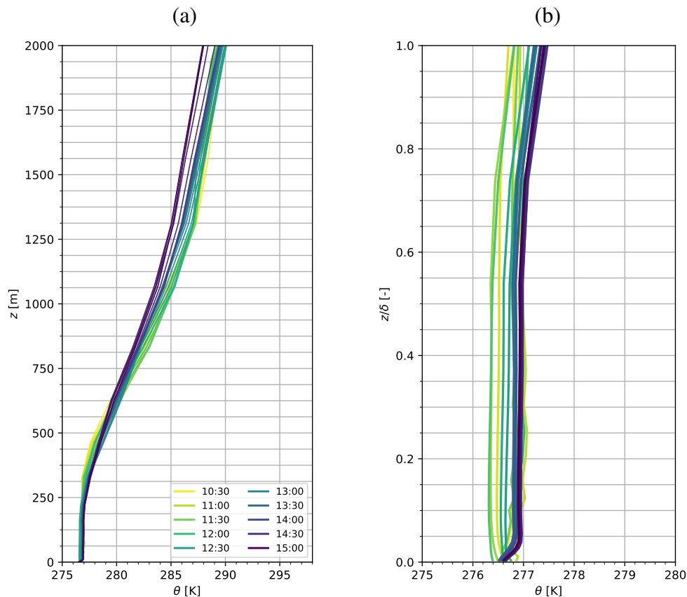
Figura 6.32: Ciclo horario del perfil de temperatura potencial virtual promedio de los 8 mástiles (con DA). (a) Resultados cada 10 minutos del perfil de \theta_v . (b) Detalle del perfil dentro de la capa límite atmosférica con resultados cada 15 minutos ( \delta \approx 300 [m]).
