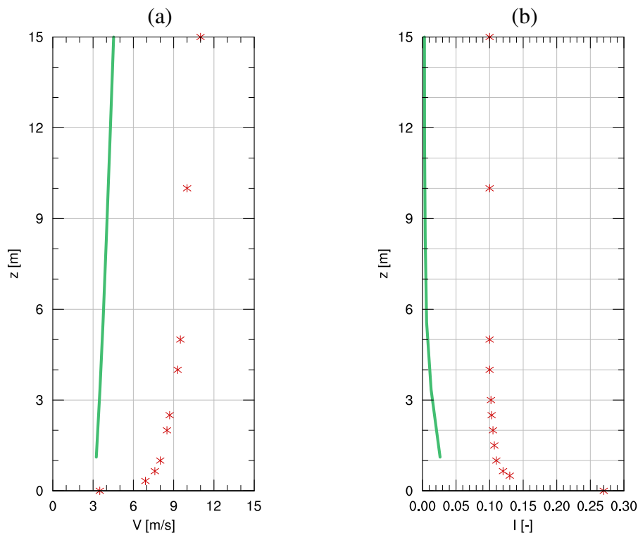
Figura 6.35: Perfiles promedio referenciales (Bolund con DA) en el flujo no perturbado para: (a) Rapidez del viento (en línea punteada se presenta la condición de contorno presentada por Bechmann et al. (2011) ) (b) Intensidad de energía cinética turbulenta (sgs).
