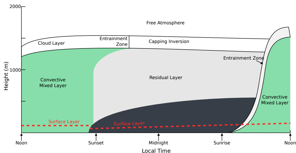
Figura 3.3: Evolución diurna de la estructura de la capa límite. Fuente: Wikimedia.
