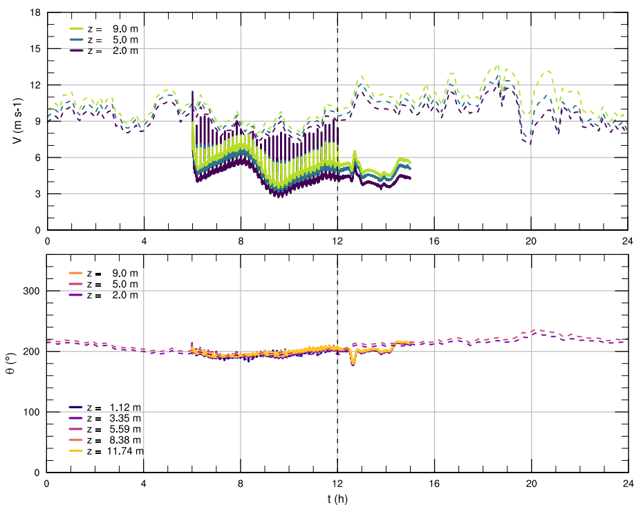
Figura 6.41: Series de tiempo para la rapidez V y dirección \theta del viento en M3 con DA.
