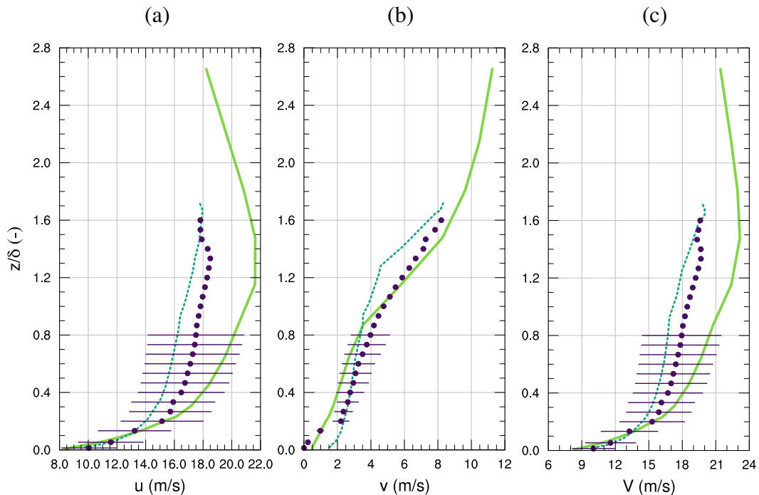
Figura 6.9: Comparación de la simulación con WRF+DA (línea continua) con la simulación de Peña et al. (2013) (línea punteada) y valores medidos para (a) componente longitudinal u de la velocidad del viento, (b) componente transversal v y (c) magnitud de la velocidad del viento. Los datos corresponden a promedios temporales entre las 12:00 y 15:00, y han sido rotados de tal forma que su dirección sea 0^\circ a los 10m sobre el suelo.
