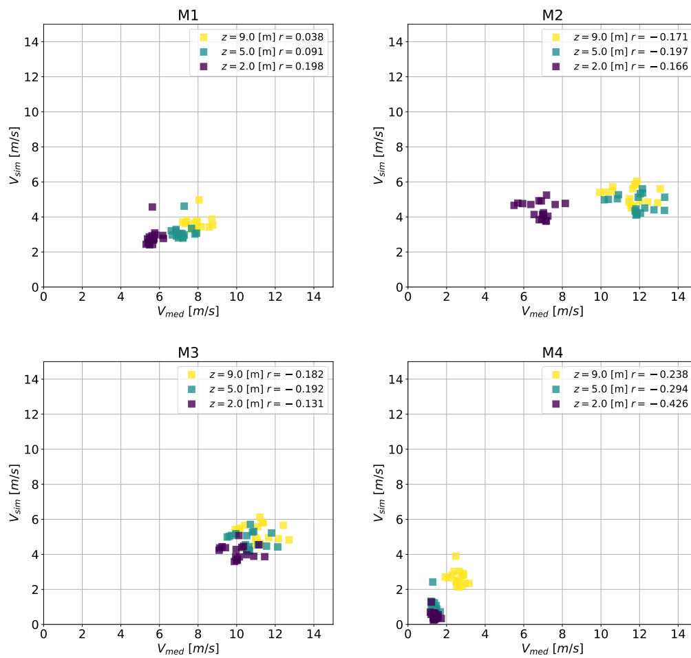
Figura 6.49: Gráfico de dispersión para las velocidades a distintas alturas en los mástiles M1-M4 en Bolund (con DA).
