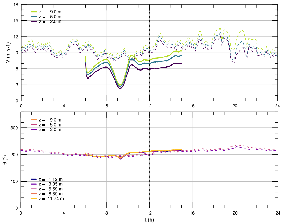
Figura 6.22: Series de tiempo para la rapidez V y dirección \theta del viento en M3.
