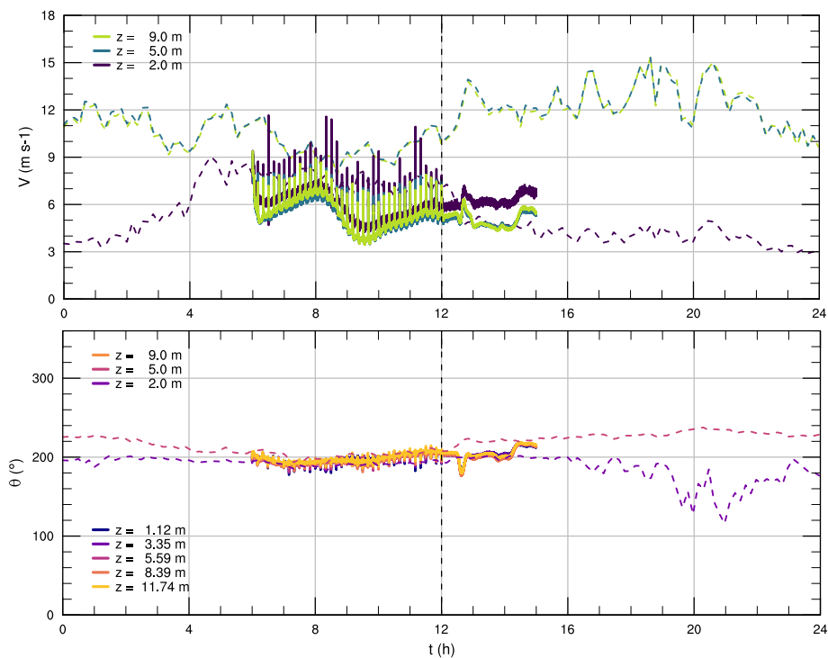
Figura 6.44: Series de tiempo para la rapidez V y dirección \theta del viento en M6 con DA.
