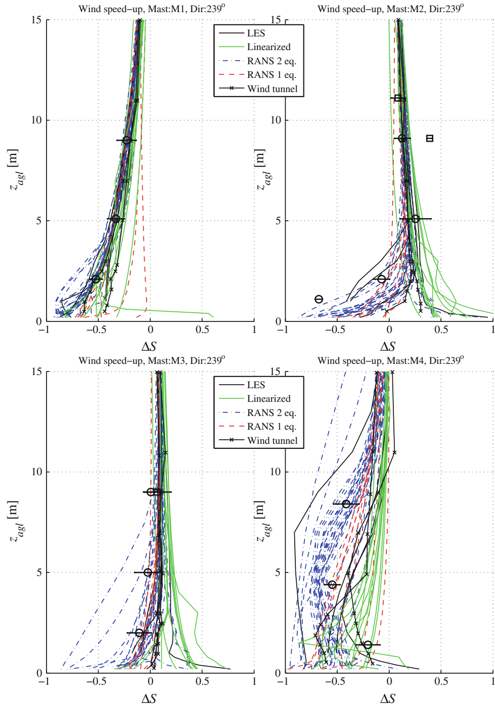
Figura A.3: Perfil de speedup medido y simulado en los distintos mástiles M1-M4.
