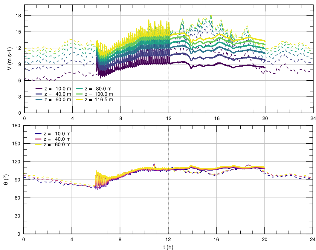
Figura 6.8: Serie de tiempo para la rapidez instantánea del viento V y su dirección en la ubicación del mástil meteorológico para el caso con asimilación puntual de datos. La línea continua corresponde a lo datos simulados interpolados a las alturas de medición (solo para V ) y la línea punteada a los datos medidos en el mástil.
