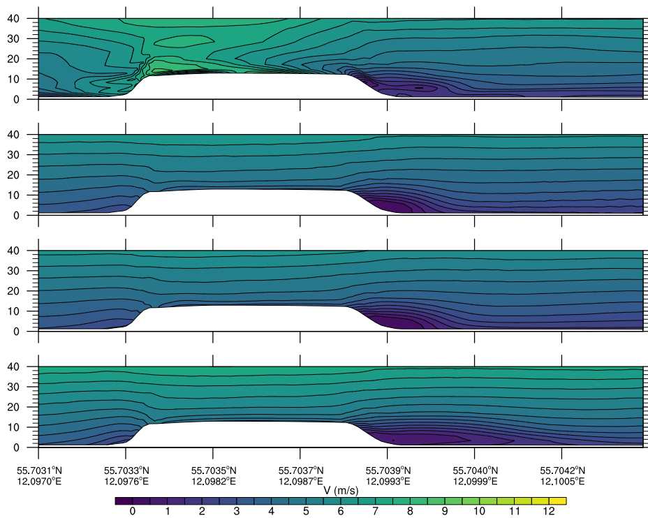
Figura 6.34: Contornos de rapidez del viento para la sección de corte vertical a 240^\circ en Bolund (con DA). Se muestran los resultados para las 12:00 (arriba), 13:00, 14:00 y 15:00 horas (abajo). Escala 1:1.
