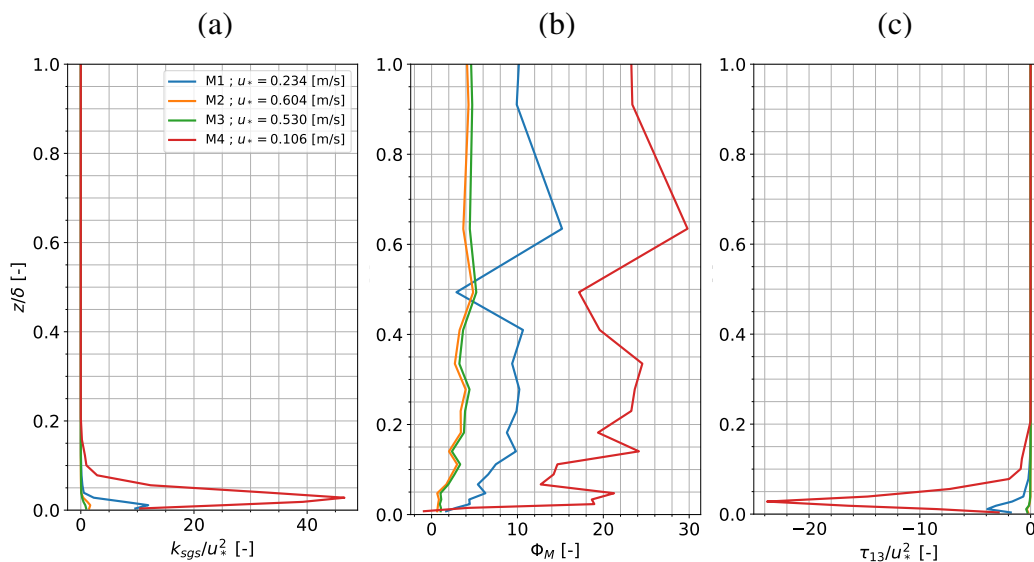
Figura 6.28: Variables adimensionalizadas de segundo orden para M1-M4 promediadas entre las 12:00 y las 15:00. (a) Energía cinética turbulenta de submalla, (b) Gradiente de velocidad, (c) Esfuerzo turbulento.
