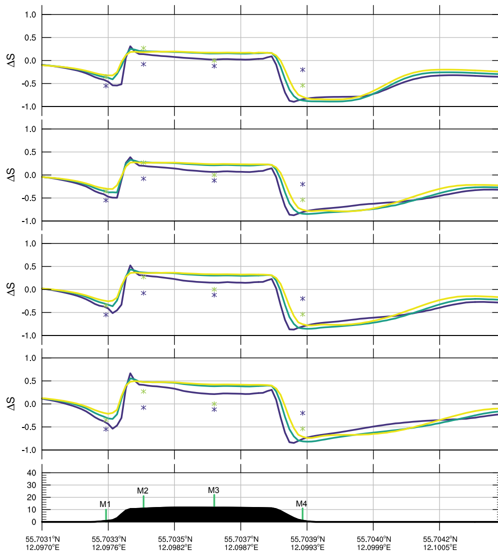
Figura 6.17: Speedup en los primeros 3 niveles del modelo (1,1 [m] azul; 3,4 [m] verde; 5,6 [m] amarillo) para la sección de corte a 240° en Bolund. Se muestran los resultados para las 12:00 (arriba), 13:00, 14:00 y 15:00 horas (abajo).
