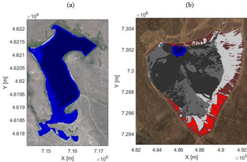
Figura 4-4: Resultado de la clasificación espectral mediante el entrenamiento. (a) Crescent Lake con los tres grupos clasificados; (b) Laguna Seca con los siete grupos clasificados.
