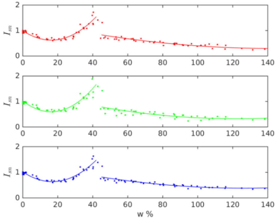
Figura 4–6: Índice normalizado de iluminación activa con láser 980 nm con cámara NIR.
