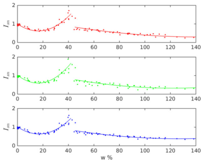
Figura 2–18: Índices iluminación activa laser 980 nm con cámara NIR. Fuente: Araya, 2018.
