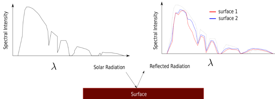
Figura 3-4: Gráficos esquemáticos de la Intensidad espectral. A la izquierda se ve la radiación solar emitida y a la derecha dos superficies de distintas propiedades.
