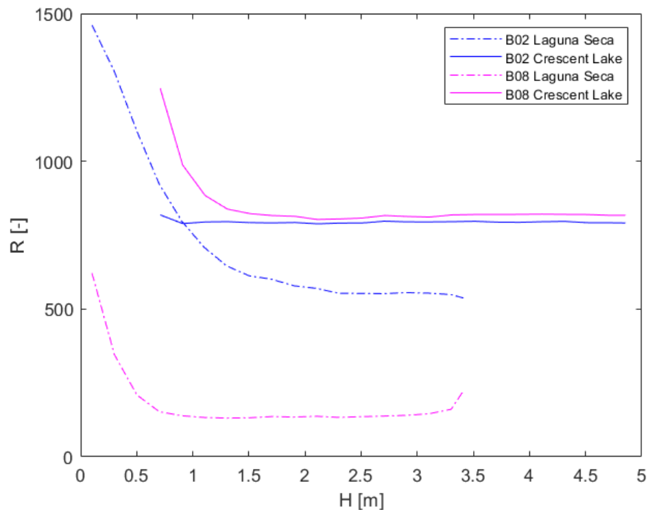
Figura 5-1: Comparación de Curvas de Altura vs Reflexión entre lago estadounidense Crescent Lake (línea continua) y tranque de relave Laguna Seca (línea segmentada). Se muestran las bandas 2 y 8 (azul y magenta respectivamente).
