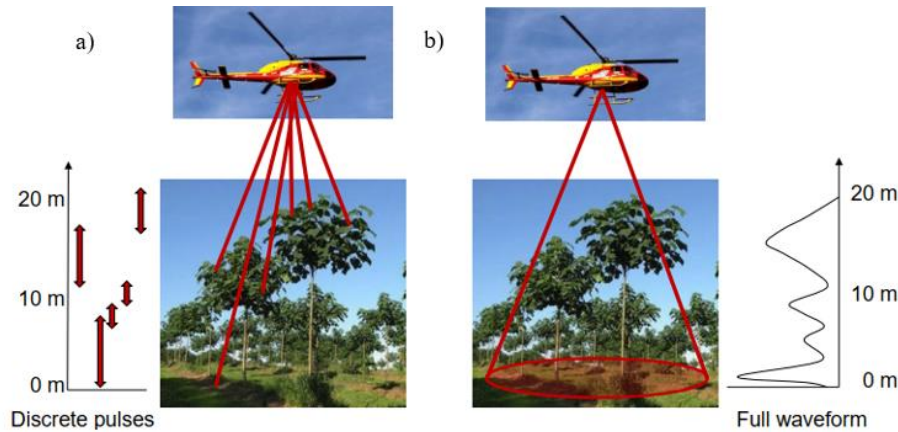
Figura 2–12: Esquema de sistema LiDAR. (a) El pulso láser es emitido de manera discreta; (b) El pulso láser es emitido de manera continua.
