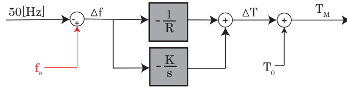
Figura 3.3: Control secundario de frecuencia
