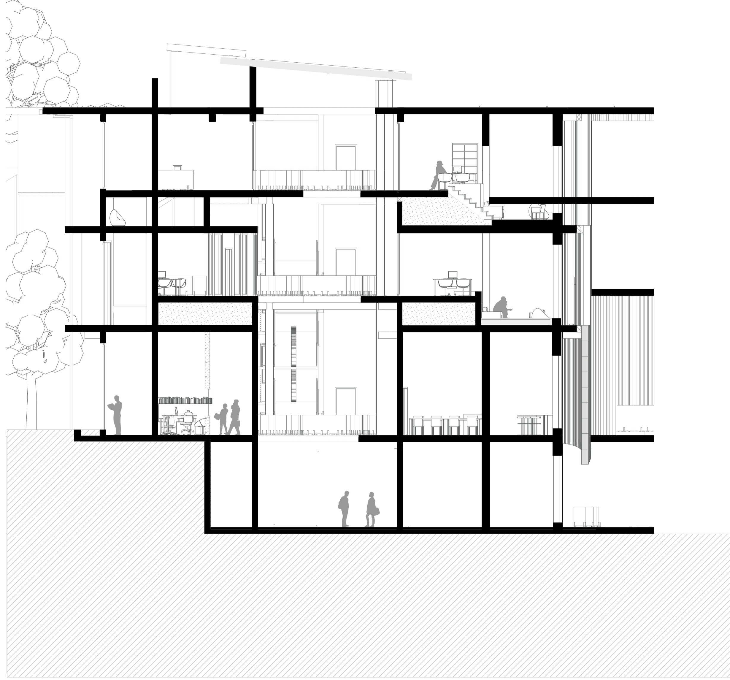
A-A' 1:100
