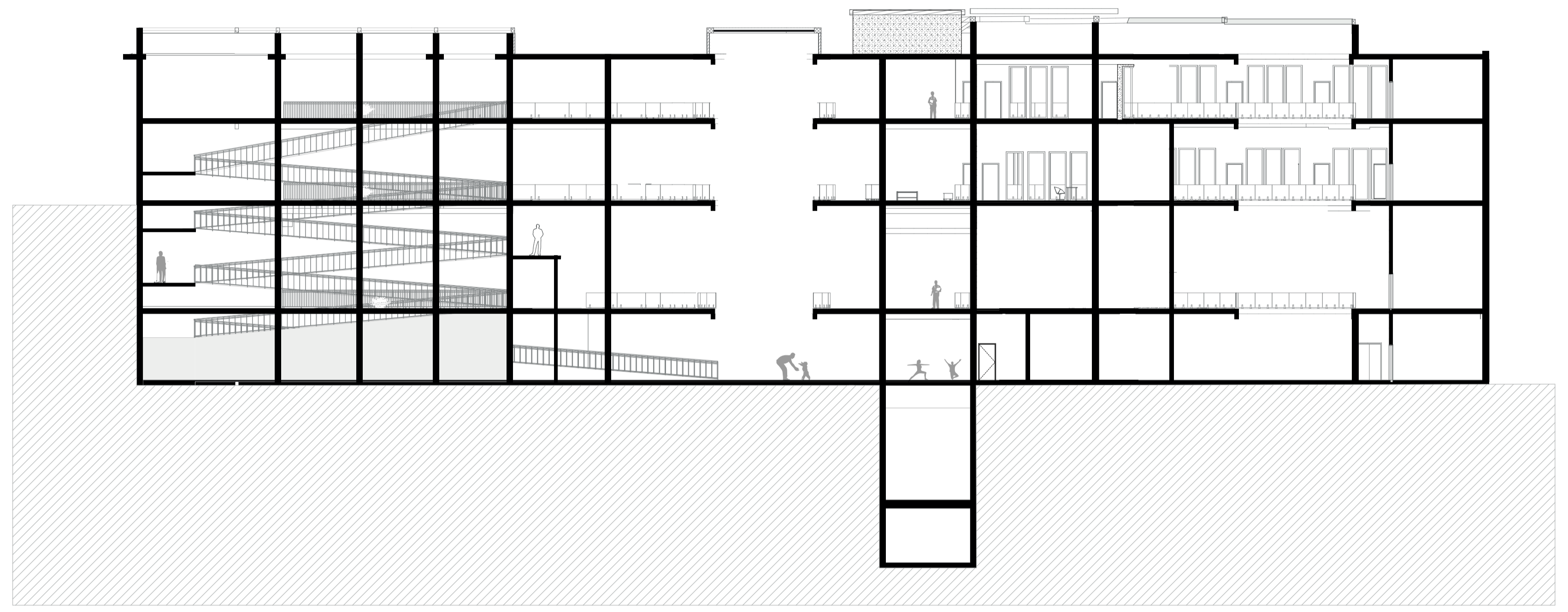
C-C' 1:200
