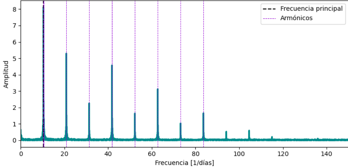
Figura 2.7: Periodograma de HS 0705-6700 tomada por TESS el 2019, en el sector 20 con un tiempo de exposición de 120(s). Se puede ver un pico grande (línea segmentada negra) alrededor de una frecuencia de 10,4551598 (1/d), que corresponde a 0,095644 d o en otras unidades, a 2,2955172813 h. Hacia el lado derecho vemos armónicos de la misma frecuencia (línea segmentada en púrpura).
