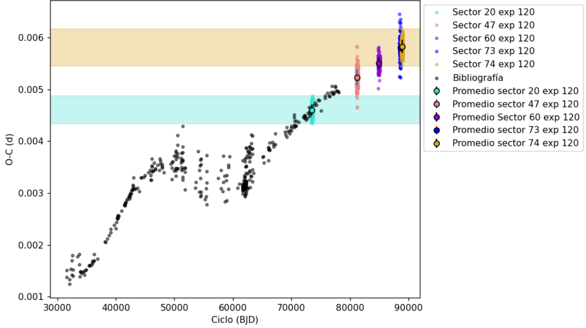
Figura 3.2: Diagrama O-C, los datos en color negro representan los puntos para la información de los mid eclipses encontrados en la literatura, los puntos de colores son datos de TESS para diferentes tiempos de exposición. Se puede ver claramente que no se superponen los puntos del sector 73 (azul) con los del sector 20 (cian) lo cual apoya el postulado de que el sistema eclipsante HS 0705+6700 presenta ETVs (variaciones del tiempo de eclipses) es real.
