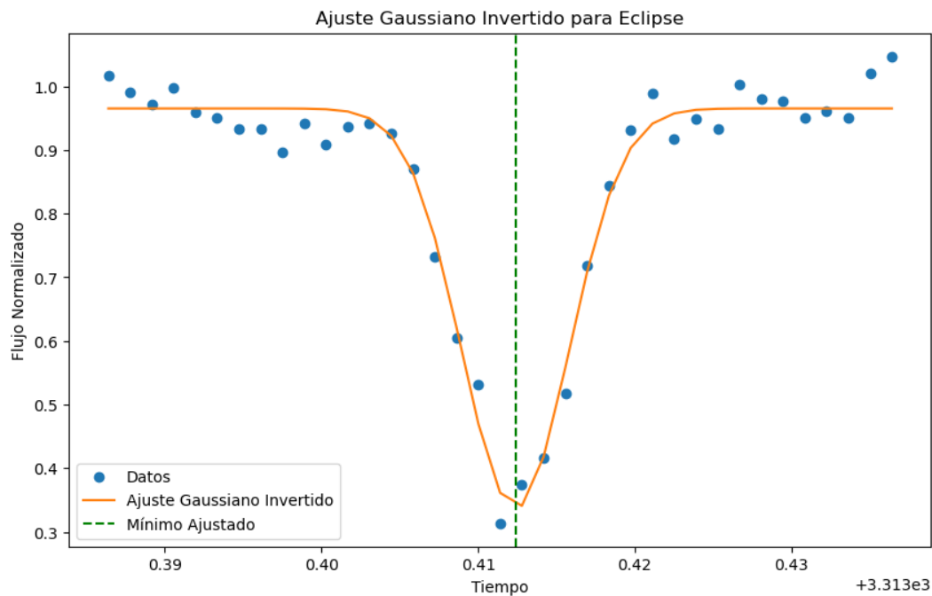
Figura 2.10: Ajuste gaussiano invertido realizado por Pablo para cada eclipse, la linea vertical verde representa el eclipse medio o mid-eclipse ( t_0 en la ecuación 2.3) de acuerdo al ajuste de la guassiana.
