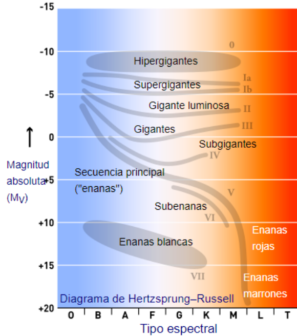
Figura 1.2: Diagrama Hertzsprung-Russell (H-R), representa la evolución de las estrellas, el cual muestra la luminosidad de los distintos tipos de estrellas en función de la temperatura usando la nomenclatura de tipo espectral (O, son estrellas muy calientes y se enfrían hasta llegar a la letra T). Dentro de los distintos tipos de estrellas, 4 tipos son relevantes de entender para esta investigación. Una subenana caliente representa un estado evolutivo avanzado de la estrella donde ha perdido sus capas externas mientras el núcleo aún está quemando helio, se encuentran justo arriba de la palabra secuencia en el diagrama. Luego, las enanas blancas son un tipo de estrellas que tiene aproximadamente la masa del Sol y el tamaño de la Tierra, por lo que se consideran masivas, y que a diferencia de las subenanas calientes estas no están quemando helio. También, estrellas de secuencia principal, son estrellas que, en su núcleo, debido a reacciones nucleares, están haciendo fusión de hidrógeno a helio. Por último, una enana marrón es un tipo de objeto que debido a su baja masa no logra tener reacciones nucleares en su núcleo (Carroll and Ostlie, 2017).
