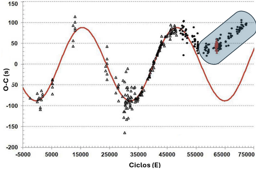
Figura 1.3: Diagrama O-C presentado por Faillace et al. (2019a) . Se puede ver como en los últimos ciclos hay un comportamiento diferente respecto a los diagramas O-C para sistemas binarios eclipsantes que presentan un comportamiento sinusoidal y comienzan a subir los datos en el eje y, los datos resaltados en el gráfico (ovalado celeste), lo que indica que la órbita está aumentando su radio.
