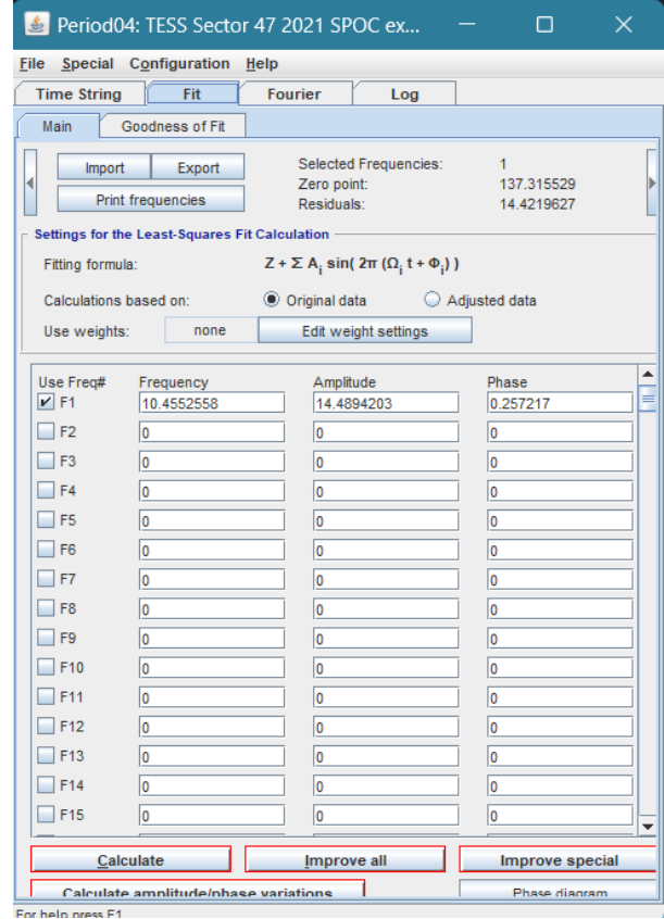
Figura 2.6: Izquierda: Imagen de la pestaña Fourier del programa PERIOD04, se puede ver el rango de frecuencias escogido, en este caso, para el sector 73 con tiempo de exposición 120(s), también en base a que datos se va a calcular la frecuencia y finalmente la frecuencia. Derecha: Imagen de la pestaña Fit del programa PERIOD04, se puede ver cual es la formula para ajustar la curva.
