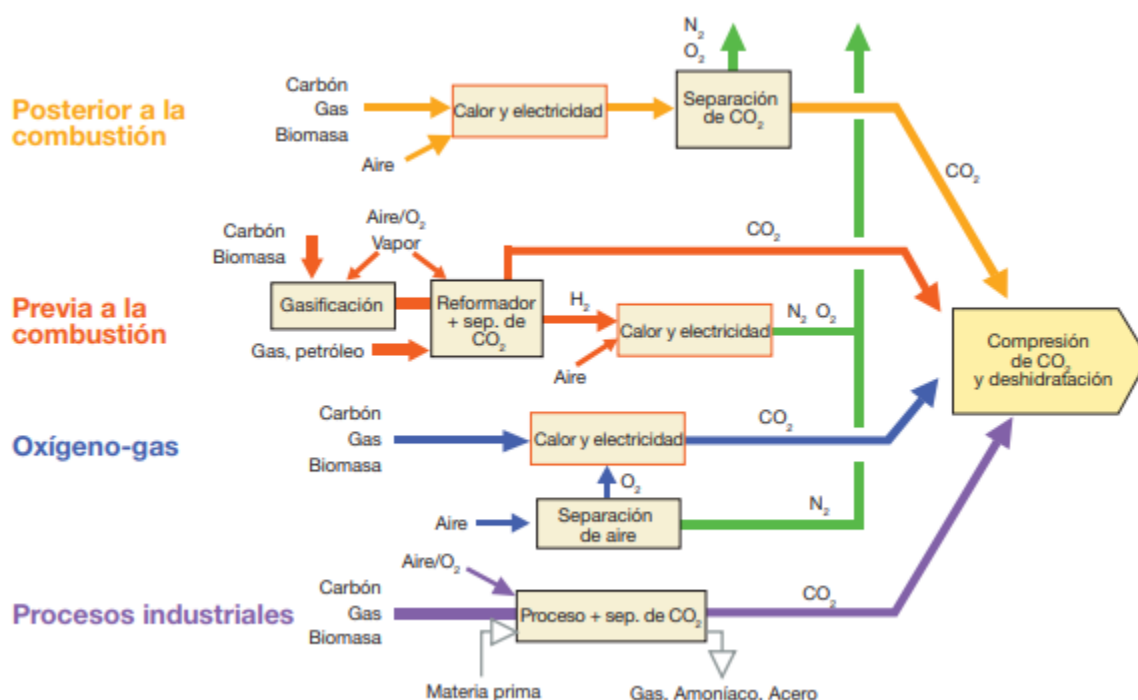
Figura 8: Visión general de los procesos y los sistemas de captación de dióxido de carbono.
