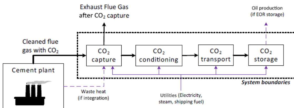
Figura 7: Estructura de bloques y límites para la captura de dióxido de carbono en la industria del cemento. Fuente: Jakobsen, Roussanly & Anantharaman (2017).
