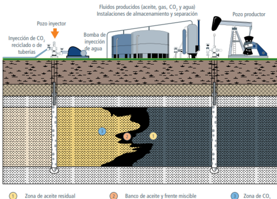
Figura 10: Proceso gráfico de la inyección de dióxido de carbono en un pozo petrolero, para la realización de la recuperación mejorada de hidrocarburo. Fuente: Santamaria (2018).
