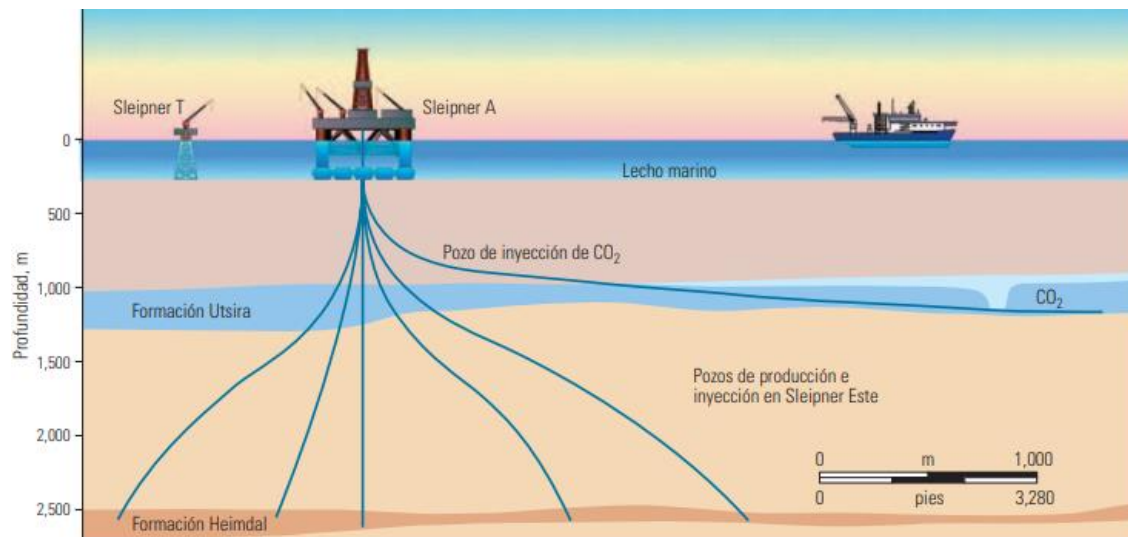
Figura 4: Separación del dióxido de carbono del gas natural producido en la Formación Heimdal, que luego es inyectado en la Formación Utsira. Fuente: Bennaceur, et al., 2017.
