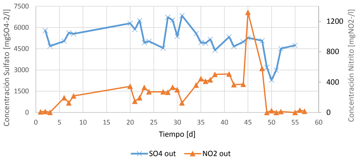
Figura 30. Acumulación de productos intermedios y finales de la metabolización de compuestos en el ril
