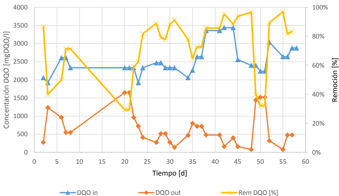
Figura 28. Remoción de materia orgánica medida como DQO, durante operación en continuo
