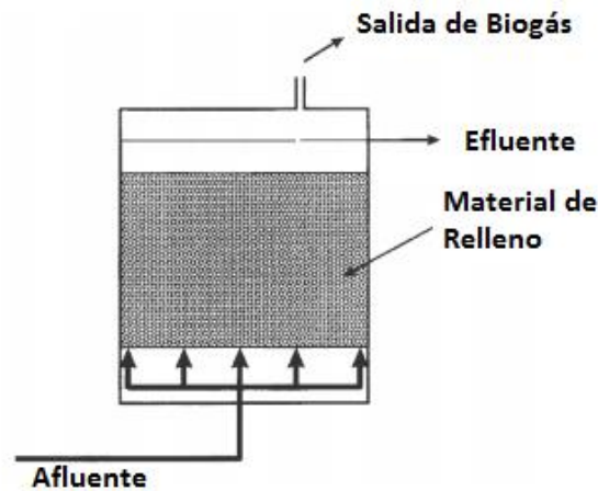
Figura 18. Bosquejo de filtro anaerobio de flujo ascendente (Adaptado de: Dahab, 1982)
