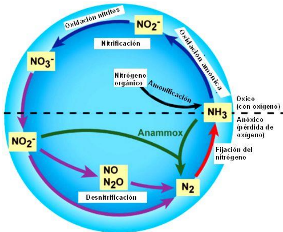
Figura 2. Ciclo del nitrógeno en la naturaleza (Elaboración propia)
