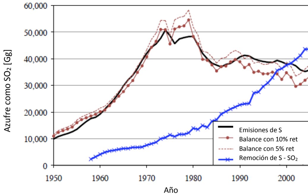
Figura 5. Emisiones de azufre como dióxido de azufre a partir de la quema de petróleo y la acción mitigadora de las refinerías (Adaptado de: Smith et al., 2011).
