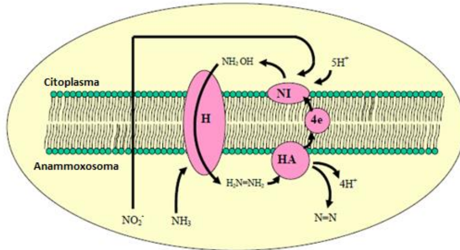
Figura 13. Ruta metabólica en bacteria anammox (Adaptado de: Karthikeyan y Joseph, 2006)
