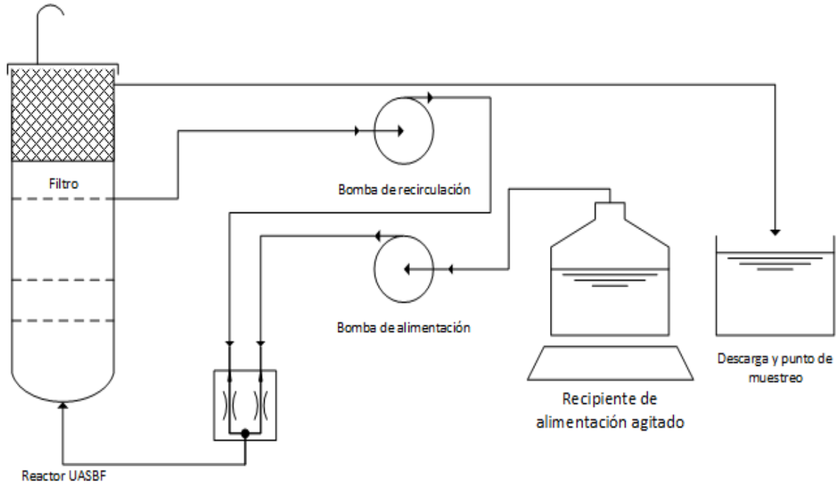
Figura 22. PFD del reactor con su respectivo sistema de alimentación y descarga
