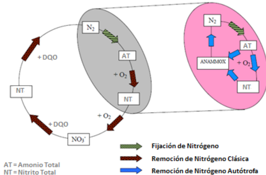
Figura 12. Proceso anammox inserto en el ciclo global del nitrógeno (Adaptado de: Karthikeyan y Joseph, 2006)
