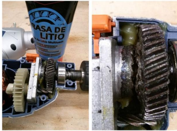
Figura 2- 26 Engranajes de un taladro
