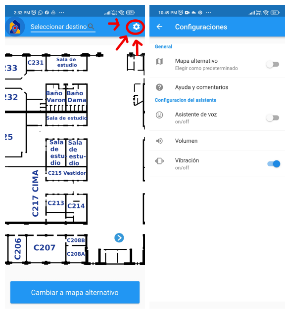
Figura 28: Izquierda: seleccionar configuraciones, Derecha: configuraciones.
