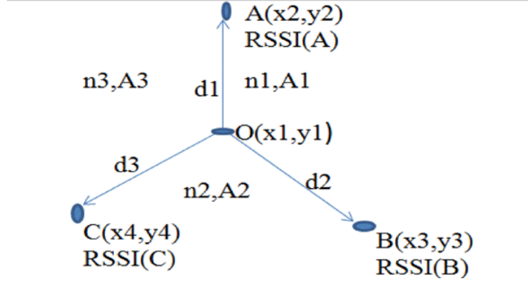
Figura 5: Esquema de triangulación.
