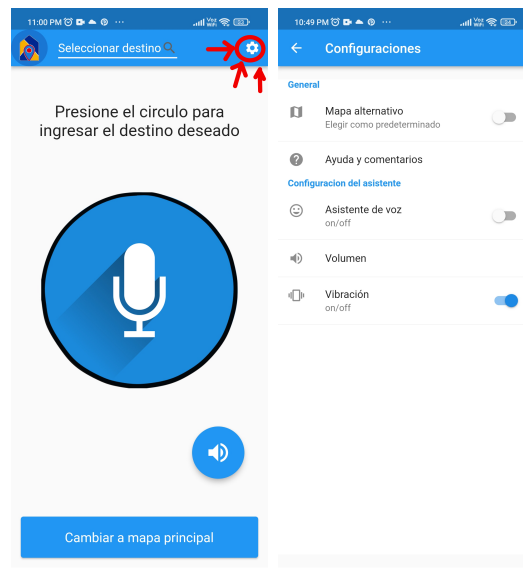
Figura 30: Izquierda: mapa alternativo, Derecha: menú configuraciones.
