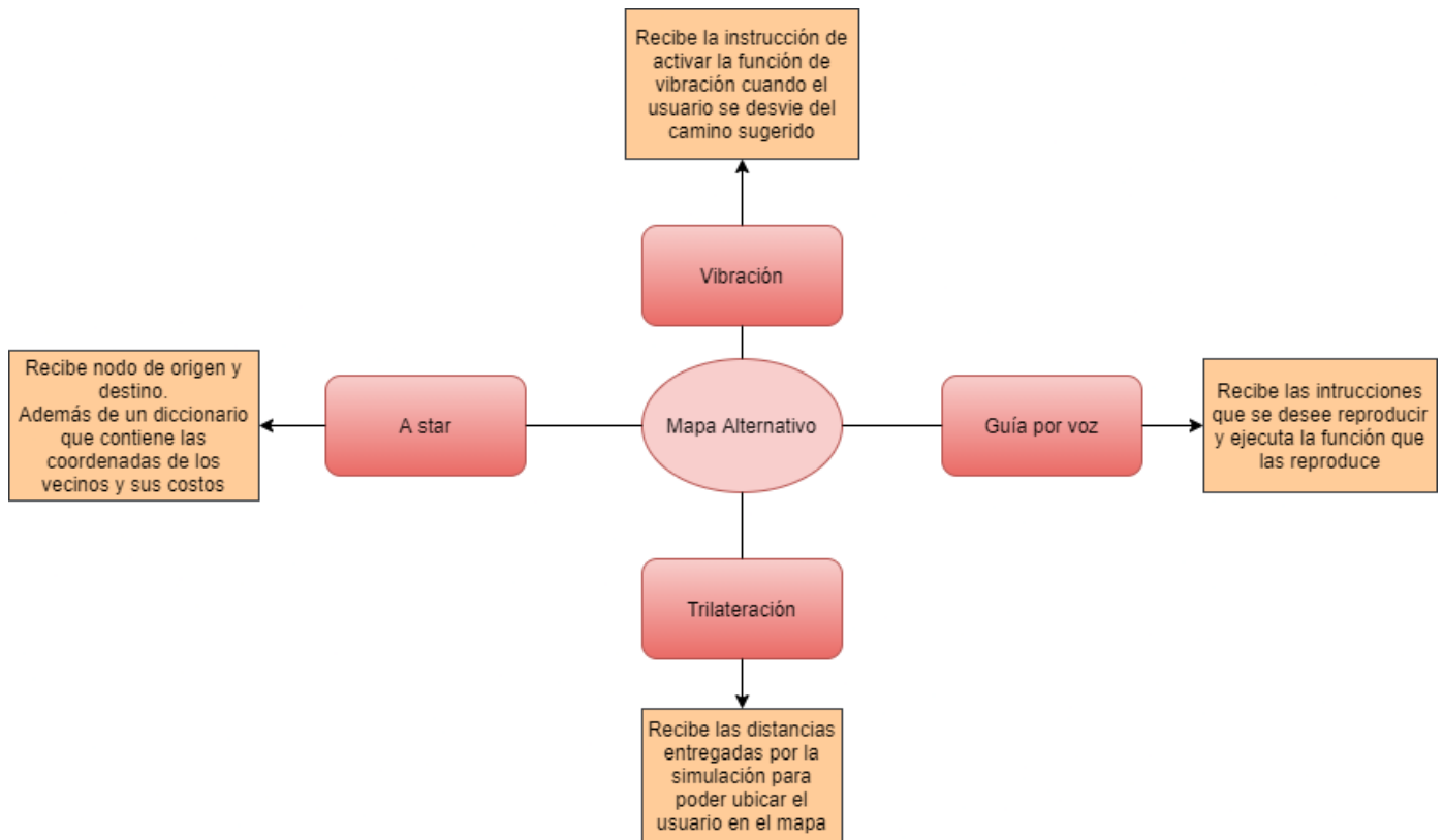
Figura 20: Funciones del mapa alternativo
