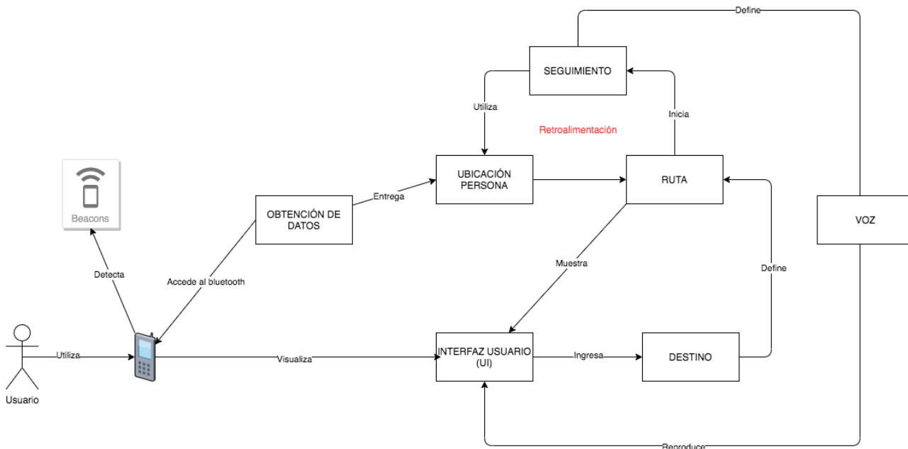
Figura 3: Esquema general del sistema
