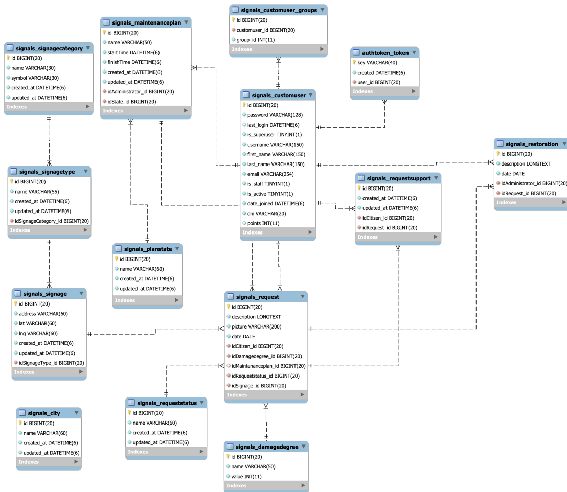
Figura 4.1: Diagrama De base de Datos simplificado
