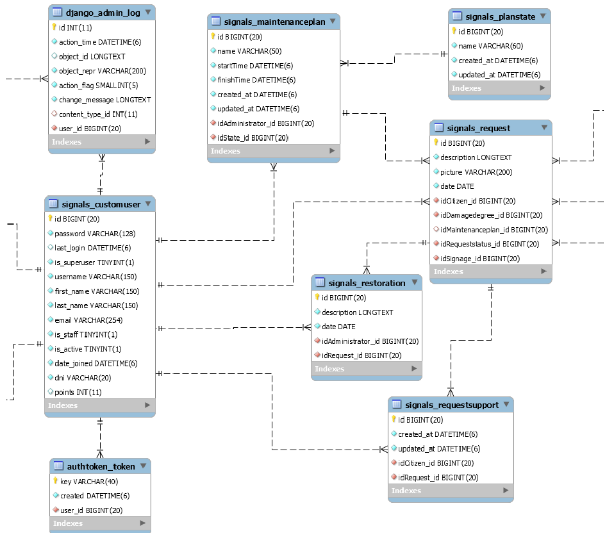
Figura A.2: Base de datos completa del sistema pt.2
