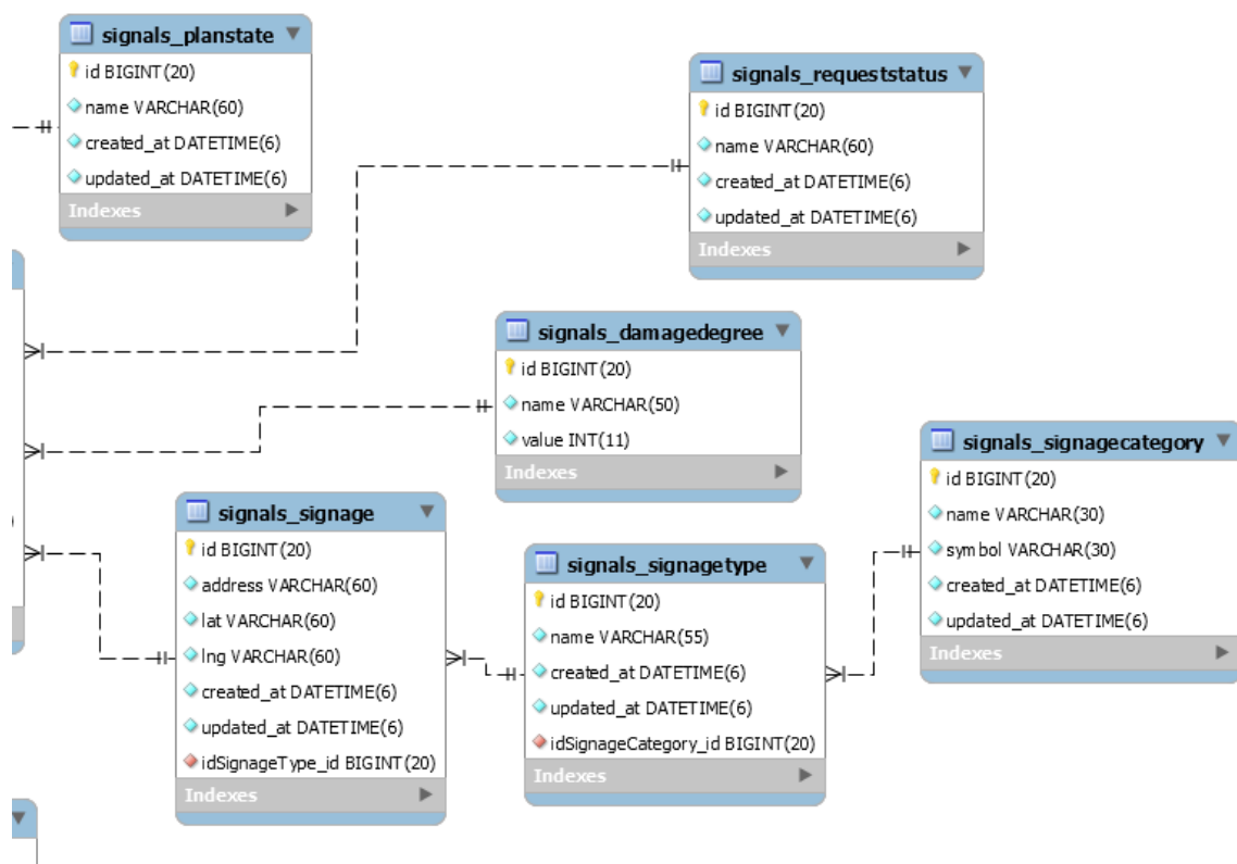
Figura A.3: Base de datos completa del sistema pt.3
