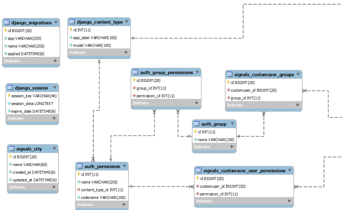
Figura A.1: Base de datos completa del sistema pt.1
