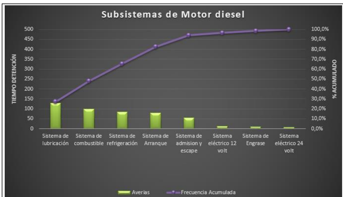
Fig. 1.6.5 Diagrama Pareto Subsistemas Motor diesel Camión 12.
