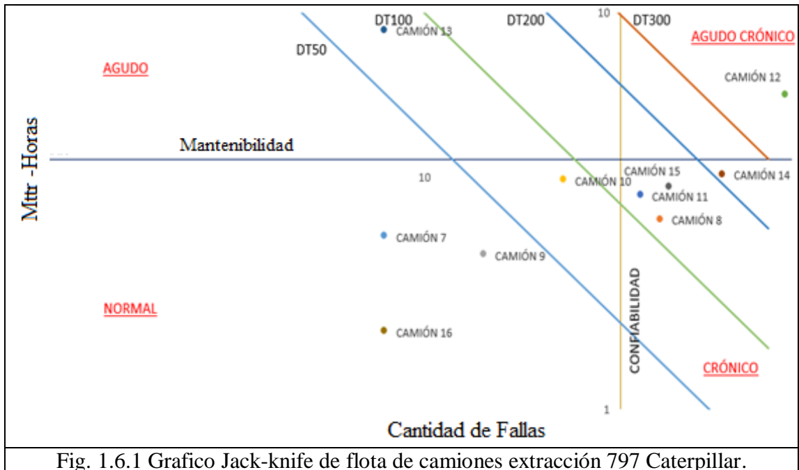
Fig. 1.6.1 Grafico Jack-knife de flota de camiones extracción 797 Caterpillar. Fuente: Fuente: Elaboración Propia apoyo Historial de detenciones por imprevistos.
