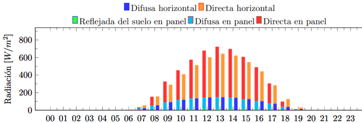
Imagen 23: Promedio horario de la radiación global instantánea incidente en un plano horizontal y en un plano inclinado, separada en sus componentes directa, difusa y reflejada en el suelo
