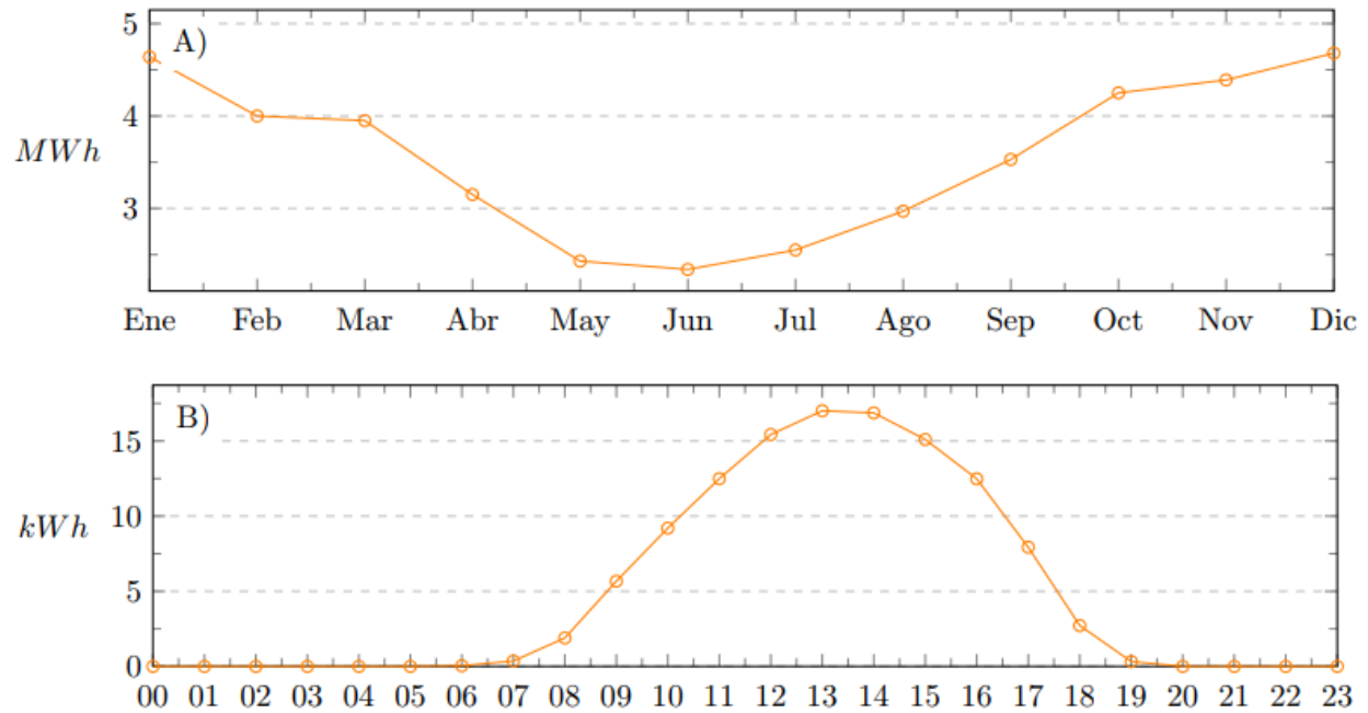
Imagen 16: A) Ciclo anual de generación, B) Ciclo diario de generación
