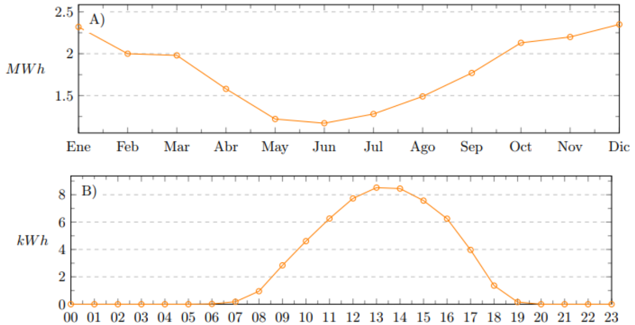
Imagen 13:A) Ciclo anual de generación, B) Ciclo diario de generación.
