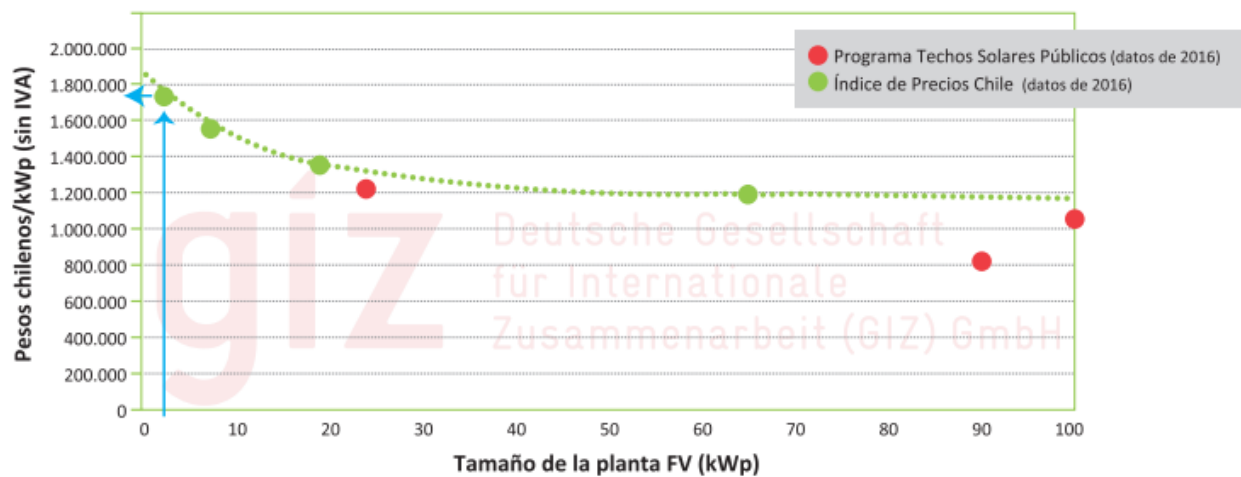
Imagen 27: Precio neto $/kWp respecto al tamaño de la planta FV kWp
