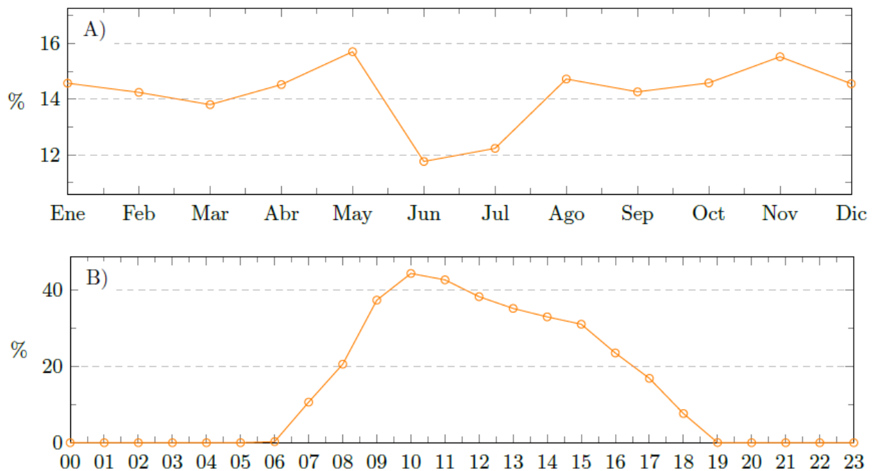
Imagen 24:A) Ciclo anual de frecuencia de nubosidad diurna, B) Ciclo diario de frecuencia de nubosidad.
