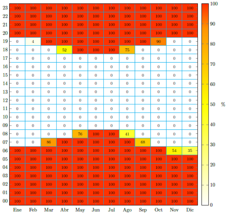
Imagen 21: Porcentaje de la hora con sombras durante cada mes.
