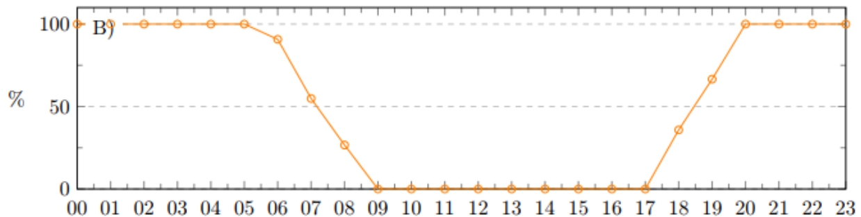
Imagen 12: Ciclo diario de frecuencia de sombras.
