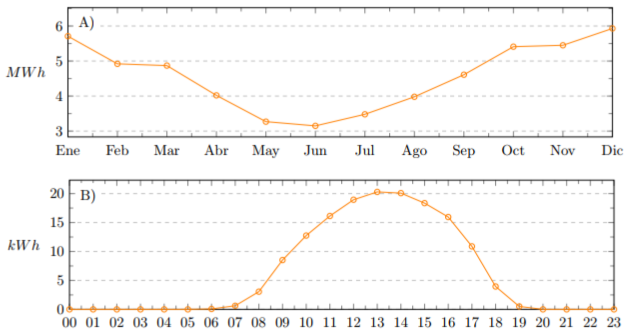
Imagen 18: A) Ciclo anual de generación, B) Ciclo diario de generación.
