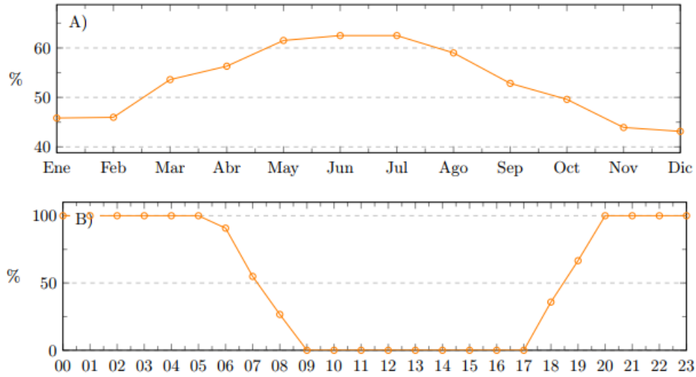
Imagen 20:A) Ciclo anual de frecuencia de sombras, B) Ciclo diario de frecuencia de sombras.
