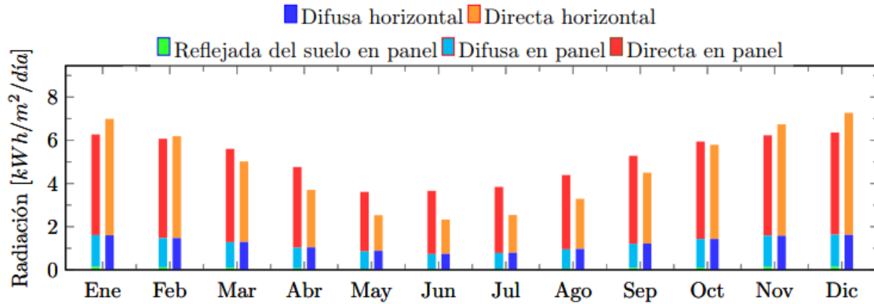
Imagen 22: Promedio mensual de la insolación diaria incidente en un plano horizontal y en un plano inclinado separada de sus componentes directa, difusa y reflejada del suelo
