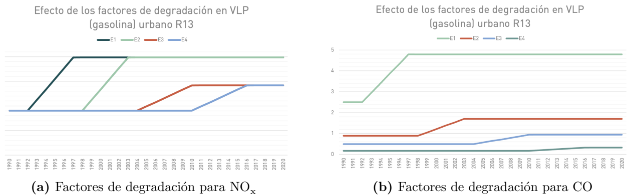
Figura 3.3: Factores de degradación para VLP urbano en la RM
