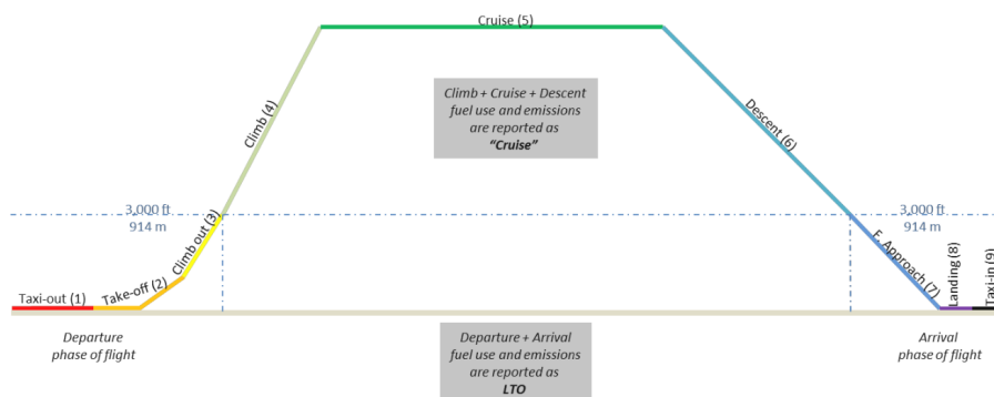
Figura 2.4: Etapas de un vuelo y agrupación en categorías para inventarios.
