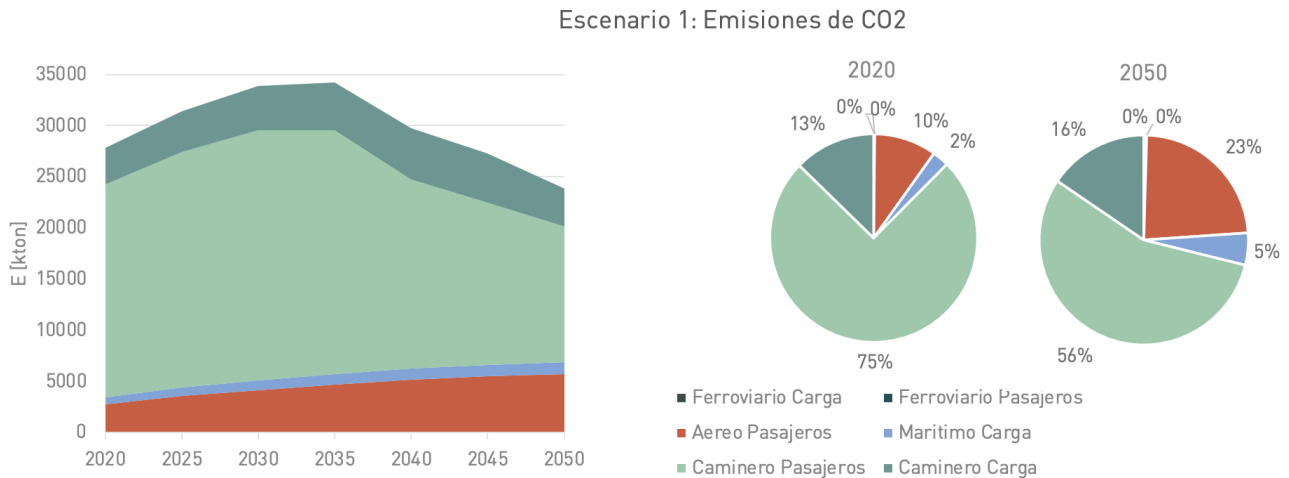
Figura 4.7: Emisiones de CO 2 para Escenario Base
