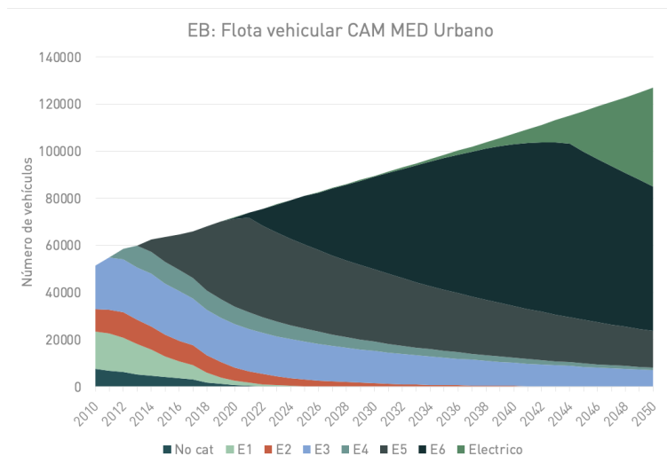
Figura 4.2: Escenario base: flota vehicular camiones medianos
