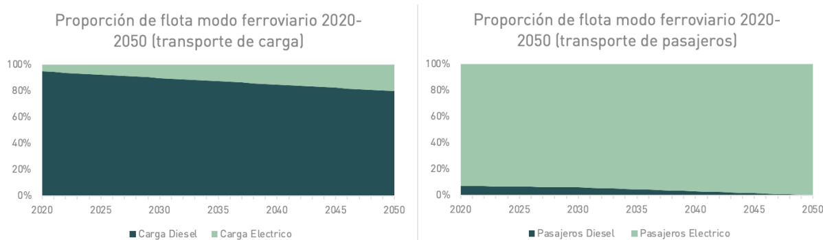
Figura 4.5: Escenario base: flota ferroviaria
