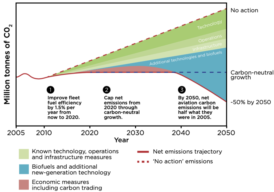
Figura 2.5: Emisiones del modo aéreo sin acciones y metas de reducción de emisiones de la industria
