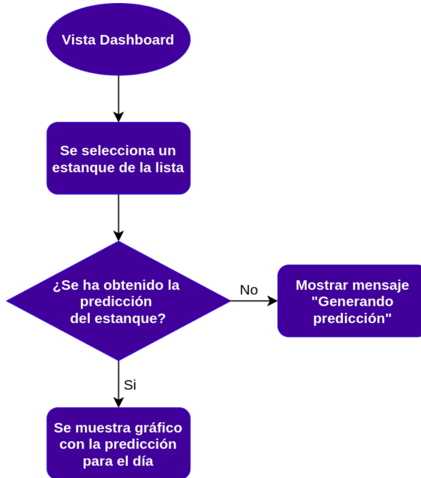
Figura 4.16: Diagrama de flujo de obtención de la predicción en vista de dashboard.
