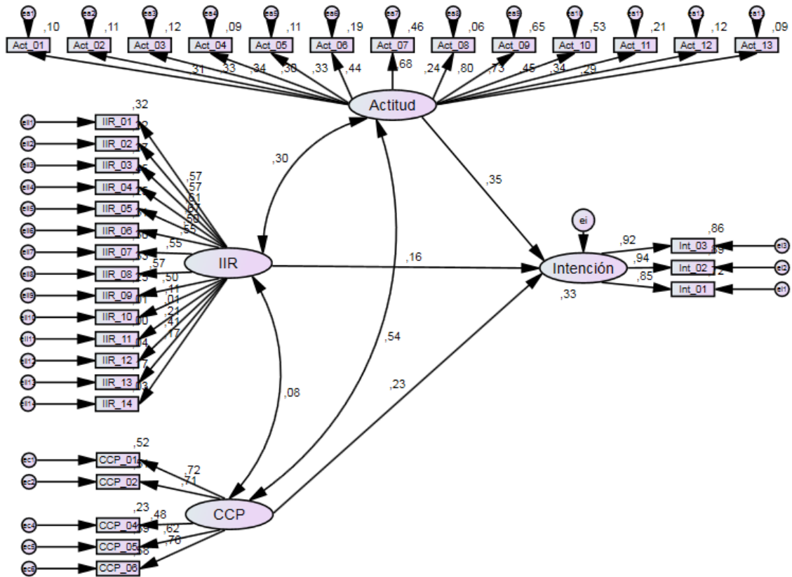
Ilustración 8: Modelo ecuación estructural resultante, eliminando variables no significativas. Fuente: Elaboración propia.
