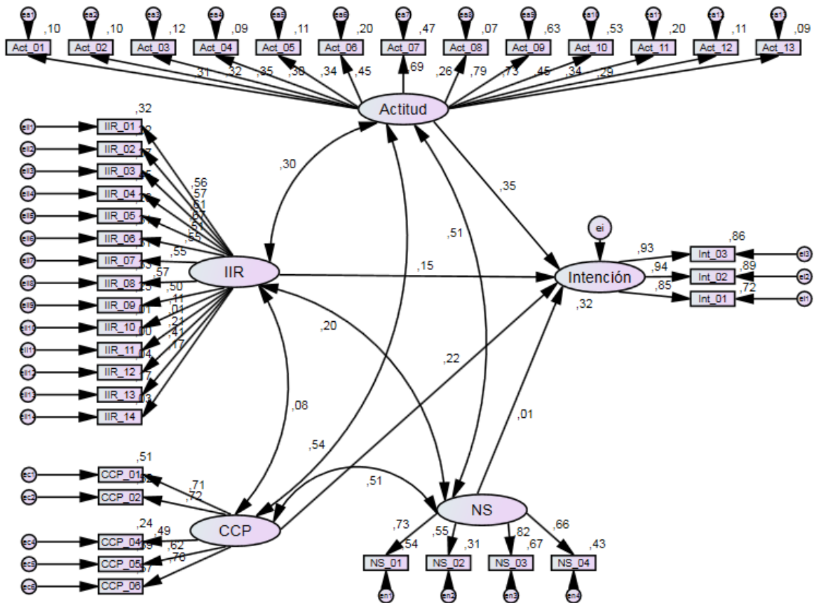
Ilustración 7: Modelo de ecuación estructural resultante
