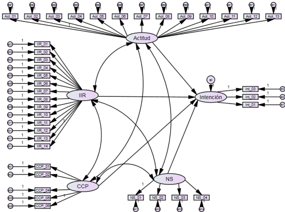
Ilustración 6: Modelo de ecuaciones estructurales.
