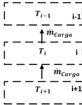
Figura 6.3: Balance energía del nodo i del termo eléctrico (Fuente: Fuente: Adaptación Trnsys 17 Documentation, 4 Mathematical Reference)
