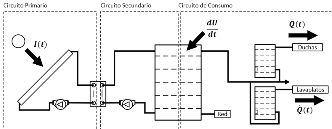
Figura 6.1: Esquema básico de una instalación termosolar centralizada (Fuente: Adaptación SSTII )
