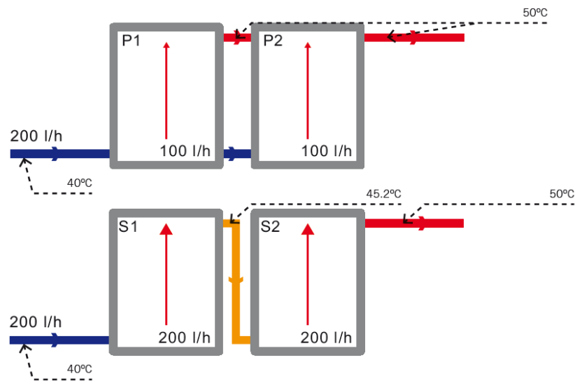
Figura 9.6: Ejemplo conexión serie paralelo de los colectores (Fuente: Sistemas Solares Térmicos II.)
