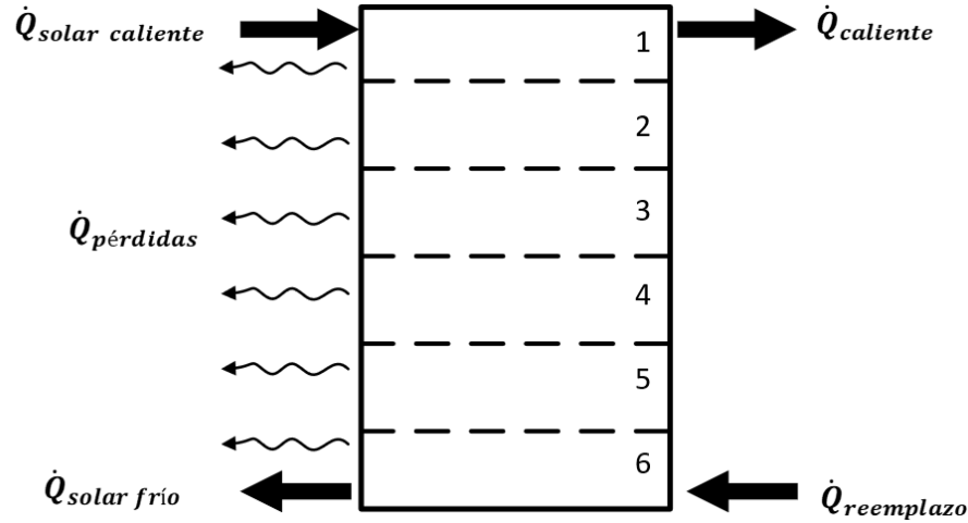
Figura 6.5: Balance energía del estanque central (Fuente: Adaptación Trnsys 17 Documentation, 4 Mathematical Reference)
