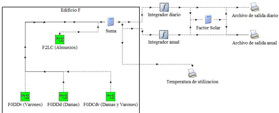
Figura 8.2: Esquema general de simulación de producción de ACS distribuida actual (Fuente: Trnsys 17)
