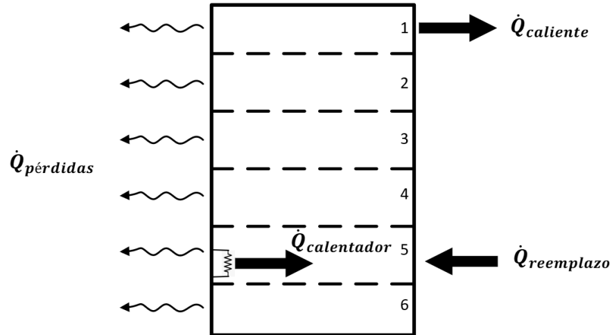
Figura 6.2: Balance energía del estanque con calentador eléctrico (Fuente: Adaptación Trnsys 17 Documentation, 4 Mathematical Reference)
