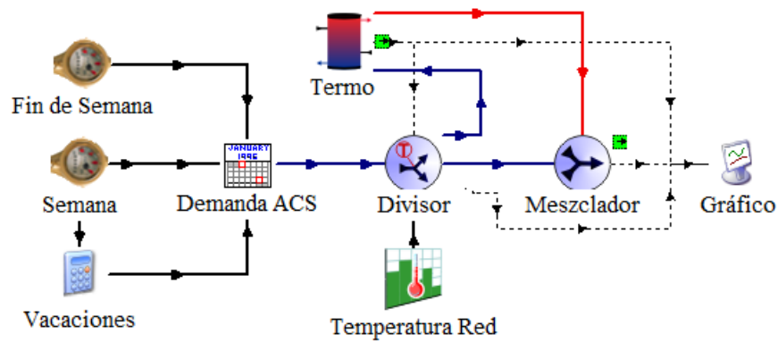
Figura 8.1: Esquema de simulación de un termo eléctrico distribuido (Fuente: Trnsys 17)
