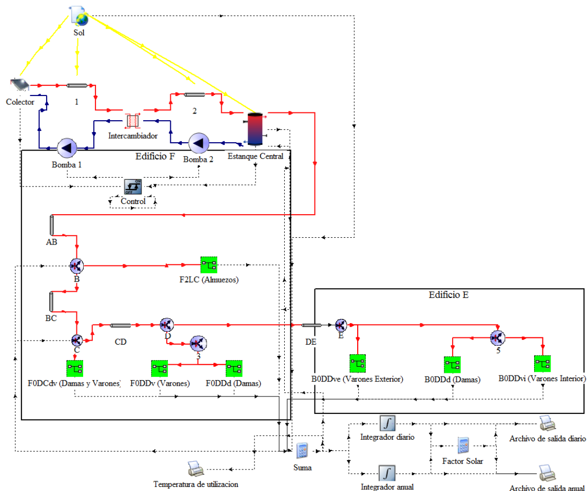
Figura 8.8: Esquema de simulación del sistema solar térmico centralizado (Fuente: Trnsys 17)
