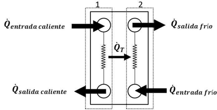
Figura 6.7: Balance energía del intercambiador de calor (Fuente: Adaptación Trnsys 17 Documentation, 4 Mathematical Reference)
