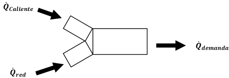
Figura 6.4: Balance energía de la válvula termostática
