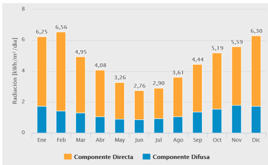
Fig 30. Radiación Global horizontal
