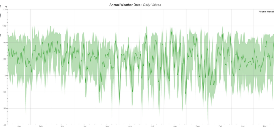
Fig 29. Humedad Relativa anual
