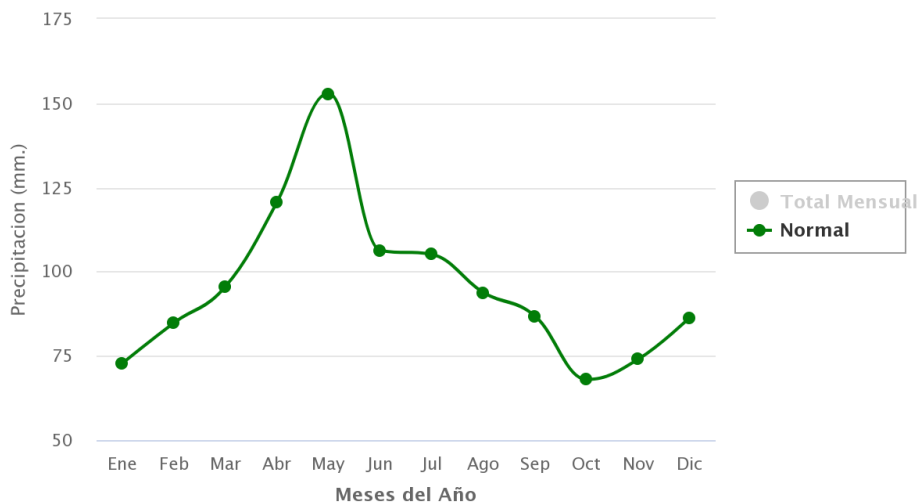
Fig.21 Precipitación mensual Normal 30 años
