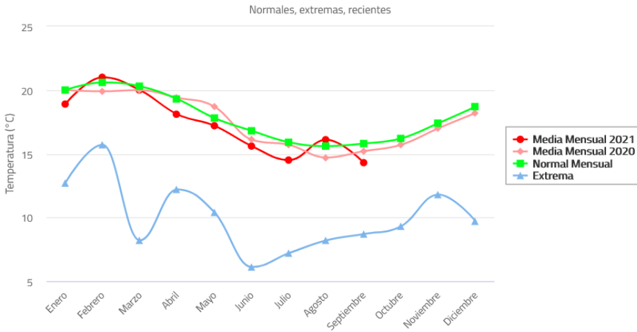
Fig 19. Temperatura mínima media mensual histórica entre 1954 y 2021
