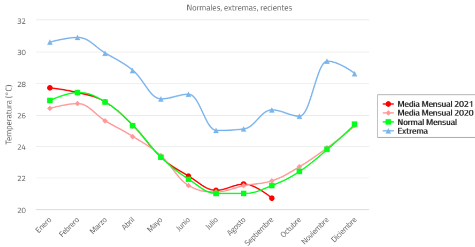
Fig 20. Temperatura máxima media mensual histórica entre 1954 y 2021
