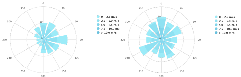
Fig 27. De izquierda a derecha Rosa de los vientos otoño, invierno.
