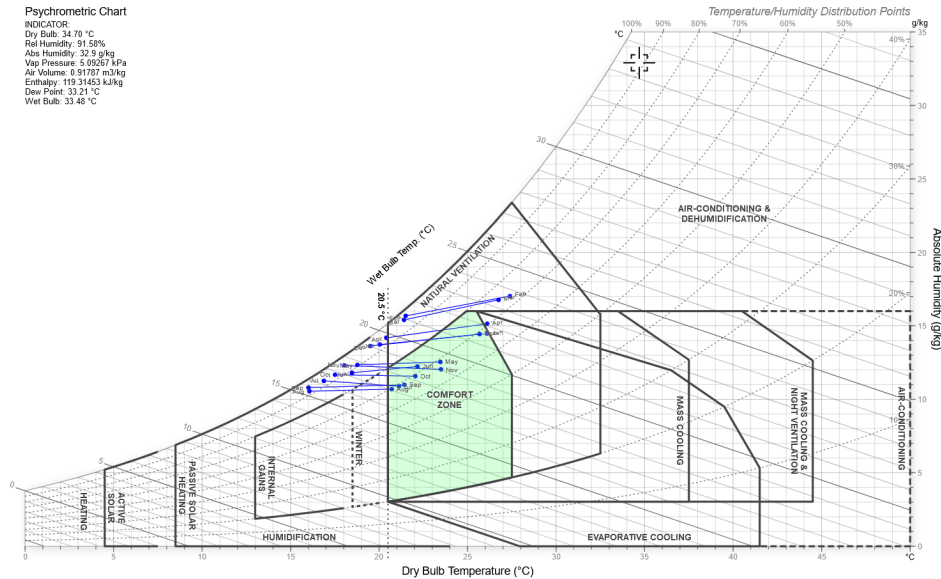
Fig 32. Diagrama Bioclimático de Givoni Fuente: andrewmarsh.com
