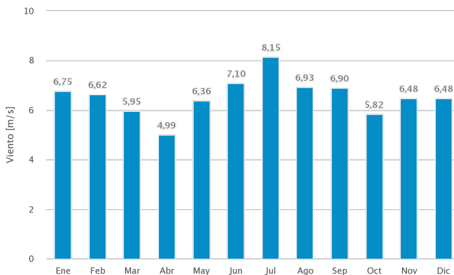
Fig 24. Promedio anual mensual de velocidad del viento
