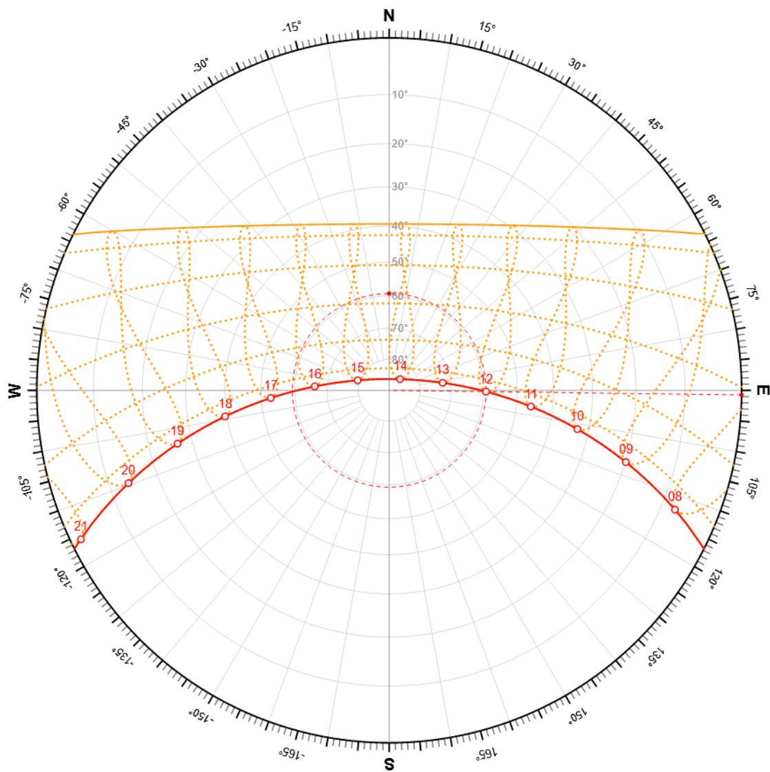
Fig 31. Carta solar Rapa Nui (trayectoria solsticio de verano)
