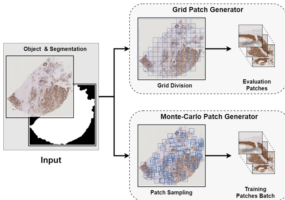
Figura 11: Patch Generators - Un objeto identificado puede ser convertido en un conjunto de pequeñas imágenes para ser utilizadas por un modelo de DL. Se disponen de dos estrategias de división: grid , para una división determinista sin superposición; o sampling para generar muestras aleatorias de toda la imagen.
