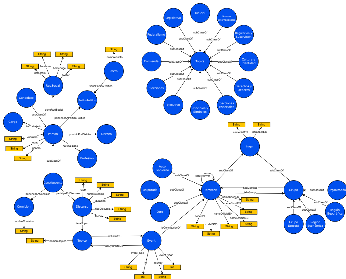
Figura 49: Representación gráfica de la ontología propuesta. Se consideró sólo un nivel de profundidad para los tópicos CCP. Fuente: elaboración propia.
