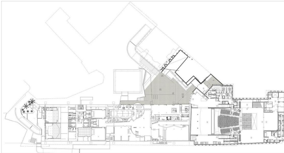
Planta nivel 1
