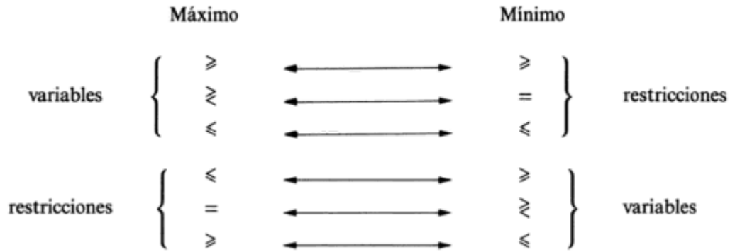
Figura 2.2: Relaciones entre el problema primal y el dual
