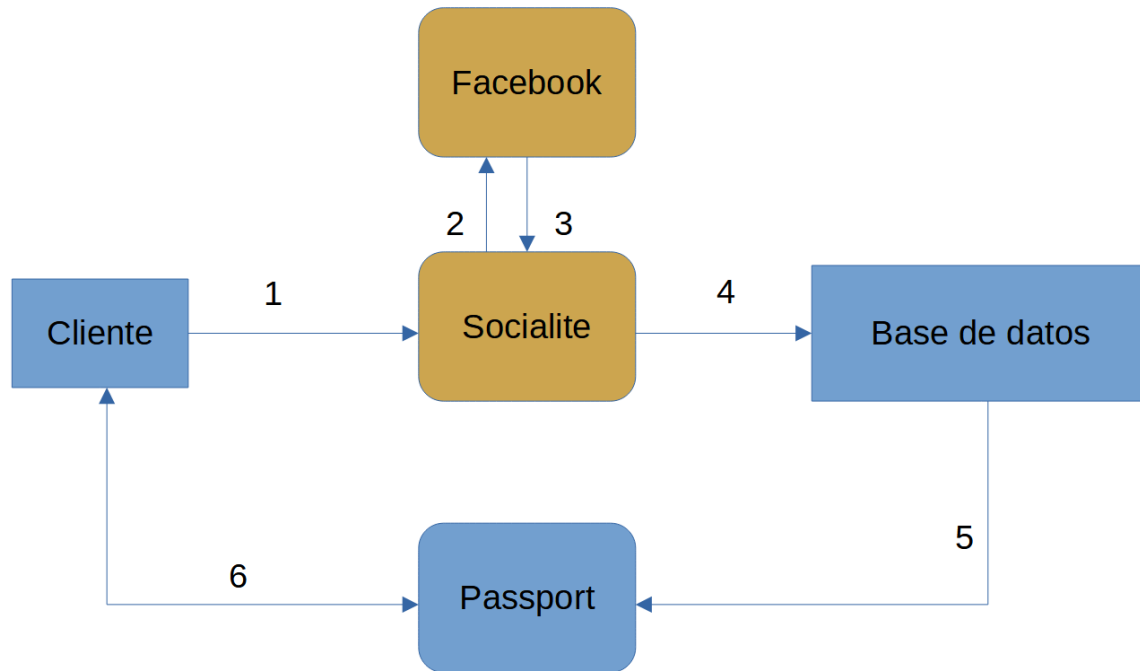
Figura 3.2: Modelo del flujo de la autenticación
