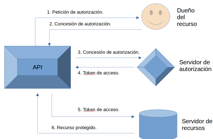
Figura 2.4: Modelo de autenticación con OAuth2.0
