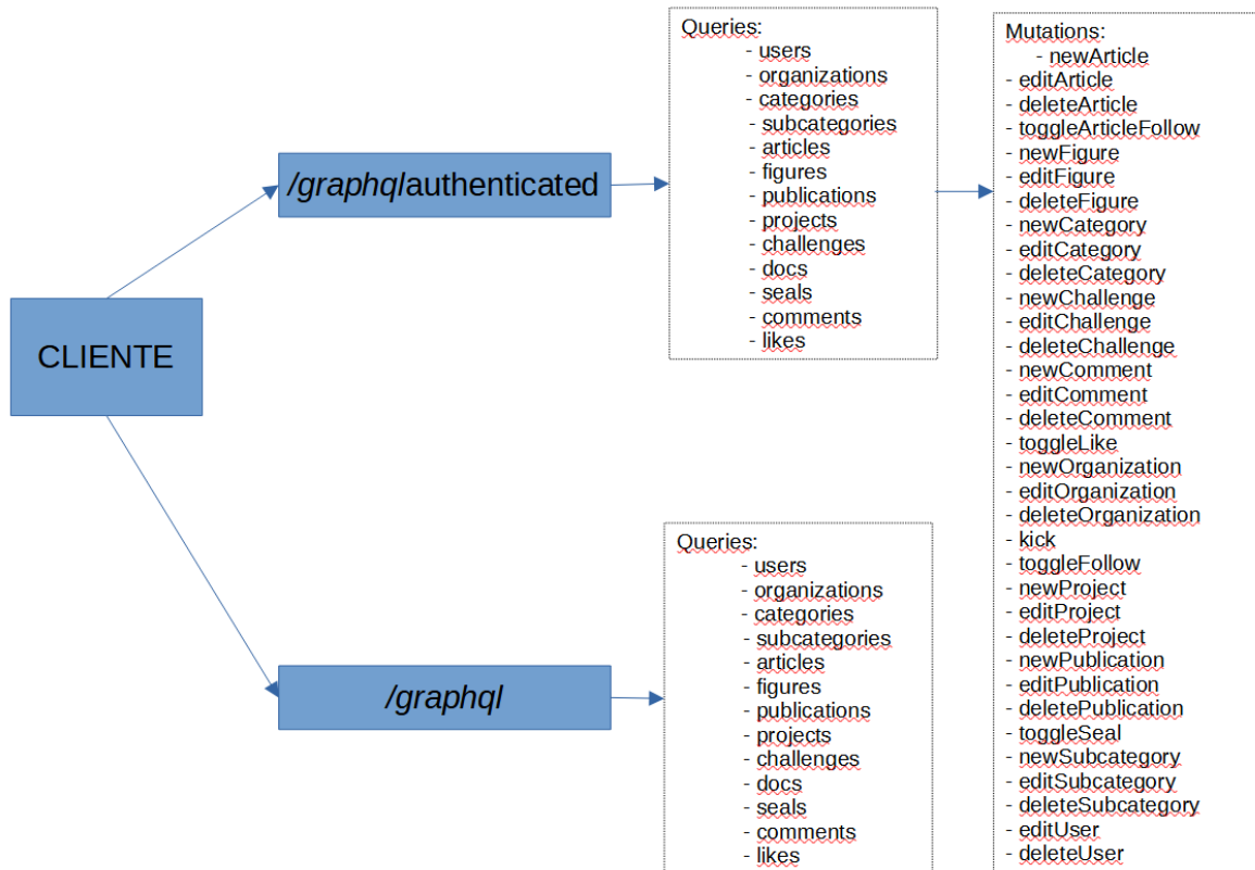
Figura 3.1: Modelo de esquema graphql para queries y mutaciones
