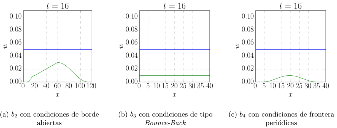
Figura 7.5: Algunos resultados de la simulación de lago en reposo.
