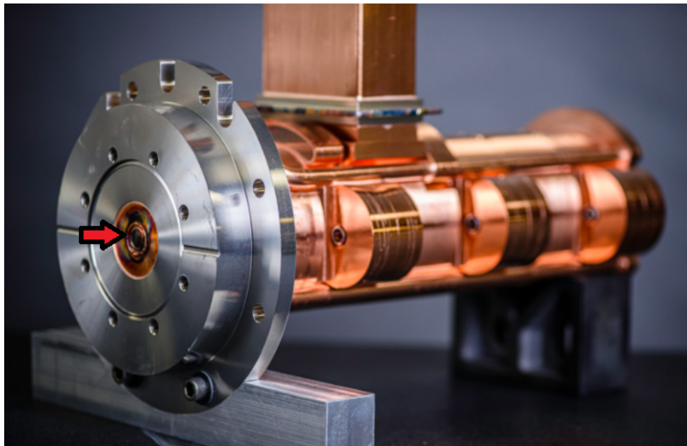
Figura 3.23: Ejemplo de aplicación de unión con técnica de Soldadura Fuerte. [16]
