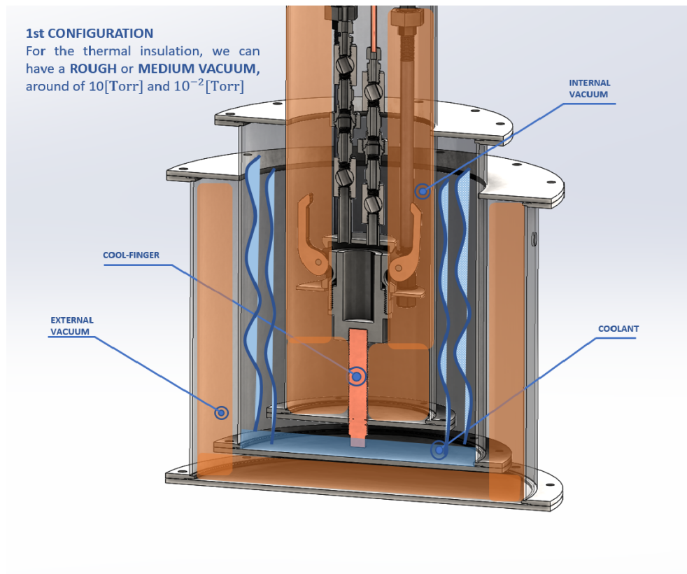
Figura 4.3: Primera configuración de operación de Criostato. [21]
