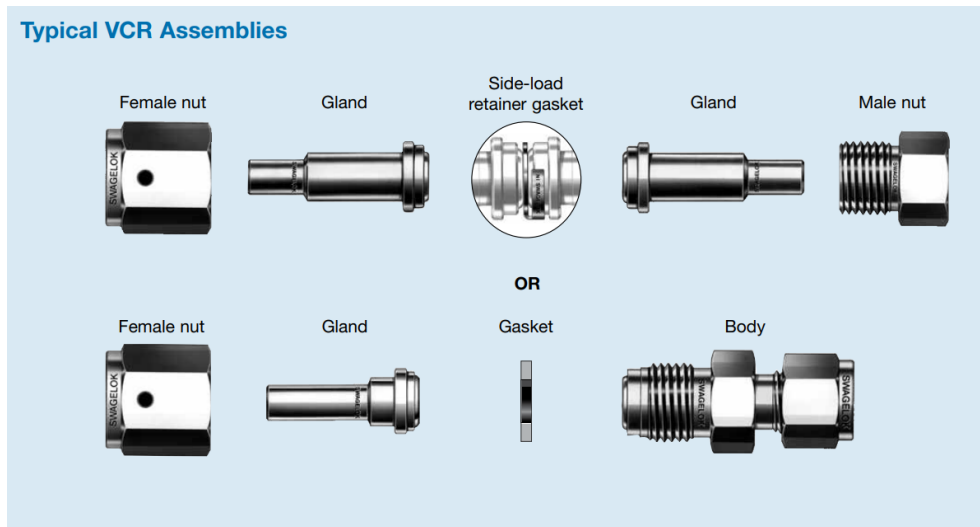
Figura 3.21: Configuración típica de junta VCR. [15]
