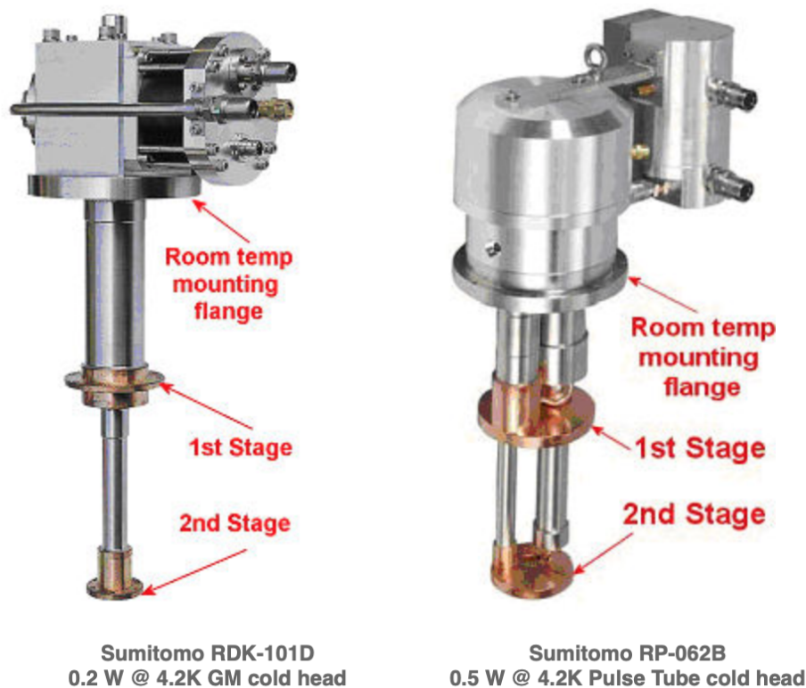
Figura 3.6: Refrigeradores criogénicos (G-M Cycle y Pulse-Tube). [9]
