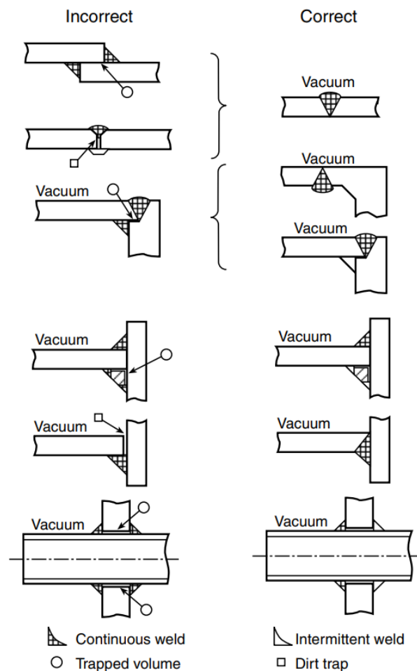
Figura 3.22: Recomendaciones para aplicación de soldadura TIG para aplicaciones de Alto-Vacío. [4]
