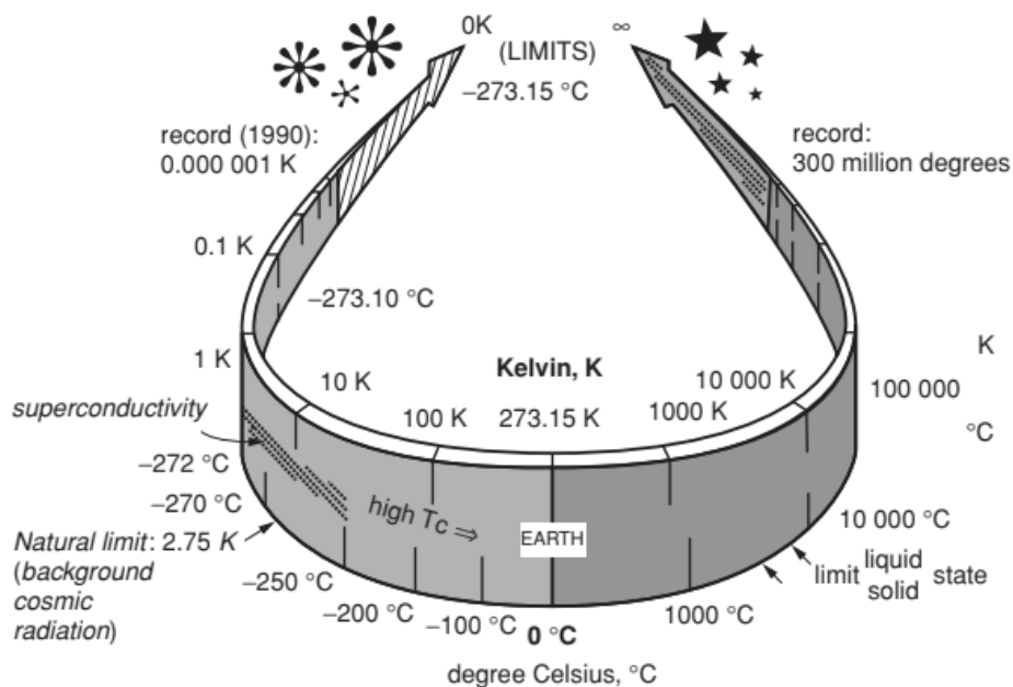
Figura 3.1: Escala logarítmica de temperatura centrada en 0^{\circ}\text{C} . [7]
