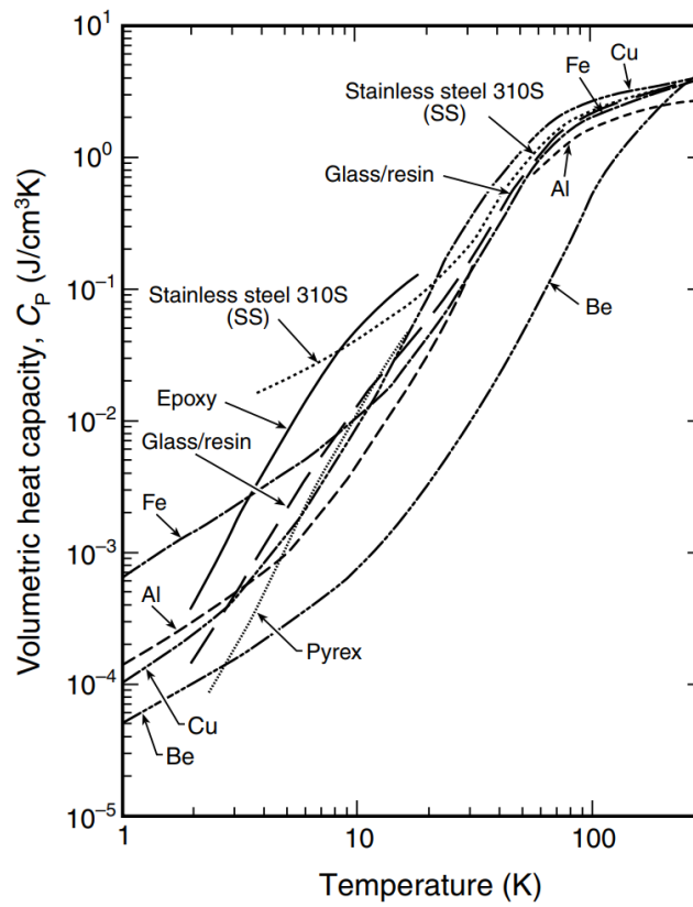
Figura 3.15: Calor específico en base volumétrica de algunos materiales de uso común en criogenia. [4]
