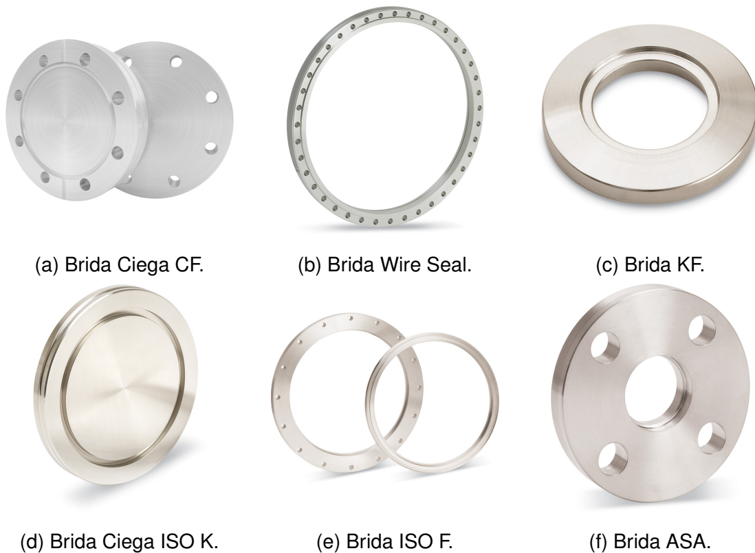
Figura 3.16: Seis tipos de bridas para aplicaciones de alto-vacío. [13]
