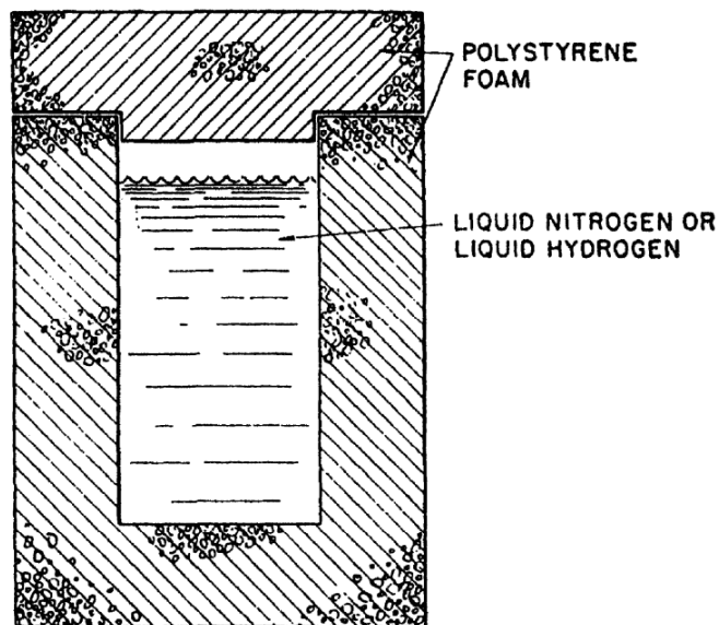
Figura 3.27: Ejemplo de aplicación de espuma de Poliéster. [11]
