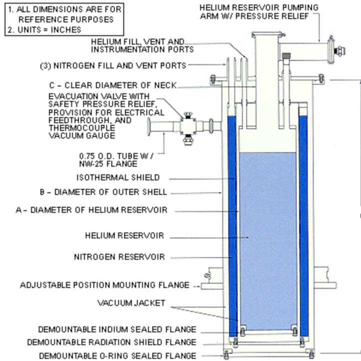
Figura 3.3: Vista en corte de criostato de inmersión. [6]
