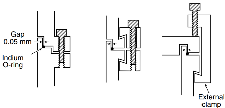
Figura 3.20: Configuración de junta con “Indium O-ring”. [4]
