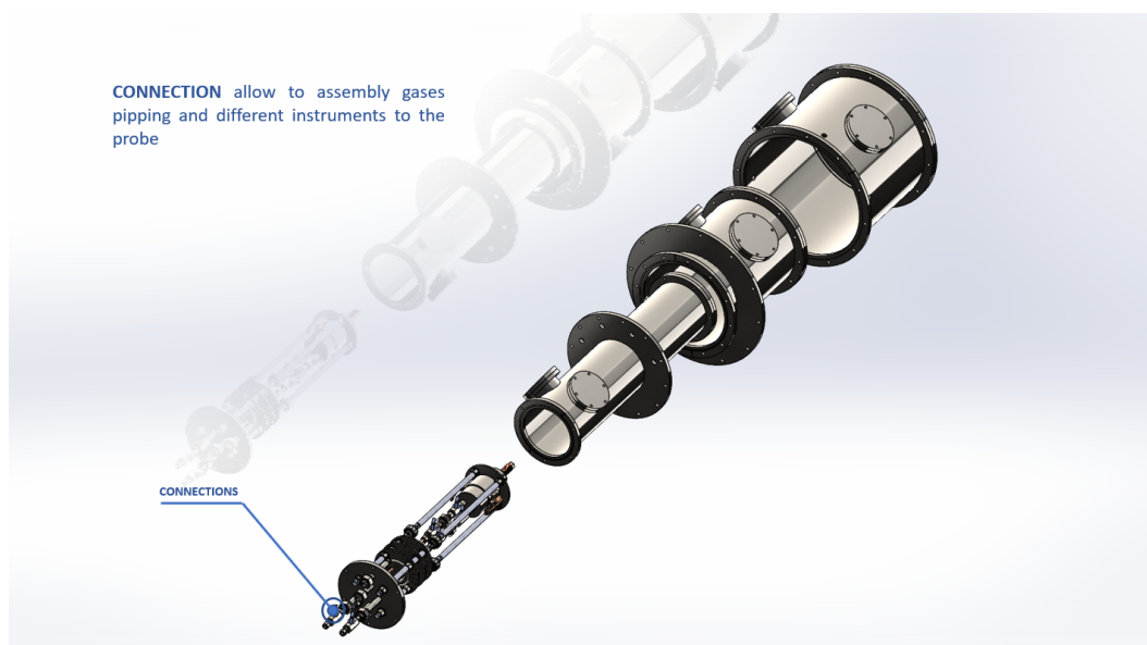
Figura 4.2: Detalle componentes principales Criostato CCTVal. [21]
