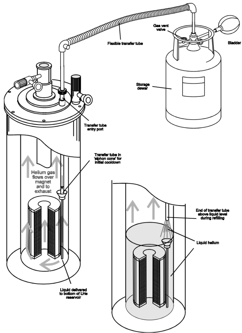
Figura 3.31: Esquema típico para el transporte de LHe en laboratorio. [19]
