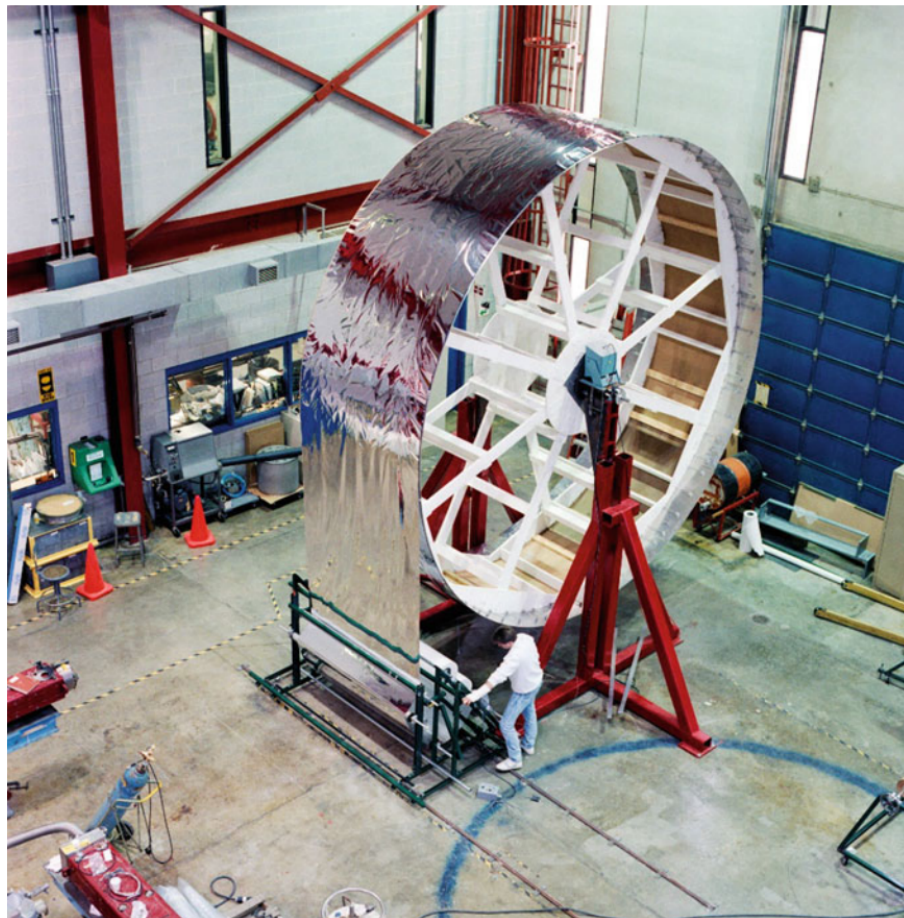
Figura 3.28: Ejemplo de aplicación MLI. [7]
