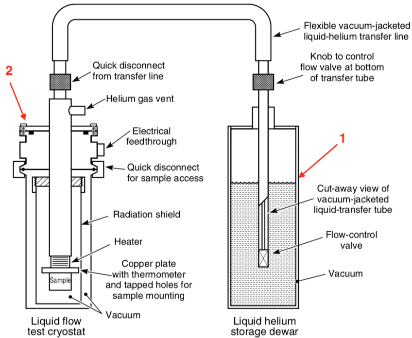
Figura 3.4: Esquema de criostato de flujo en configuración simple. [4]
