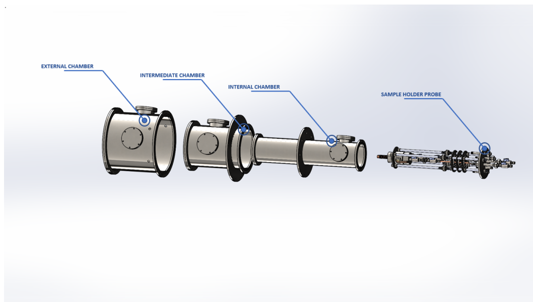
Figura 4.1: Componentes principales de Criostato CCTVal. [21]
