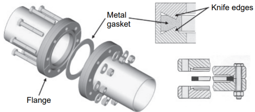
Figura 3.17: Detalle de junta bridada CF. [14]
