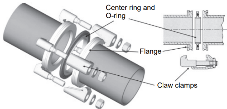
Figura 3.18: Detalle de junta bridada ISO K. [14]
