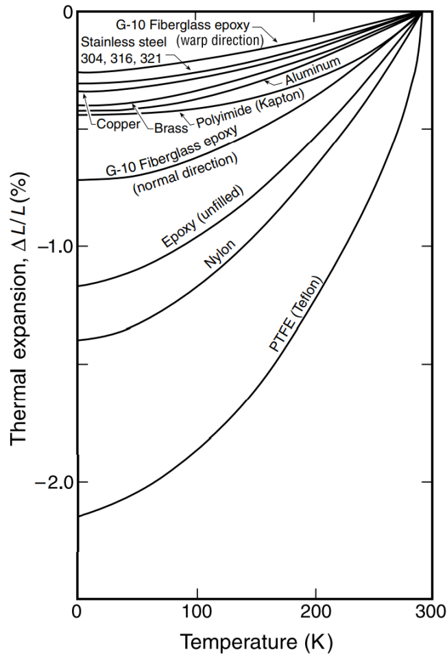
Figura 3.13: Contracción/Dilatación térmica de algunos materiales de uso común en criogenia. [4]
