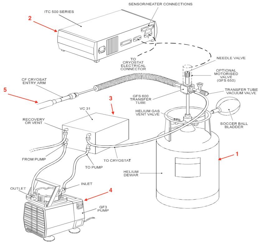
Figura 3.5: Esquema general de sistema de refrigeración de flujo continuo. [4]
