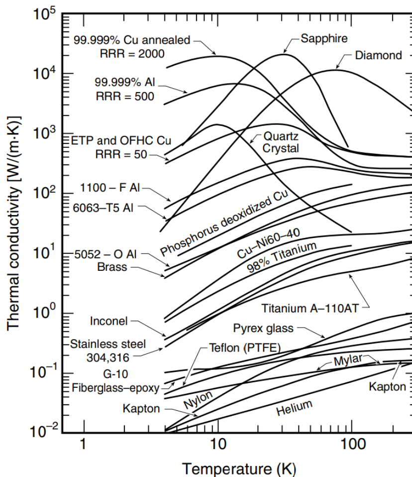
Figura 3.14: Conductividad térmica de algunos materiales de uso común en criogenia. [4]
