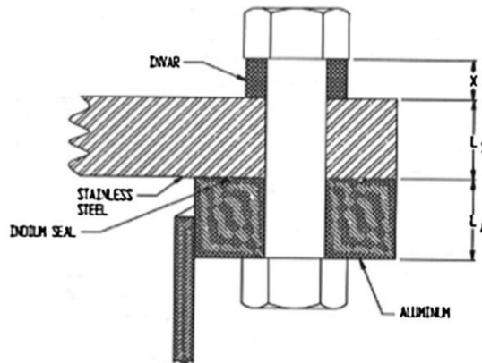
Figura 3.12: Arreglo de junta utilizando una golilla de Invar. [12]
