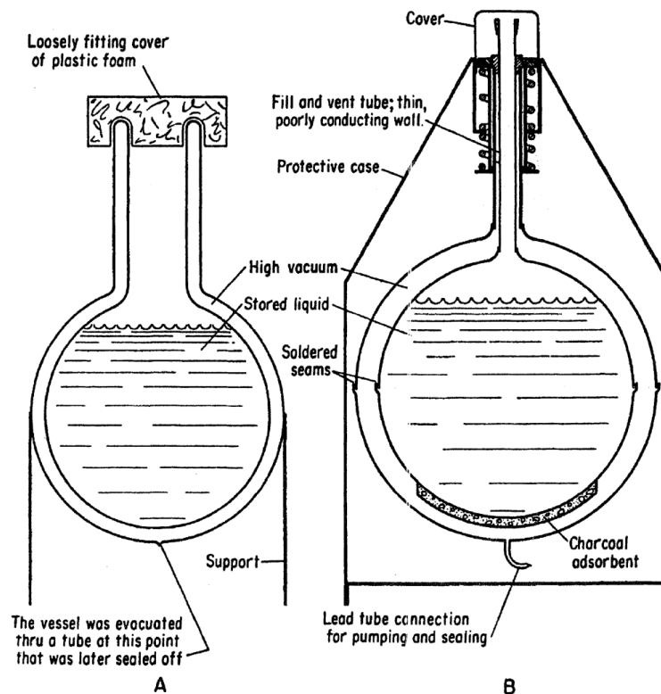
Figura 3.25: Ejemplo de aplicación de técnica de Alto Vacío. [11]
