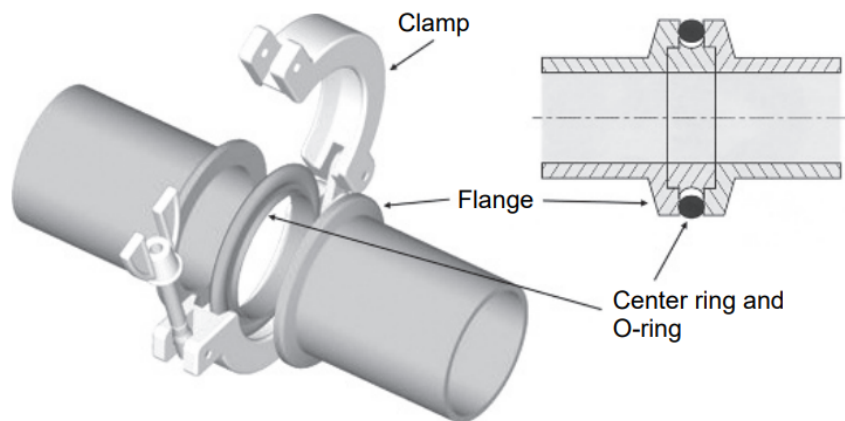
Figura 3.19: Detalle de junta bridada ISO KF. [14]
