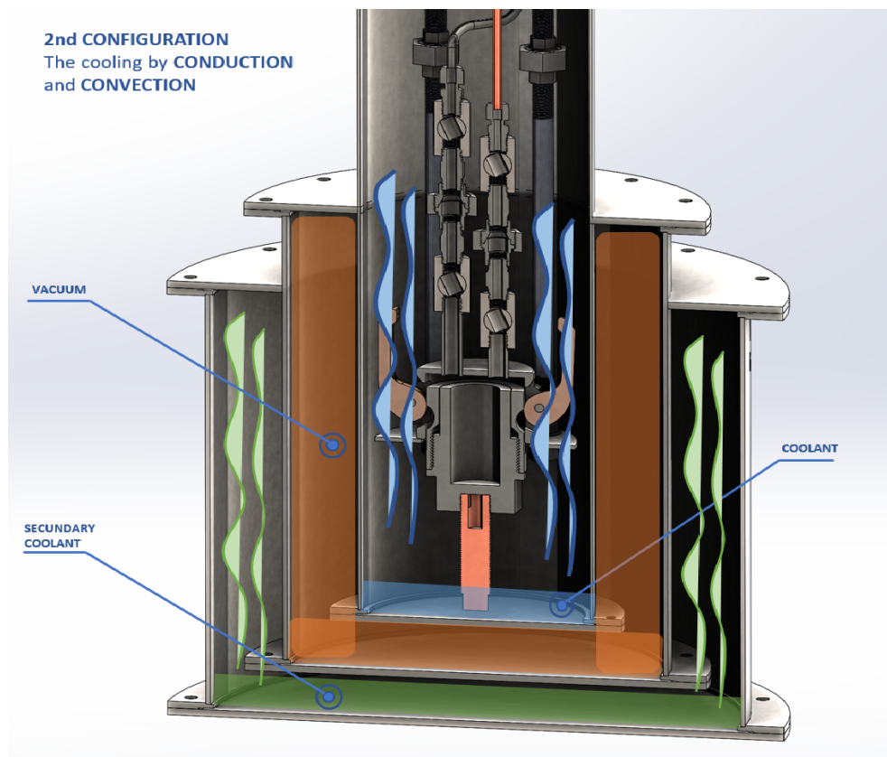
Figura 4.4: Segunda configuración de operación de Criostato. [21]
