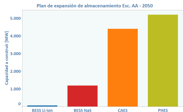
Fig. 4.7: Plan de expansión de almacenamiento por tecnología en Escenario AA año 2050.
