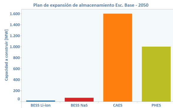
Fig. 4.3: Plan de expansión de almacenamiento por tecnología en Escenario Base año 2050.
