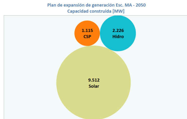
Fig. 4.14: Plan de expansión de generación por tecnología en Escenario MA año 2050.
