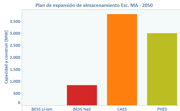
Fig. 4.15: Plan de expansión de almacenamiento por tecnología en Escenario MA año 2050.
