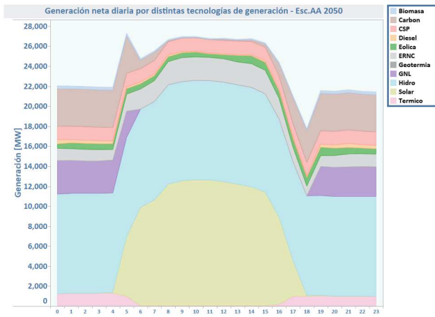
Fig. A.7: Generación horaria por tecnología de generación en Escenario AA - 2050
