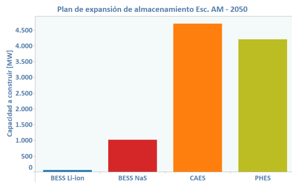
Fig. 4.11: Plan de expansión de almacenamiento por tecnología en Escenario AM año 2050.
