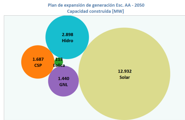
Fig. 4.6: Plan de expansión de generación por tecnología en Escenario AA año 2050.
