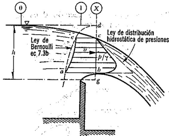
Figura 2.7. Distribución real de presiones y velocidades sobre el vertedero (Sotelo Ávila, 1997).
