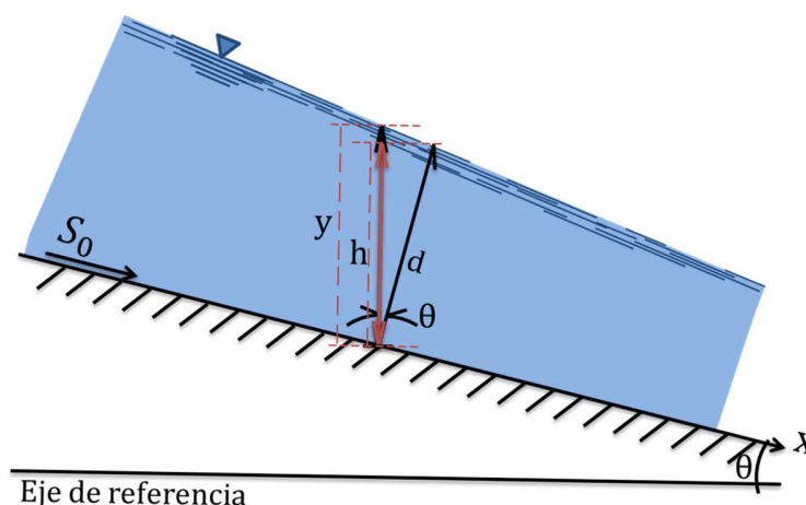
Figura A - 3. Altura de presión para un flujo paralelo al fondo en canales de pendiente alta.
