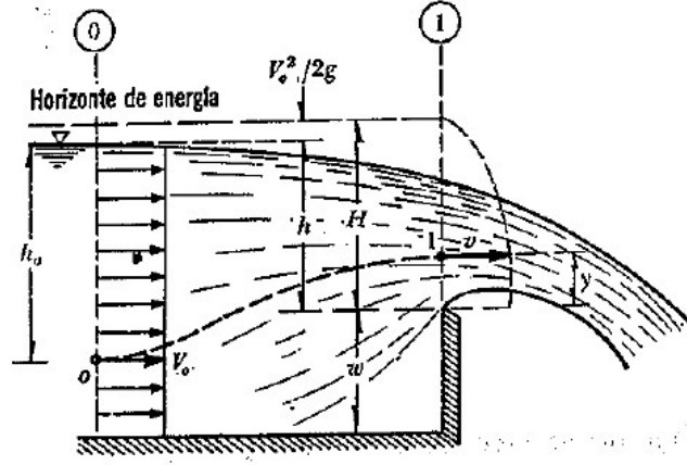
Figura 2.6. Vertedero de pared delgada, obtención de la ecuación general del caudal (Sotelo Ávila, 1997).
