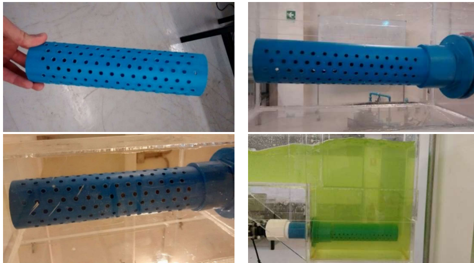
Figura 5.19. Tubería con orificios para aplacar la turbulencia en el estanque de regulación.
