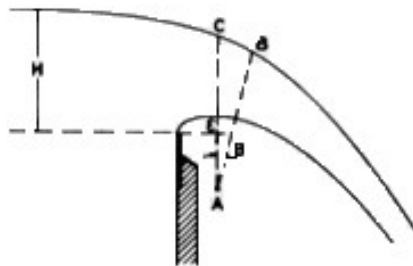
Figura 2.3. Secciones de la napa consideradas para las hipótesis del escurrimiento por un vertedero frontal de napa libre (Dominguez, 1999).
