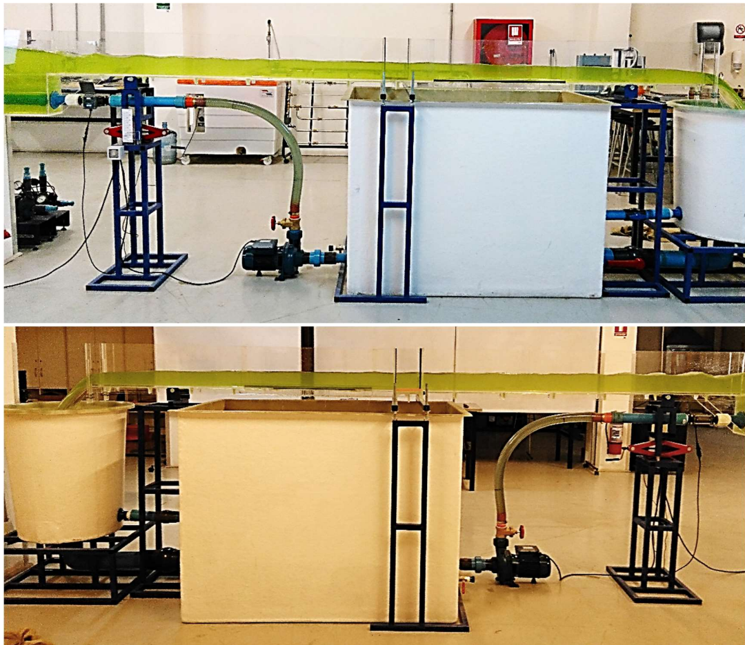
Figura 5.21. Canal terminado y funcionando.
