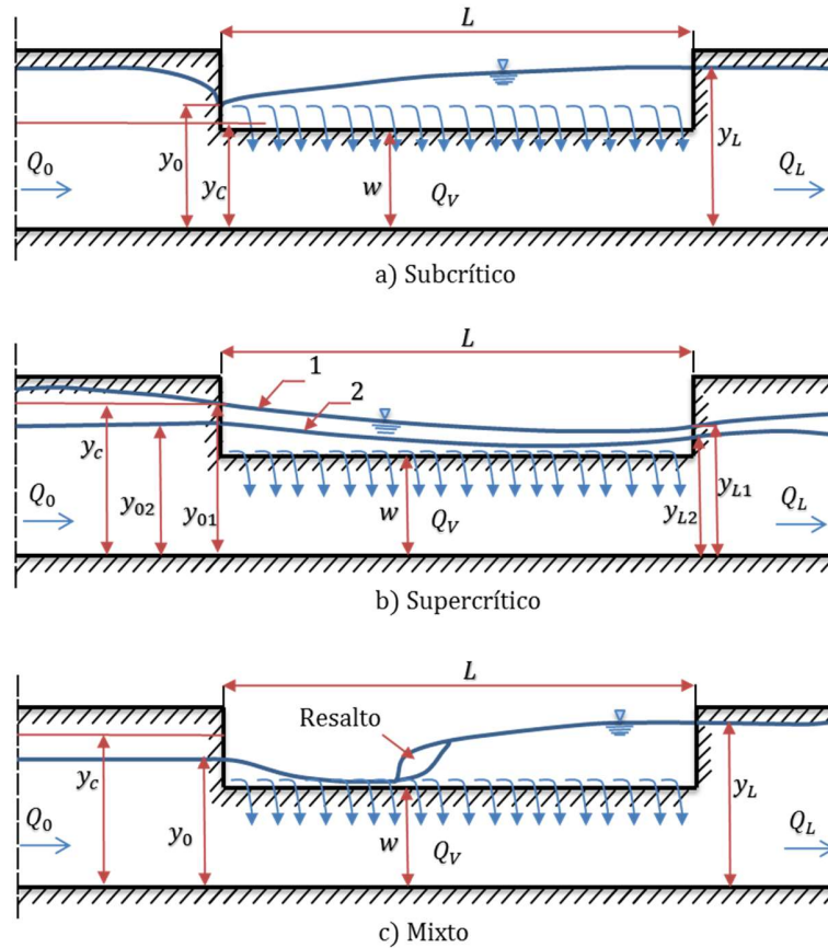
Figura 2.2. Perfiles de flujo en el vertedero lateral de un canal.
