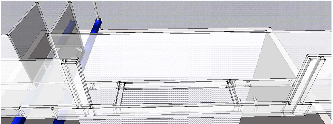
Figura 3.38. Modelo 3D del equipo vista en detalle de la sección del vertedero lateral en el canal.
