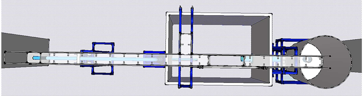
Figura 3.35. Vista superior del Modelo 3D del equipo.
