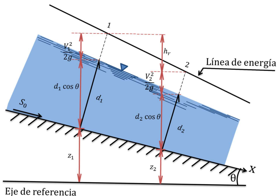
Figura A - 5. Variación de la energía del agua entre dos secciones de un canal abierto
