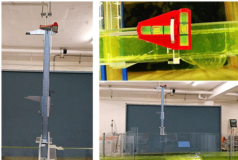
Figura 6.6. Pie de metro instalado en el canal para medir alturas de escurrimiento.
