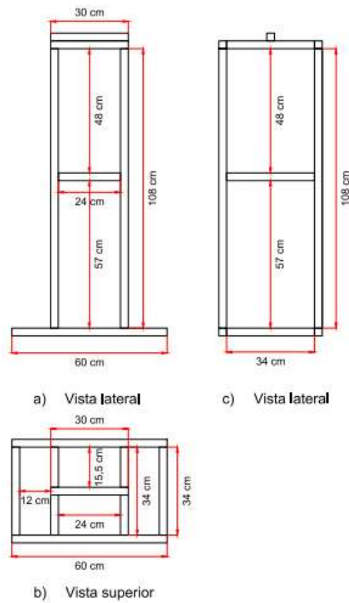
Figura 3.30. Plano de diseño estructura B.
