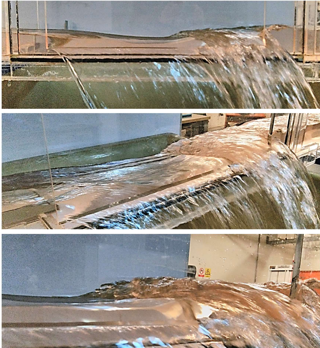
Figura 7.3. Perfil de flujo mixto en el vertedero lateral del canal.
