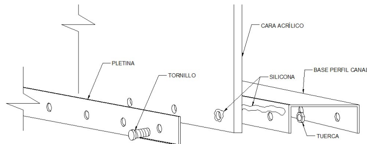
Figura 3.3. Detalle del sistema estructural del canal, para la etapa de prediseño.
