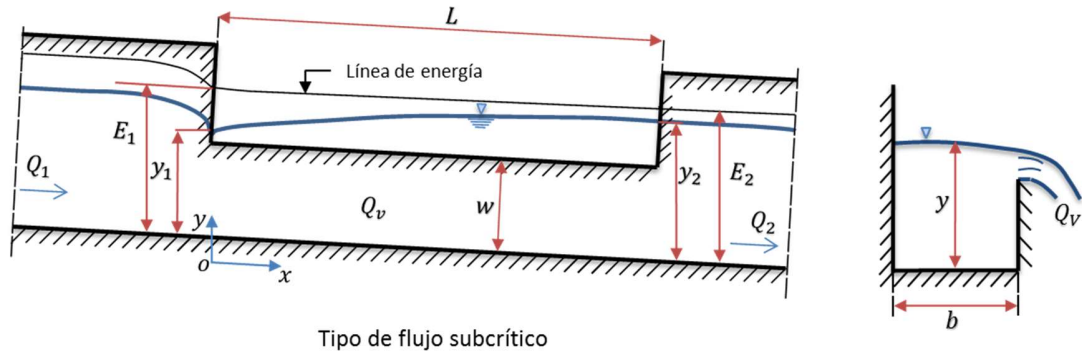
Figura 2.8. Vertedero lateral con flujo subcrítico y energía específica constante en el vertedero.
