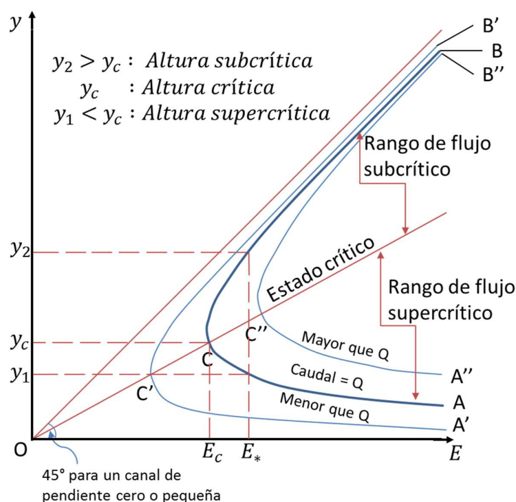
Figura A - 6. Curva de energía específica.
