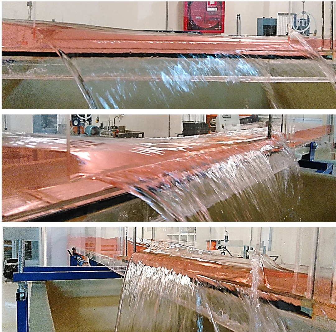
Figura 7.2. Perfil de flujo supercrítico en el vertedero lateral del canal.
