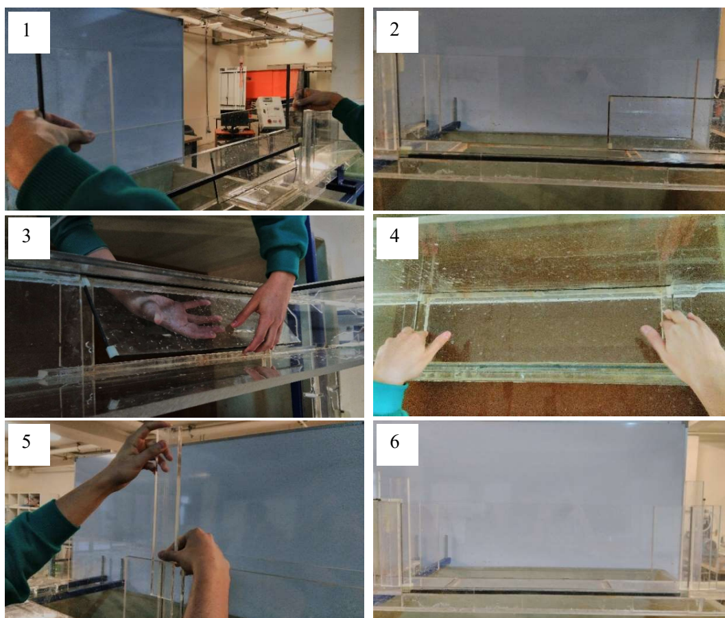
Figura 9.1. Secuencia de pasos para la correcta postura de la pieza de vertedero en el canal
