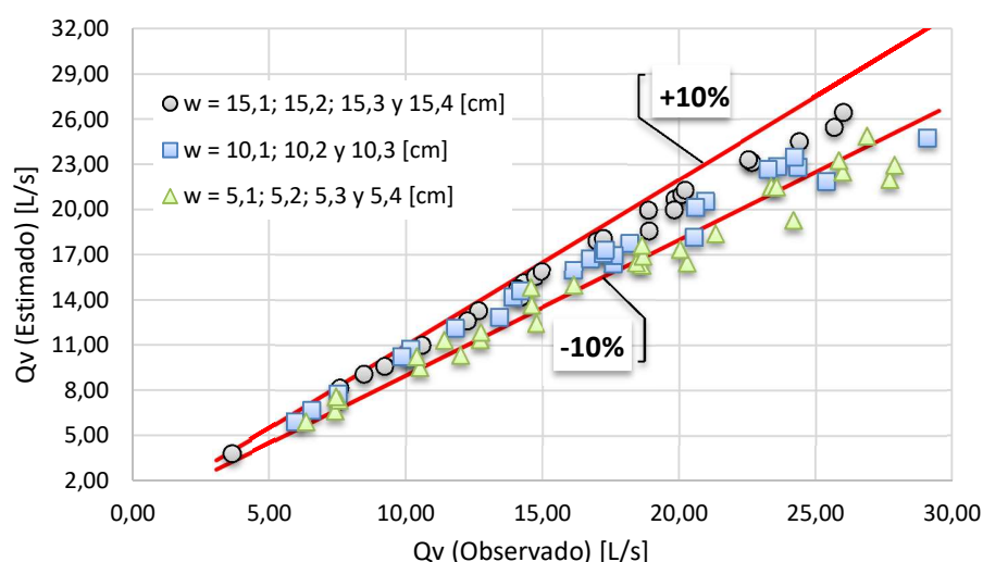
Figura 7.9. Caudales vertidos estimados para el set de datos de validación.
