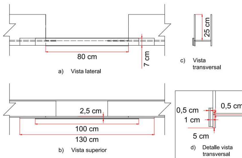
Figura 3.9. Planos de la unión del canal en la zona del vertedero lateral.
