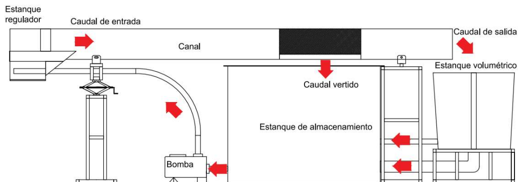
Figura 3.23. Diagrama de recirculación del agua en el equipo.
