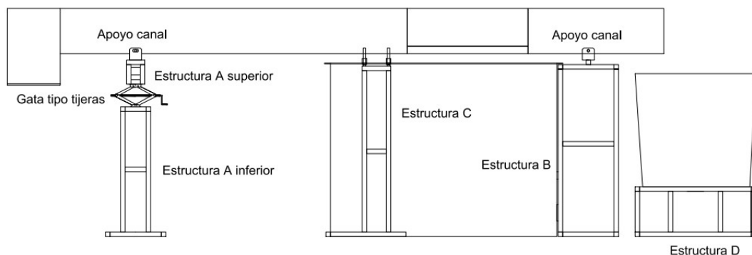
Figura 3.27. Estructuras metálicas del canal.
