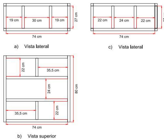
Figura 3.34. Plano de diseño estructura D.
