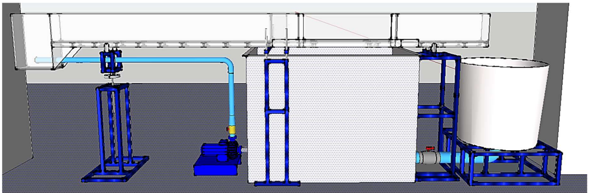
Figura 3.36. Vista lateral del Modelo 3D del equipo, lado donde se ubica el vertedero lateral.
