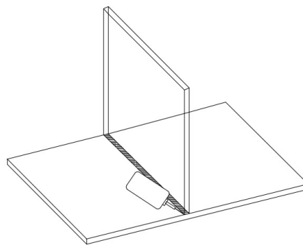
Figura 3.5. Método por capilaridad para pegar acrílico, zona a pegar achurada en la figura.
