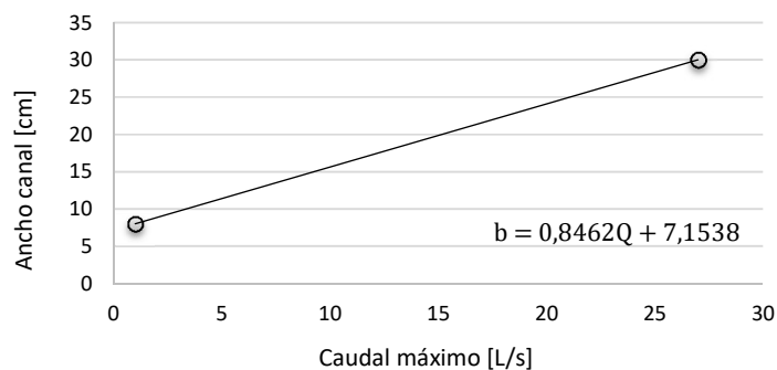
Figura 3.24. Grafico Ancho vs caudal máximo de los canales del Laboratorio.
