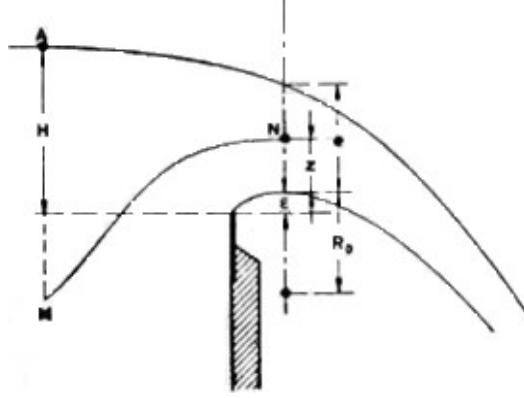
Figura 2.4. Trayectoria a la cual se aplica el teorema de Bernoulli en el flujo sobre el vertedero lateral (Dominguez, 1999).
