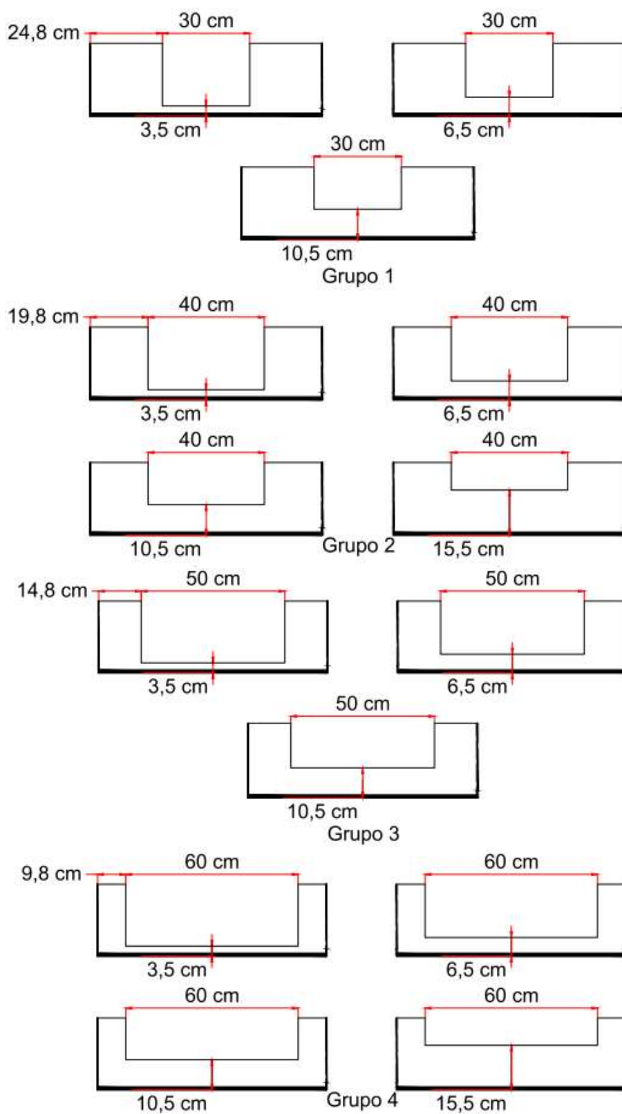
Figura 3.13. Plano de diseño del largo y la altura de vertedero para cada pieza.
