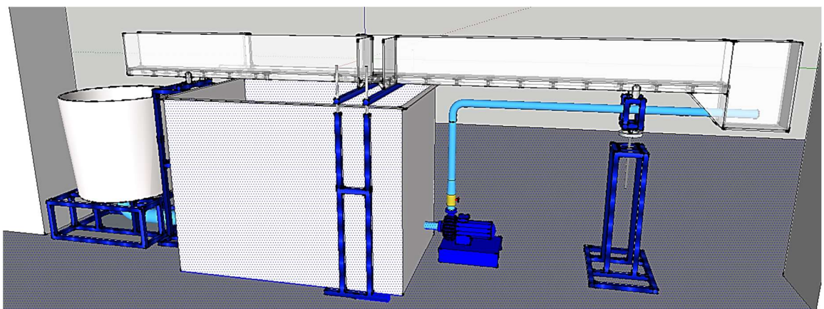
Figura 3.37. Vista lateral del Modelo 3D del equipo, lado donde se ubica la compuerta lateral.
