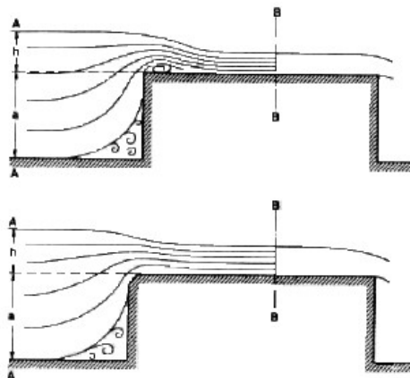
Figura 2.10. Pérdida de energía de entrada en un vertedero de pared gruesa con arista viva (Dominguez, 1999).
