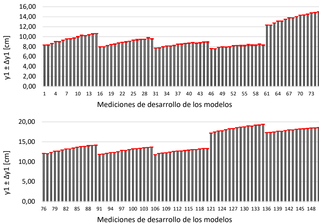
Figura 6.7. Barras de error de las mediciones de altura de escurrimiento aguas arriba del vertedero.
