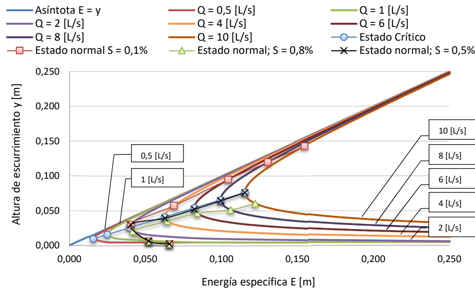
Figura 3.26. Familia de curvas de energía específica del canal.
