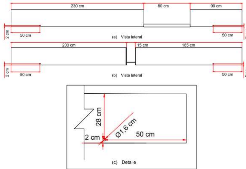
Figura 3.8. Plano de perforaciones en el canal para su unión con la estructura de soporte.
