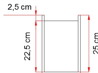
Figura 3.25. Plano de diseño del borde libre del canal.
