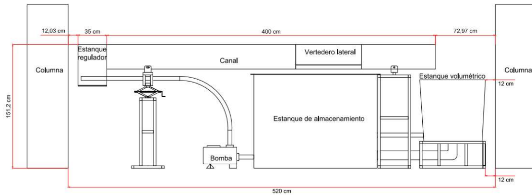
Figura 3.4. Plano de ubicación de la infraestructura del canal en el Laboratorio.
