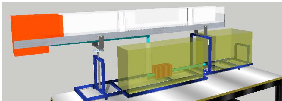
Figura 3.2. Modelo 3D en SketchUp Make para el prediseño del canal con vertedero lateral.
