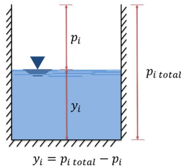
Figura 8.2. Esquema para medir alturas de escurrimiento en el vertedero.
