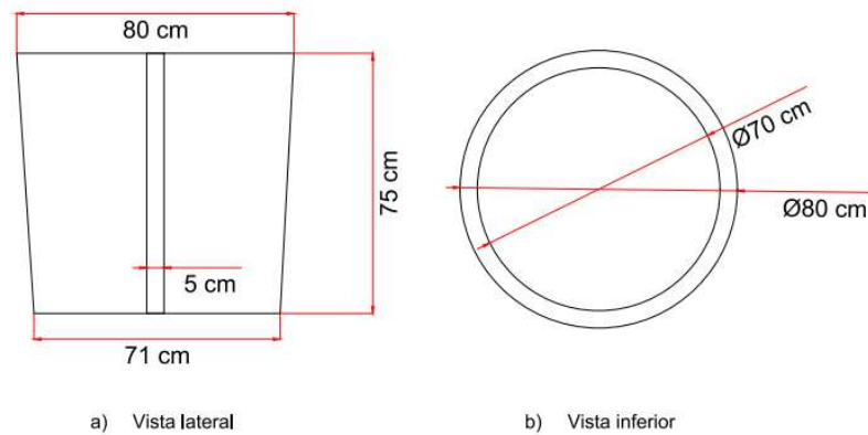
Figura 3.22. Plano estanque volumétrico.
