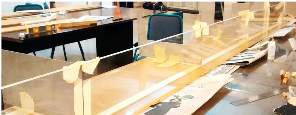
Figura 5.3. Pegado de secciones del canal principal.
