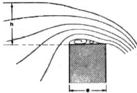
Figura 2.11. Vertedero de pared intermedia, sin influenciar desde aguas abajo de la pared (Dominguez, 1999).
