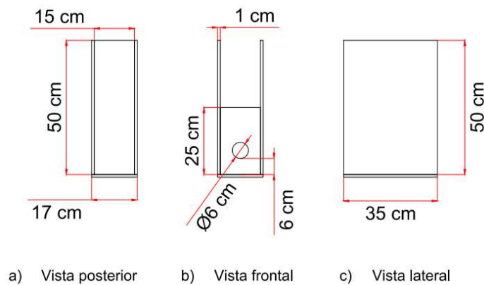
Figura 3.20. Plano de diseño estanque de regulación.
