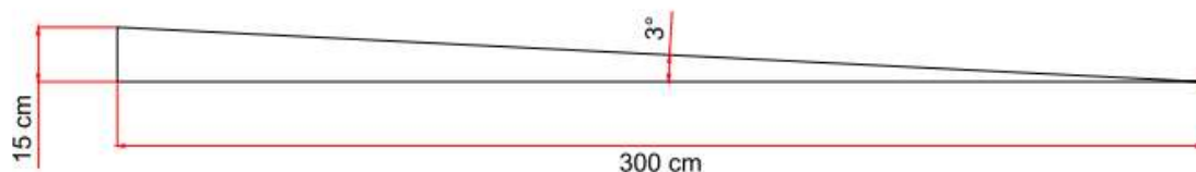
Figura 3.18. Esquema de la máxima pendiente permitida por diseño en el canal.
