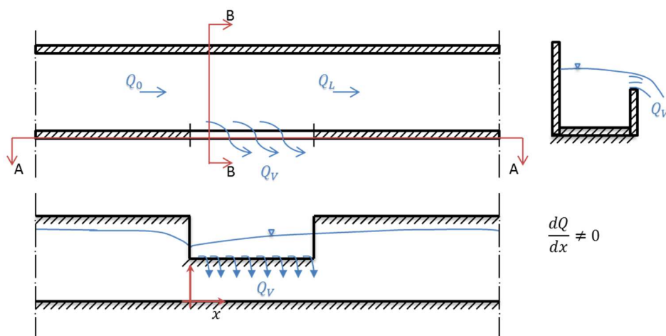
Figura 2.1. Canal con caudal decreciente debido a un vertedero lateral.
