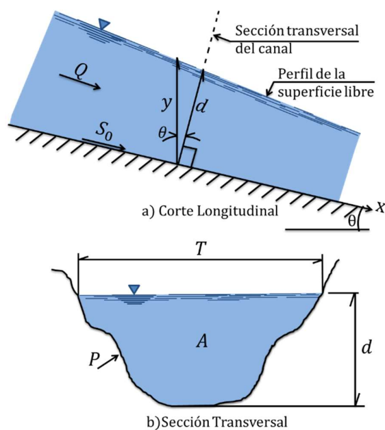
Figura A - 1. Elementos geométricos de un canal.
