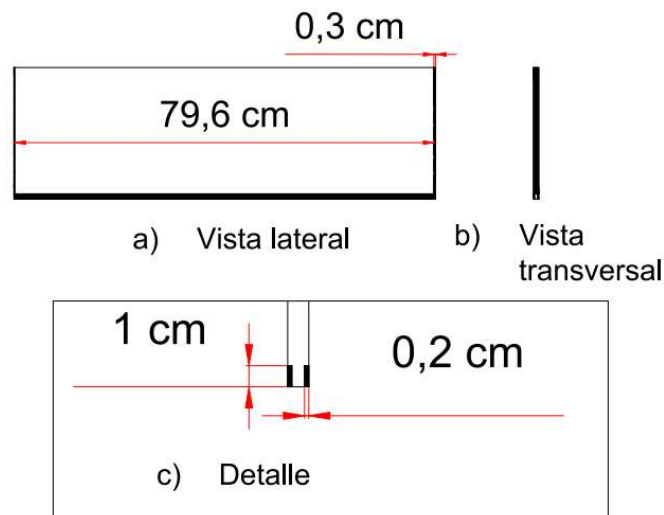
Figura 3.11. Plano de diseño contra filtraciones en la unión entre el canal y la pieza de vertedero lateral.
