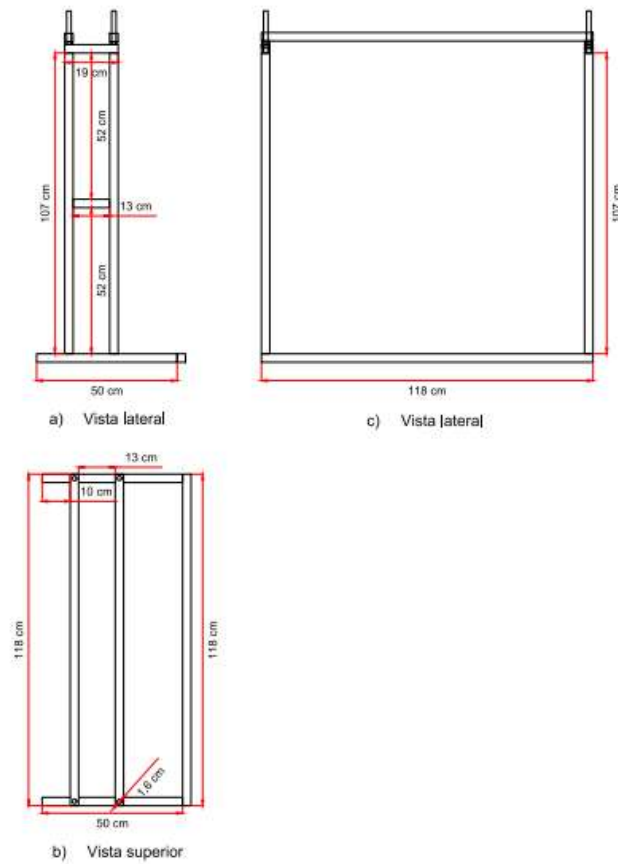
Figura 3.33. Planos de diseño estructura C.
