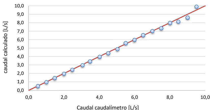
Figura 6.3. Gráfico de verificación del método de cálculo del caudal de salida del canal.
