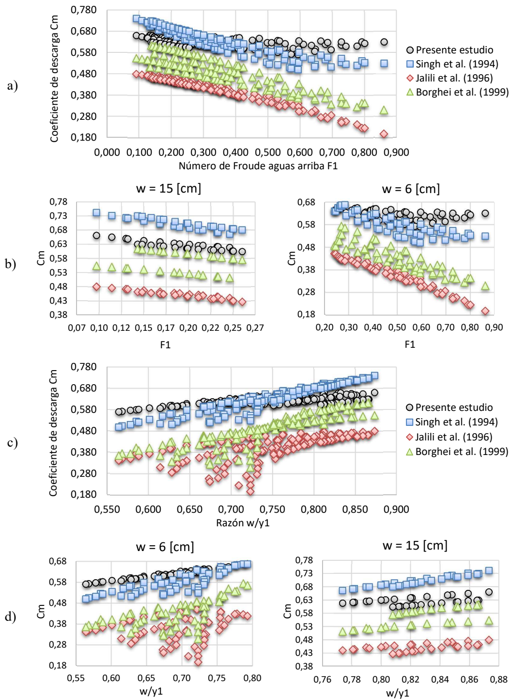
Figura 7.10. a) Coeficiente de descarga versus número de Froude aguas arriba del vertedero lateral, b) Detalle del comportamiento de F_1 en vertederos con w = 6 y 15 [cm], c) Coeficiente de descarga versus razón w/y_1 , d) Detalle del comportamiento de w/y_1 en vertederos con w = 6 y 15 [cm]
