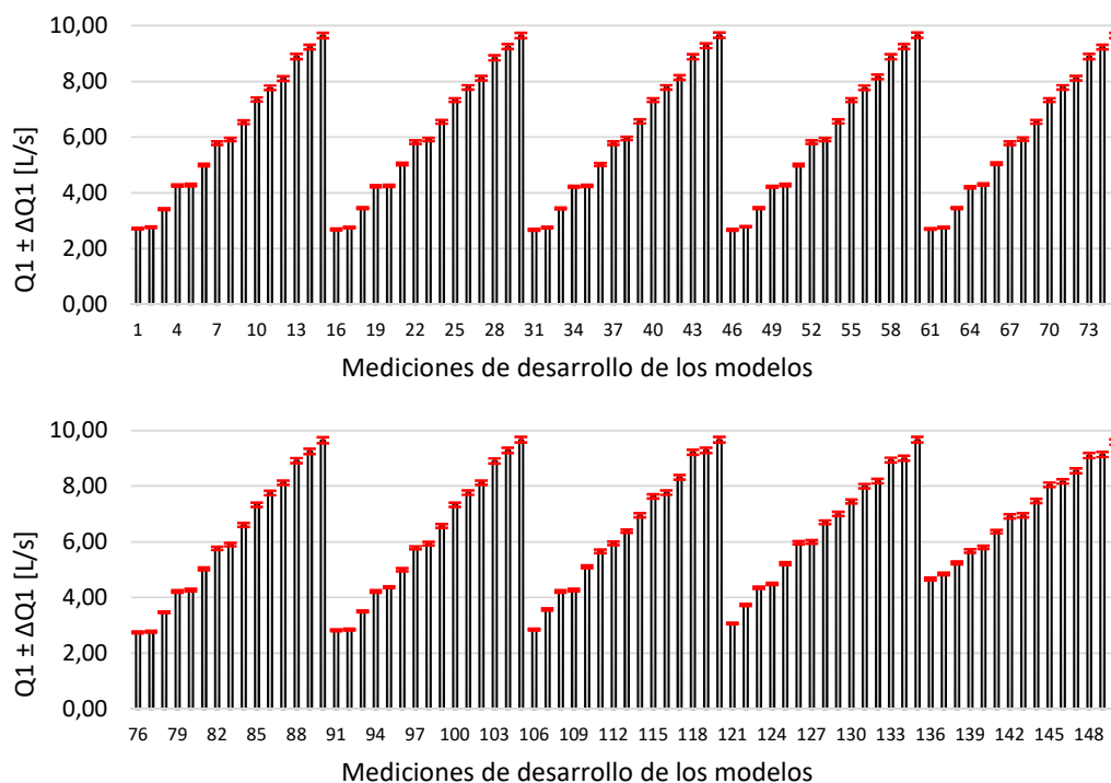
Figura 6.9. Barras de error de las mediciones de caudal aguas arriba del vertedero.
