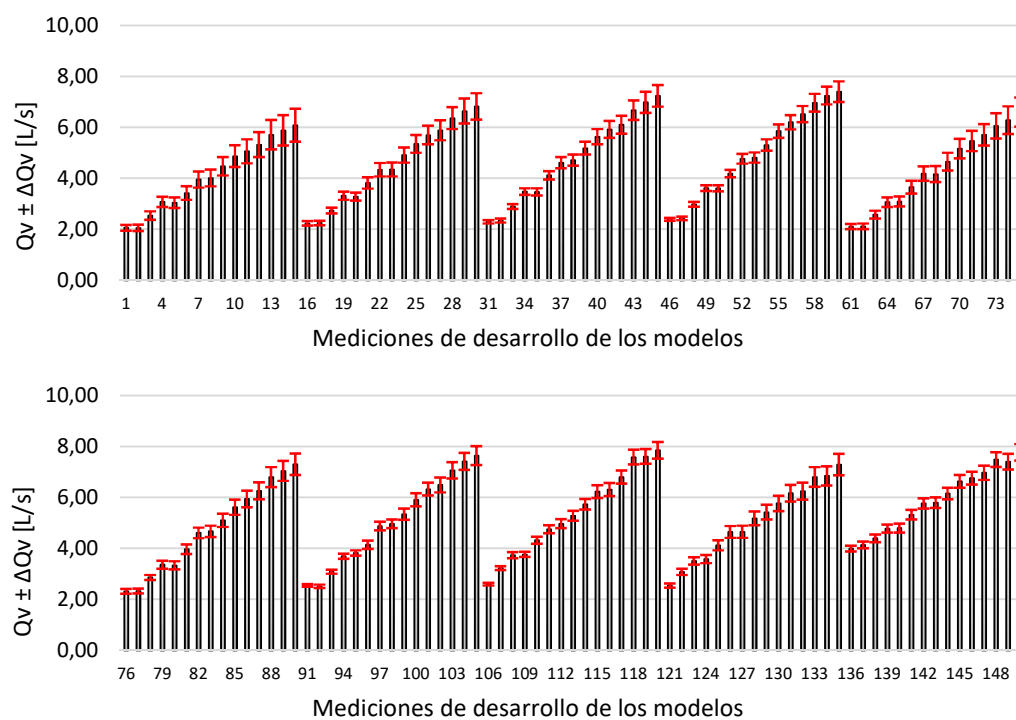
Figura 6.11. Barras de error de las mediciones de caudal vertido por el vertedero.
