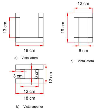
Figura 3.28. Plano de diseño estructura A parte superior.
