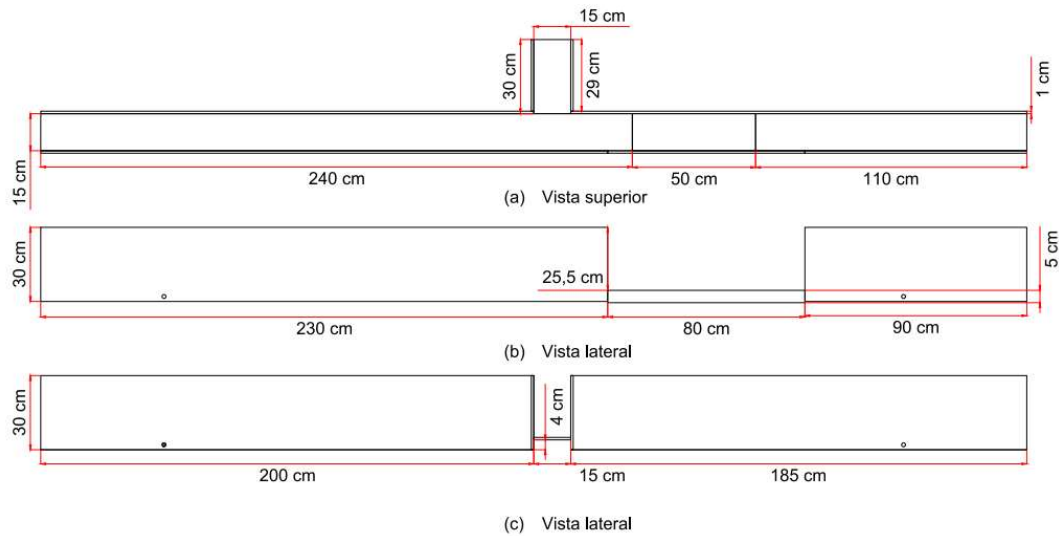
Figura 3.6. Planos de diseño del canal de acrílico con sus cotas principales.
