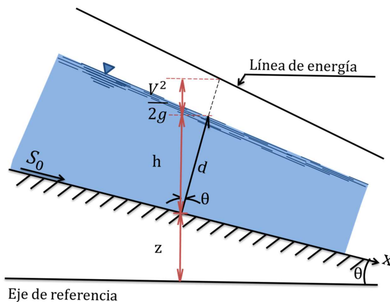
Figura A - 4. Energía total del agua por unidad de peso en una sección del canal.
