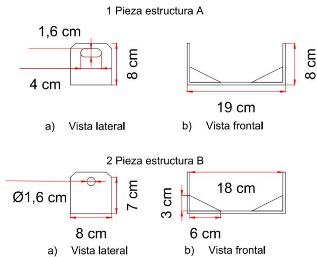
Figura 3.31. Planos de diseño de las piezas de apoyo entre el canal y las estructuras metálicas de soporte.
