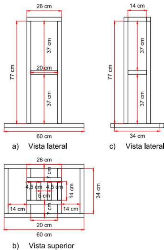
Figura 3.29. Plano de diseño estructura A parte inferior.
