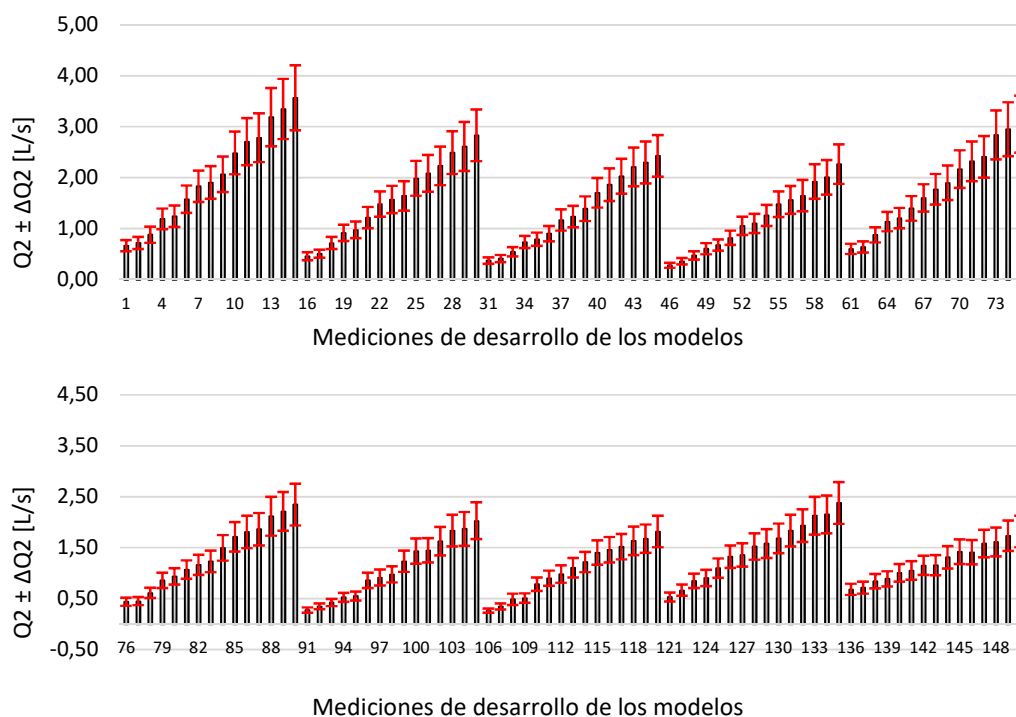
Figura 6.10. Barras de error de las mediciones de caudal aguas abajo del vertedero.
