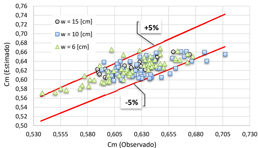
Figura 7.7. Coeficientes de descarga de De Marchi estimados versus observados.
