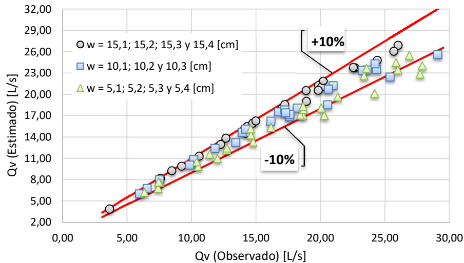
Figura 7.14. Caudales vertidos estimados para el set de datos de validación.
