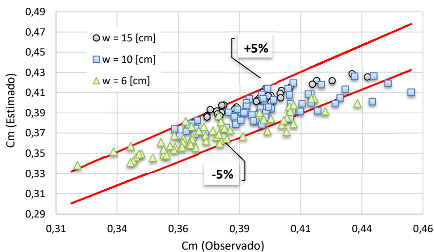
Figura 7.12. Coeficientes de descarga de Domínguez estimados versus observados.
