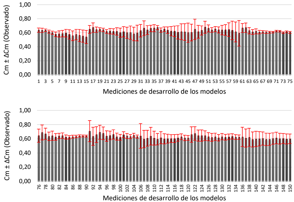
Figura 7.6. Gráfico de barras de error del coeficiente de descarga de De Marchi calculado.
