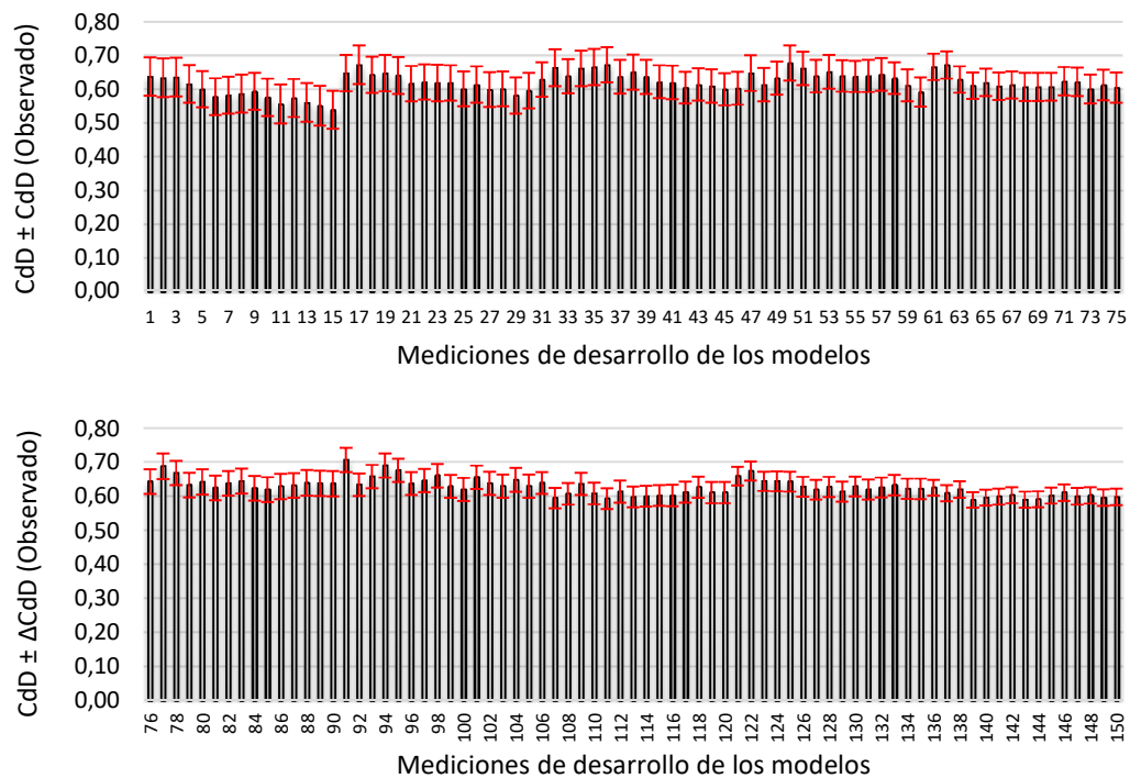
Figura 7.11. Gráfico de barras de error del coeficiente de descarga de Domínguez calculado.
