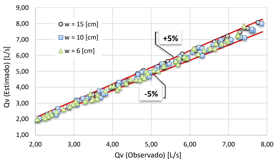
Figura 7.13. Caudales vertidos estimados mediante el método de Domínguez versus caudales vertidos observados.
