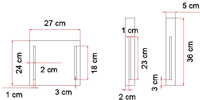
Figura 3.12. Plano de diseño del vertedero frontal del canal.
