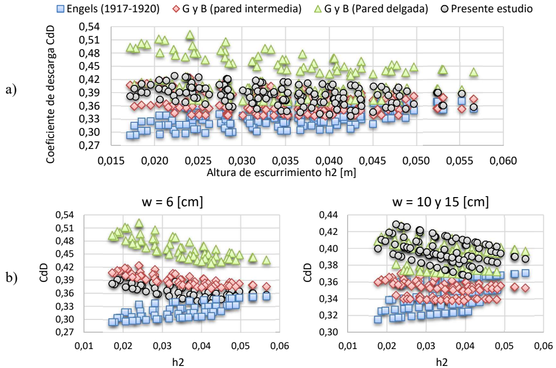
Figura 7.15. a) Coeficientes de descarga versus altura de escurrimiento final sobre el vertedero h_2 , b) Detalle del comportamiento de C_{dD} respecto a h_2 diferenciando por altura del vertedero.
