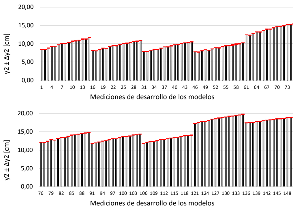
Figura 6.8. Barras de error de las mediciones de altura de escurrimiento aguas abajo del vertedero.
