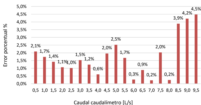
Figura 6.4. Error porcentual obtenido para cada valor calculado del caudal de salida mediante el estanque volumétrico.
