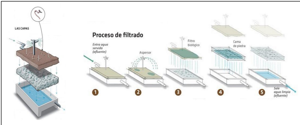
Figura 1 Gráfico de operación del Lombrifiltro. Fuente Fleming, Z. 2014
