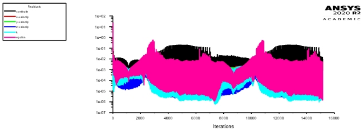
Figura 58: Gráfico residual algoritmo PISO con 1200 pasos de tiempo y discretización temporal de segundo orden
