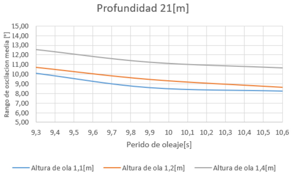
Figura 93: Curvas de amplitud de movimiento angular para una ubicación con 21[m] de profundidad
