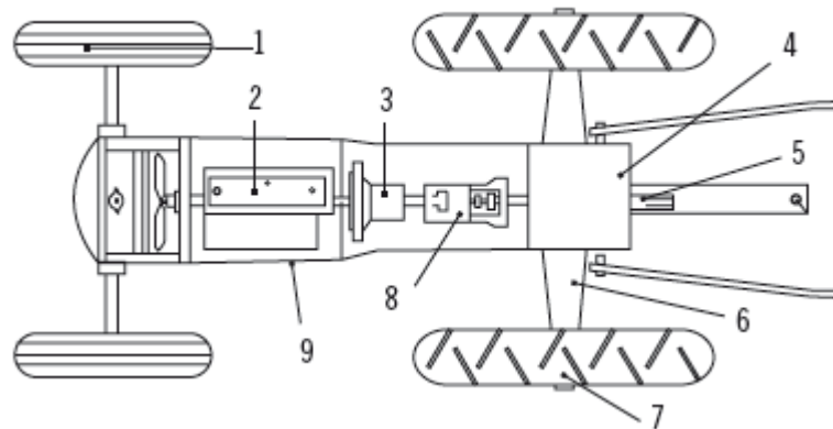
Figura 3-2. Partes del tractor.
