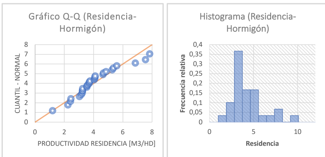
Gráfico 31: Q-Q Plot e Histograma. Obra "Residencia – San Pedro de Atacama". Actividad Hormigonado. Referencia: Elaboración propia.
