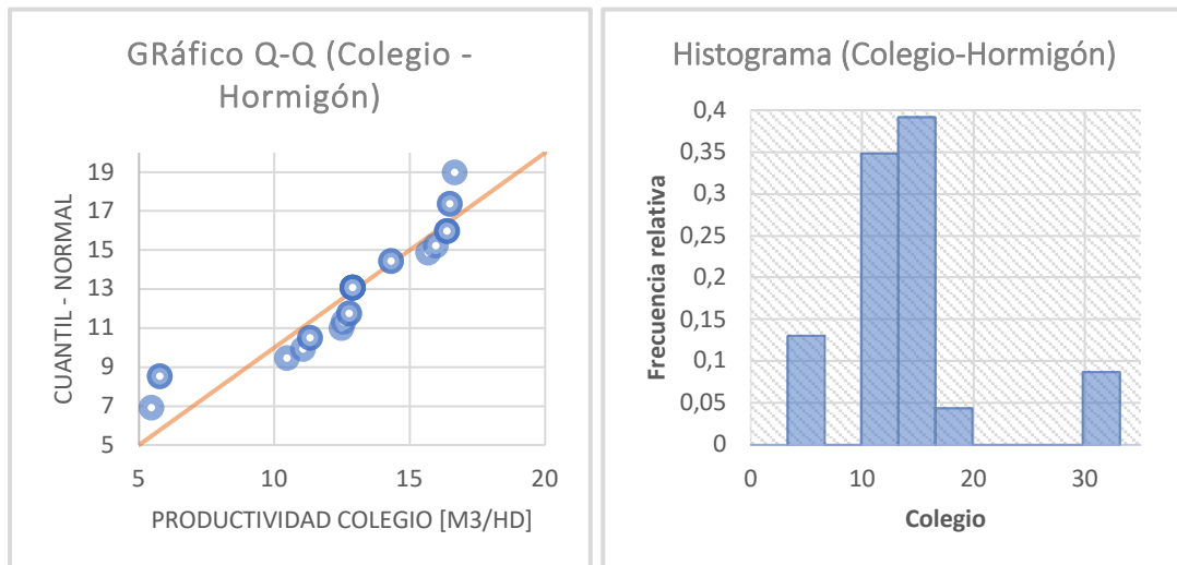
Gráfico 33: Q-Q Plot e Histograma. Obra “Colegio – Santiago”. Actividad Hormigonado. Referencia: Elaboración propia.
