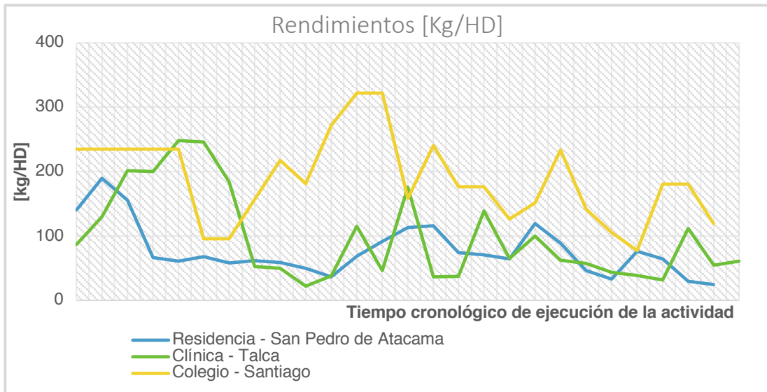
Gráfico 10: Rendimientos Obras, Actividad Enfierradura. Referencia: Elaboración propia.
