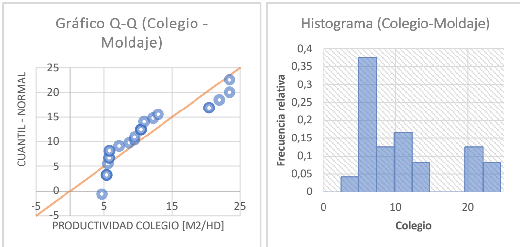
Gráfico 30: Q-Q Plot e Histograma. Obra "Colegio – Santiago". Actividad Moldaje. Referencia: Elaboración propia.
