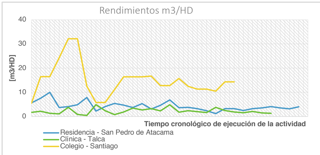
Gráfico 14: Rendimiento Obras, Actividad Hormigón. Referencia: Elaboración propia.
