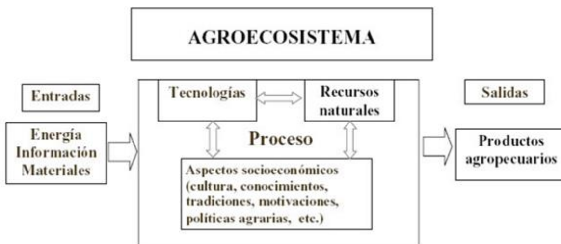
Figura 4: Agroecosistema.
