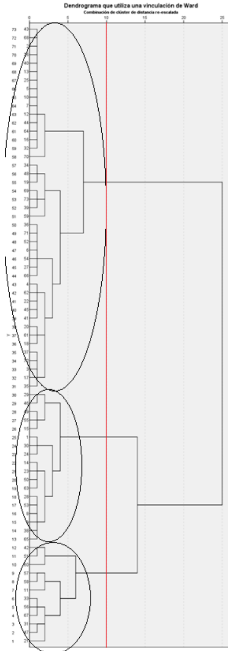
Figura 39: Dendrograma.
