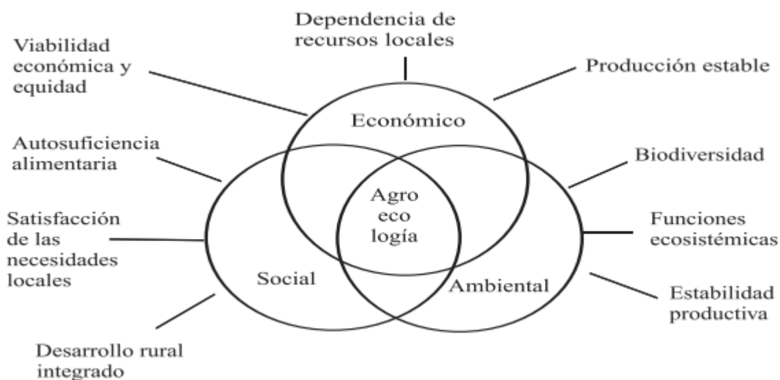
Figura 7: Estrategia agroecológica.
