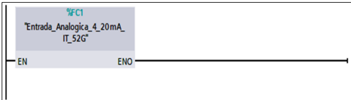
Figura 2-12. Segmento N°1, entrada analógica de Interruptores 52G.
