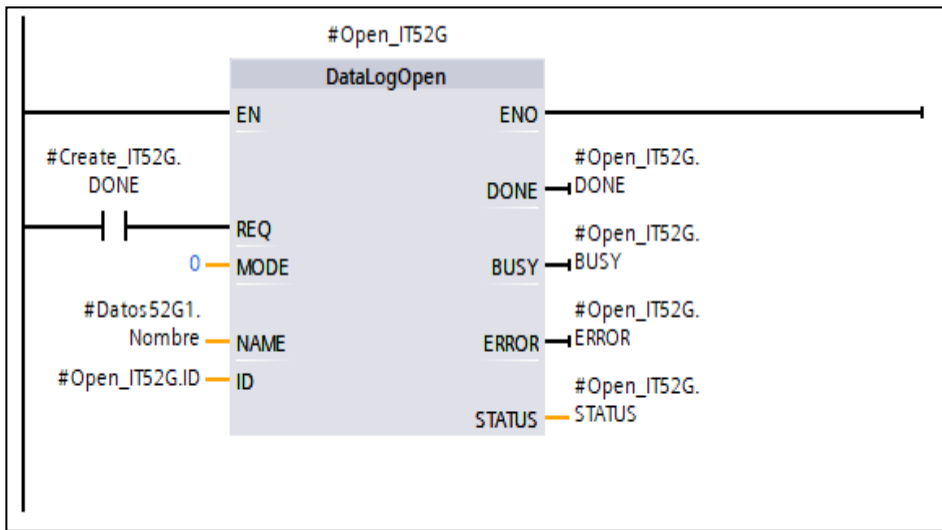
Figura 2-19. Ejemplo de instrucción DataLogOpen en IT52G.
