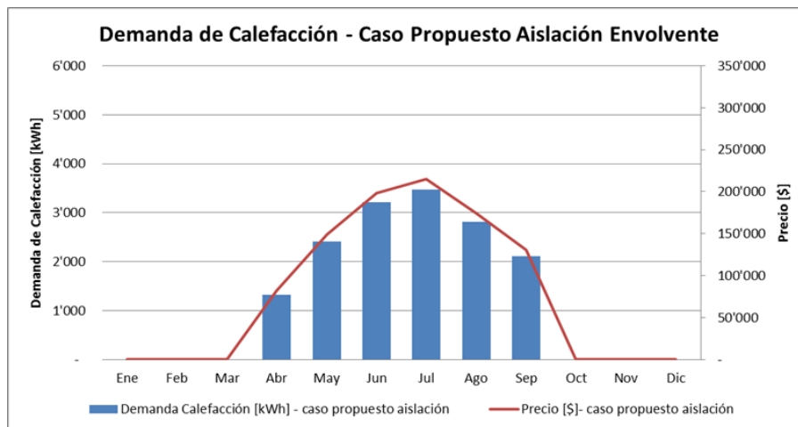
Figura 4-2 Demanda de calefacción para la casa con aislación térmica, y el costo asociado a calefaccionar con una estufa a parafina.
