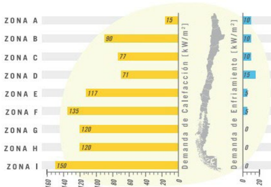
Figura 2.1 Demanda Según Zona Térmica
