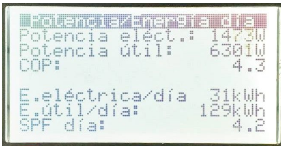
Figura 4.7. Con envolvente y parámetros térmicos de la instalación
