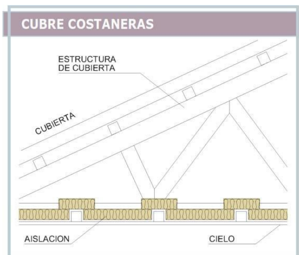
Figura 3.8 Instalación de la aislación de la techumbre.
