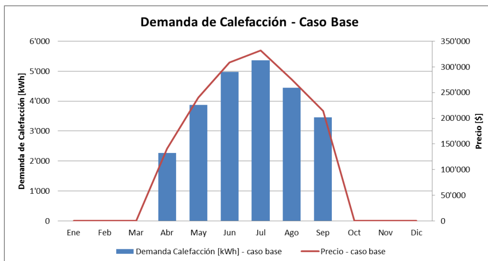
Figura 4.1 Demanda de calefacción para el caso base y el costo asociado a calefacción con estufa a parafina.
