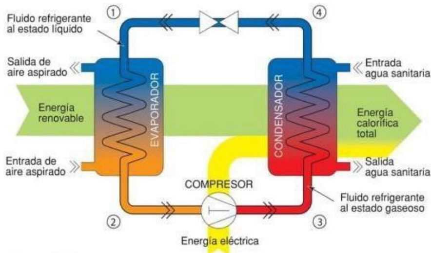
Figura 3-8 Ciclo de operación de una bomba de calor.
