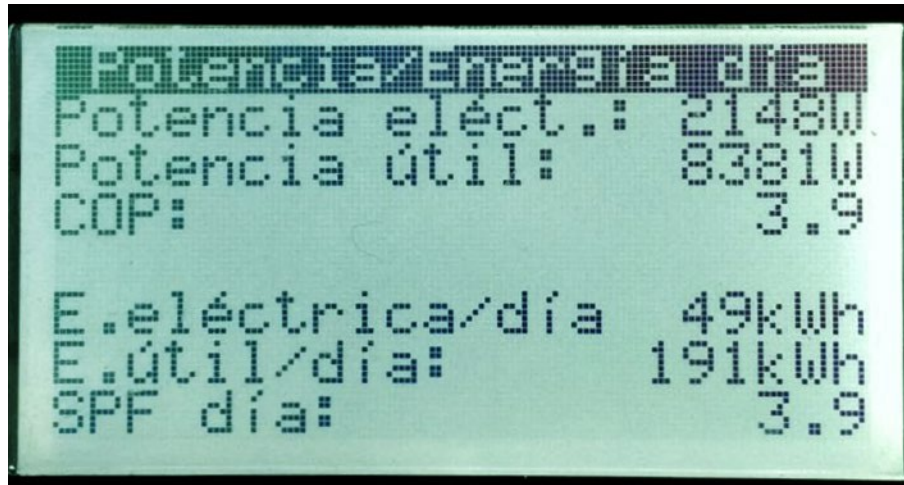
Figura 4.8. Sin envolvente y parámetros térmicos de la instalación
