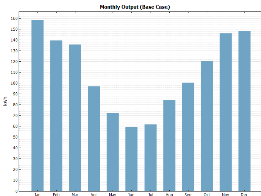
Gráfico 3.1 Generación mensual de energía durante un año para 900 W de potencia instalada en paneles fotovoltaicos
