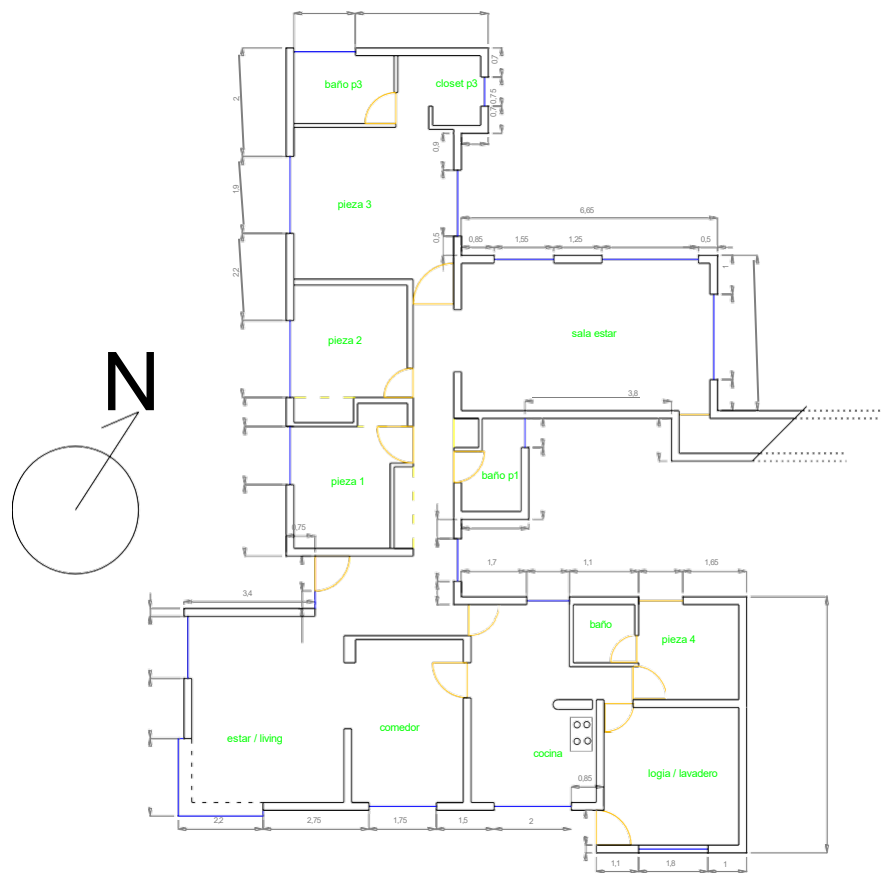
Figura 1.1 Plano de vivienda de la casa habitación
