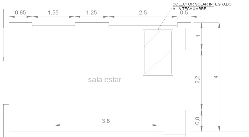
Figura 3-3 Colector Solar integrado a la techumbre
