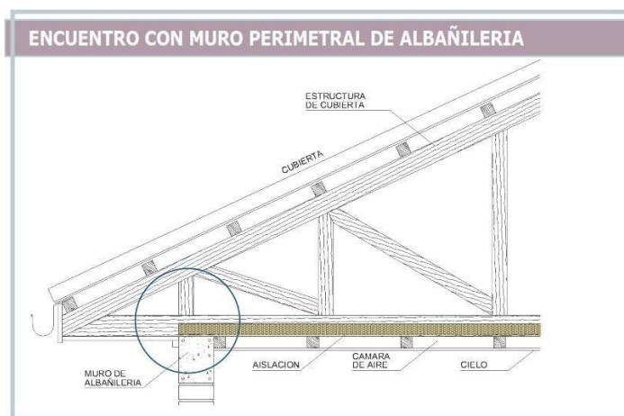
Figura 3-9 Aislación en el encuentro de la techumbre con los muros perimetrales
