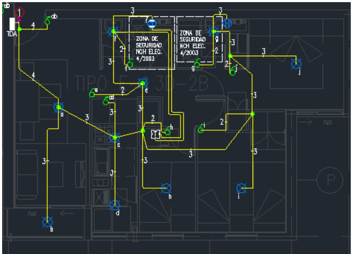
Figura 2-17. "Plano tipo D Alumbrado"
