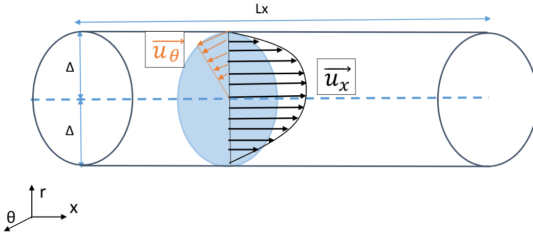
Figura 3.2: Esquema del flujo a través de una tubería en coordenadas cilíndricas.
