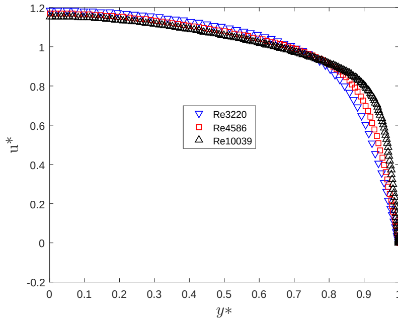
Figura 4.1: Velocidad Axial Canal DNS [12].
