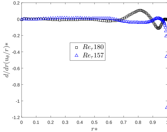
Figura 4.14: Derivada de la velocidad tangencial relativa al radio \frac{\partial}{\partial r} \frac{\bar{u}_\theta}{r} tubería DNS [5].
