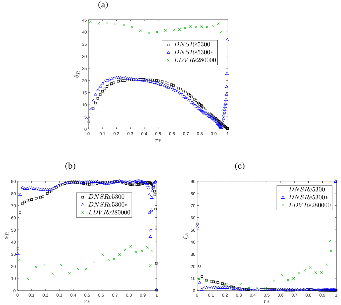
Figura 4.17: Ángulos entre D_R - X\theta r tubería DNS [5].
