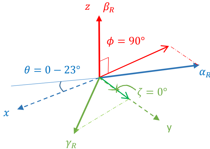
Figura 4.6: Representación direcciones principales de R y ángulos con respecto XZY a para el canal DNS [12].
