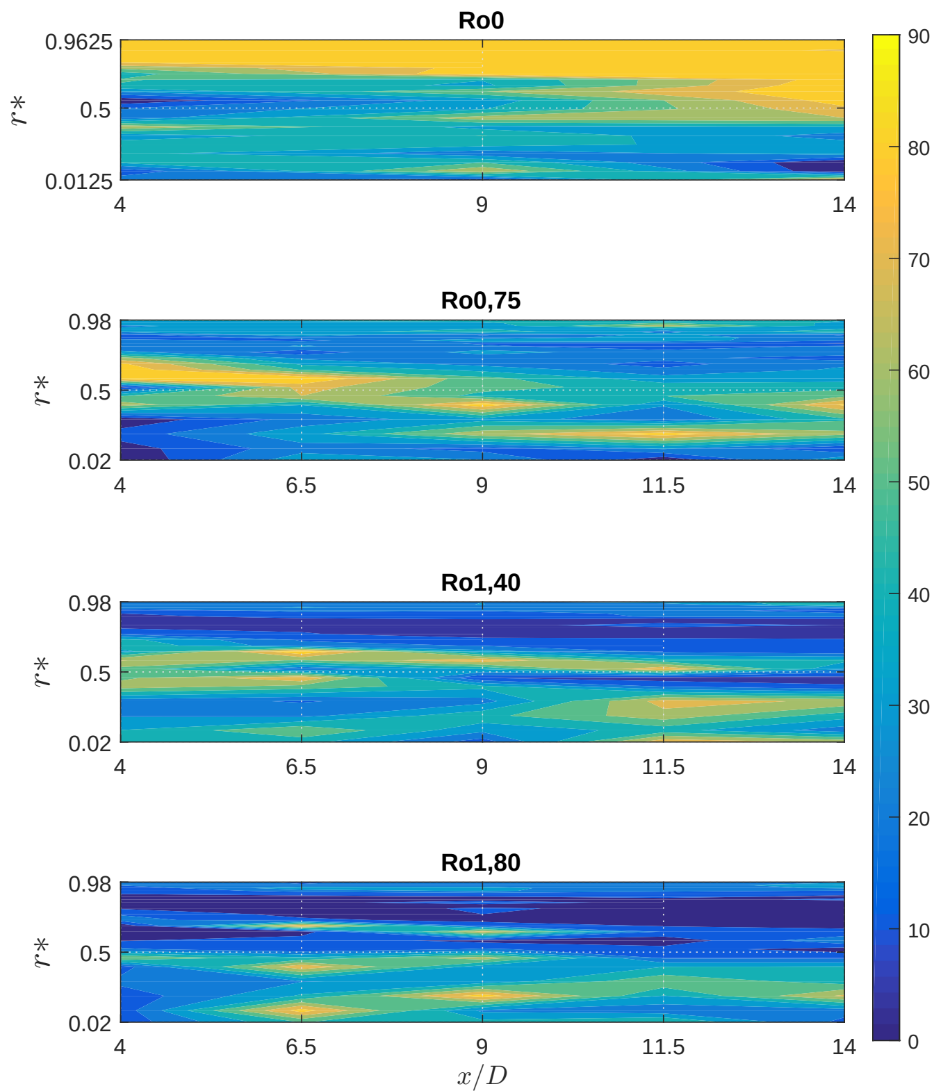
Figura 6.2: Ángulo \phi_S tubería LDV [14].
