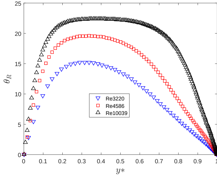
Figura 4.5: Ángulos de elevación de R para el canal DNS [12] ( D_p - XZY ).
