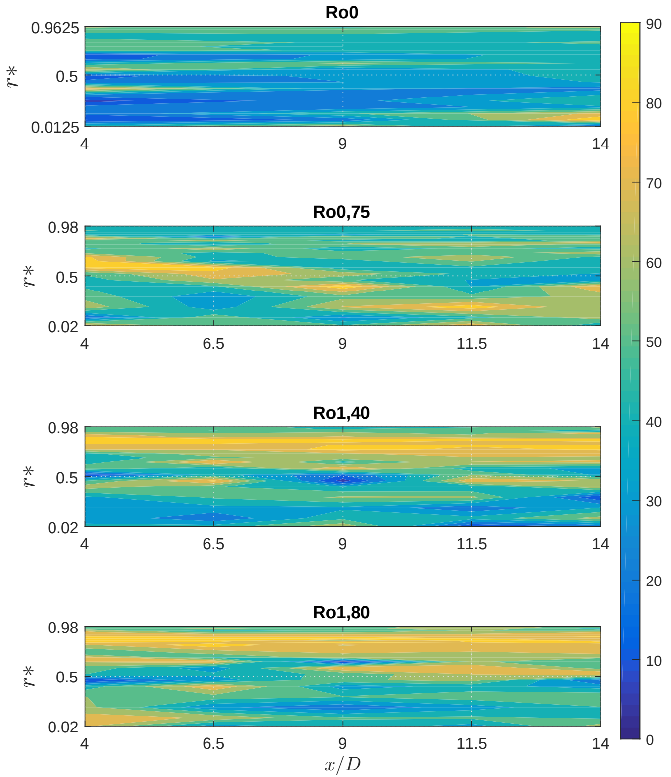
Figura 6.8: Ángulo \phi tubería LDV [14].
