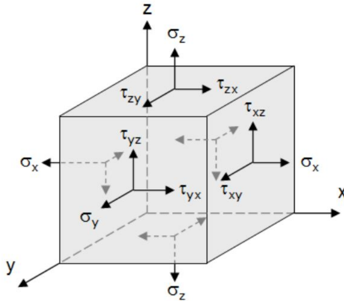
Figura 2.1: Tensor de esfuerzos que actúan sobre un elemento infinitesimal.
