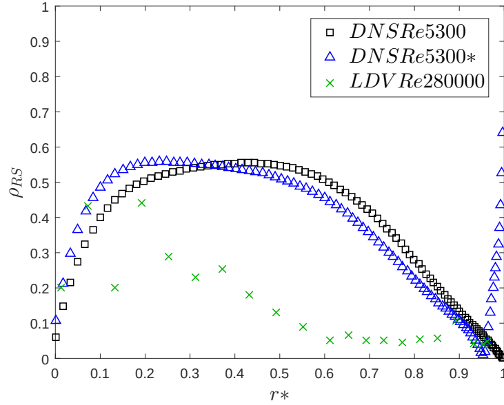
Figura 4.19: Índice de Orientación relativa entre R y S para tubería DNS.
