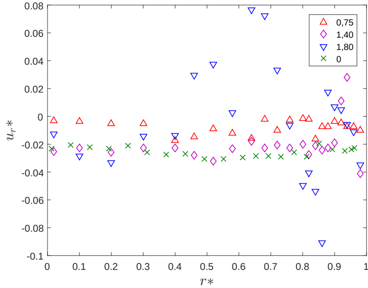
Figura 4.21: Perfiles de velocidad para Ro distintos, en la posición x = 14D en tubería LDV [14].
