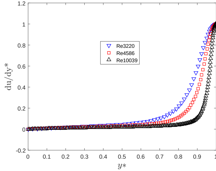
Figura 4.2: Derivada de la velocidad \bar{u}^* con respecto al ancho y^* del canal DNS .
