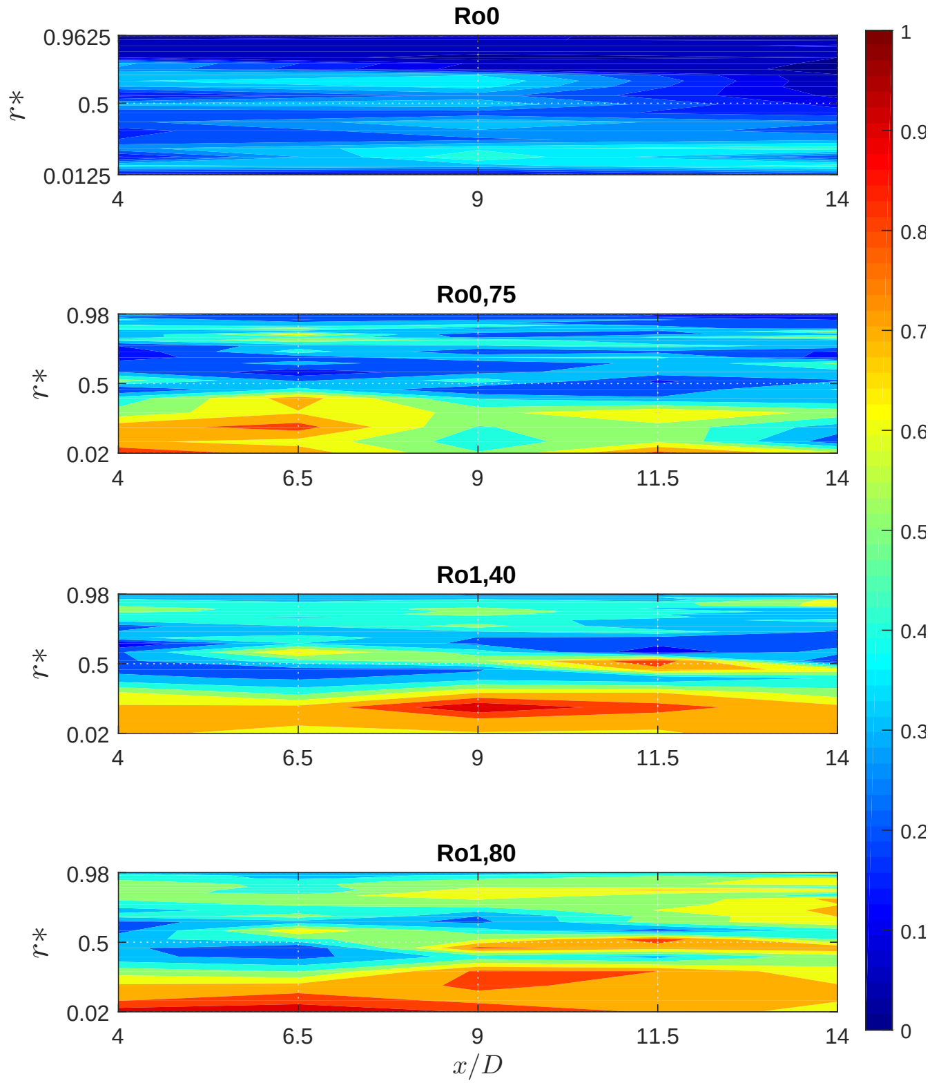
Figura 4.26: Orientación relativa entre R y S para datos LVD [14] con Ro = 0, 0,75, 1,40, 1,80 en tubería LDV [14].
