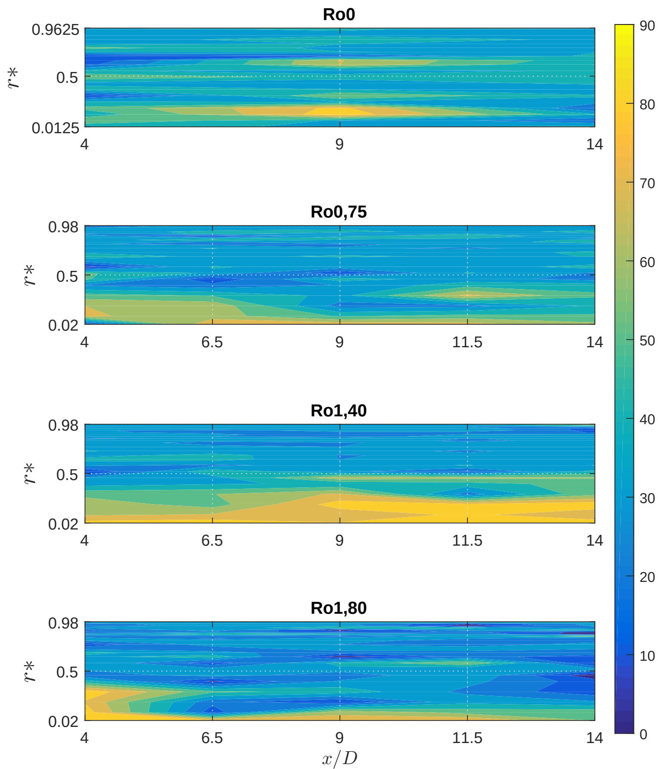
Figura 6.7: Ángulo \theta tubería LDV [14].
