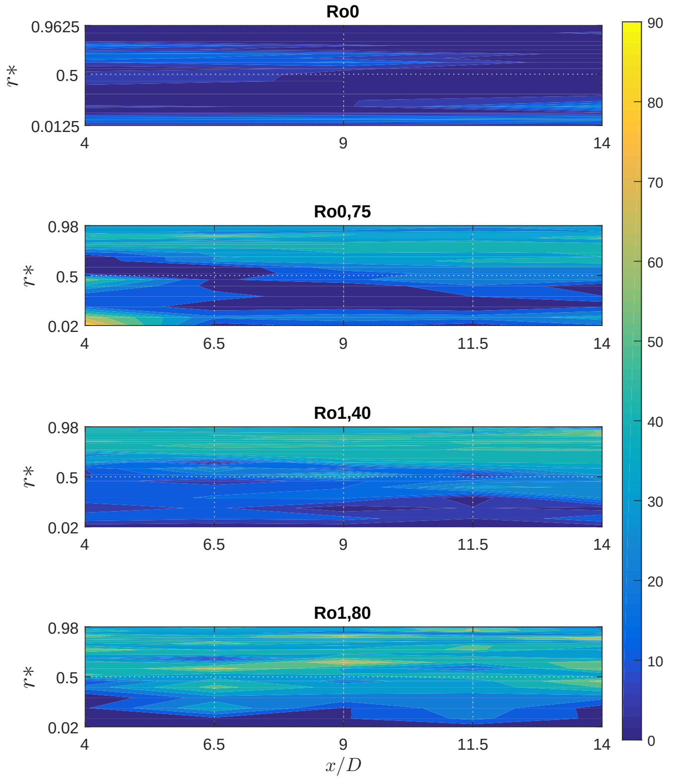
Figura 6.3: Ángulo \zeta_S tubería LDV [14].
