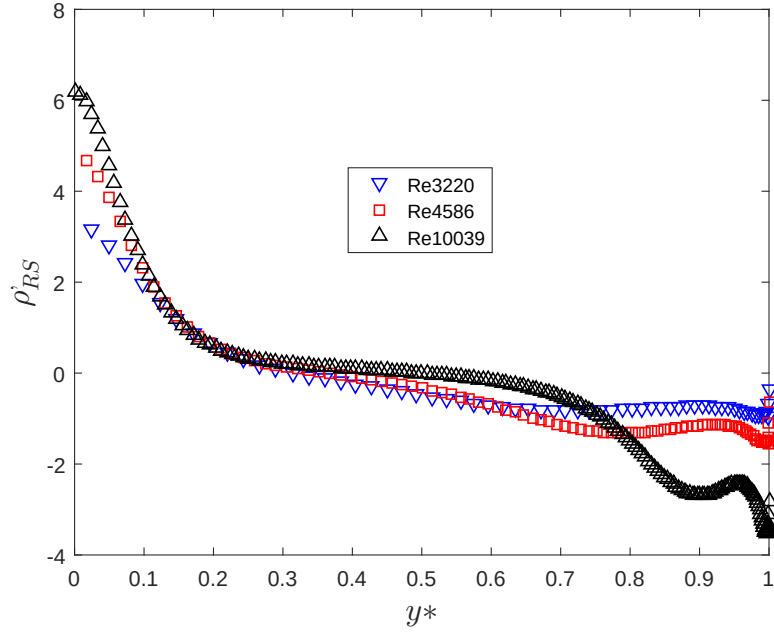
Figura 4.11: Derivada de \rho_{RS} con respecto a y^* canal DNS [12].
