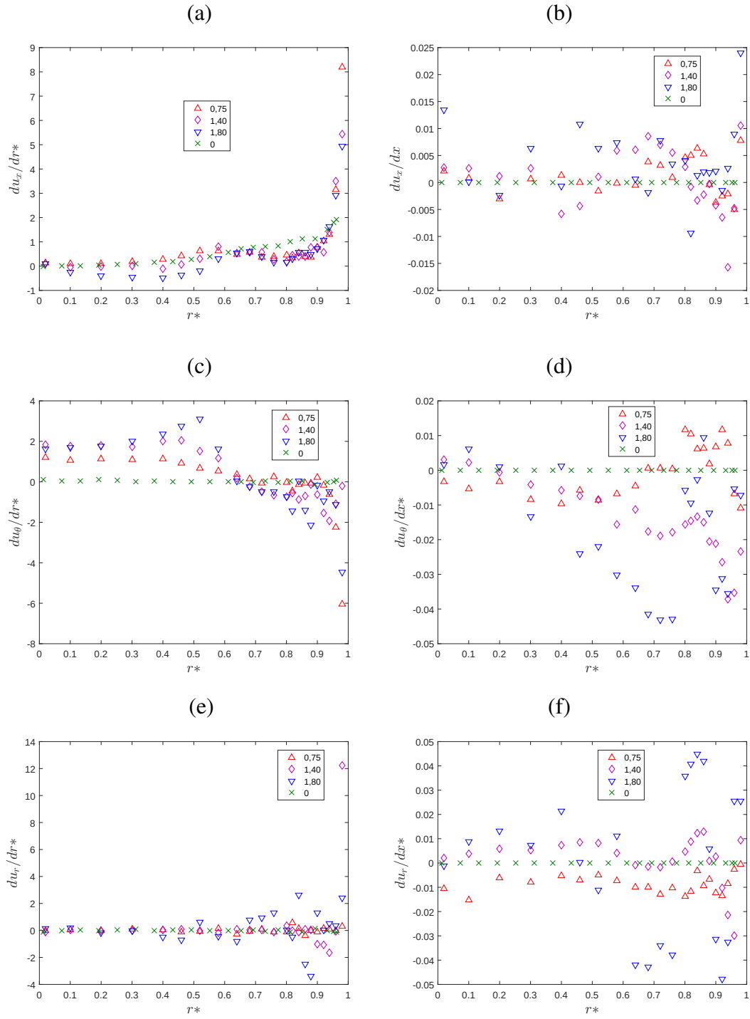
Figura 4.22: Derivadas direccionales de Datos LVD en la posición x = 14D en tubería LDV [14].
