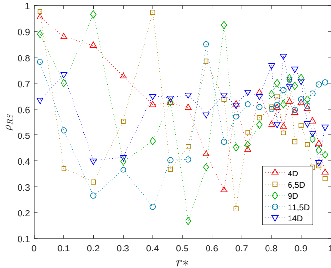
Figura 4.27: Evolución de \rho_{RS} a lo largo de la tubería LVD [14] para Ro = 1,80 .
