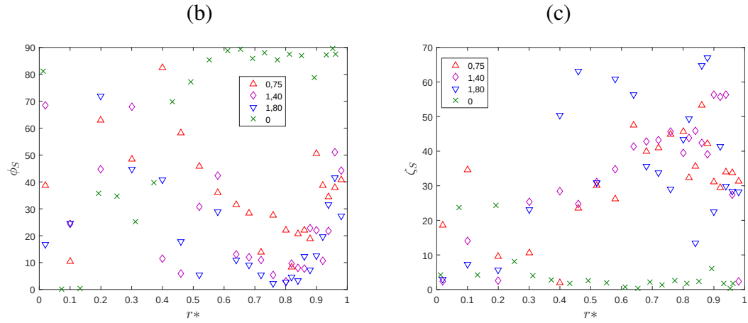
Figura 4.23: Ángulos entre D_S y X\theta r para datos LDV con x = 14D en tubería LDV [14].
