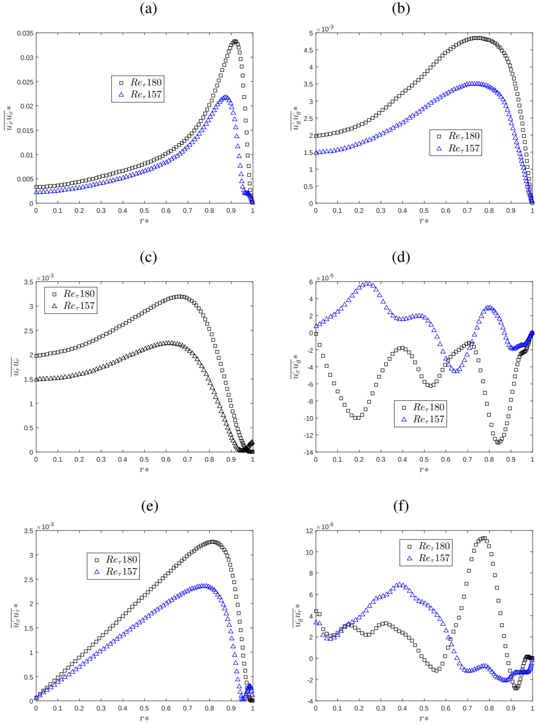
Figura 4.16: Componentes \overline{u'_i u'_j} tensor de Reynolds en tubería DNS [5]. Datos \triangle con control de Drag y \square sin.
