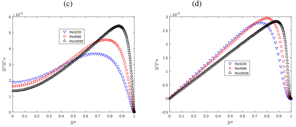
Figura 4.4: Componentes \overline{u'_i u'_j} no nulas de R en canal DNS [12].
