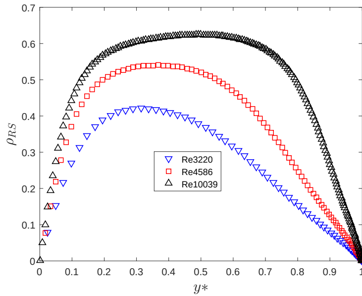
Figura 4.9: Índice \rho_{RS} canal DNS [12].
