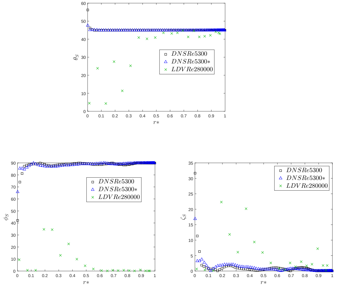
Figura 4.15: Ángulos entre D_S - X\theta r tubería DNS [5].
