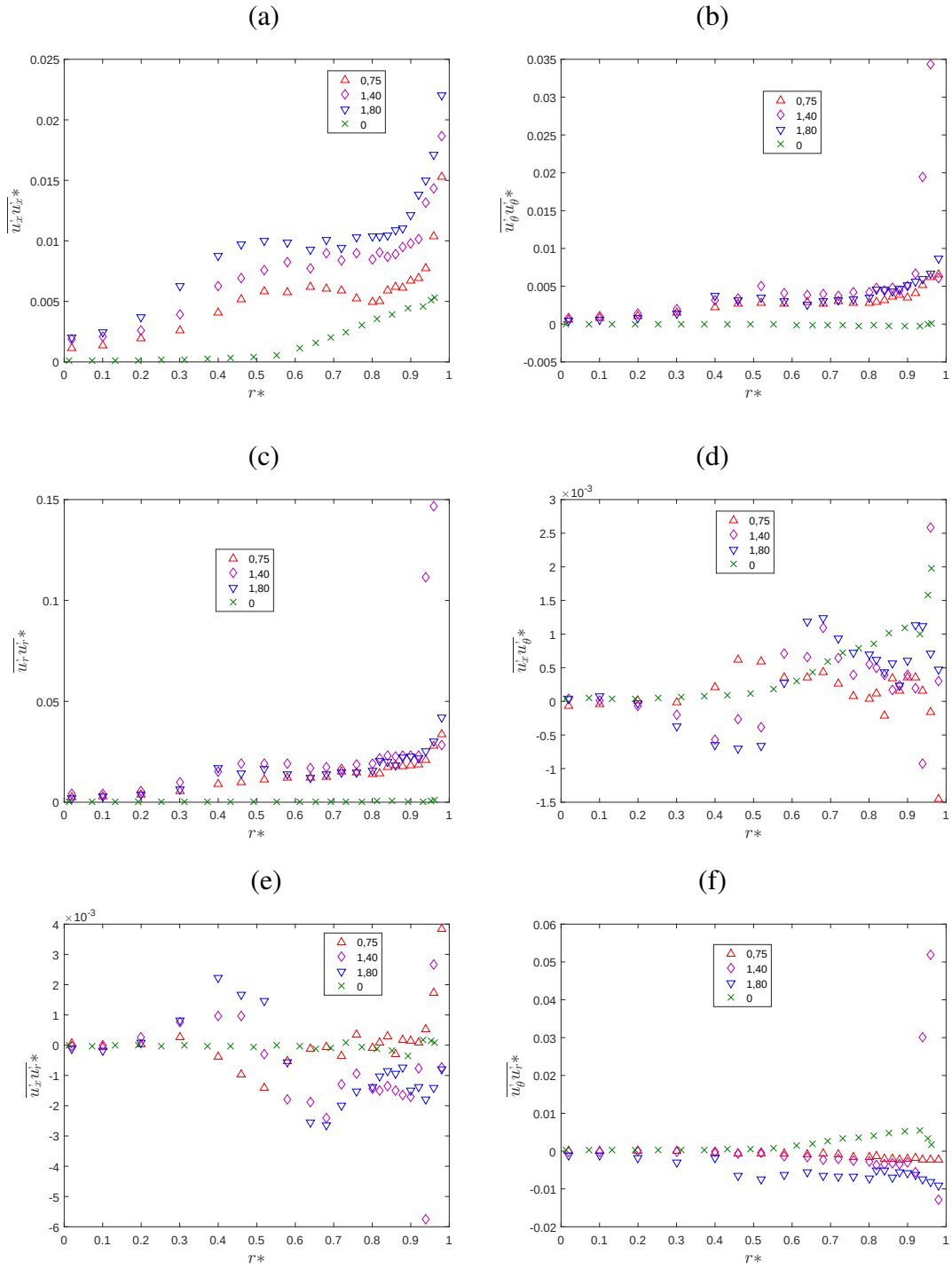
Figura 4.24: Estadísticas de turbulencia para Ro distintos, en la posición x = 14D en tubería LDV [14].
