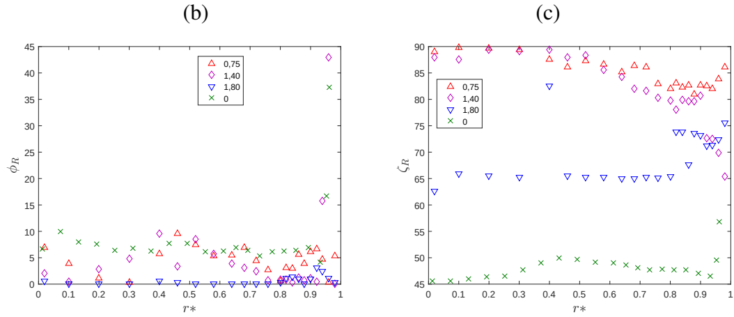
Figura 4.25: Ángulos entre D_R y X\theta r para datos LDV con x = 14D en tubería LDV [14].
