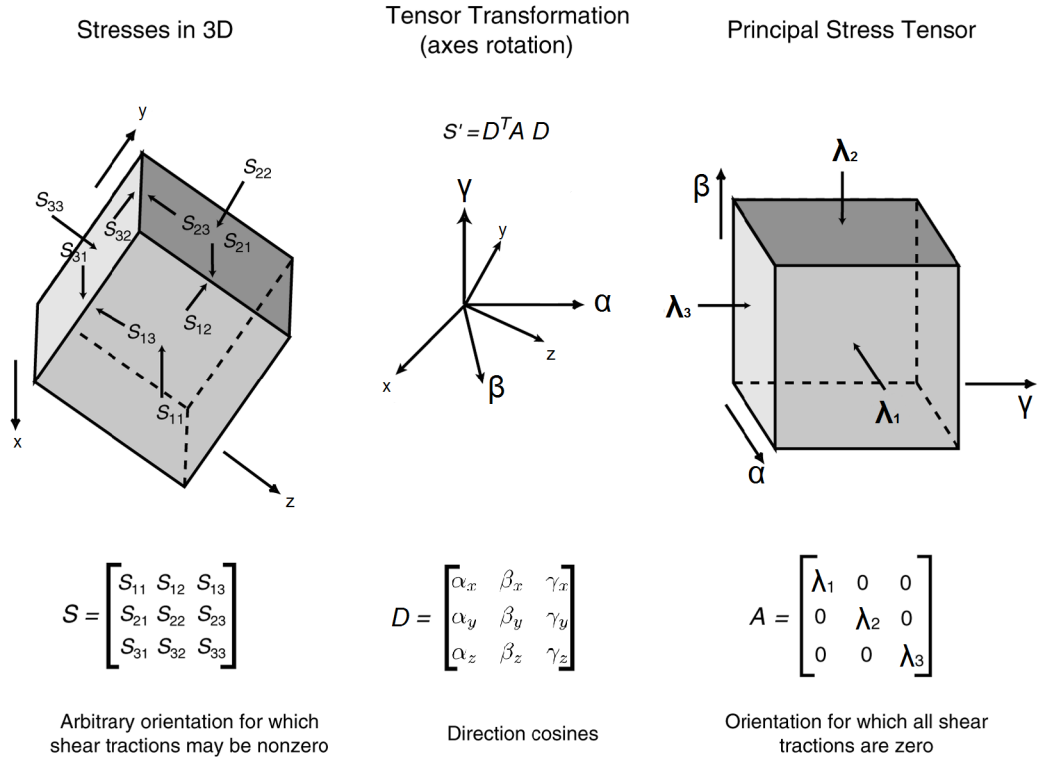
Figura 3.4: Rotación de un tensor hacia sus ejes principales.
