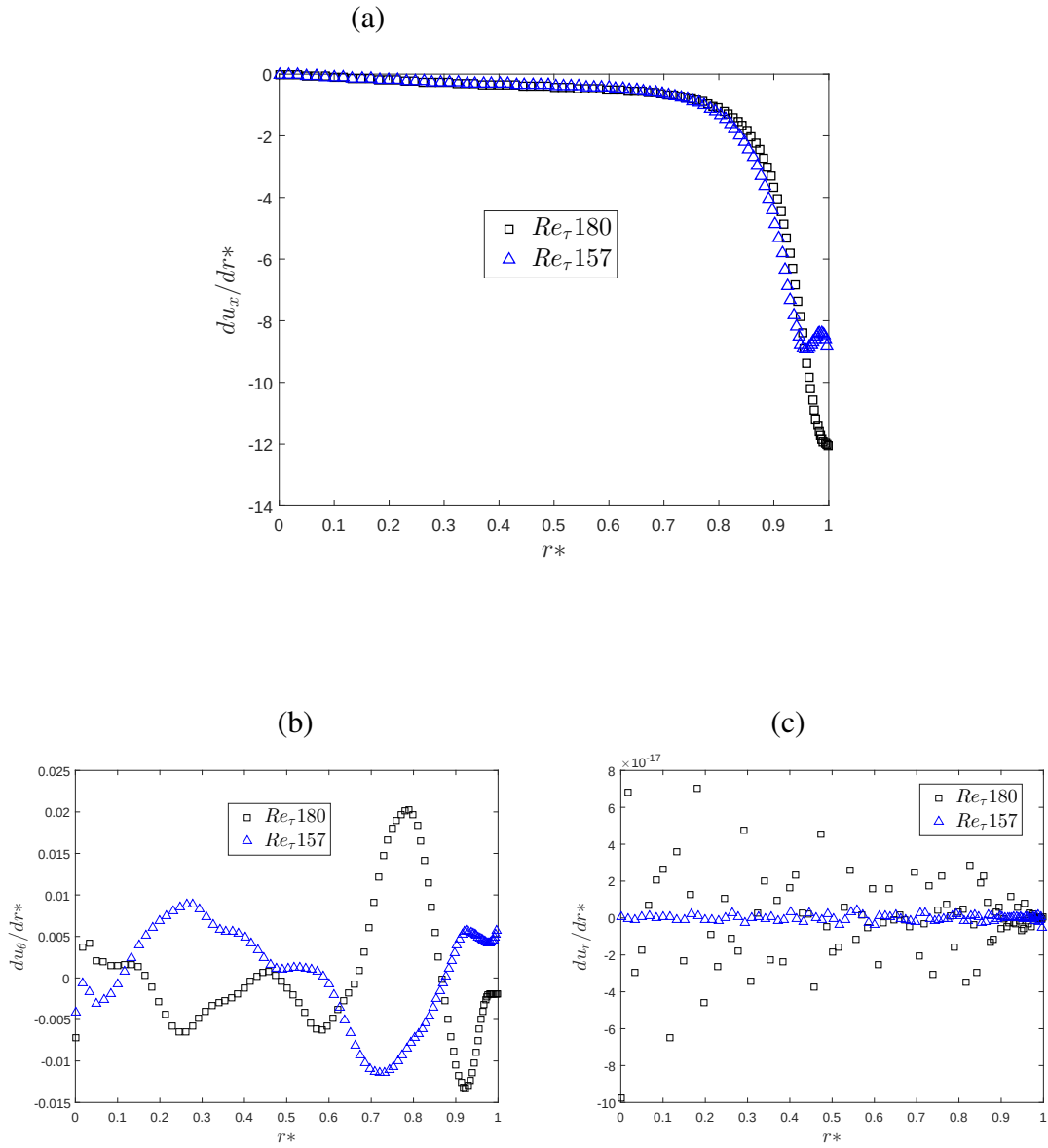
Figura 4.13: Derivadas de la velocidad con respecto a r en tubería DNS [5].
