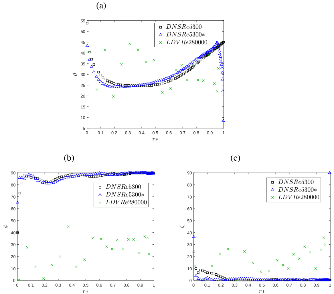
Figura 4.18: Ángulos entre D_R - D_S para tubería DNS con \triangle y sin \square control de turbulencia.
