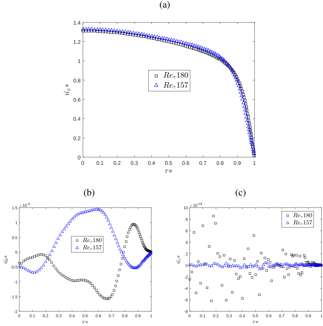
Figura 4.12: Campos de velocidad promedio (a) Axial, (b) Tangencial y (c) Radial en Tubería DNS de THTlab [5].
