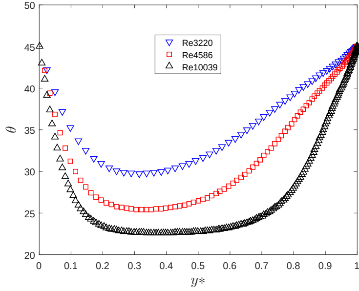
Figura 4.7: Ángulo Elevación \theta canal DNS [12] ( D_R - D_S ).
