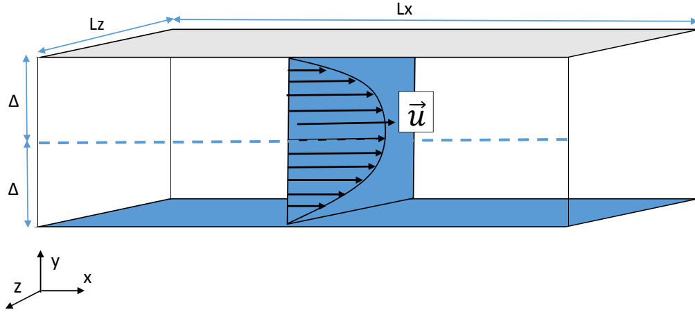
Figura 3.1: Esquema de un flujo a través de placas paralelas en coordenadas cartesianas.
