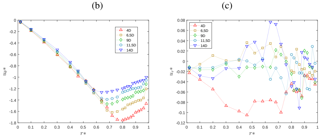
Figura 4.20: Perfiles de velocidad para Ro = 180 a lo largo de la tubería LDV [14].
