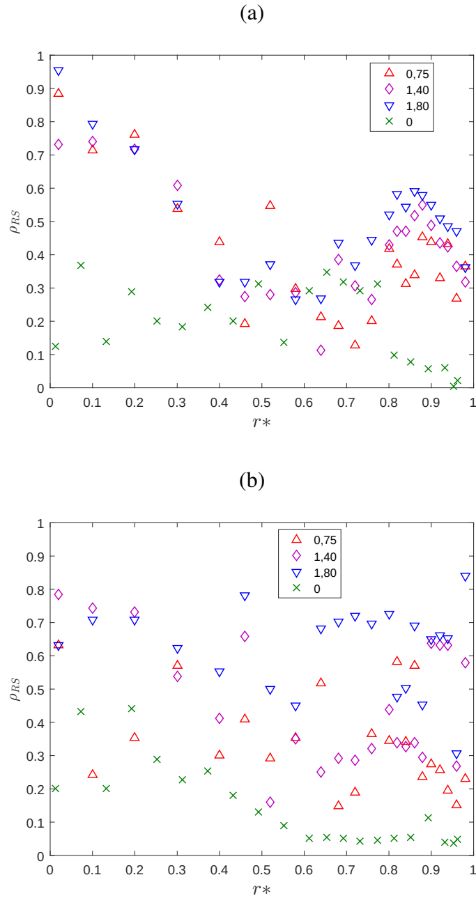
Figura 4.28: \rho_{RS} a lo largo de la tubería LVD [14] para (a) x = 4D y (b) x = 14D .
