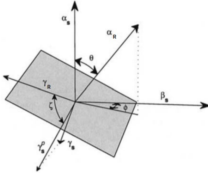
Figura 3.5: Descripción del alineamiento relativo entre dos tensores ortogonales [10].
