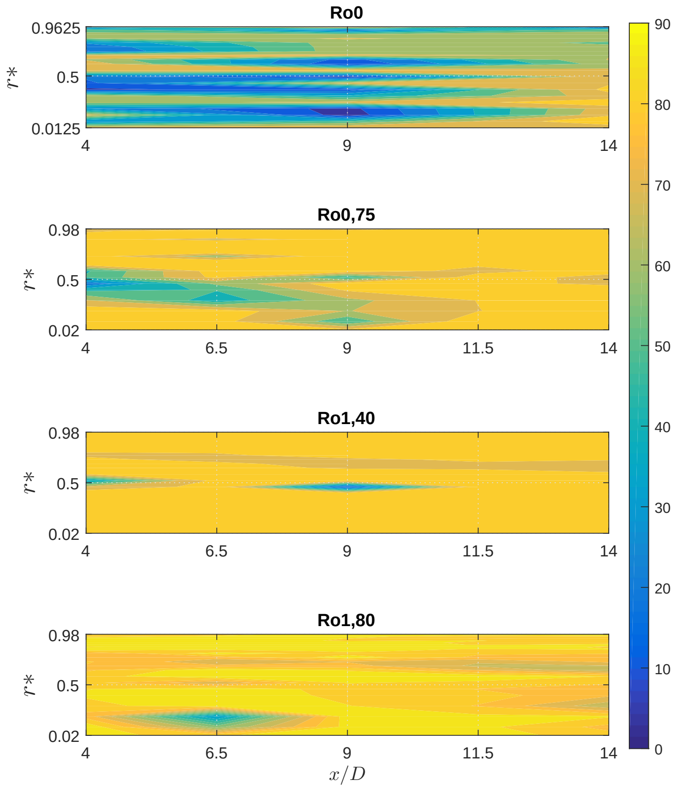
Figura 6.6: Ángulo \zeta_R tubería LDV [14].
