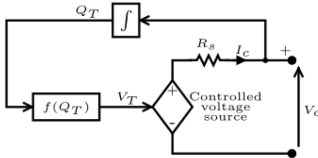
Figura 3.10: Modelo no lineal de SC [7]
