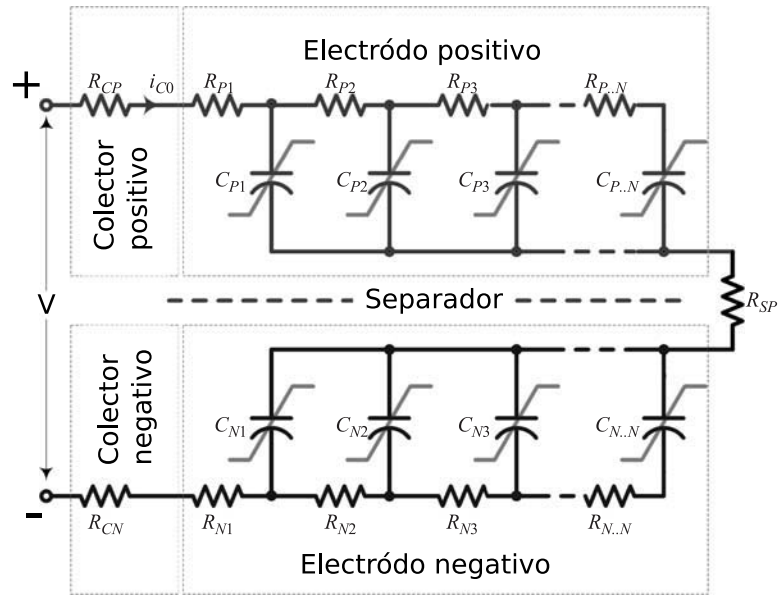
Figura 2.4: Modelo equivalente elctrico de SC [2]
