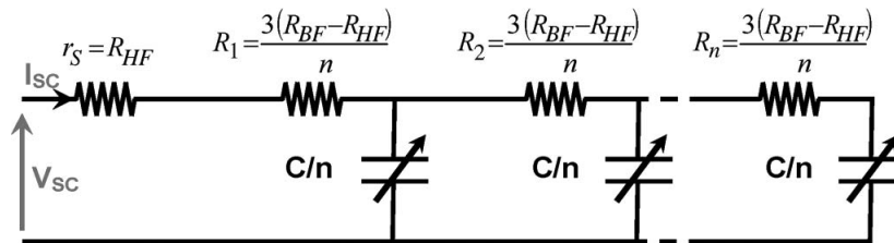
Figura 3.6: Modelo híbrido de SC
