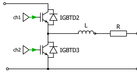
Figura 8.3: Convertidor Chopper
