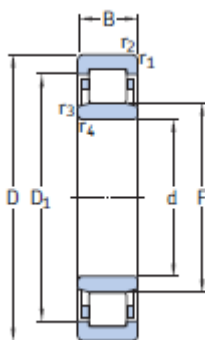
Figura 2-1. Plano rodamiento tipo NU
