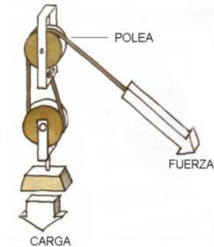
Figura 2: Polipasto griego.
