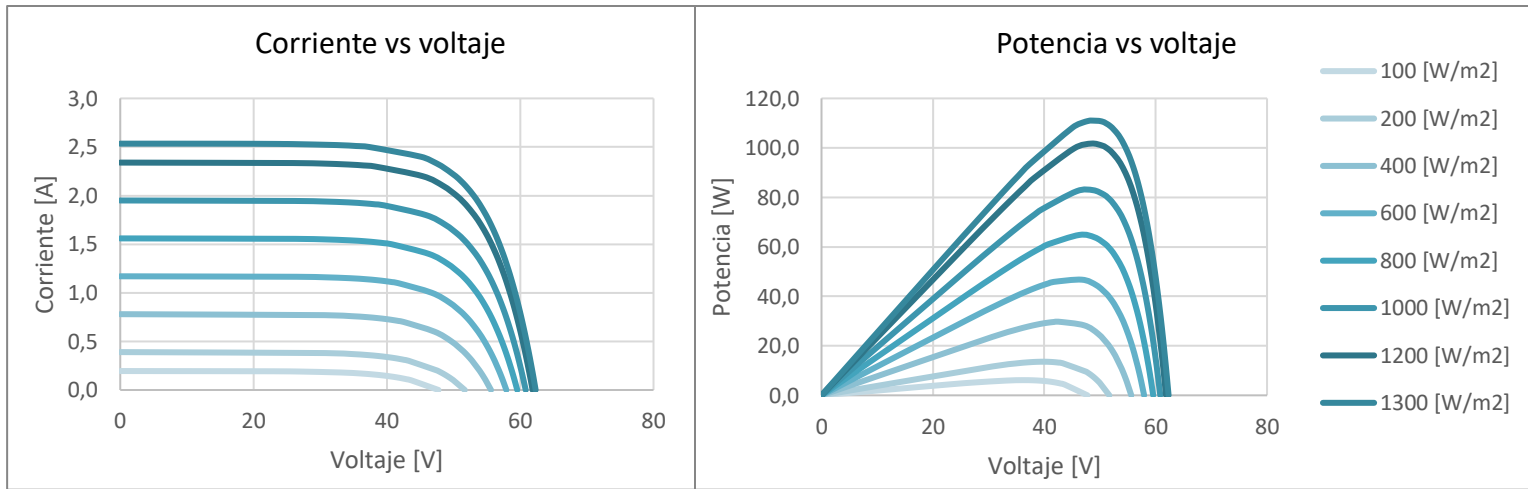
Figura 8.2 Curvas características celda fotovoltaica modelo FS-382
