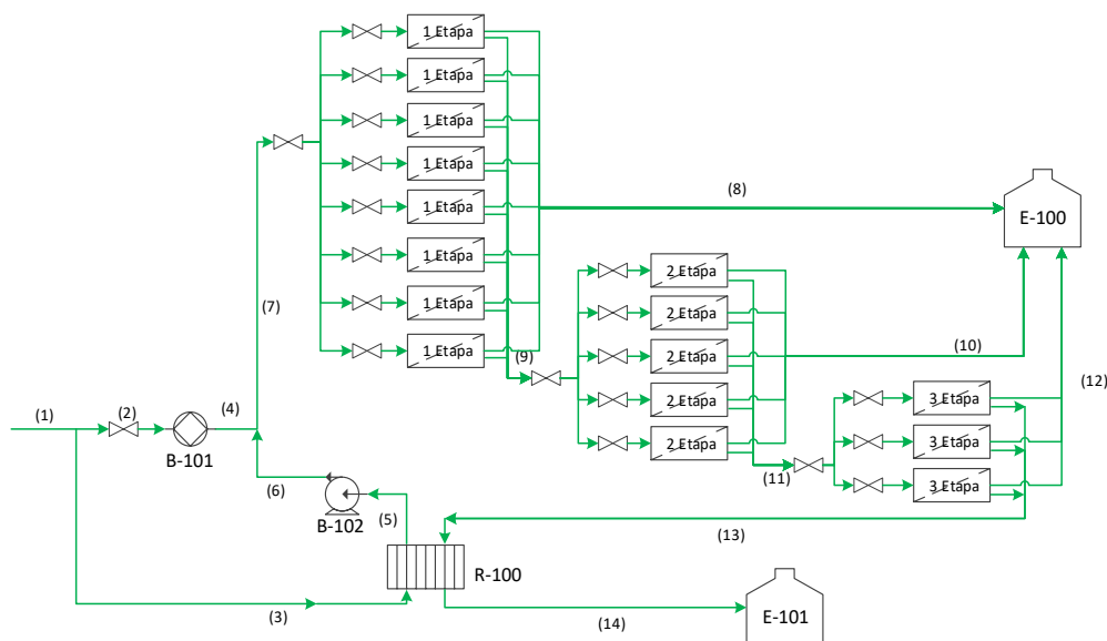
Figura 8.4 Configuración propuesta para el sistema de osmosis inversa
