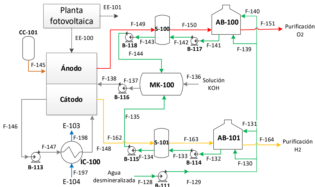
Figura 5.9 Diagrama de flujo de electrolizador alcalino
