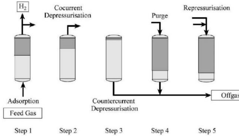
Figura 5.18 Esquema simplificado del proceso de adsorción por oscilación de presión (PSA) [270]
