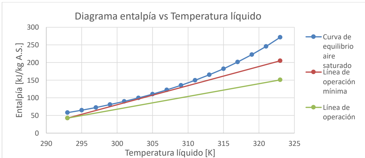
Figura 5.31 Curva de equilibrio y línea de operación de la torre de enfriamiento
