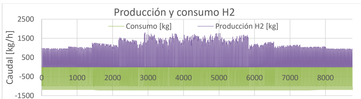
Figura 5.8 Producción y consumo de H 2 en estanques
