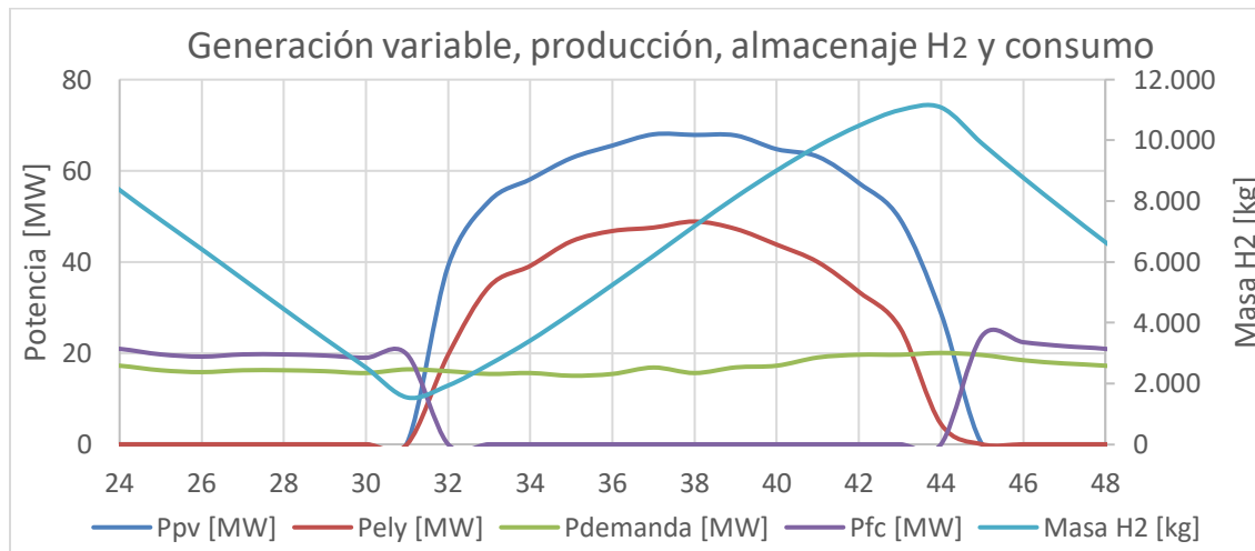
Figura 5.6 Perfil de potencia del sistema de almacenamiento 2do día de enero
