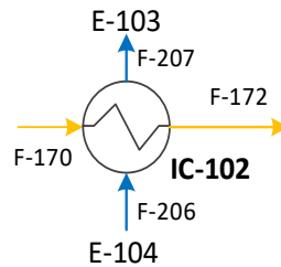
Figura 5.23 Intercambiador de calor IC-102 corriente de proceso de H 2 a 350 [bar]
