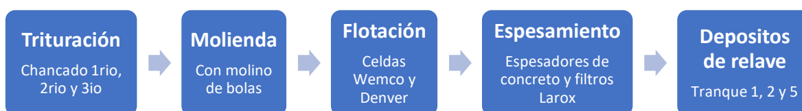
Figura 5.3 Diagrama de la planta Cerrillos [240]
