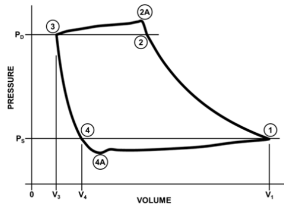
Figura 5.22 Ciclo real de compresión [281]
