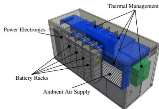
Figura 7.1 Componentes de un sistema de almacenamiento de energía en baterías [399]
