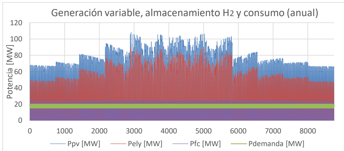
Figura 5.7 Resultados balance de energía anual
