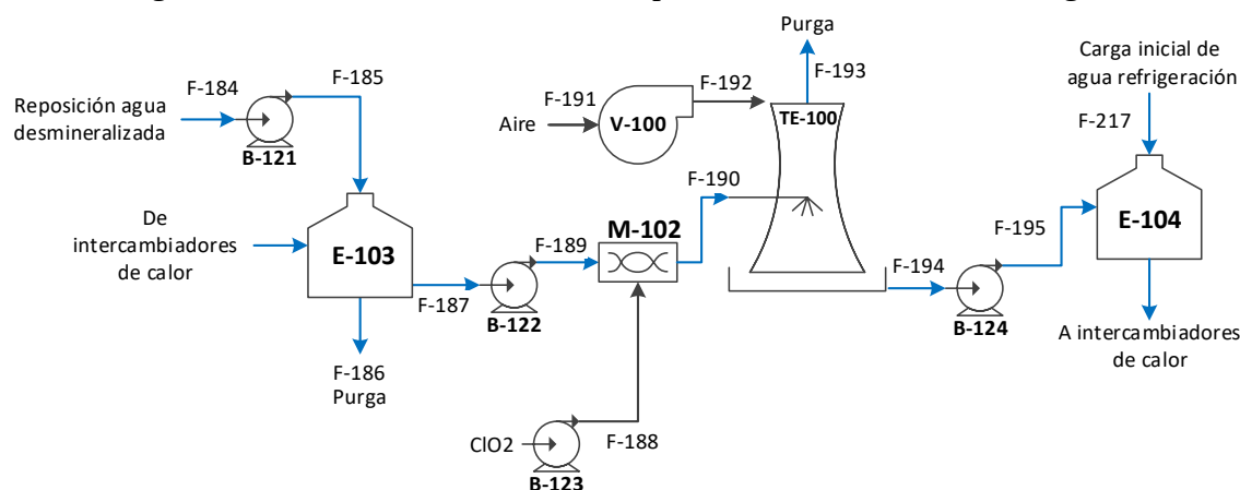
Figura 5.30 Diagrama de flujo sistema de refrigeración
