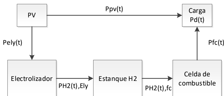
Figura 5.5 Esquema general del proceso
