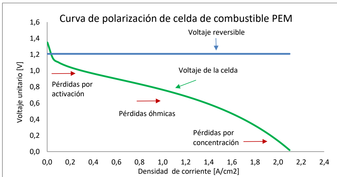
Figura 5.26 Curva de polarización de celda de combustible PEM
