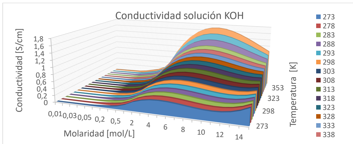
Figura 5.10 Conductividad de KOH en función de la temperatura y concentración [251]
