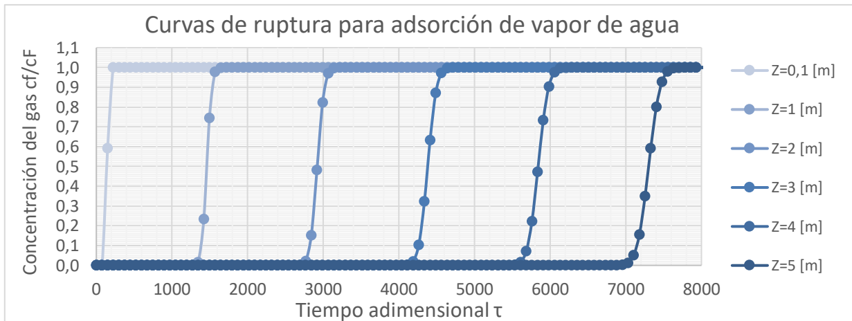
Figura 5.19 Curvas de ruptura de la columna de adsorción de vapor de agua.
