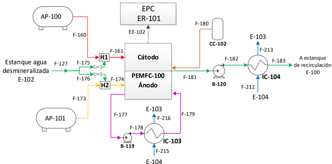
Figura 5.25 Proceso de generación de electricidad mediante PEMFC
