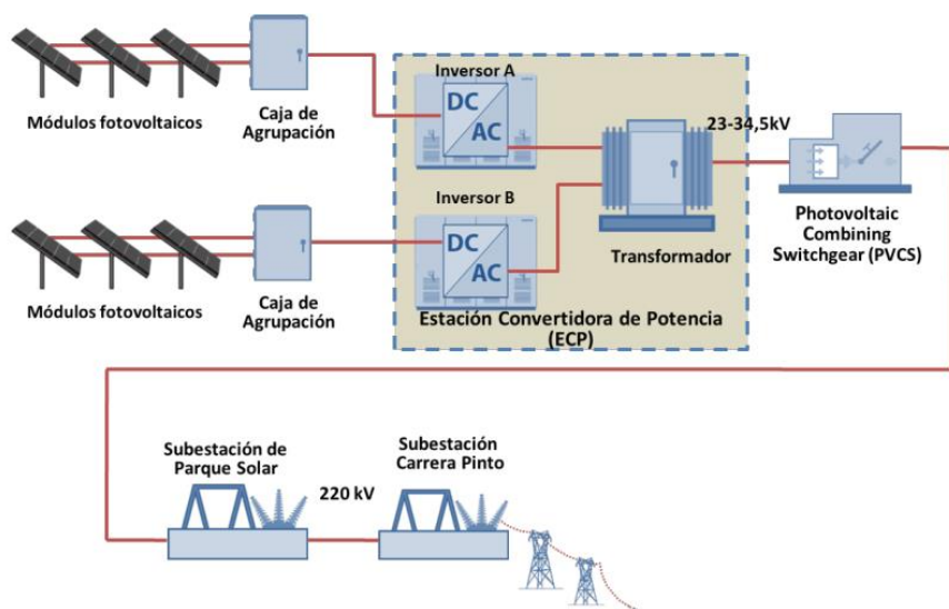
Figura 5.2 Esquema de los componentes de la planta fotovoltaica Luz del Norte [237]
