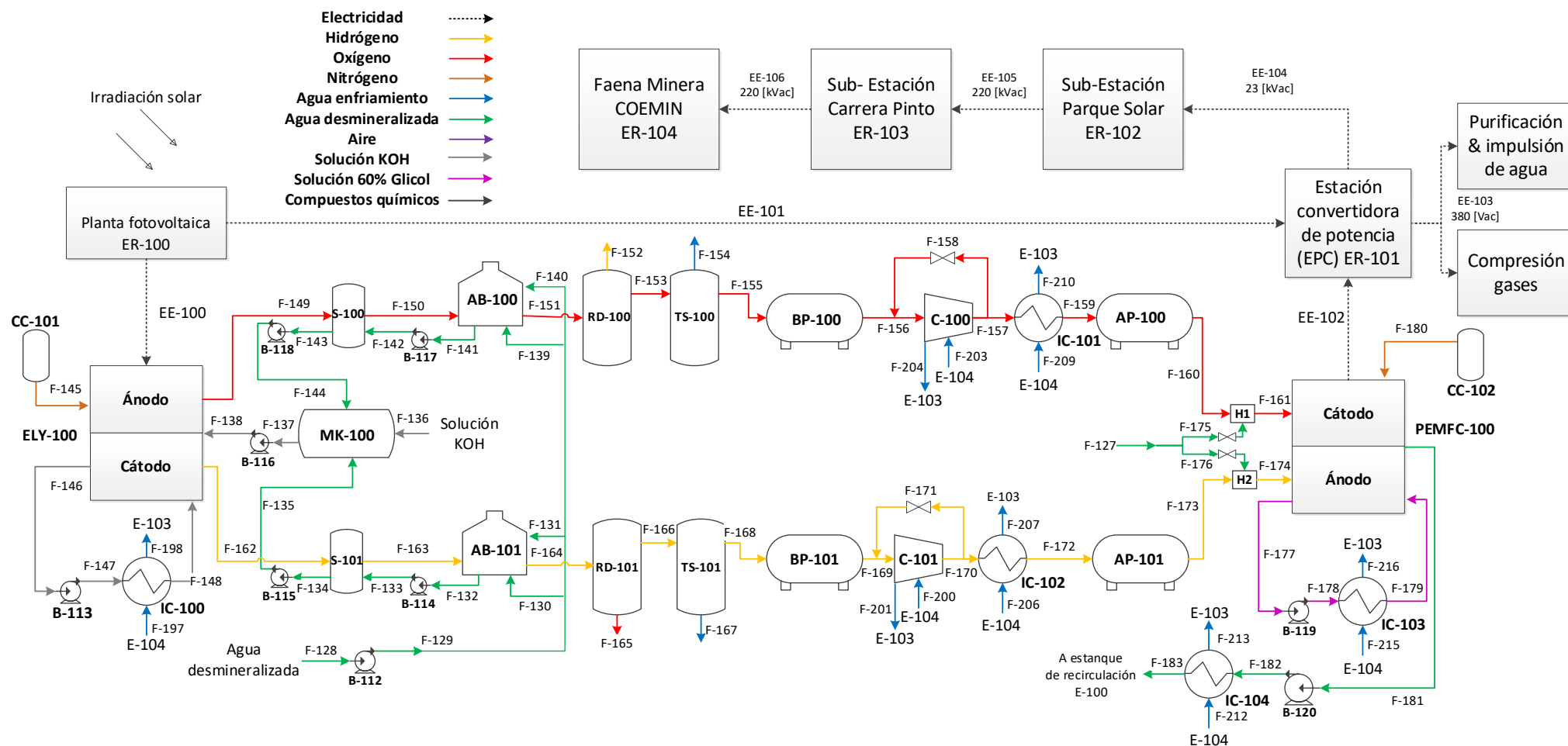
Figura 5.4 Diagrama de flujo de sistema de almacenamiento de energía de H 2
