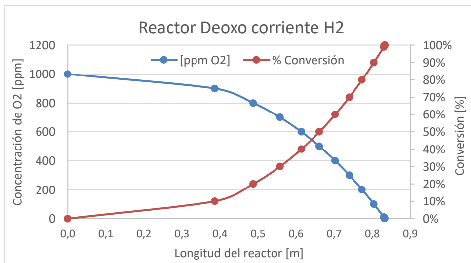
Figura 5.17 Conversión del oxígeno a lo largo del reactor
