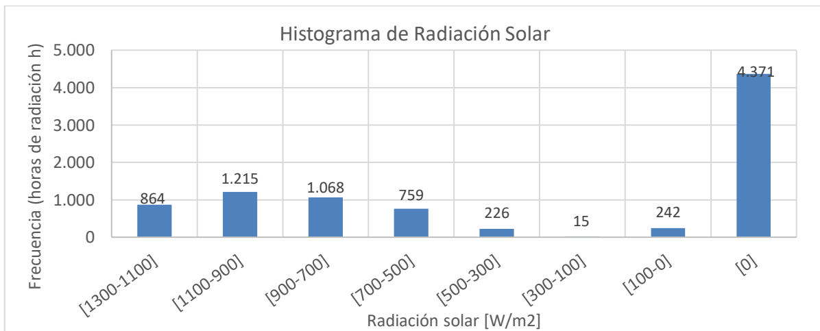
Figura 5.14 Histograma de frecuencias de radiación solar para planta fotovoltaica Luz del Norte [262]
