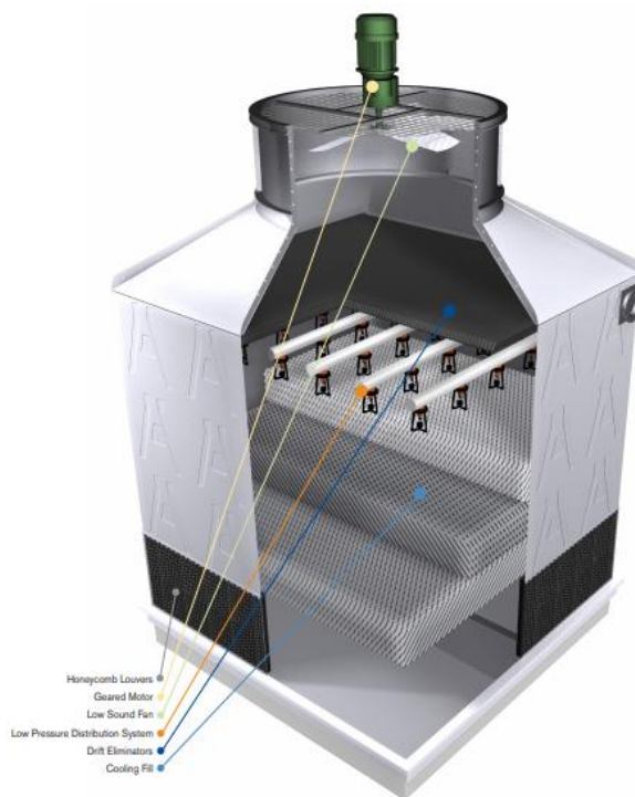
Figura 5.37 Torre enfriamiento tiro inducido modelo CP2000 [342]
