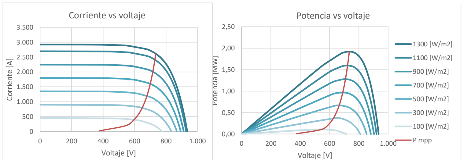
Figura 8.3 curvas características arreglo planta Luz del Norte
