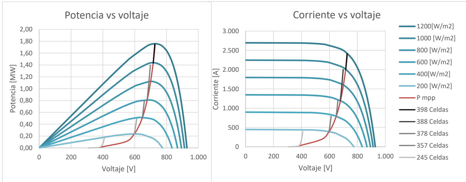
Figura 5.13 Curvas características arreglo fotovoltaico y electrolizador
