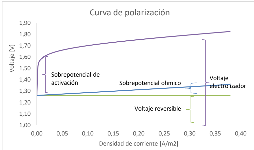
Figura 5.11 Curva de polarización del electrolizador alcalino
