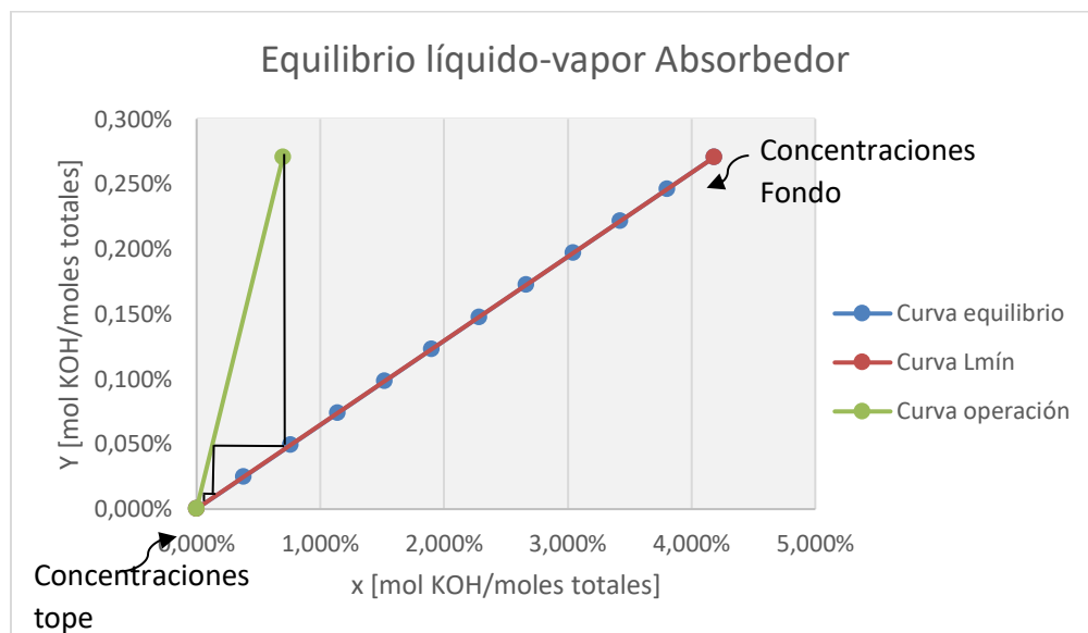
Figura 5.16 Curva de equilibrio, operación mínima y operación en columna de absorción
