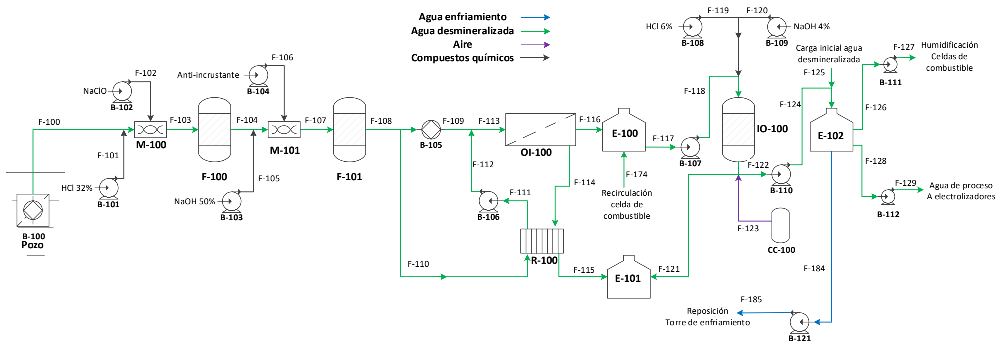
Figura 5.29 Diagrama de flujo planta de purificación de agua
