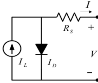
Figura 8.1 Circuito equivalente simplificado de una celda fotovoltaica [414]
