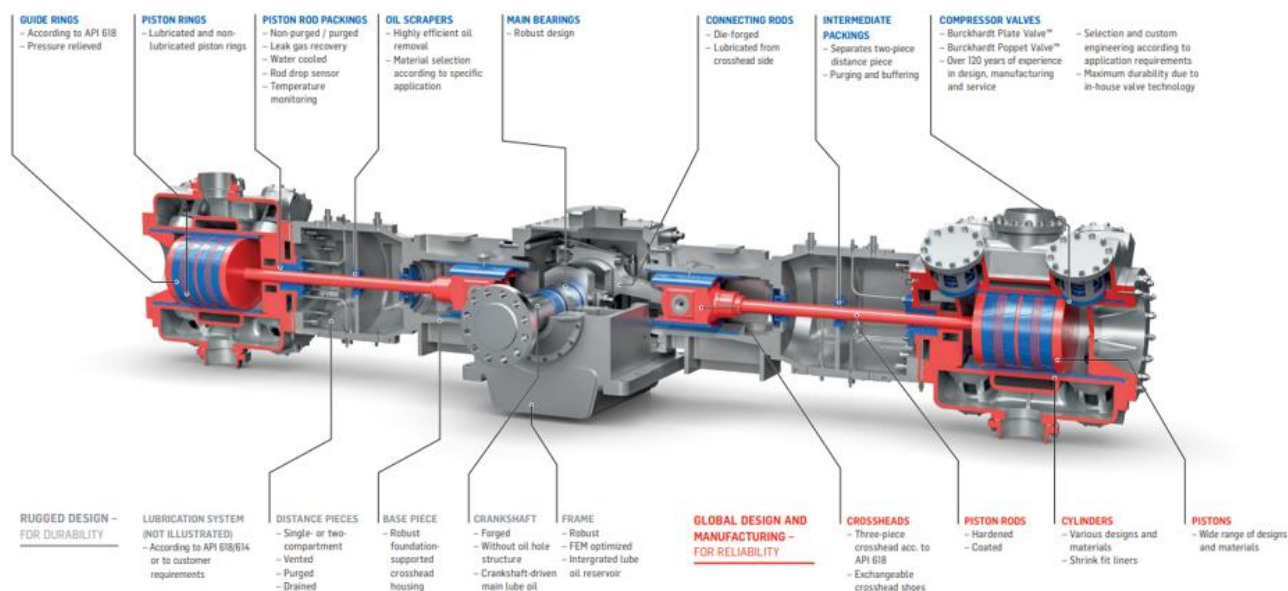
Figura 5.34 Compresor recíproco de cabezal cruzado, Burckhardt Compression [340]
