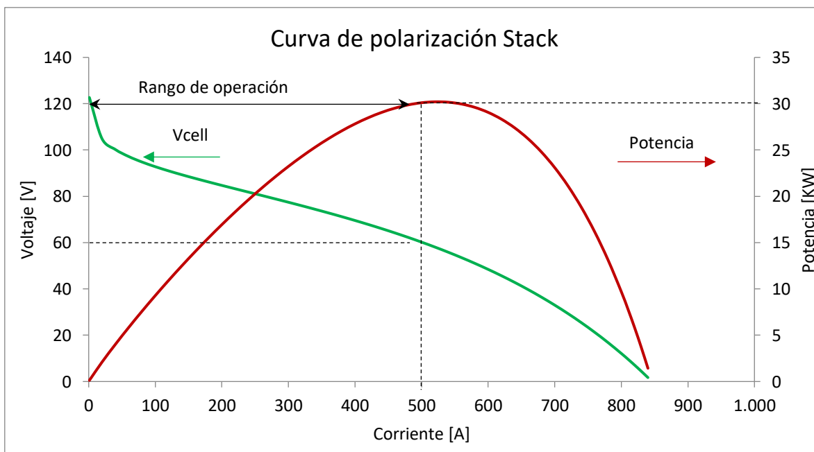
Figura 5.27 Curva operacional de la celda de combustible propuesta
