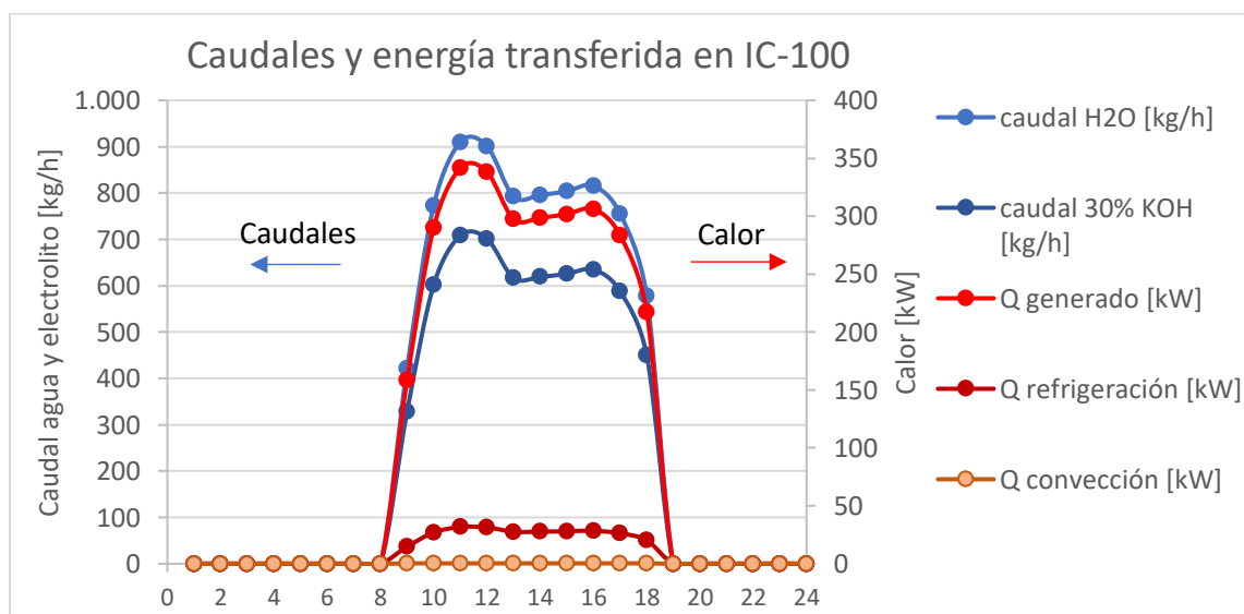
Figura 5.12 Resultados balance de energía electrolizador alcalino
