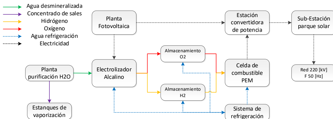
Figura 5.39 Layout del proceso
