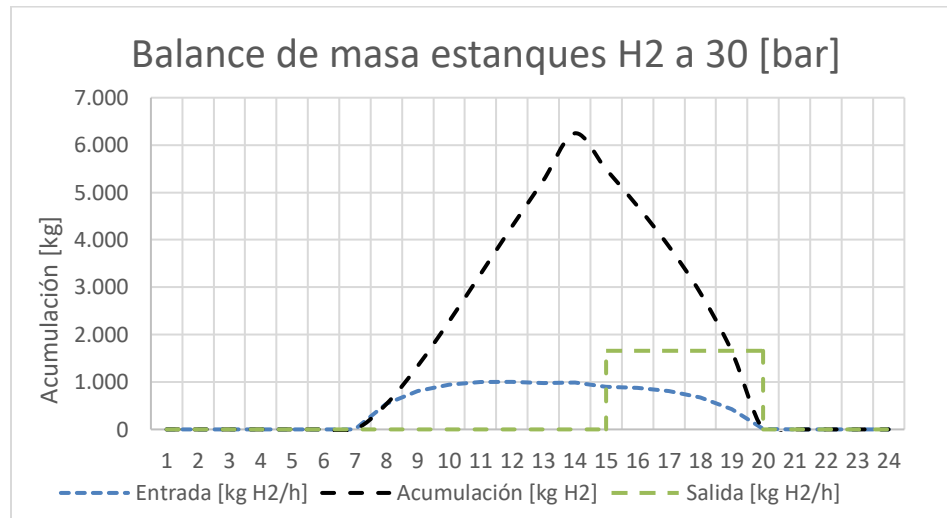
Figura 5.21 Resultado de balance de masa estanques de hidrógeno a presión de 30 [bar]
