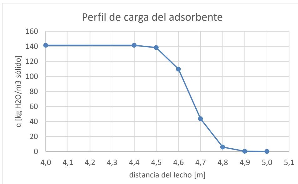
Figura 5.20 Perfil de carga de la columna de adsorción
