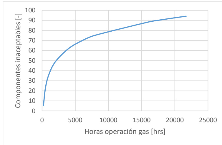
Gráfico 4.6: Curva teórica del modelo de regresión obtenido, alabe móvil de 1º etapa SI2.
