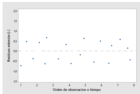
Gráfico 1.1: Grafico que representa ausencia de errores o residuos (estándar) correlacionados en el orden de observación o tiempo.
