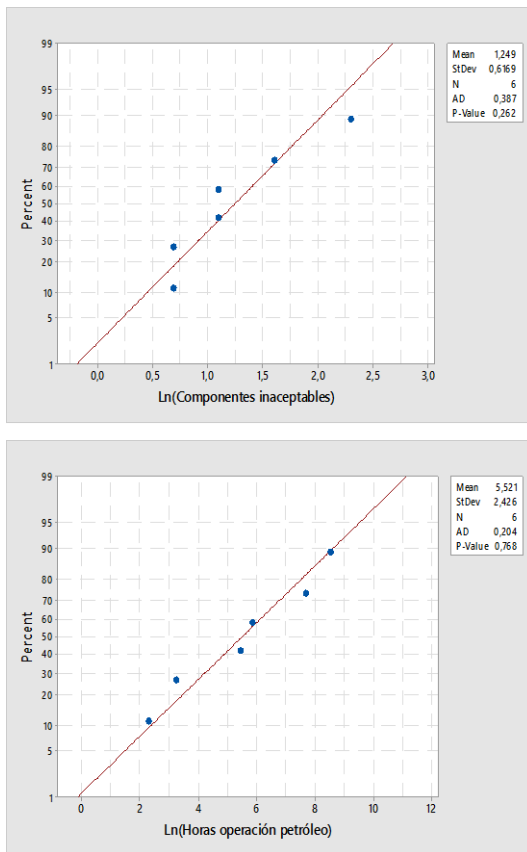
Figura 3.23: Gráfico de probabilidad normal y estadístico AD para variable Ln(Componentes inaceptables) (izquierda), y Ln(Horas operación petróleo) (derecha), cámara de combustión SI1.
