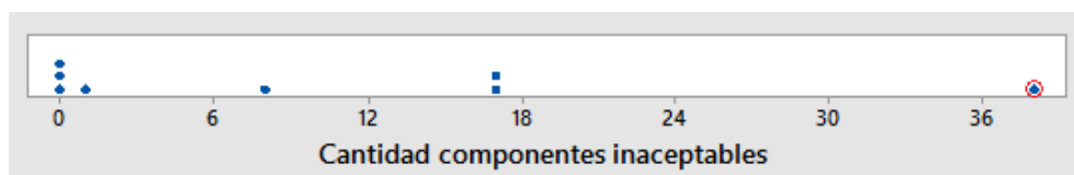
Figura 3.14: Gráfico de puntos alabe móvil de 4º etapa SI1.
