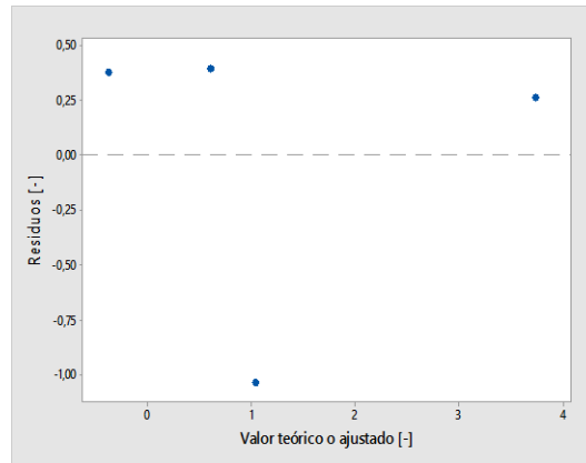
Gráfico 3.7: Grafico de residuos v/s valor teórico o ajustado del modelo, tobera piloto gas SI2.
