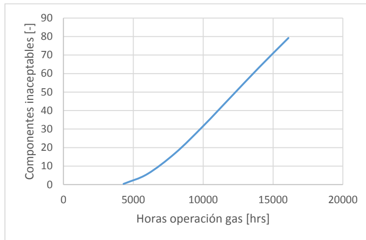
Gráfico 4.7: Curva teórica del modelo de regresión obtenido, alabe móvil de 3º etapa SI1.
