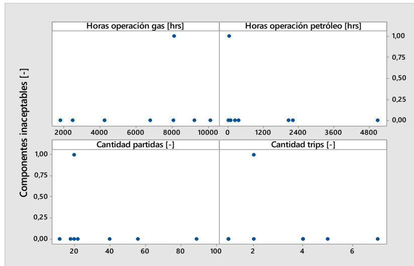
Figura 3.19: Gráficos de dispersión, datos tobera piloto principal SI1.
