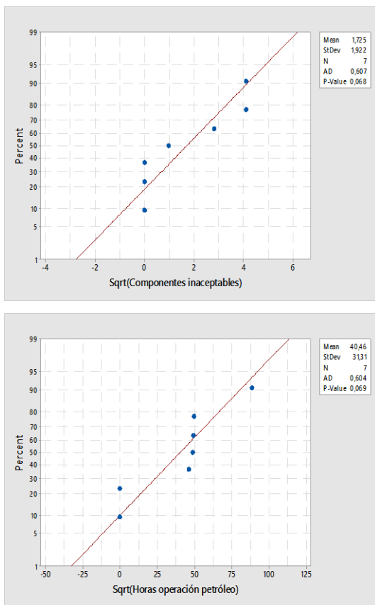
Figura 3.38: Gráfico de probabilidad normal y estadístico AD para variable Componentes inaceptables transformada (izquierda), y Horas operación petróleo transformada (derecha), alabe móvil de 4° etapa SI1.
