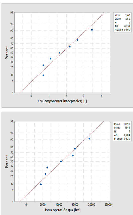
Figura 3.29: Gráficos de probabilidad normal y estadístico AD para la variable \text{Ln}(\text{Componentes inaceptable}) (derecha) y Horas operación gas (izquierda), alabe fijo de 2° etapa SI1.
