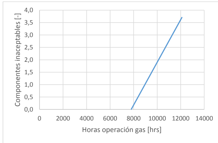
Gráfico 4.2: Curva teórica del modelo de regresión obtenido, tobera piloto gas SI2.
