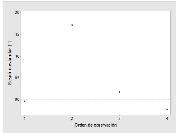
Gráfico 3.17: Gráfico de residuo estándar v/s orden de observación, ring segment de 1° etapa SI2.
