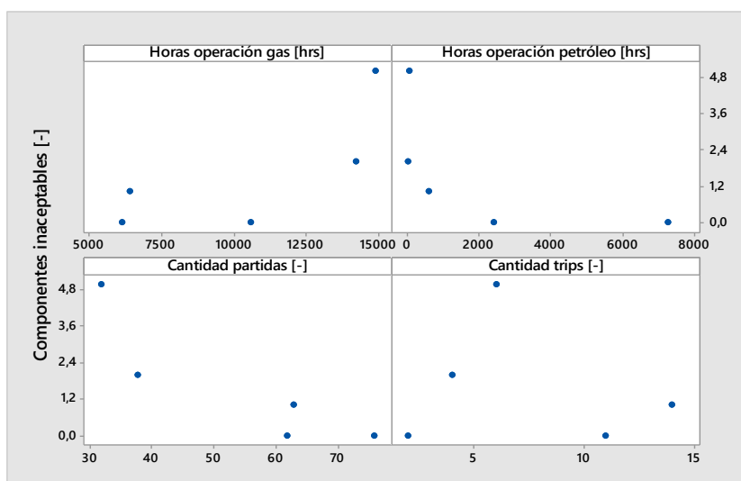
Figura 3.31: Gráficos de dispersión datos alabe móvil de 2° etapa SI1.
