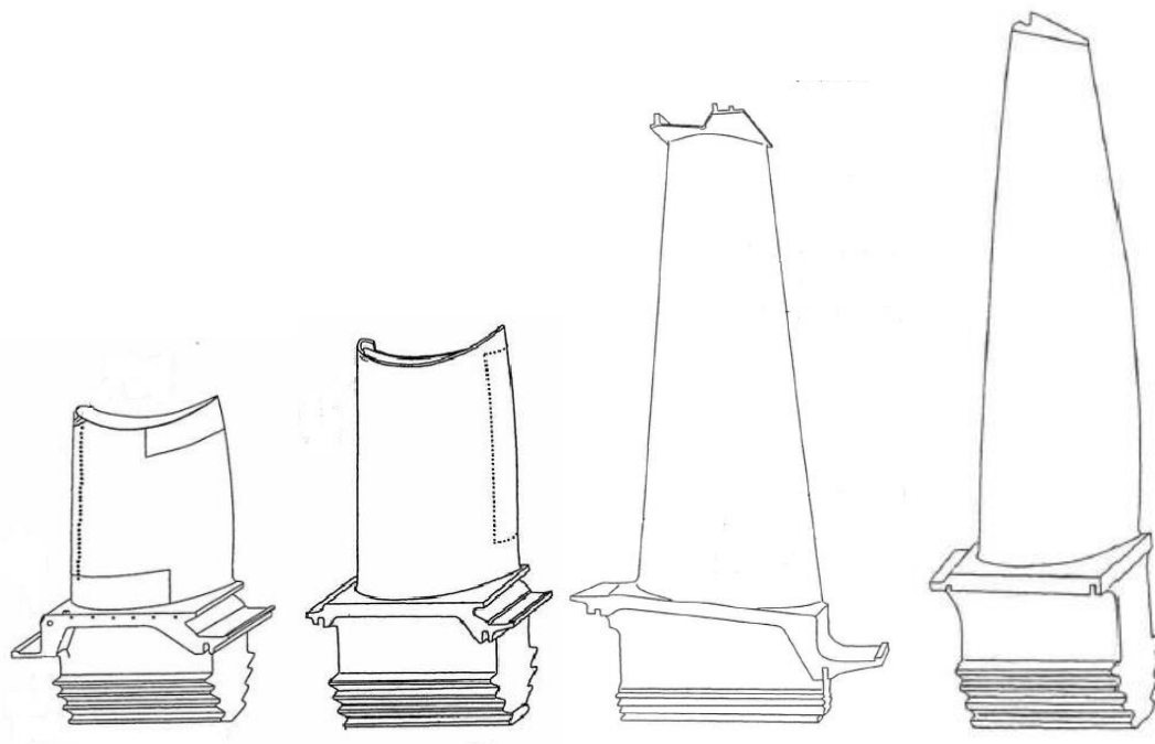
Figura 3.8: Alabes móviles de 1°, 2°, 3° y 4° etapa (en ese orden) [9]
