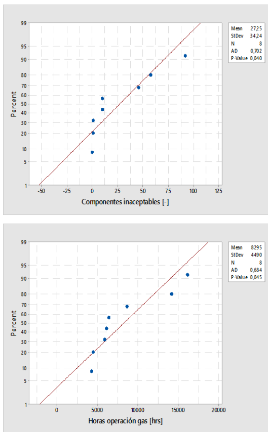
Figura 3.33: Gráfico de probabilidad normal y estadístico AD para Componentes inaceptable (izquierda), y Horas operación gas (derecha), alabe móvil de 3° etapa SI1.
