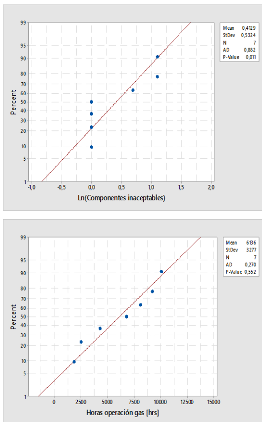
Figura 3.25: Gráfico de probabilidad normal y estadístico AD para variable Ln(Componentes inaceptables) (izquierda), y Horas operación gas (derecha), pieza de transición SI1.
