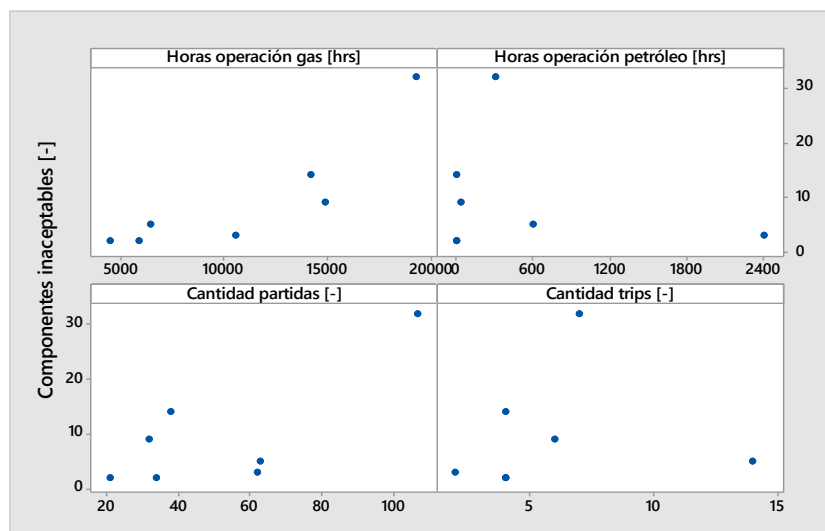
Figura 3.28: Gráficos de dispersión datos alabe fijo de 2° etapa SI1.
