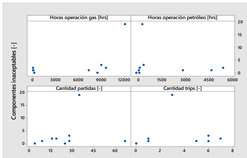
Figura 3.49: Gráficos de dispersión, pieza de transición SI2.
