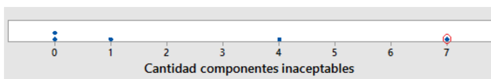
Figura 3.15: Gráfico de puntos tobera piloto gas SI2.
