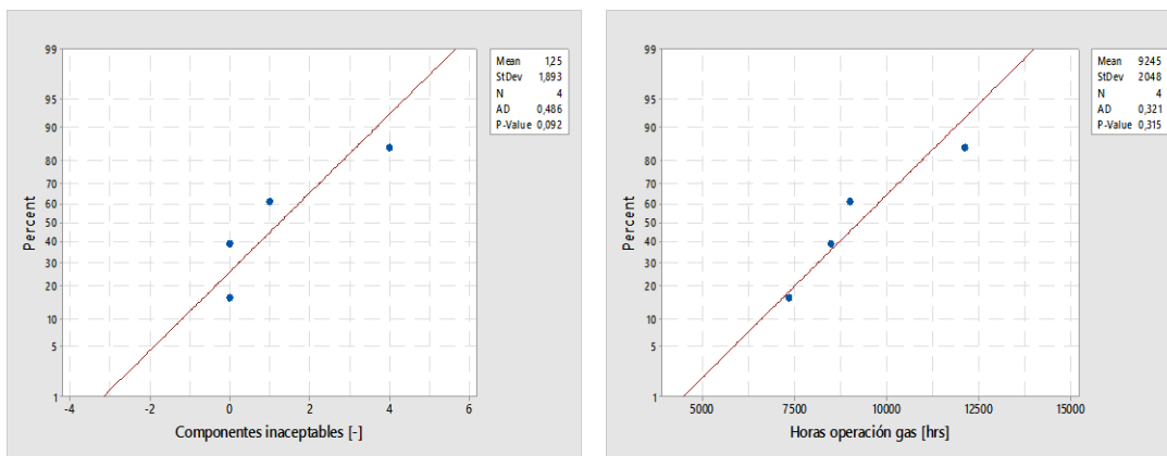
Figura 3.44: Gráficos de probabilidad normal y estadístico AD para las variables Componentes inaceptables (izquierda) y Horas operación gas (derecha), tobera piloto gas SI2.
