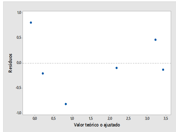
Gráfico 3.1: Residuos v/s valor teórico o ajustado del modelo, alabe fijo de 1º etapa SI1.
