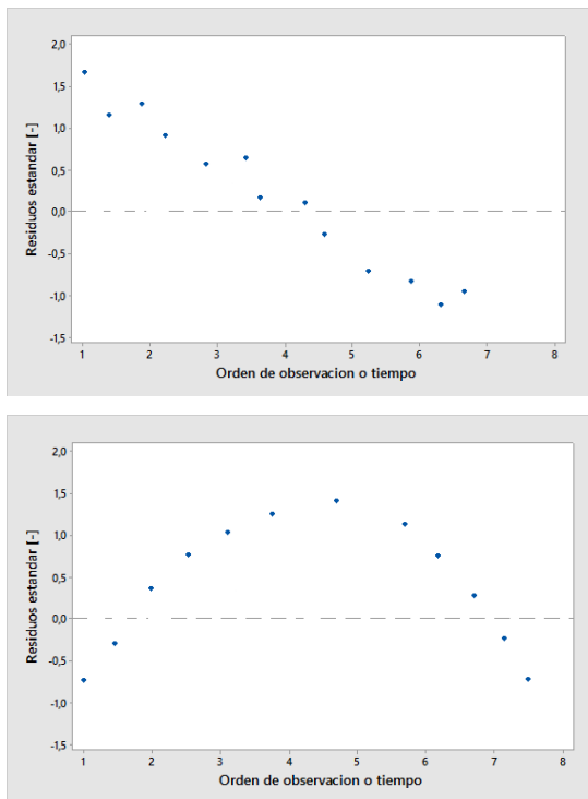
Figura 1.5: Gráficos con patrones comunes que representan presencia de errores correlacionados.
