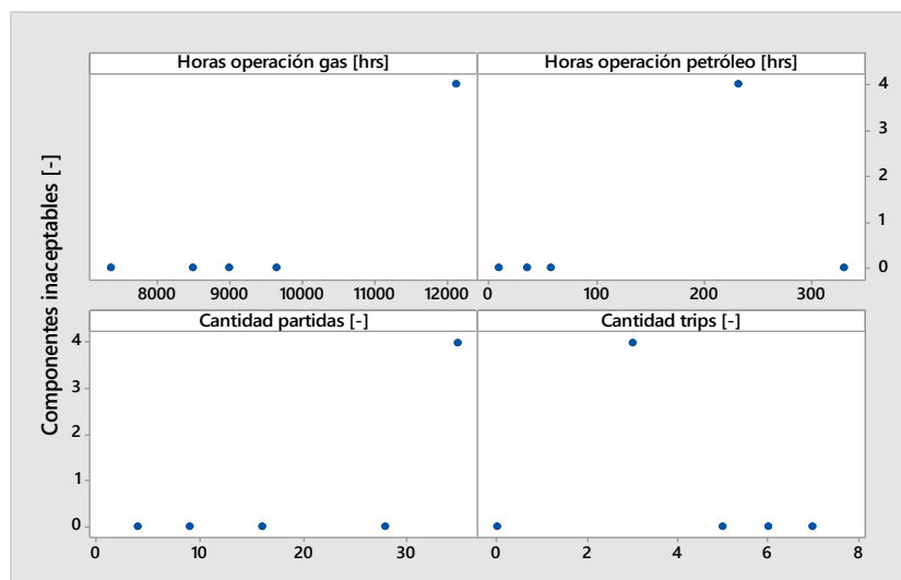
Figura 3.45: Gráficos de dispersión tobera piloto petróleo SI2.
