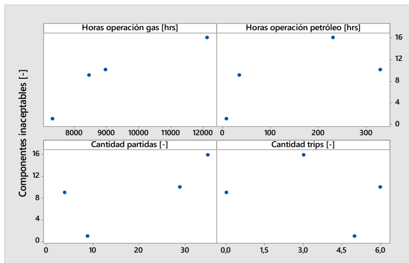
Figura 3.47: Gráficos de dispersión, cámara de combustión SI2.
