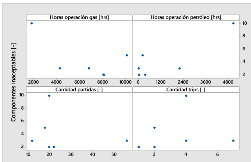
Figura 3.21: Gráficos de dispersión, datos cámara combustión SI1.
