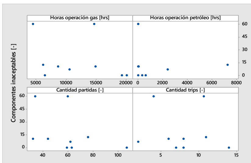
Figura 3.39: Gráficos de dispersión datos ring segment de 1° etapa SI1.
