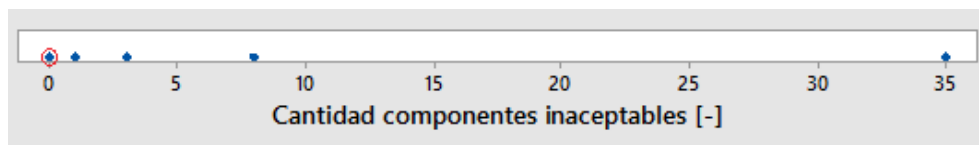
Figura 3.17: Gráfico de puntos ring segment de 1° etapa SI2.
