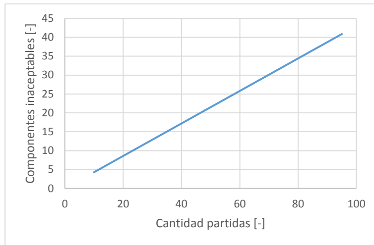
Gráfico 4.4: Curva teórica del modelo de regresión obtenido, alabe fijo de 1° etapa SI2.
