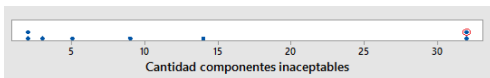
Figura 3.12: Gráfico de puntos alabe fijo de 2° etapa SI1
