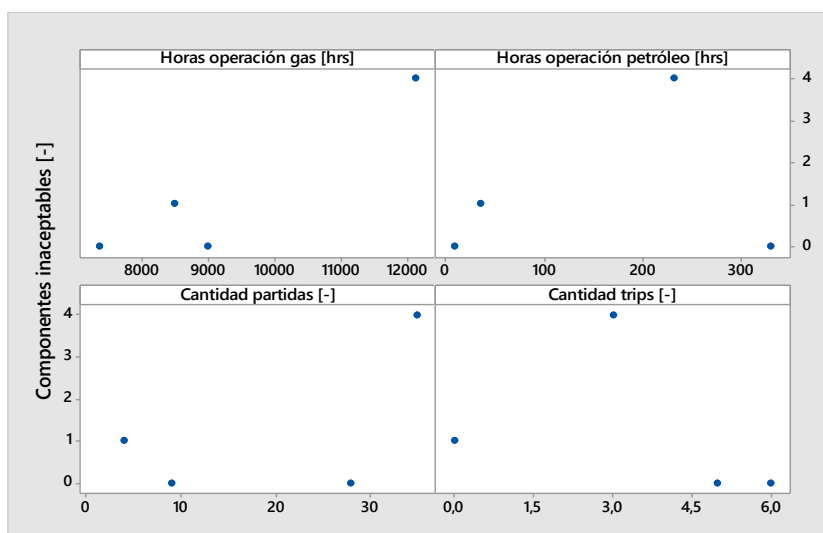
Figura 3.43: Gráficos de dispersión tobera piloto gas SI2.
