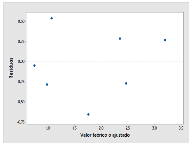
Gráfico 3.2: Residuos v/s valor teórico o ajustado del modelo, alabe fijo de 2° etapa SI1.
