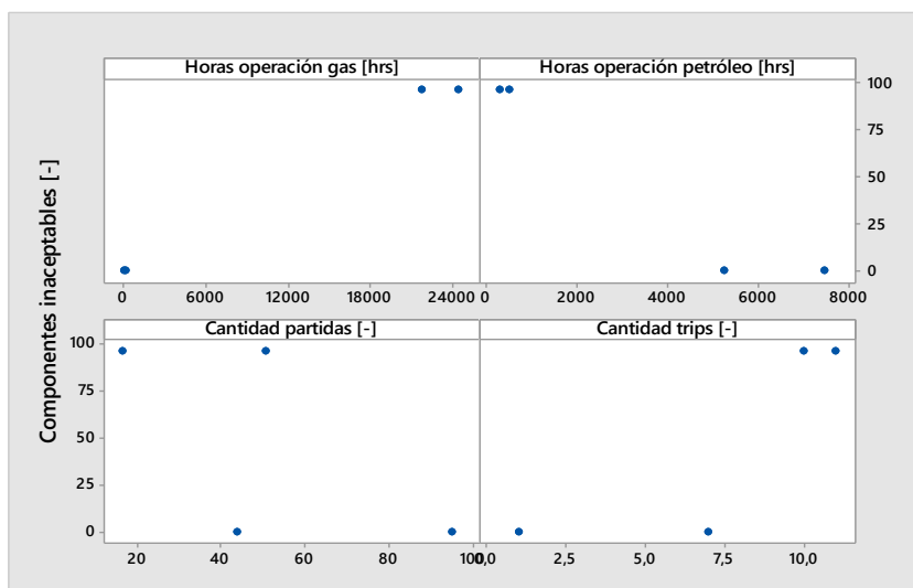
Figura 3.53: Gráficos de dispersión, alabe móvil de 1° etapa SI2.
