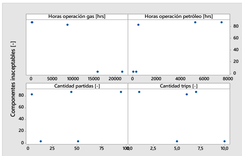
Figura 3.55: Gráficos de dispersión, alabe móvil de 2° etapa SI2.
