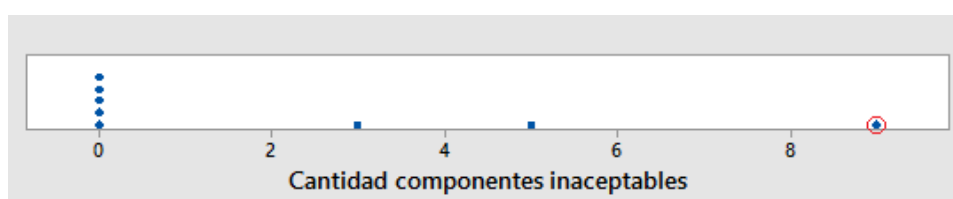
Figura 3.9: Gráfico de puntos tobera piloto combustible (gas, petróleo) SI1.
