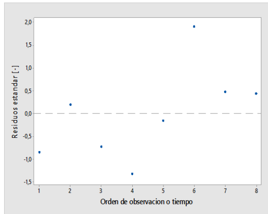
Gráfico 3.4: Residuos estándar v/s orden de observación, alabe móvil de 3° etapa SI1.
