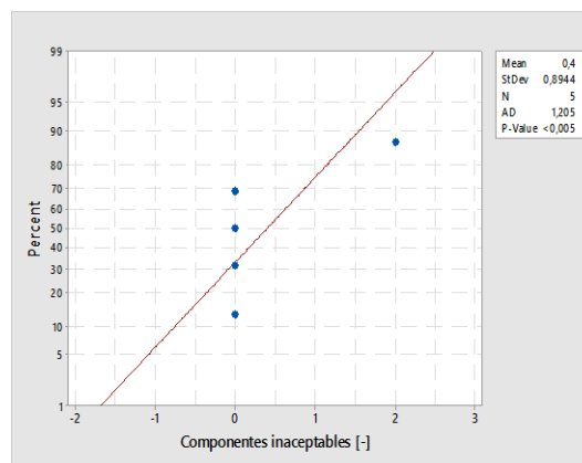
Gráfico 3.6: Probabilidad normal y estadístico AD para Componentes inaceptables, tobera piloto principal SI2.
