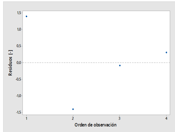
Gráfico 3.15: Gráfico de residuos estándar v/s orden de observación, alabe móvil de 1° etapa SI2.
