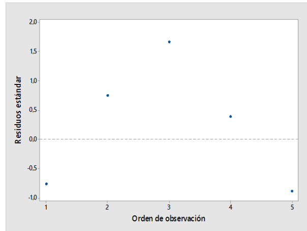
Gráfico 3.12: Residuos estándar v/s orden de observación, alabe fijo de 1° etapa SI2.
