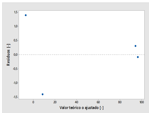
Gráfico 3.14: Residuos v/s valor teórico o ajustado del modelo, alabe móvil de 1º etapa SI2.
