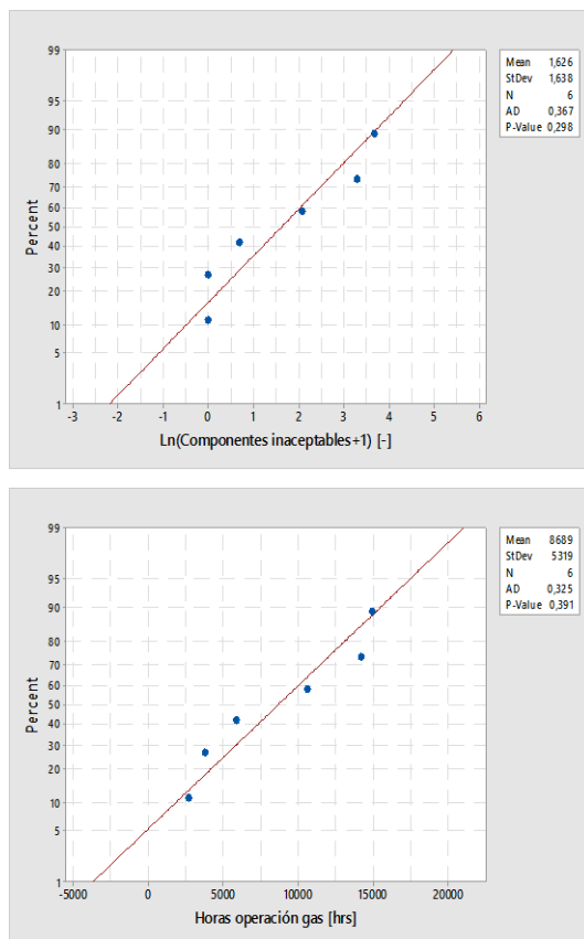
Figura 3.27: Gráfico de probabilidad normal y estadístico AD para variable Ln(Componentes inaceptables) (izquierda), y Horas operación gas (derecha), alabe fijo de 1° etapa SI1.
