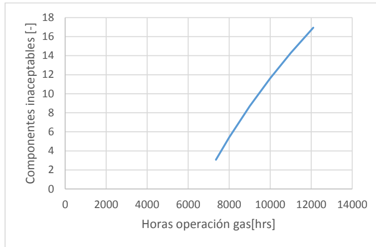
Gráfico 4.1: Curva teórica del modelo de regresión obtenido, cámara de combustión SI2.
