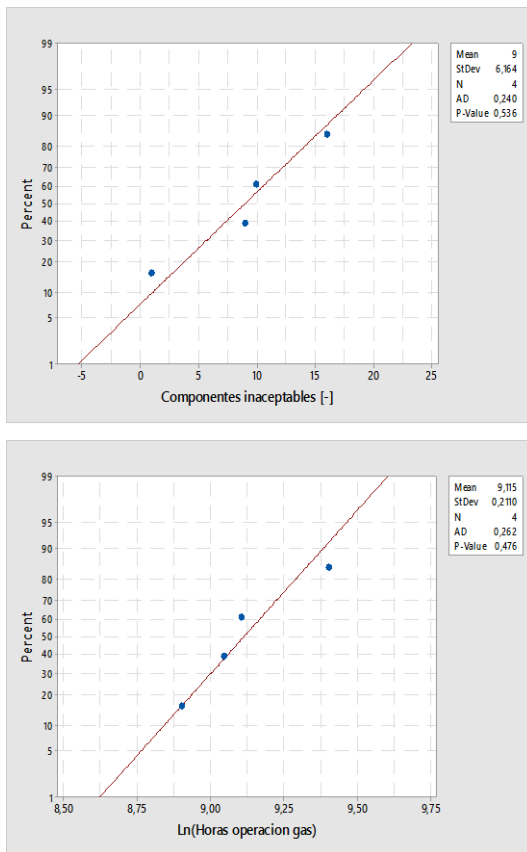
Figura 3.48: Gráficos de probabilidad normal y estadístico AD para Componentes inaceptables (izquierda) y Ln(Horas operación gas) (derecha), cámara de combustión SI2.
