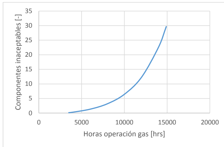
Gráfico 4.3: Curva teórica del modelo de regresión obtenido, alabe fijo de 1º etapa SI1.
