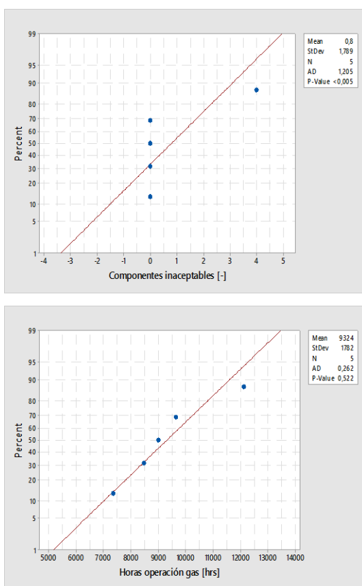
Figura 3.46: Gráficos de probabilidad normal y estadístico AD para Componentes inaceptables (izquierda) y Horas operación gas (derecha), tobera piloto petróleo SI2.
