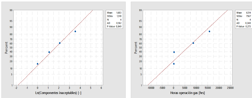
Figura 3.57: Gráficos de probabilidad normal y estadístico AD para variables Ln(componentes inaceptables) (izquierda) y Horas operación gas (derecha), ring segment de 1° etapa SI2.
