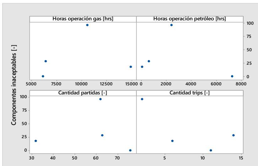
Figura 3.30: Gráficos de dispersión de datos, alabe móvil de 1° etapa SI1.
