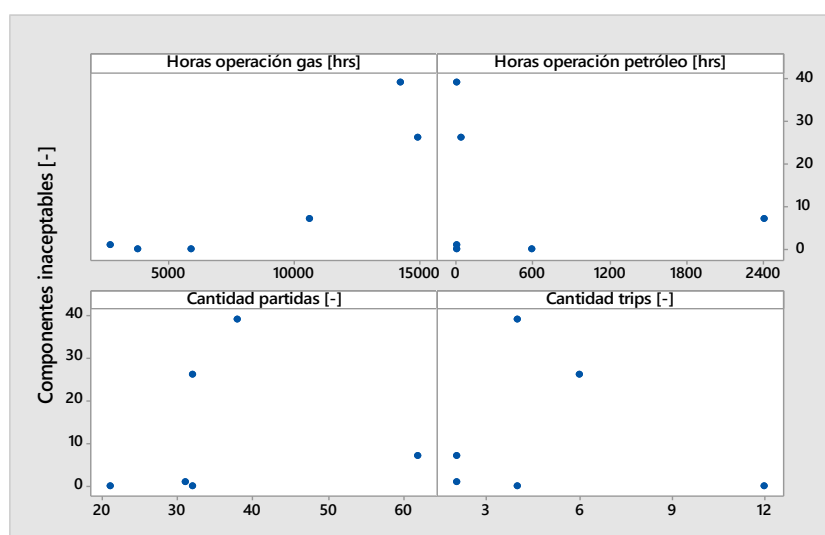
Figura 3.26: Gráficos de dispersión datos alabe fijo de 1° etapa SI1.
