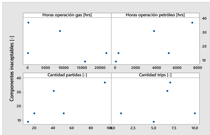
Figura 3.50: Gráficos de dispersión alabe fijo de 1° etapa SI2.
