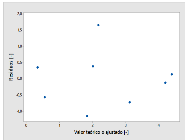
Gráfico 3.3: Residuos v/s valor teórico o ajustado del modelo obtenido, alabe móvil de 3° etapa SI1.
