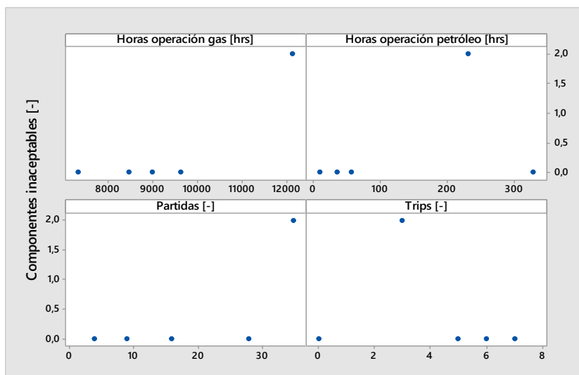
Figura 3.42: Gráficos de dispersión tobera piloto principal SI2.
