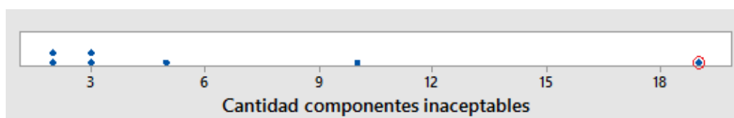
Figura 3.10: Gráfico de puntos cámara de combustión SI1
