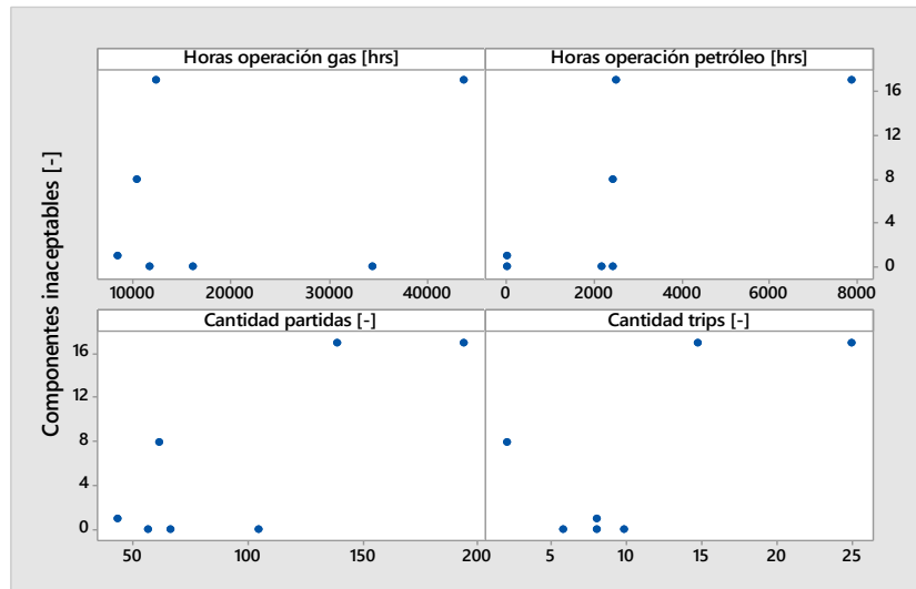
Figura 3.35: Gráficos de dispersión datos alabe móvil de 4° etapa SI1.
