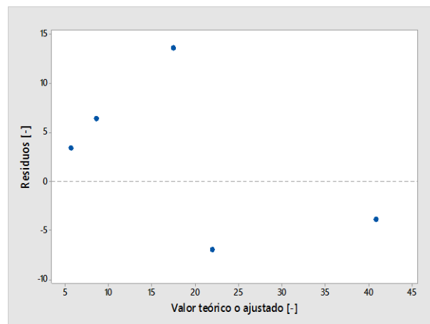
Gráfico 3.11: Residuos v/s valor teórico o ajustado del modelo, alabe fijo de 1° etapa SI2.
