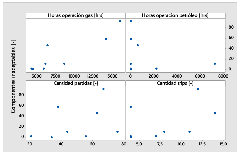
Figura 3.32: Gráficos de dispersión datos alabe móvil de 3° etapa SI1.
