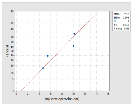
Gráfico 3.13: Grafico de probabilidad normal para variable \text{Ln}(\text{Horas operación gas}) , alabe móvil de 1° etapa SI2.
