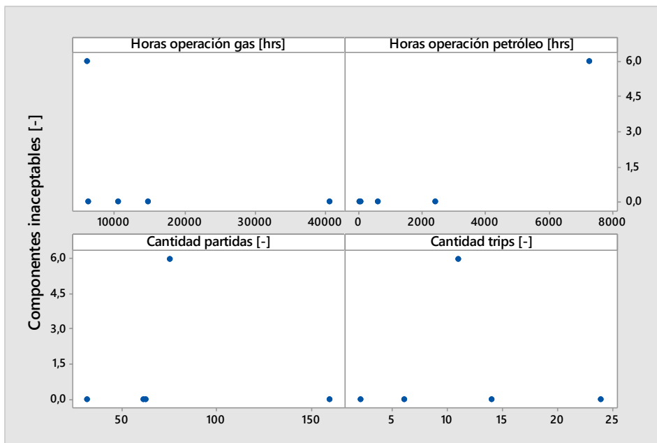
Figura 3.40: Gráficos de dispersión datos ring segment de 2° etapa SI1.
