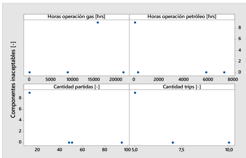
Figura 3.52: Gráficos de dispersión, alabe fijo de 2° etapa SI2.
