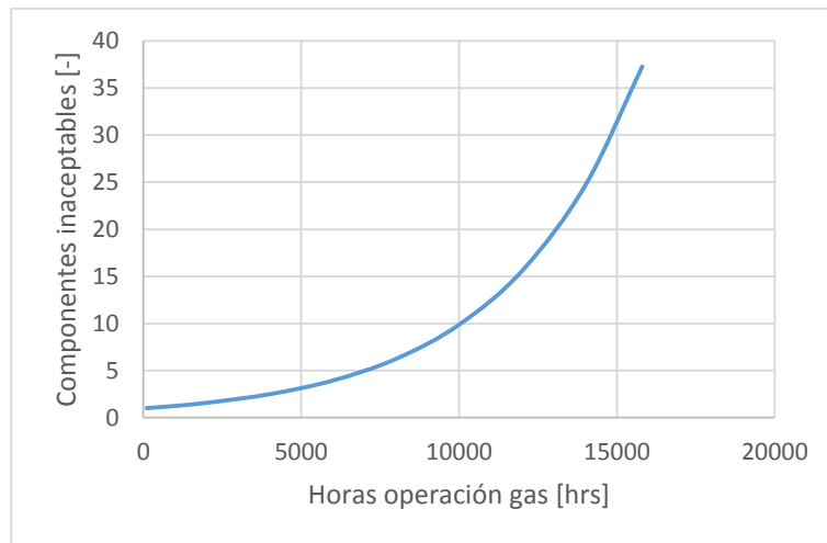
Gráfico 4.9: Curva teórica del modelo de regresión obtenido, ring segment de 1° etapa SI2.
