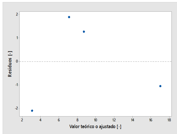
Gráfico 3.9: Residuos v/s valor teórico o ajustado, cámara de combustión SI2.
