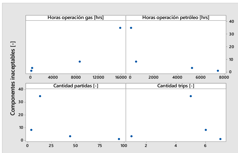
Figura 3.56: Gráficos de dispersión, ring segment de 1° etapa SI2.
