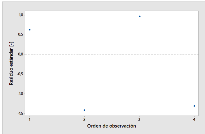
Gráfico 3.10: Residuo estándar v/s orden de observación, cámara de combustión SI2.
