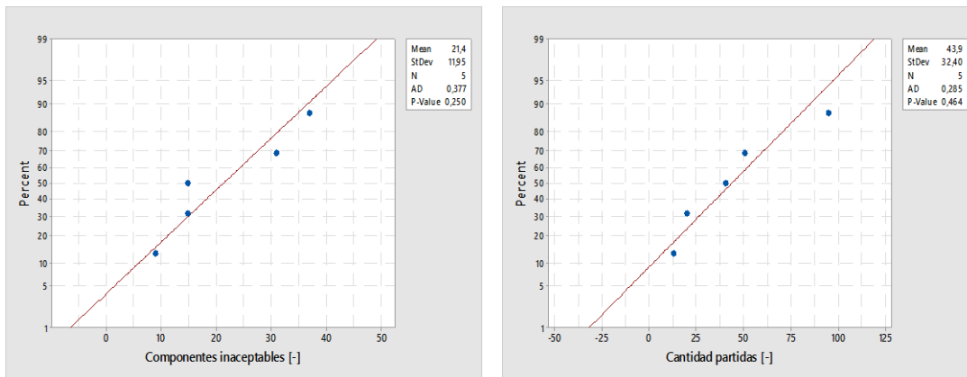
Figura 3.51: Gráficos de probabilidad normal y estadístico AD para Componentes inaceptables (izquierda) y Cantidad partidas (derecha), alabe fijo de 1° etapa SI2.
