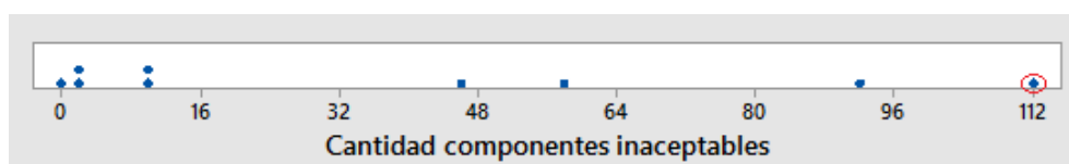
Figura 3.13: Gráfico de puntos alabe móvil de 3° etapa SI1
