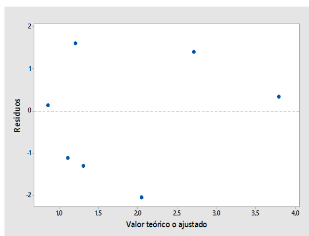
Gráfico 3.5: Residuos v/s valor teórico o ajustado del modelo, alabe móvil de 4° etapa SI1.
