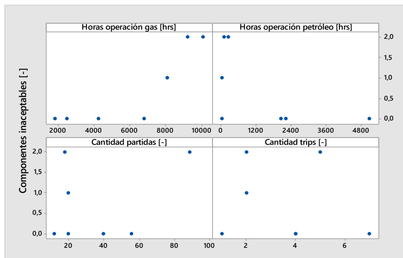
Figura 3.24: Gráficos de dispersión, datos pieza de transición SI1.
