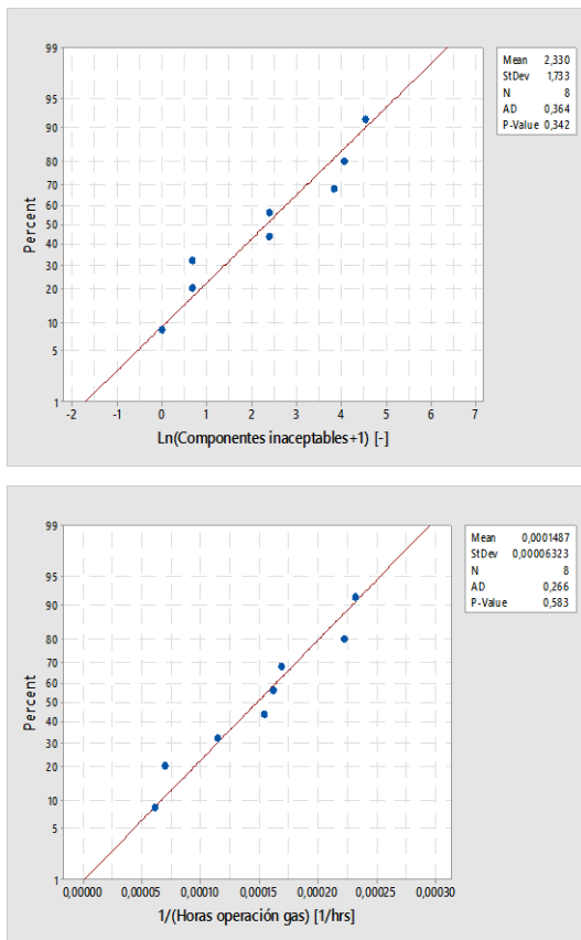
Figura 3.34: Gráfico de probabilidad normal y estadístico AD para Componentes inaceptable transformada (izquierda), y Horas operación gas transformada (derecha), alabe móvil de 3° etapa SI1.
