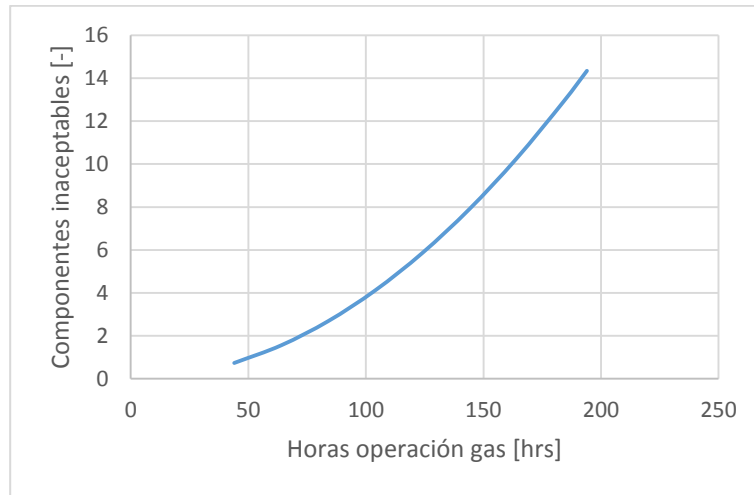
Gráfico 4.8: Curva teórica del modelo de regresión obtenido, alabe móvil de 4° etapa SI1.
