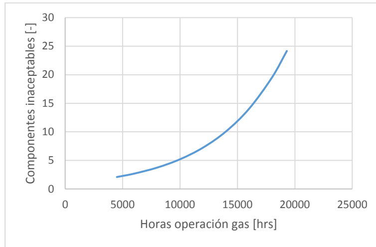
Gráfico 4.5: Curva teórica del modelo de regresión obtenido, alabe fijo de 2° etapa SI1.
