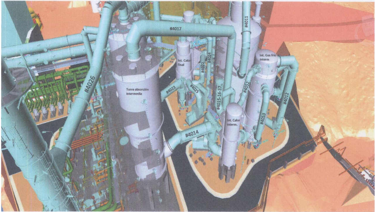
Figura 2-11. Planta Cap.4 con Líneas N°3
