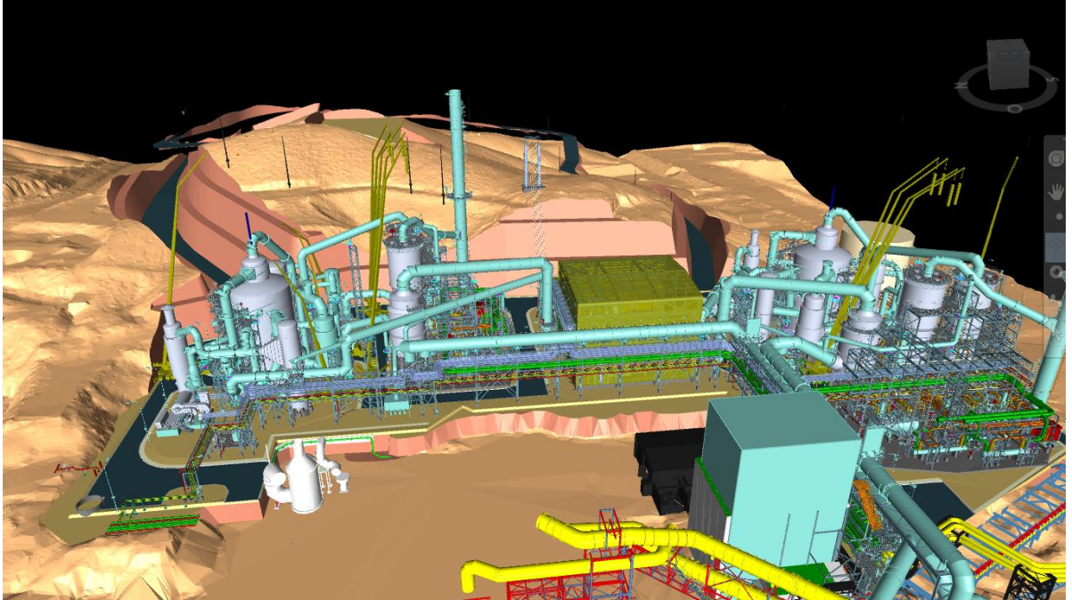
Figura 2-7. Planta de ácido doble absorción y doble contacto
