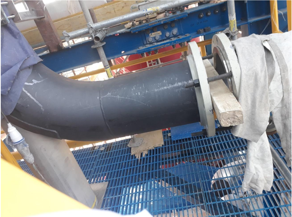
Figura 2-37 Unión flange en proceso
