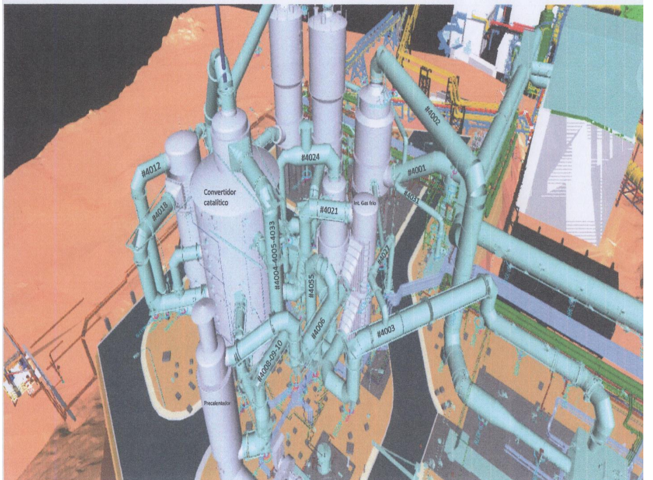
Figura 2-10. Planta Cap.4 con Líneas N°2
