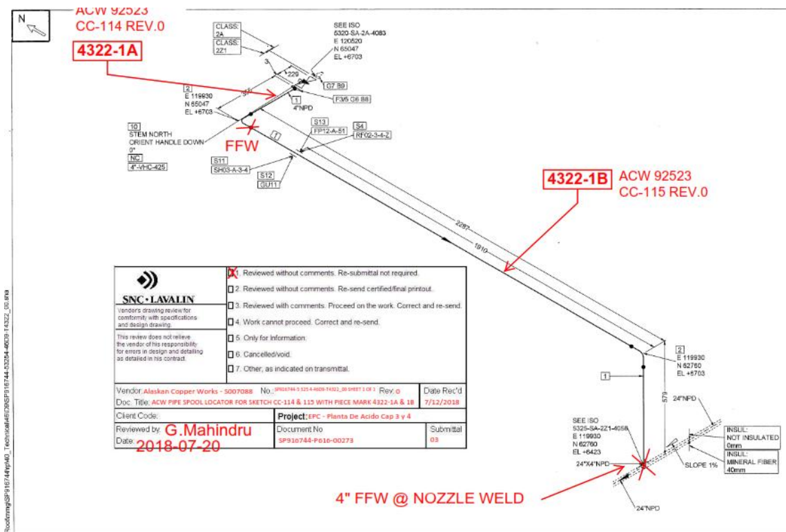
Figura 2-30 Plano Isométrico Línea 4322
