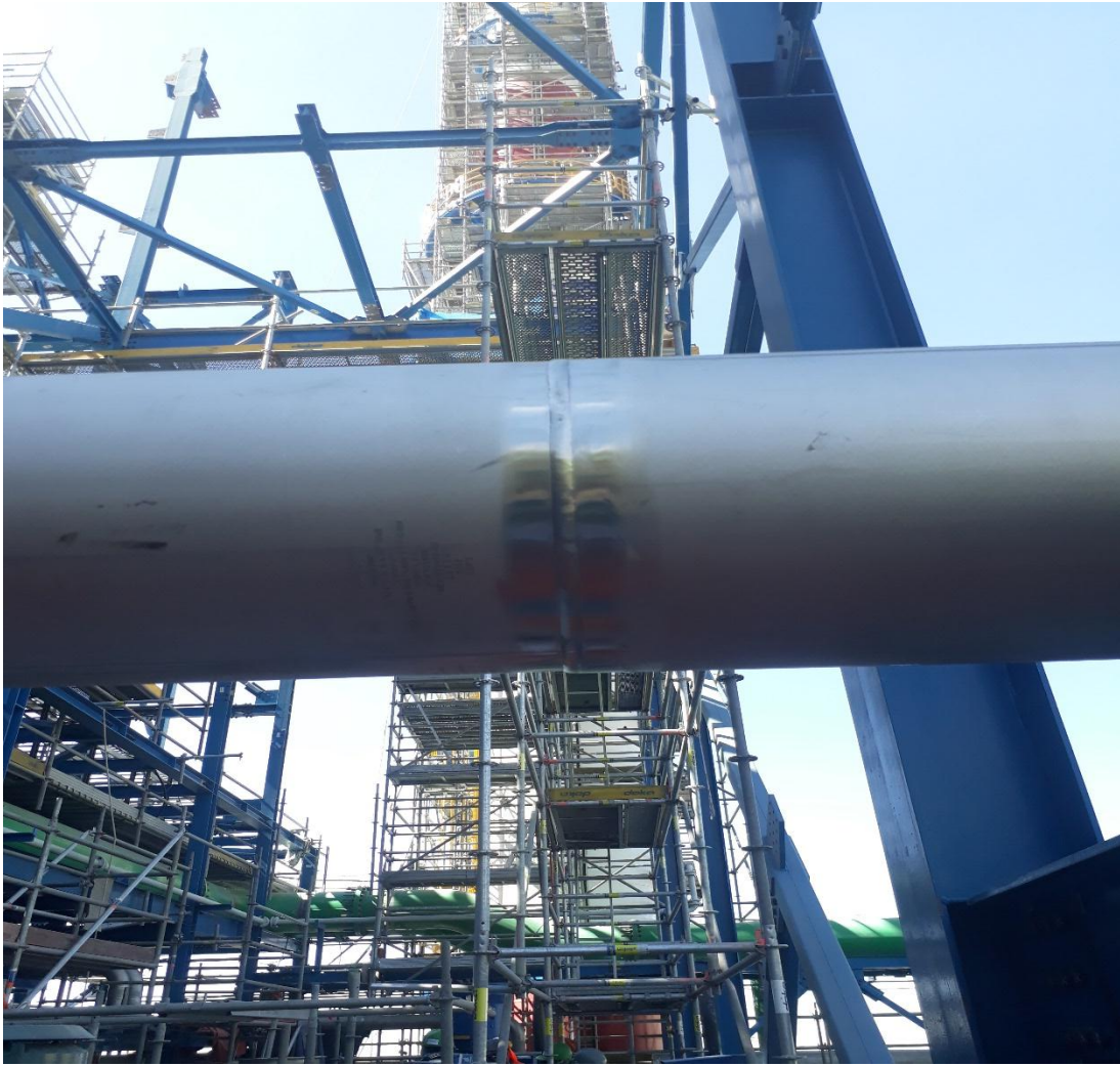
Figura 2-35 Unión BUTTWELD
