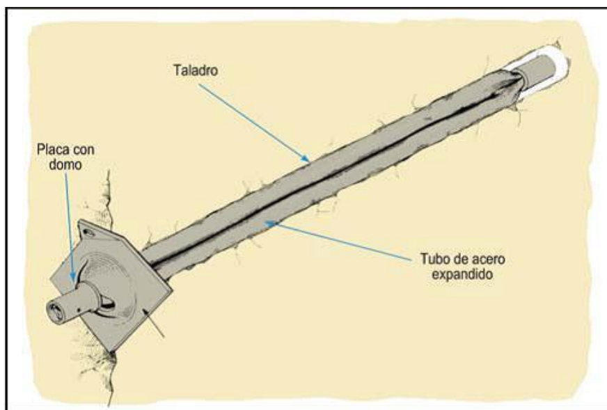
Figura 2-22 Perno Swellex, vista general.
