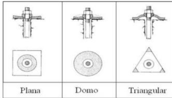
Figura 2-24 Tipos de planchuela.
