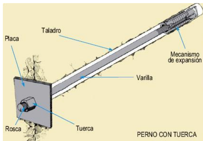
Figura 2-18 Perno con tuerca anclado mecánicamente.
