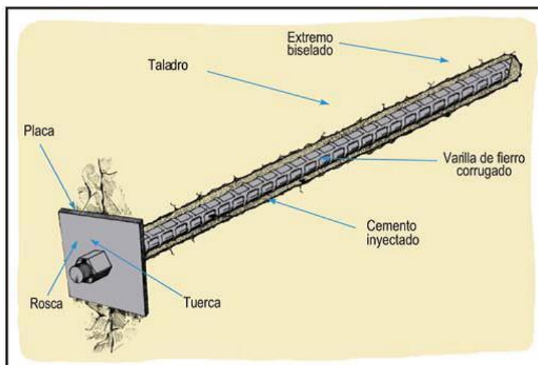
Figura 2-19 Perno con resina o lechada.
