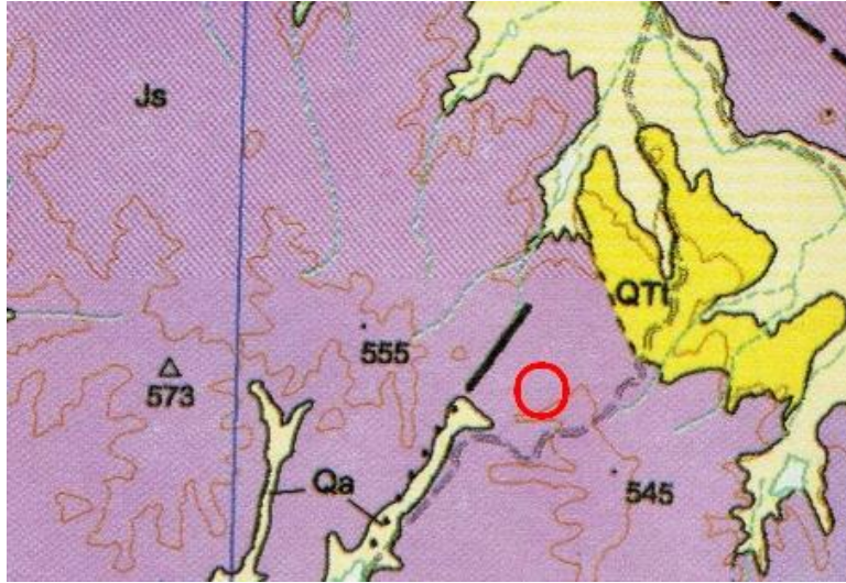
Fuente 4: Mapa geológico del área de Valparaíso-Curacaví 1996. Extraído Informe geológico mina
