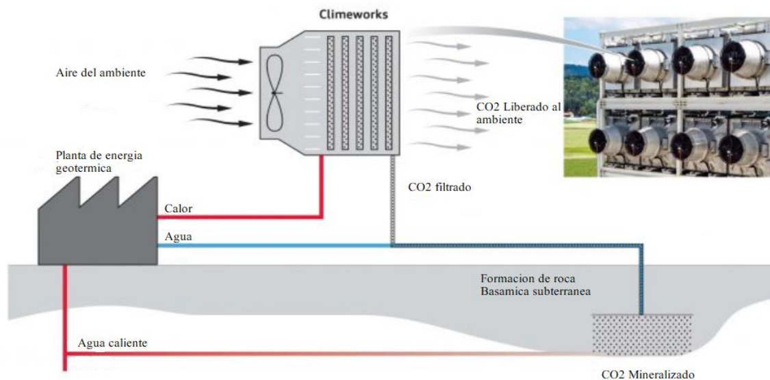
Diagrama de flujo 2 Proceso de captura CO2
