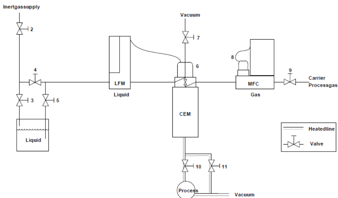
Figura 3.28: Esquema de funcionamiento del sistema.
