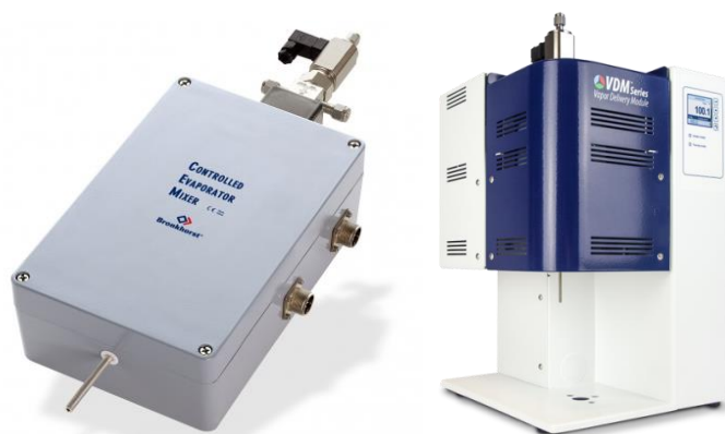
Figura 3.16: Módulos vaporizadores. Izquierda: Evaporador y mezclador controlado (CEM). Derecha: Módulo de suministro de vapor (VDM).
