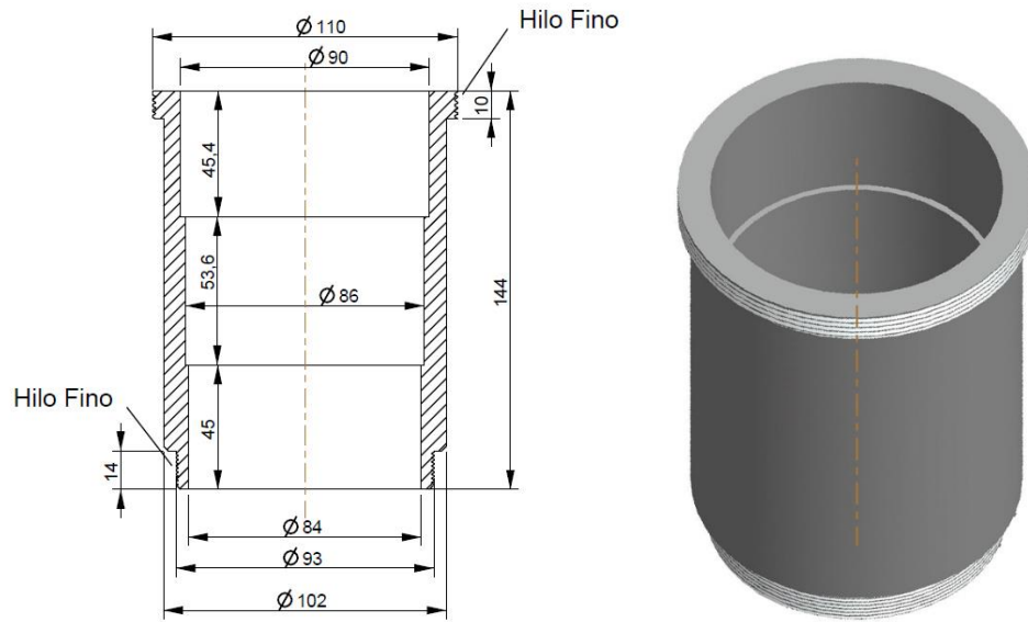
Figura 3.13: Diseño del tubo exterior del quemador.
