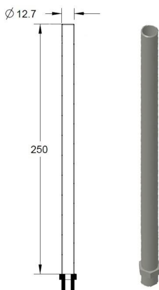
Figura 3.12: Diseño del tubo interior del quemador.
