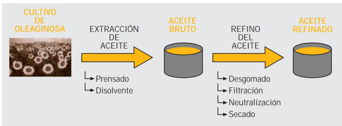
Figura 2.11: Proceso de obtención de aceite refinado.
