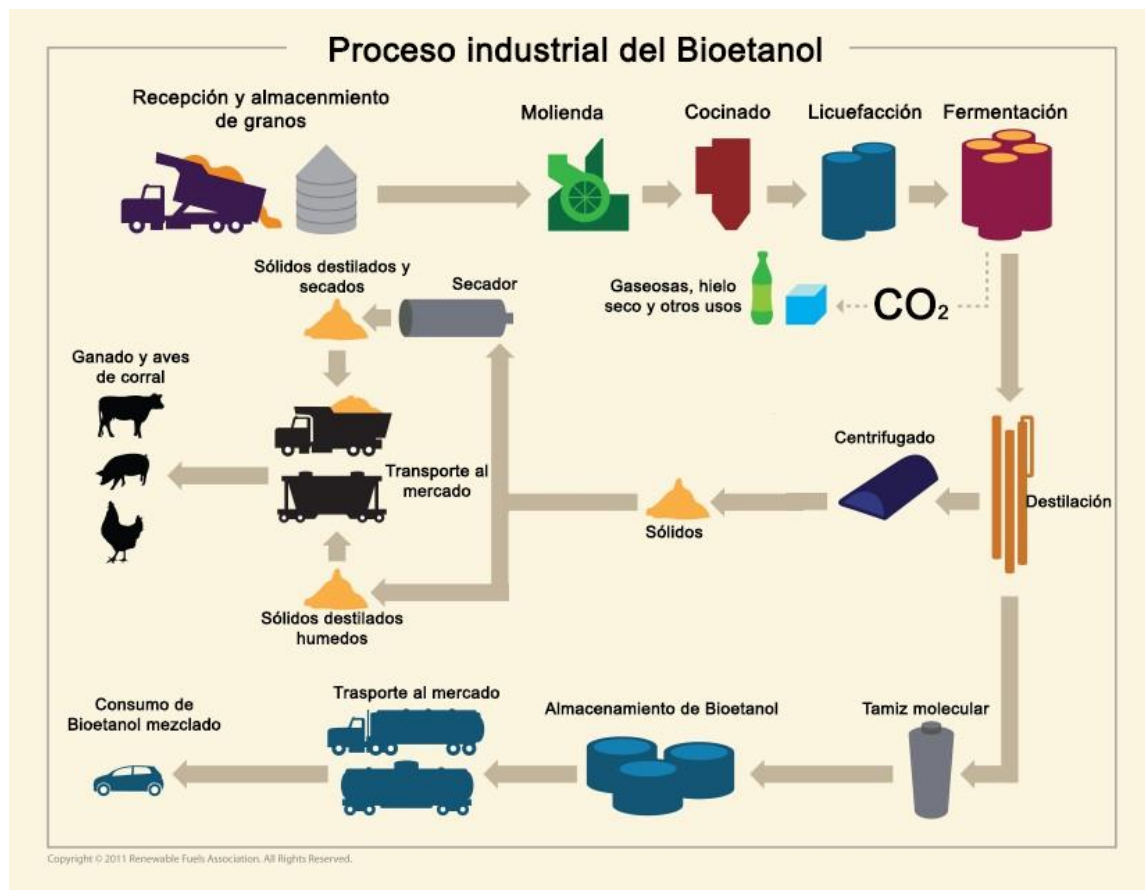
Figura 2.8: Proceso Industrial del bioetanol de maíz.
