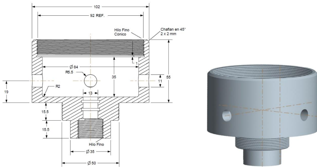
Figura 3.14: Diseño de la base del quemador.
