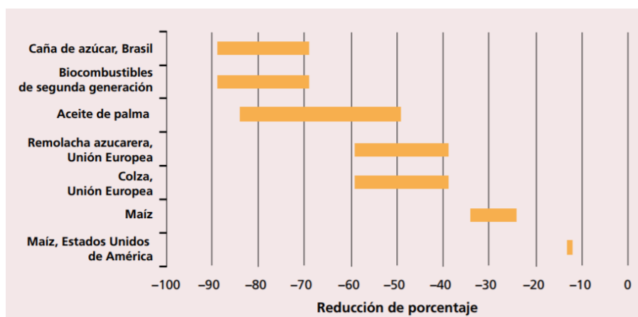
Figura 2.17: Reducción de gases de efecto invernadero en comparación con combustibles fósiles.
