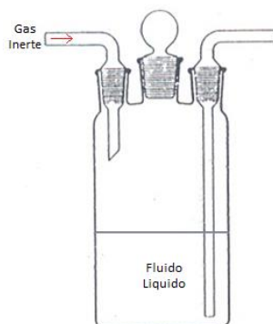
Figura 3.10: Funcionamiento del tanque presurizado.
