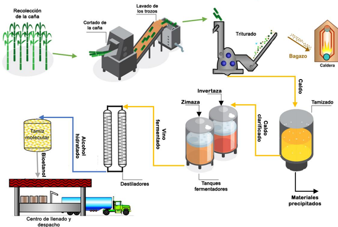
Figura 2.9: Proceso productivo de etanol de caña de azúcar.
