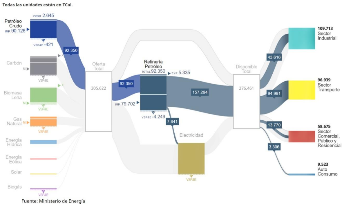
Figura 2.2: Diagrama Sankey de la oferta y demanda de petróleo en Chile, año 2015.
