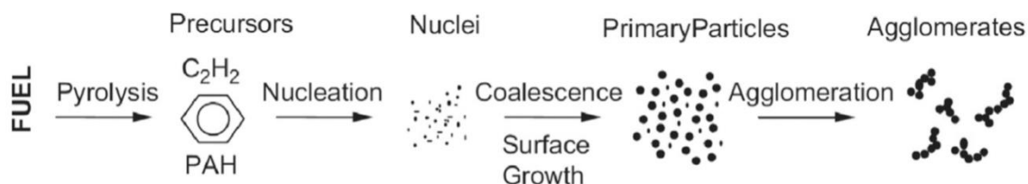
Figura 3.3: Procesos en la formación de hollín.
