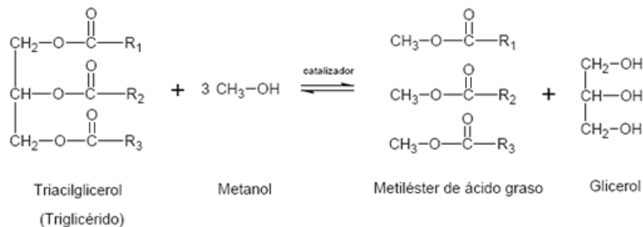
Figura 2.12: Reacción de transesterificación metílica.
