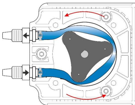
Figura 3.9: Esquema de una bomba peristáltica.
