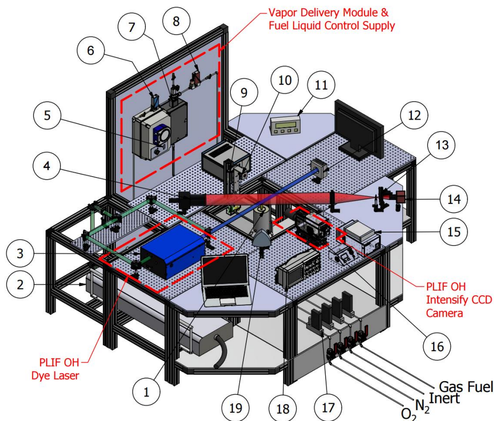
Figura 3.4: Esquema del montaje de dispositivo.
