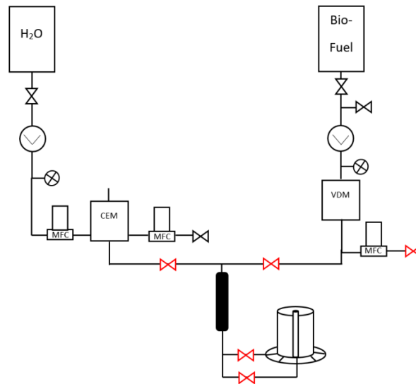
Figura 3.21: Diagrama del modelo 4.
