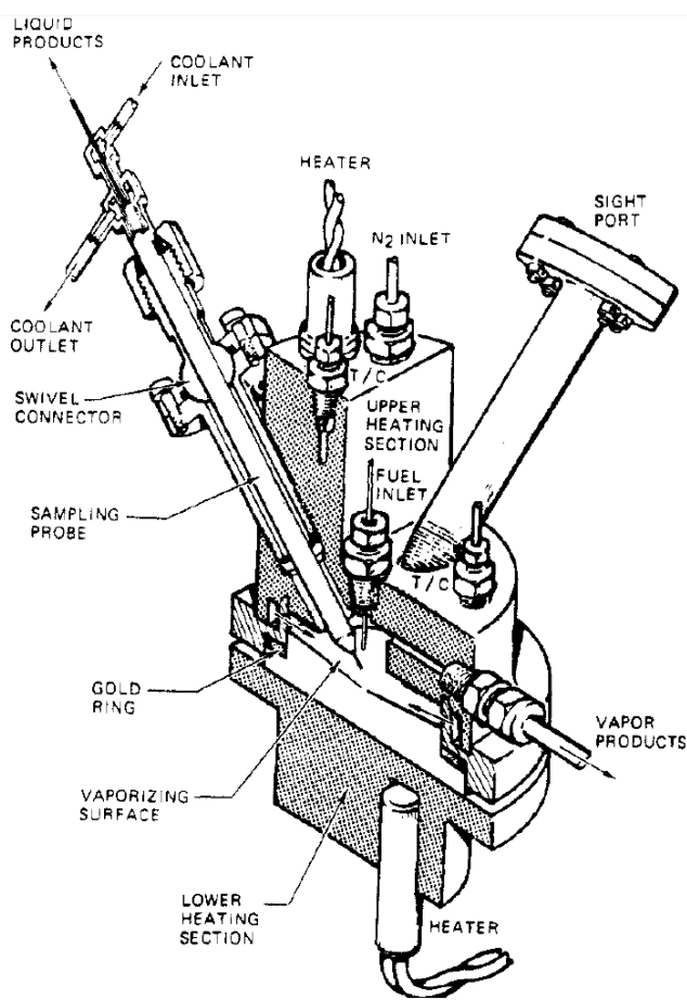
Figura 3.6: Diagrama del evaporador de placa caliente.
