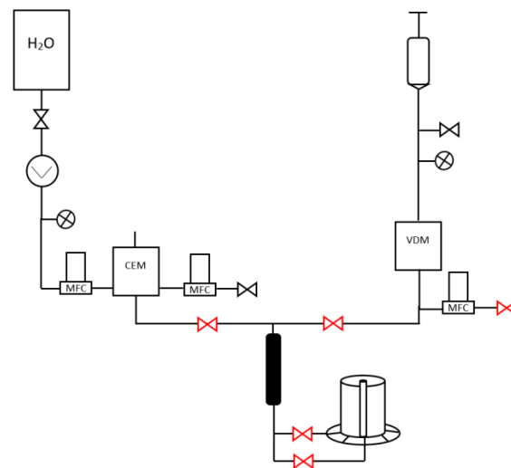
Figura 3.22: Diagrama del modelo 5.
