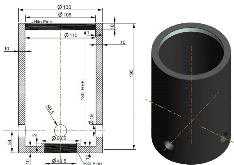
Figura 3.15: Diseño de la funda de aislación térmica para el quemador.
