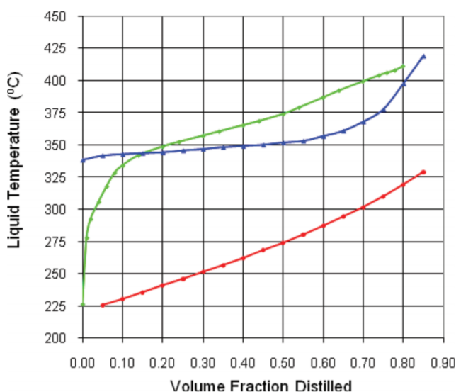
Figura 2.10: Curva de destilación para biodiésel de aceite de soja (verde) en comparación con las del biodiésel comercial (azul) y diésel N°2 (rojo).
