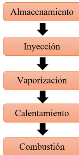
Figura 3.1: Diagrama de flujo del funcionamiento del dispositivo experimental.
