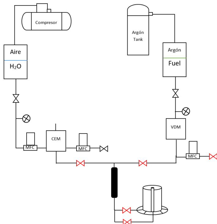
Figura 3.19: Diagrama del modelo 2.
