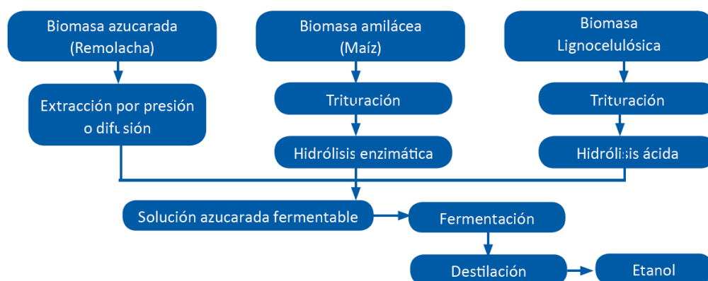
Figura 2.5: Rutas para obtener etanol desde distintas materias primas.
