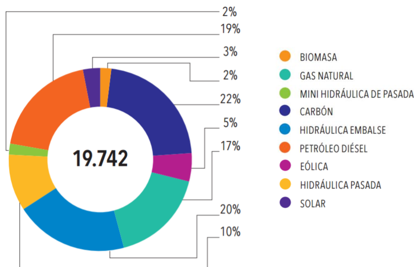
Figura 2.1: Capacidad instalada en MW al año 2015 y su descomposición.
