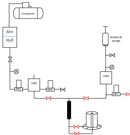
Figura 3.23: Diagrama del modelo 6.
