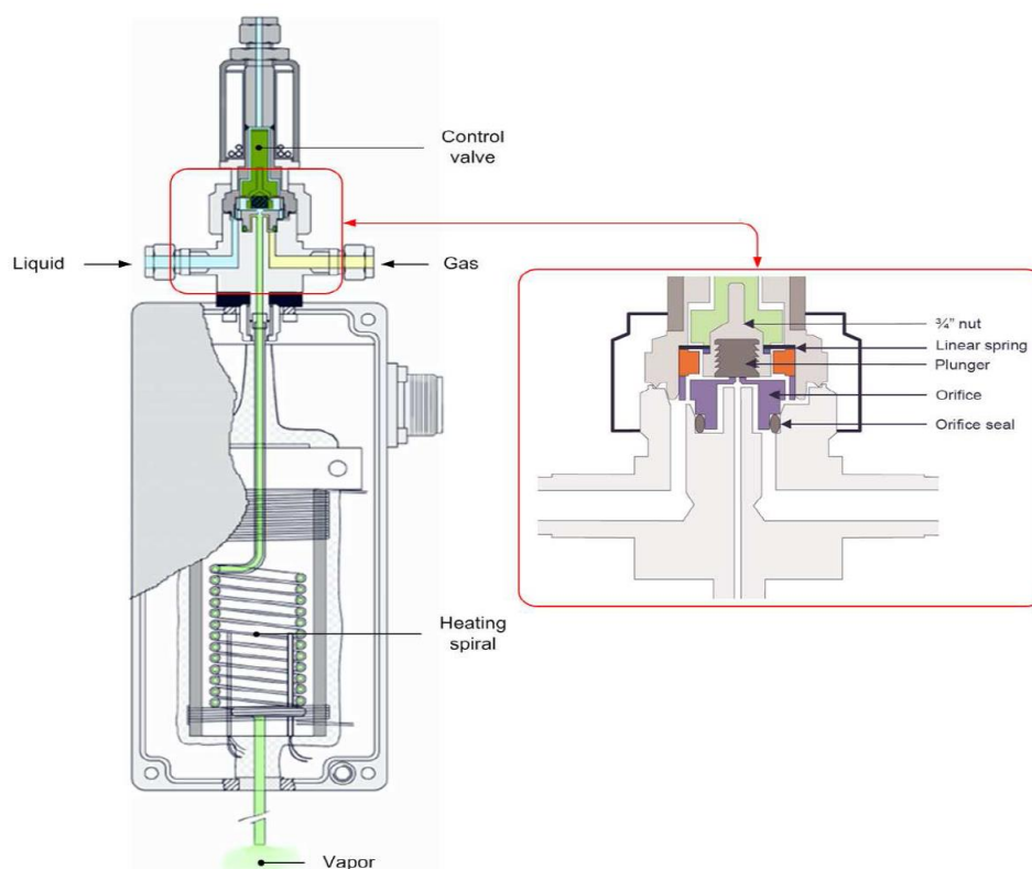
Figura 3.7: Diagrama del Mezclador y Vaporizador Controlado (CEM).
