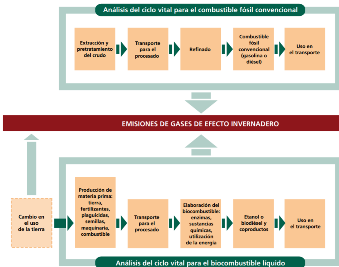
Figura 2.16: Desglose del ACV para combustibles fósiles y biocombustibles líquidos.
