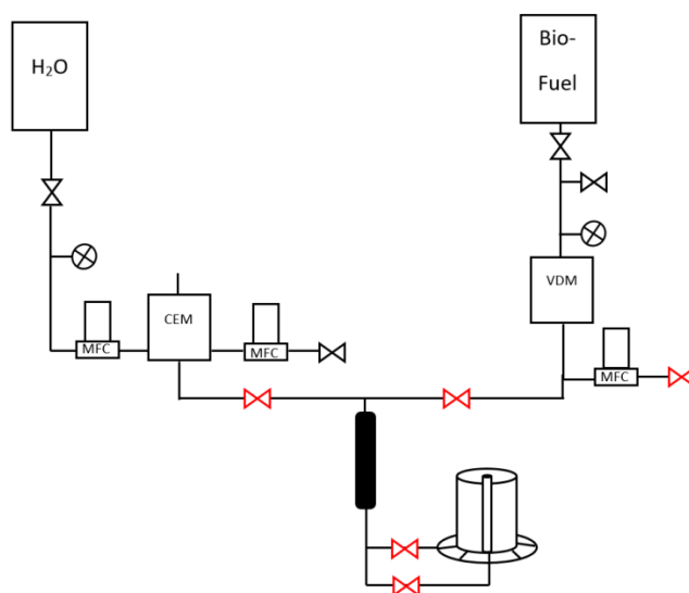
Figura 3.18: Diagrama del modelo 1.
