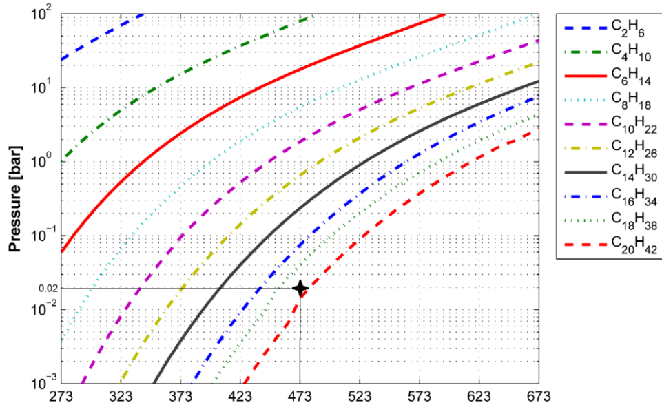
Figura 3.17: Presión de vapor para distintos hidrocarburos. Fuente: Bronkhorst.
