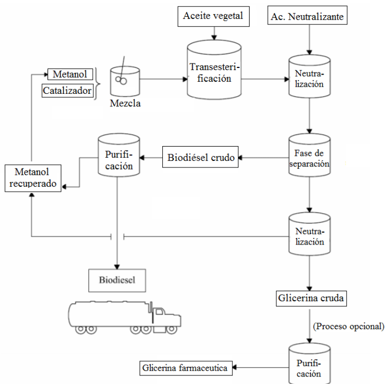
Figura 2.15: Proceso productivo para la obtención de biodiésel.
