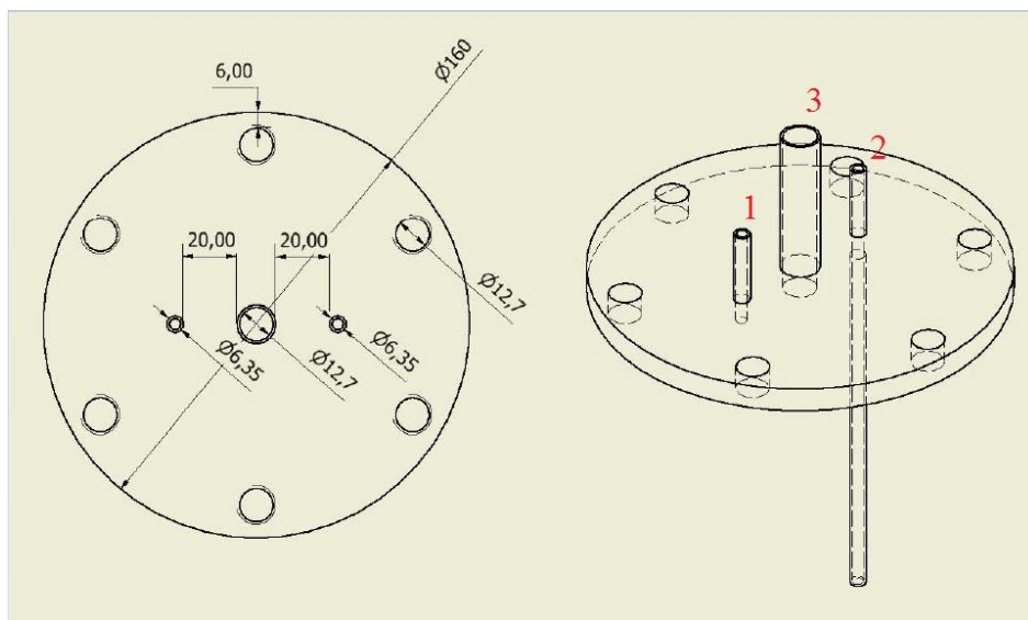
Figura 3.25: Diseño de la tapa del tanque presurizado.
