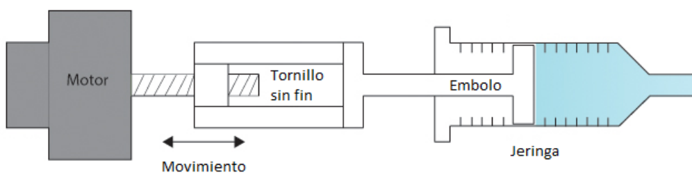
Figura 3.8: Funcionamiento de la bomba de jeringa.
