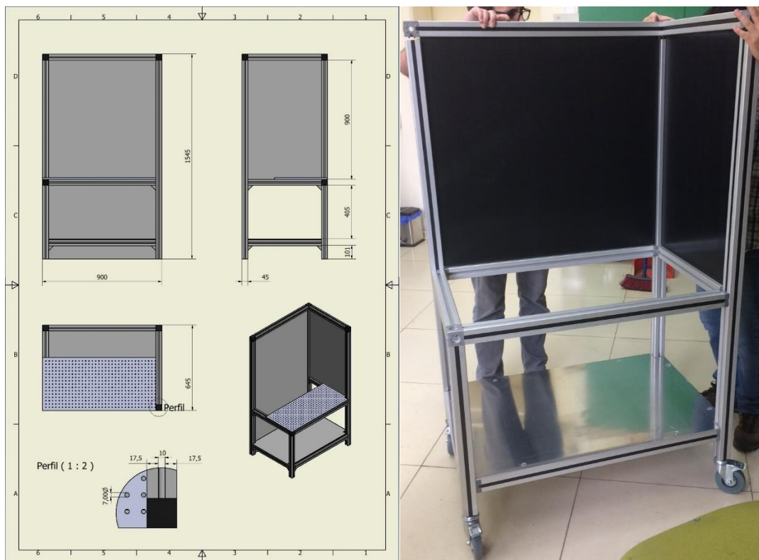
Figura 3.11: Dibujo isométrico del banco experimental (izquierda) y construcción (derecha).
