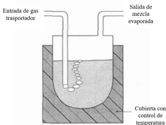
Figura 3.5: Diagrama de evaporador por sistema de burbujeo.
