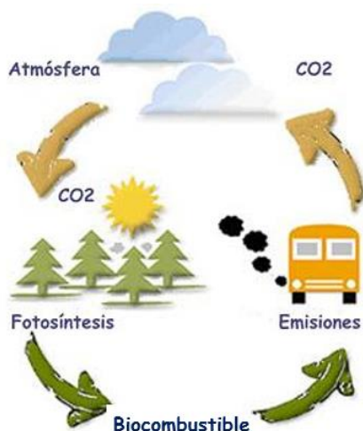
Figura 2.4: Ciclo de absorción y emisión de dióxido de carbono.
