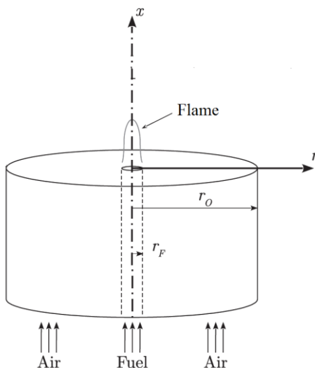
Figura 3.2: Esquema de una llama de difusión producida en co-corriente.
