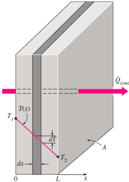
Fig. 6 En condiciones estacionarias, la distribución de temperatura en una pared plana es una línea recta.
