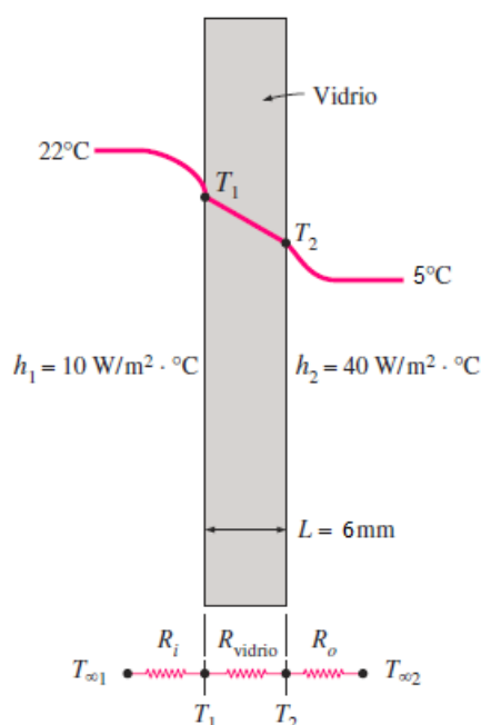
Fig. 9 Esquema de Ventana de vidrio simple
