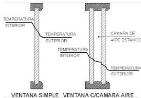
Fig. 3 Tipos de aislación térmica para ventanas (doble vidrio y cámara de aire)
