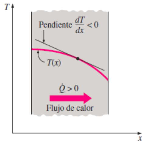
Fig. 5 El gradiente de temperatura dT/dx corresponde a la pendiente de la curva de temperatura en el gráfico T-x.
