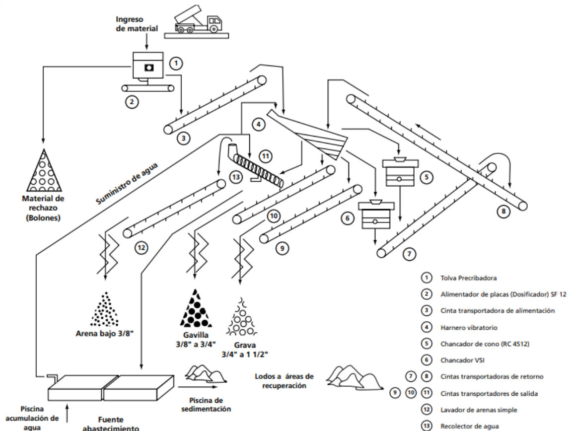
Figura 1-6. Plata procesamiento de áridos fuente: Industria del árido en Chile tomo I, CChC
