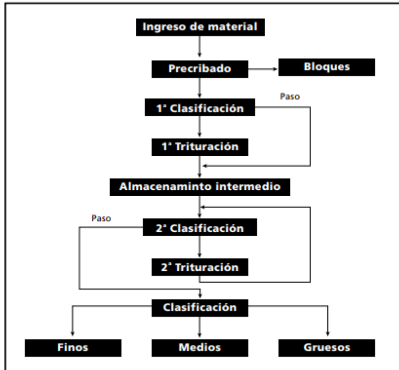
Figura 1-4. Operación proceso en seco
