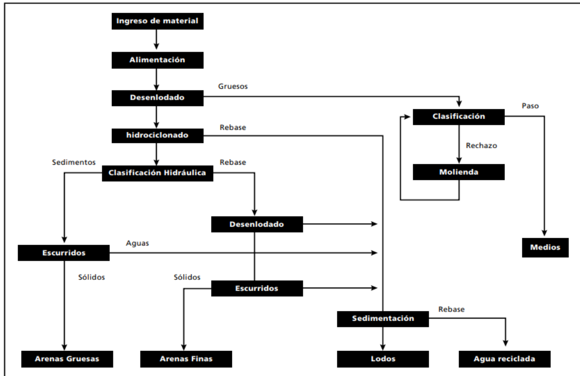
Figura 1-5. Operación proceso húmedo
