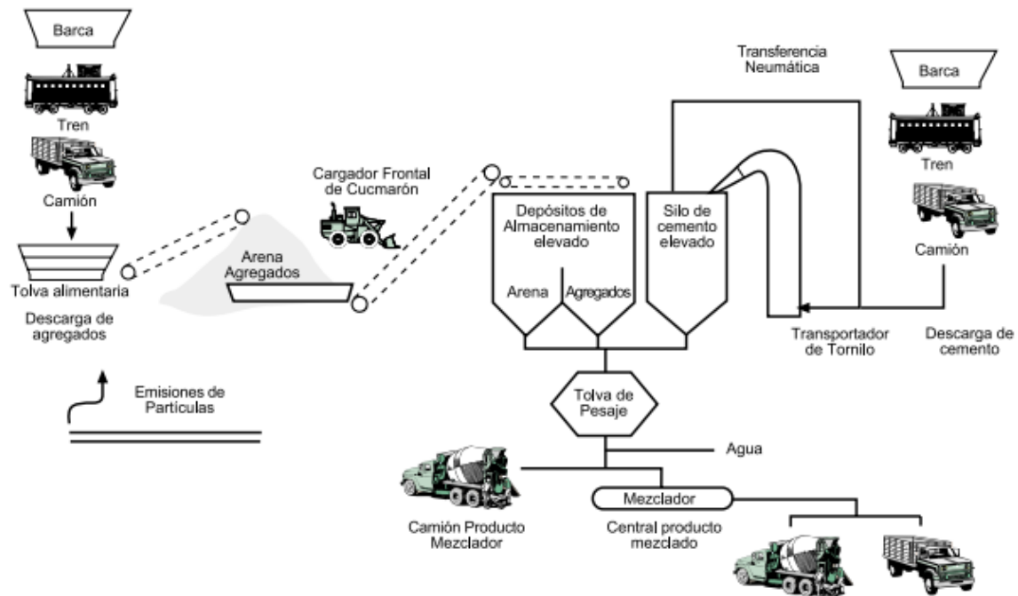
Figura 1-7. Proceso de producción de hormigón premezclado.
