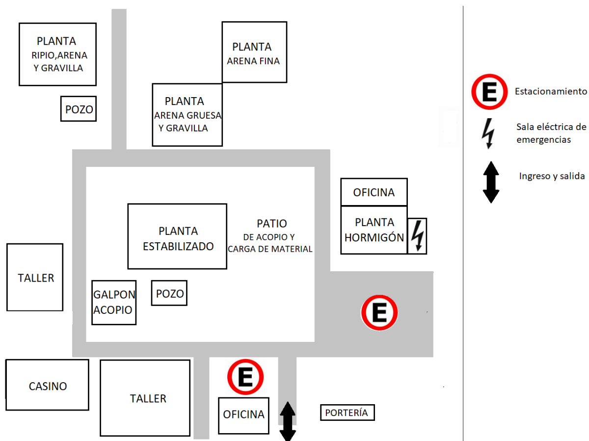
Figura 1-2. Layout instalaciones planta de áridos y hormigones
