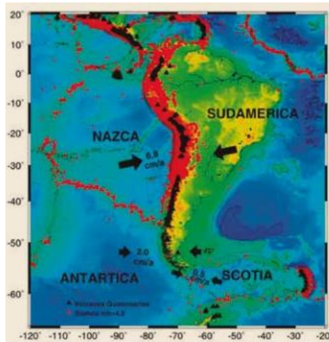
Figura 2-1. Marco Tectónico en Chile.
